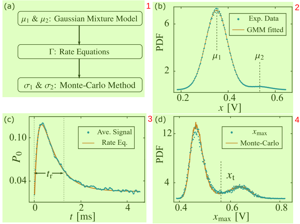
图 3.2 (a) 从单发读出的信号中提取参数的三个步骤：(b) 使用高斯混合模型（Gaussian mixture model, GMM）方法，对读取信号中所有数据的概率密度分布函数（PDF）进行拟合，可以提取出图 3.1c 中高电平和低电平信号的均值 \mu_1, \mu_2 。对于提取到的标准差，由于线路中滤波的影响，并不能直接用于 Monte-Carlo 方法生成模拟数据；(c) 使用速率方程计算信号均值 \bar{x} 随读取阶段时间 t_{\text{read}} 的变化，计算时，需要用第一步中提取的 \mu_1, \mu_2 对 \bar{x} 进行归一化，得到激发态电子的平均概率随读取时间的变化。图中 \bar{x} 形成鼓包形状，这是因为处于激发态的电子在读取阶段开始后，跳出量子点的隧穿速率为 \Gamma_{\uparrow}^{\text{out}} ，跳出量子点后，源漏中的电子又会以隧穿速率 \Gamma_{\downarrow}^{\text{out}} 跳进量子点中；(d) 利用第二步中提取的 \Gamma_{\uparrow, \downarrow}^{\text{in, out}} ，我们可以用 Monte-Carlo 方法生成无噪声且归一化的模拟隧穿信号；然后我们使用 \mu_1, \mu_2 将归一化的信号转换成无噪声的电平信号，再添加白噪声以模拟环境噪声，最后用数字滤波器来模拟 8 阶贝塞尔低通滤波，生成最终的模拟信号。我们对读取信号中每一次读取信号最大值 x_{\text{max}} 的概率密度分布函数进行拟合，得到读取信号滤波前的标准差 \sigma_1, \sigma_2 。至此我们完成了从单发读出信号中提取参数的所有步骤。
