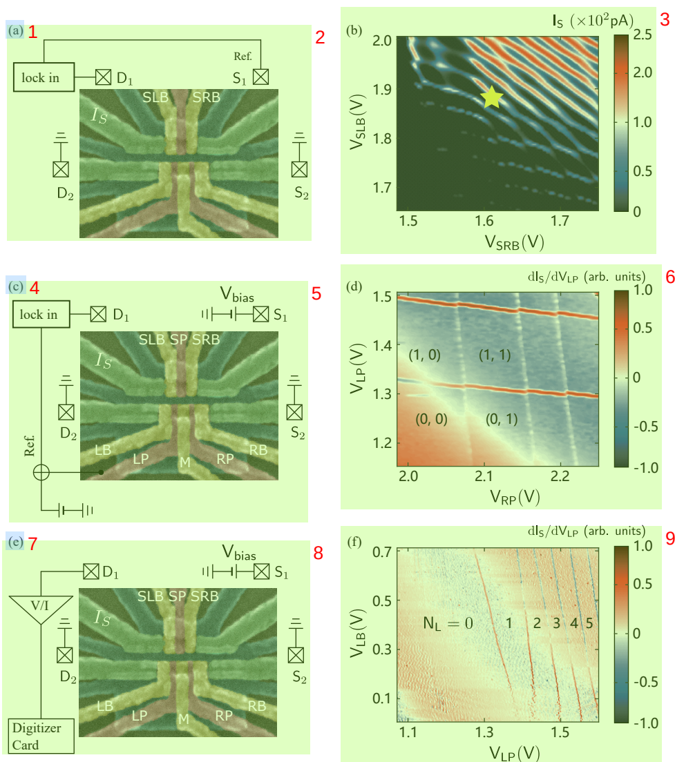
图 2.7 三种不同的室温测量线路 (a) 使用锁相放大器测量单电子晶体管的线路示意图; (b) 由 (a) 图中线路测量得到的单电子晶体管库仑峰, 图中黄色星号表示单电子晶体管用于探测量子点中电荷数的最佳工作位置; (c) 使用锁相放大器通过单电子晶体管探测量子点电荷数的线路示意图, 注意此时 lock-in 的参考信号输出端接在量子点的势垒电极上, 信号输入接在单电子晶体管的漏极; (d) 扫描量子点势垒电极得到的电荷稳定图; (e) 使用电流-电压放大器测量量子点的线路示意图; (f) 扫描量子点势垒电极得到的电荷稳定图。
