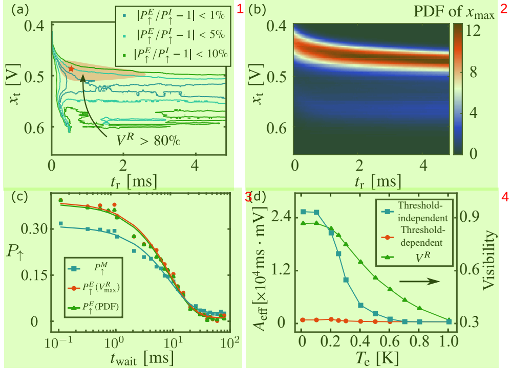
图 3.5 (a) 期望概率 P^E 与读取阶段初始概率 P^I 的偏差关于时间窗口和电压阈值的轮廓图。 5 图中蓝色、青色和绿色实线分别为 |P^E/P^I - 1| < 1\% 、 5\% 和 10\% 区域的轮廓线。作为对比，我们用红色星形符号标识出了 V_{\max}^R 的位置，并用粉色阴影区域标识出了 V^R > 80\% 的区域；(b) 不同时间窗口下，读取信号最大值的分布相图。图中可以明显看出信号最大值分布中的双峰位置随着时间窗口增大而向增大的方向平移。图中双峰之间的低谷区域轮廓和 (a) 图中的青色轮廓线相近；(c) 采用阈值无关单发读出方法处理实验数据，我们比较了在 V_{\max}^R 处（红色圆点）和同样时间窗口下读取信号最大值分布的双峰之间最小值位置处（绿色三角形）的 P^E ，并用指数衰减函数拟合，发现两者差异较小；与用传统方法处理得到的测量概率 P^M （蓝色方形）相比，采用阈值无关单发读出方法处理得到的 P^E 更加接近目标值 P^I 、且暗记数较小；(d) 蓝色方形和红色圆形分别表示不同电子温度下阈值无关单发读出方法和传统方法的有效参数空间大小 A_{\text{eff}} ，绿色三角形为该温度下的最大读取可见度。
