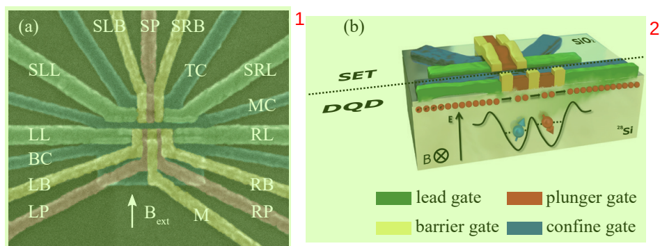
图 1.4 (a) 硅量子点中双量子点 (Double quantum dots, DQD) 结构的扫描电子显微镜 (SEM) 照片, 两个量子点分别形成在电极 LP 和 RP 下方, 通过调节电极 M 的电压, 可以控制电子在两个量子点之间的隧穿速率; (b) 双量子点结构的截面示意图, 通过调节中间五根电极的电压, 可以在衬底中形成双量子点结构的势阱。以虚线为界, 上方的电极则形成了单电子晶体管 (Single electron transistor, SET) 结构, 用于探测虚线下方双量子点中的电子数目。
