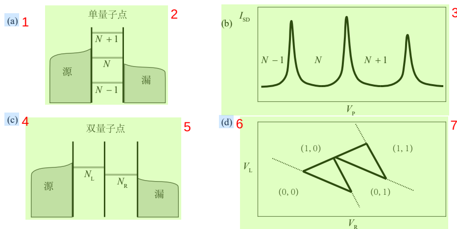
图 1.5 (a) 硅量子点中单量子点能级结构的示意图；(b) 库仑阻塞示意图。当单量子点中的能级进入源漏之间的偏压窗口时，会在源漏之间形成电流 I_{SD} ；(c) 硅量子点中双量子点能级结构的示意图；(d) 偏压三角形示意图。当双量子点中的能级都进入偏压窗口且左边量子点能级高于右边时，才能在源漏之间形成电流。实验中由于不同电极与量子点之间都存在电容耦合，偏压窗口的边界与坐标轴不完全垂直。
