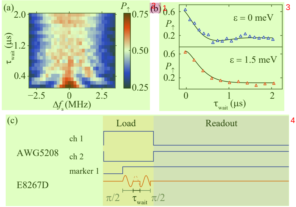
图 5.8 (a) 自旋比特的 Ramsey 实验退相干振荡条纹。对应的双量子点能级失谐 \epsilon = \pm 0.5 meV; (b) 不同双量子点能级失谐处的退相干振荡图: 上图 \epsilon = 0 meV, T_2^* = 0.42 \pm 0.31 \mu\text{s} ; 下图 \epsilon = 1.5 meV, T_2^* = 0.43 \pm 0.02 \mu\text{s} ; (c) Ramsey 实验过程中 AWG5208 的 ch 1 端口输出的方波信号、marker 1 输出的触发信号和 E8267D 输出的微波脉冲。其中微波信号由两段相位连续的 \pi/2 脉冲和中间的等待时间 \tau_{\text{wait}} 组成。
