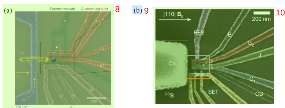
图 1.7 硅量子点中实现自旋单比特门操作的两种实验方案 (a) 硅量子点中带有天线结构样品的扫描电子显微镜（SEM）照片，图中右侧上方红色和绿色电极构成量子点，右侧下方棕色电极构成单电子晶体管，左侧蓝色电极天线；图片摘录自文献 [13] ；(b) 硅量子点中带有微磁体结构样品的扫描电子显微镜（SEM）照片，图中右侧上方的彩色电极构成量子点，右侧下方黄色电极构成单电子晶体管，左侧绿色的为钴制微磁体；图片摘录自文献 [30] 。 11
