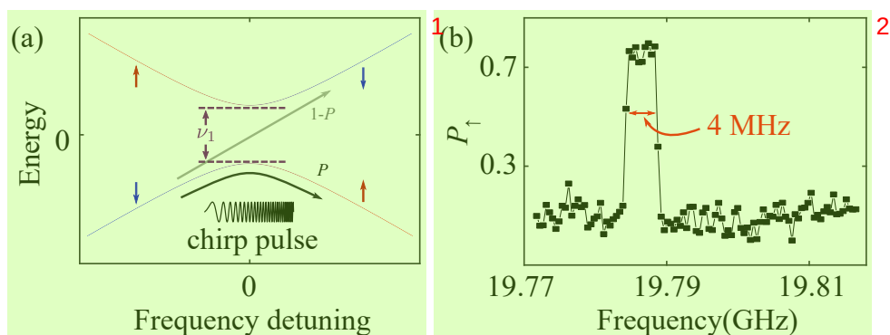
图 4.5 (a) 快速绝热通道翻转自旋比特的原理示意图，随着微波频率的变化，自旋比特从基态翻转到激发态；(b) 使用啁啾脉冲寻找比特频率，脉冲时长为 0.1 ms，带宽为 4 MHz。
