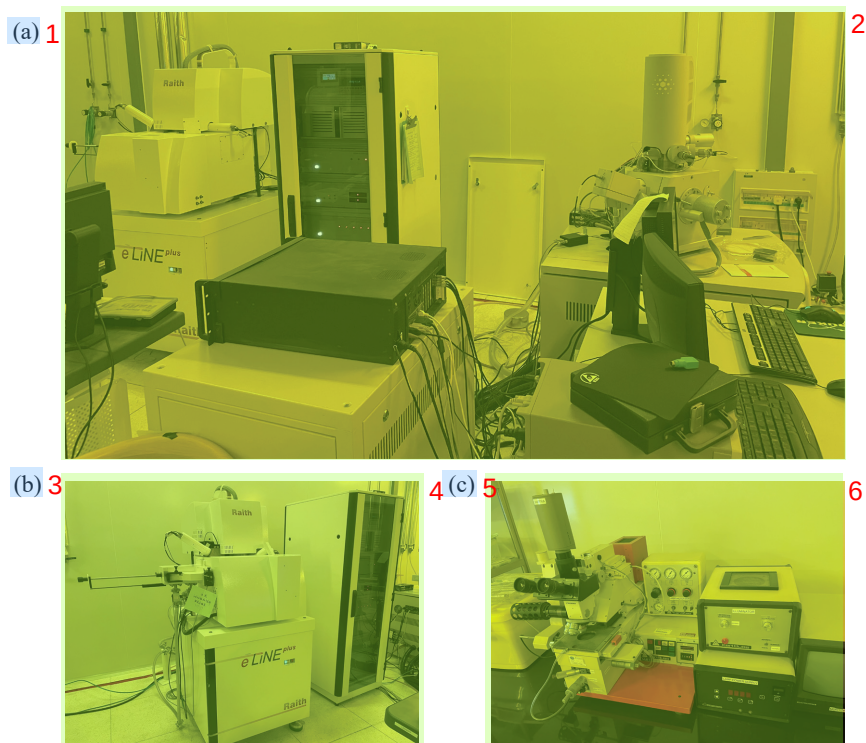
图 2.4 超净室环境展示 (a) 左侧为 eline Plus 和其控制机柜，右侧为 FEI Inspect 50 型号的扫描电镜；(b) eline Plus 特写，左侧上方结构为电子枪，中间为真空腔体，样品和样品台均放置其中，下方为分子泵，右侧为控制机柜；(c) 用于深紫外光刻的 SuSS MJB3 型光刻机。
