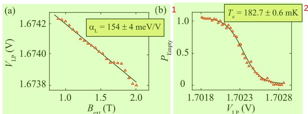
图 5.2 (a) 双量子点中电极 LP 下方量子点中电子填充的能级随磁场的变化，可以提取出臂杆系数 \alpha_{LP} = 154 \pm 4 \text{ meV/V} ；(b) 电极 LP 下方的量子点中电子排空的概率随 V_{LP} 的变化。利用臂杆系数，我们可以从中提取出量子点中的电子温度。图中红线对应拟合得到的电子温度是 182.7 \pm 0.6 \text{ mK} 。
