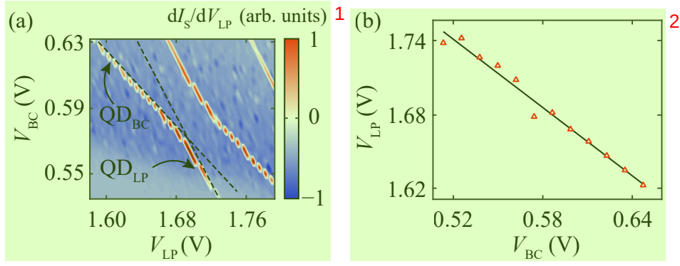
图 5.3 (a) 细扫电极 LP 和电极 BC 得到双量子点的电荷稳定图。在已知电极 LP 对双量子点中第一个量子点的臂杆系数后，我们可以通过第一个量子点输运线线性区间的斜率（图中 QD_{LP} 所指虚线）计算出电极 BC 对第一个量子点的臂杆系数；同理我们可以计算出电极 LP 对第二个量子点的臂杆系数；(b) 测量翻转模式单自旋量子比特过程中，电极 LP 电压随电极 BC 电压的变化情况。可以看到测量过程中为了保持单发读出过程中隧穿速率不变，电极 LP 的电压随着电极 BC 的电压线性变化，同理还有电极 LB 的电压也会随着电极 BC 的电压线性变化。
