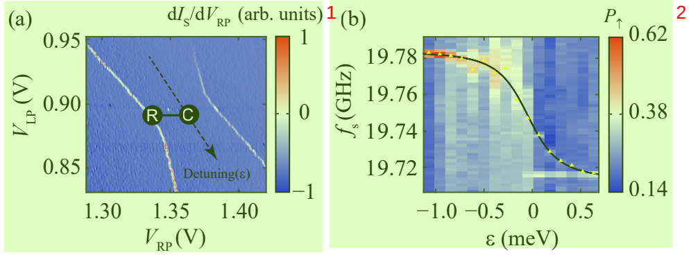
图 5.9 (a) 电极 LP 和 RP 下方双量子点系统的电荷稳定图，图中用箭头标出了能级失谐 detuning 的方向，用 R、C 分别标识出了 AWG5208 输出的方波信号中读取、控制阶段的位置；(b) 通过快速绝热通道方法扫描了不同能级失谐下的比特谐振峰信号。
