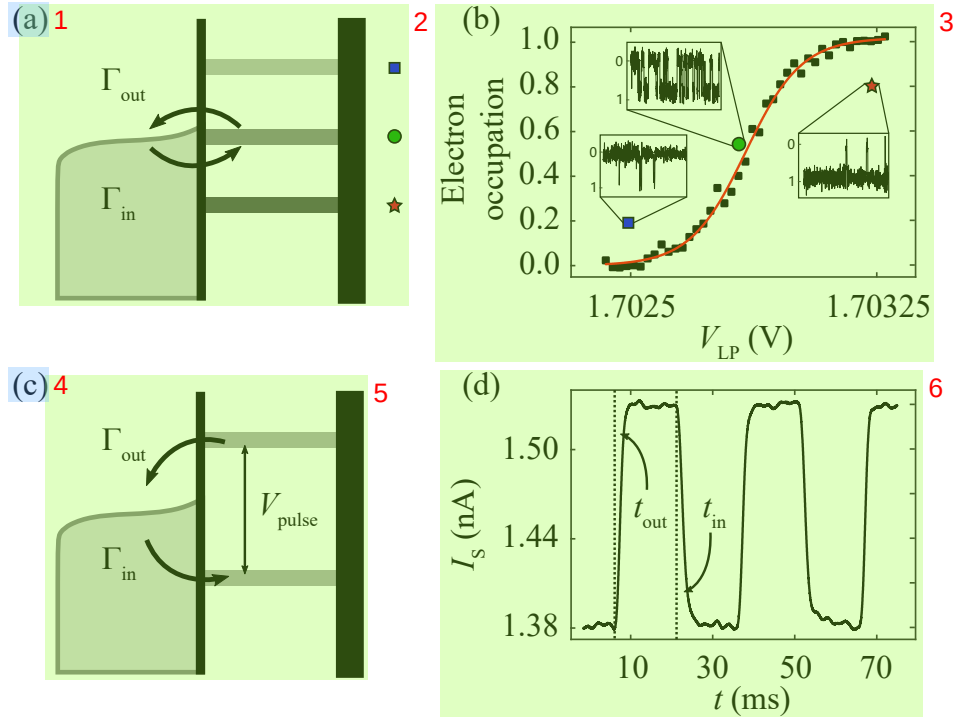
图 4.3 利用随机电报信号测量电子温度和隧穿速率。(a) 硅量子点中在电子隧穿线附近量子点能级和源漏费米面位置的对比示意图；(b) 电极 LP 下方的量子点中电子占据概率随 V_{LP} 的变化。利用臂杆系数，我们可以从中提取出量子点中的电子温度。图中红线对应拟合得到的电子温度是 223.8 \pm 0.8 \text{ mK} 。插图中绿色圆形、蓝色方形和红色星形分别对应 (a) 图中量子点能级对齐、高于和低于源漏费米面的情况；(c) 在电极 LP 上施加周期性的方波，当源漏费米面位于方波高低电平之间时，电子可以在量子点和源漏之间来回隧穿；(d) 施加周期 30 ms 的方波，测量 SET 中响应电流的平均信号，通过拟合波形的上升沿和下降沿，可以得到平均隧穿时间 t_{out} 和 t_{in} ，分别对应隧穿速率 \Gamma_{out} 和 \Gamma_{in} 。
