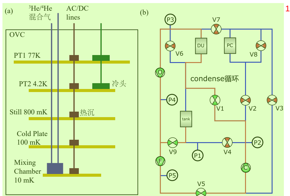
图 2.6 稀释制冷机 (a) 稀释制冷机内部结构示意图，蓝色管路为 ^3\text{He}/^4\text{He} 混合气的循环管路，红色为测量线路，通过热沉与每一层达成热平衡，绿色为脉冲管制冷的管路和冷头；(b) 稀释制冷机控制面板。当系统稳定运行时，外部压缩机帮助 ^3\text{He}/^4\text{He} 混合气完成循环，图中绿色的阀门为开启状态、红色关断，红色管路为气体循环的管路部分，DU 代表 (a) 图中蓝色的 ^3\text{He}/^4\text{He} 混合气的循环管路。
