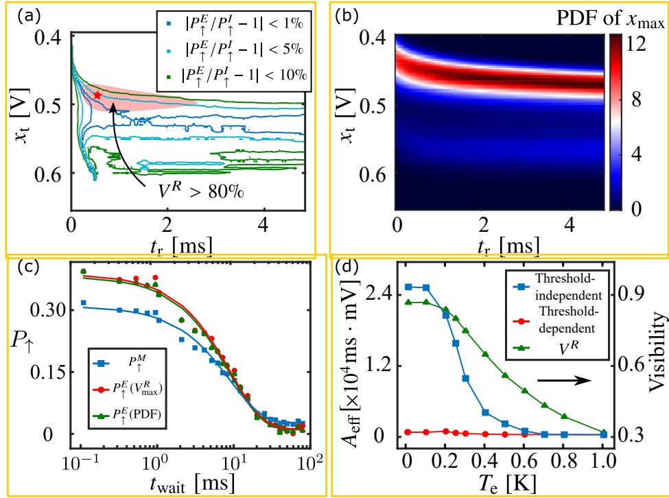
图 3.5 (a) 期望概率 P_{\uparrow}^E 与读取阶段初始概率 P_{\uparrow}^I 的偏差关于时间窗口和电压阈值的轮廓图。图中蓝色、青色和绿色实线分别为 |P_{\uparrow}^E/P_{\uparrow}^I - 1| < 1\% 、5% 和 10% 区域的轮廓线。作为对比，我们用红色星形符号标识出了 V_{\max}^R 的位置，并用粉色阴影区域标识出了 V^R > 80\% 的区域；(b) 不同时间窗口下，读取信号最大值的分布相图。图中可以明显看出信号最大值分布中的双峰位置随着时间窗口增大而向增大的方向平移。图中双峰之间的低谷区域轮廓和 (a) 图中的青色轮廓线相近；(c) 采用阈值无关单发读出方法处理实验数据，我们比较了在 V_{\max}^R 处（红色圆点）和同样时间窗口下读取信号最大值分布的双峰之间最小值位置处（绿色三角形）的 P_{\uparrow}^E ，并用指数衰减函数拟合，发现两者差异较小；与用传统方法处理得到的测量概率 P_{\uparrow}^M （蓝色方形）相比，采用阈值无关单发读出方法处理得到的 P_{\uparrow}^E 更加接近目标值 P_{\uparrow}^I ，且暗记数较小；(d) 蓝色方形和红色圆形分别表示不同电子温度下阈值无关单发读出方法和传统方法的有效参数空间大小 A_{\text{eff}} ，绿色三角形为该温度下的最大读取可见度。
