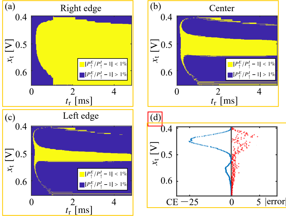
图 3.6 在使用 Monte-Carlo 方法计算 V^R 时，我们需要将电压阈值参数离散化成连续的区域。在计算模拟数据的 P_{\uparrow}^E 时，使用区间中哪一点作为电压阈值会极大影响 P_{\uparrow}^E 的准确性：(a) 使用区间的右边界计算 P_{\uparrow}^E ，则几乎所有参数都可以满足条件 |P_{\uparrow}^E/P_{\uparrow}^I - 1| < 1\% ；(b) 使用区间的中间位置计算 P_{\uparrow}^E ，满足条件 |P_{\uparrow}^E/P_{\uparrow}^I - 1| < 1\% 的参数空间明显减小，虽然计算 P_{\uparrow}^E 时的电压阈值仅变化了 1 mV；(c) 使用区间的左边界计算 P_{\uparrow}^E ，满足条件 |P_{\uparrow}^E/P_{\uparrow}^I - 1| < 1\% 的参数空间继续减小；(d) 拟合参数生成模拟信号的最大值分布于实验数据最大值分布的误差绝对值 ( |error| ，图中红点) 和累积误差 (cumulative error, CE, 图中蓝点)。
