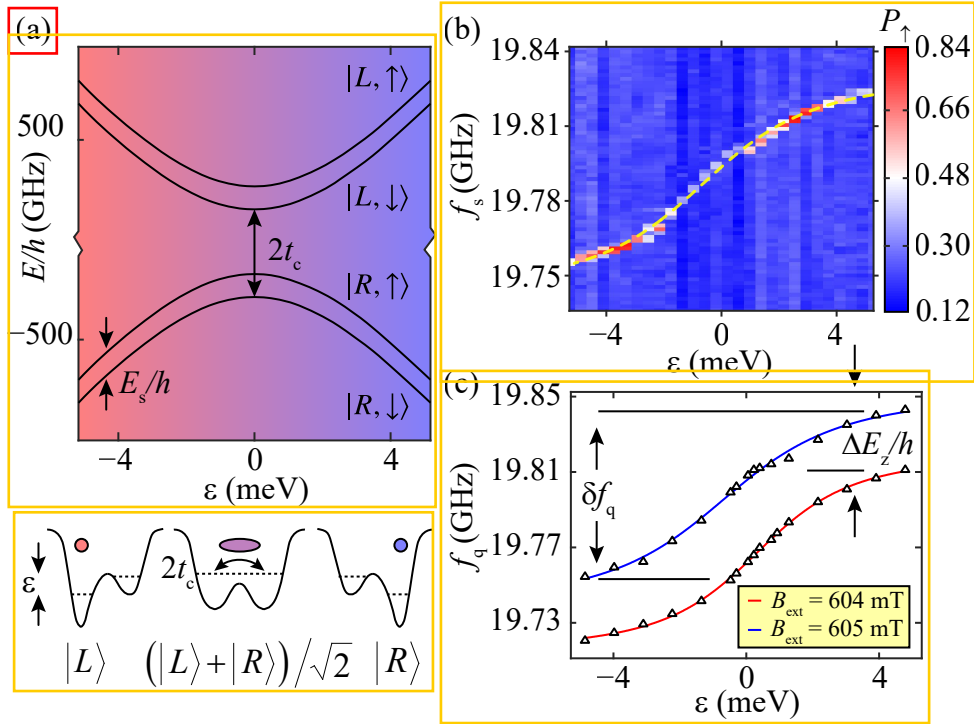
图 5.6 (a) 翻转模式单自旋量子比特中, 电子的本征态和对应的本征能级随双量子点能级失谐的变化, 下方是不同的能级失谐情况下电子在双量子点中的分布情况; (b) 通过快速绝热通道方法, 我们扫描了不同能级失谐下的比特谐振峰信号; (c) 在 (b) 图基础上, 我们通过单频微波测量了单比特谐振频率 f_q 随能级失谐的变化, 此外我们还测量不同外磁场大小下的比特谐振频率曲线, 两条曲线的差值是 \Delta E_z/h 。
