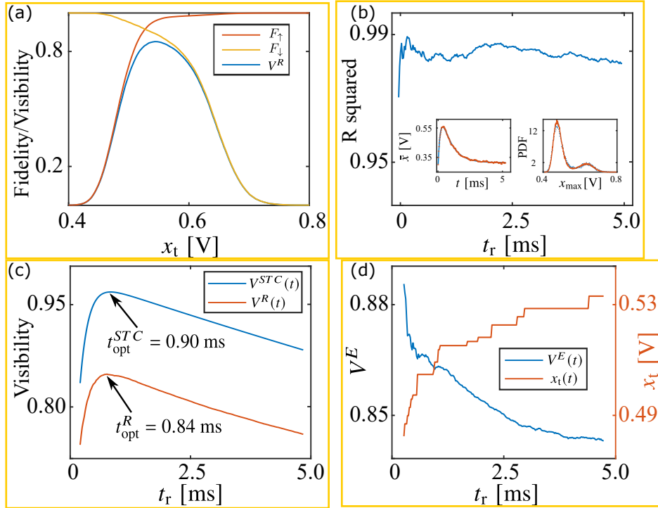
图 3.3 (a) 通过读取保真度 F_{\uparrow} 和 F_{\downarrow} 计算读取可见度 V^R ，最大读取可见度为 85.4%；(b) 用 Monte-Carlo 方法生成模拟数据来拟合实验数据，我们计算了不同时间窗口长度中模拟数据和实验数据最大值分布的残差；对于不同的时间窗口长度，残差值稳定在 0.98 附近；插图分别为多次测量数据的平均值和数据最大值分布的拟合情况；(c) 蓝线为自旋-电荷转换过程中可见度 V^{STC} 随不同时间窗口的变化，红线为读取可见度随不同时间窗口的变化，可以看到两种可见度的最大值位置不同；(d) 蓝线和红线分别为电荷探测可见度 V^E 最大值及其对应的电压阈值随时间窗口的变化，可以看到 V^E 随时间窗口增大而减小，对应的电压阈值则随时间窗口减小而增大。
