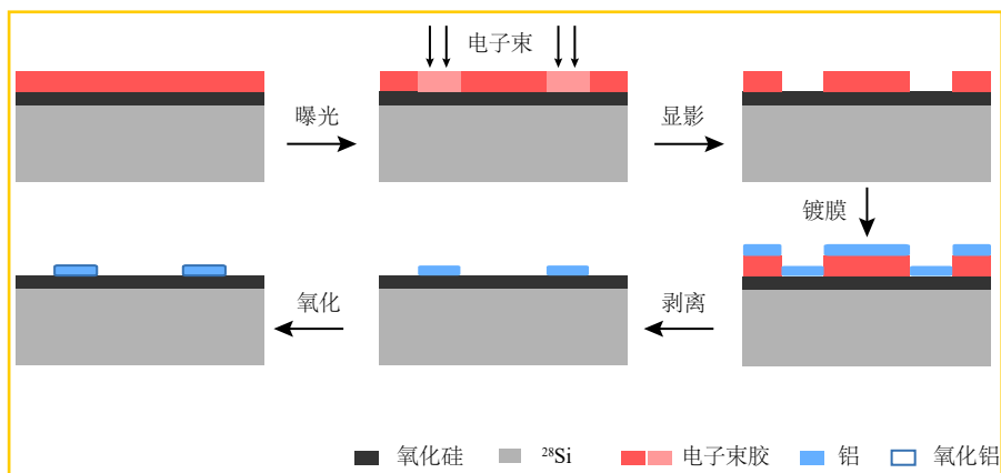
图 2.3 电子束曝光流程图：1. 图中红色区域为电子束胶，型号为 PMMA A4，厚度约 200 nm；2. 粉红色区域为曝光后的电子束胶；3. 显影后，在被曝光的区域形成窗口；4. 使用电子束蒸发镀膜沉积 30-60 nm 厚度的金属铝（蓝色区域）；5. 剥离剩余的电子束胶及附着在胶上的金属，留在硅片表面的金属形成电极结构；6. 对于铝电极，经过原位氧化后，其表面会形成氧化铝绝缘层（深蓝色边缘）。
