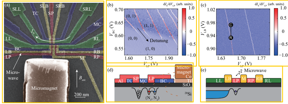
图 5.1 (a) MRL-34-3-1 型号样品的 SEM 照片。与第四章中不同，电极 LP 和 BC 下方各形成了一个量子点，构成了另一组双量子点结构。 I_S 表示流经 SET 的电流，箭头标识了电流的方向。 B_{ext} 标识了外磁场的大小和方向；(b) 电极 LP 和 BC 下方双量子点系统的电荷稳定图。图中不同颜色表示通过单电子晶体管的电流微分信号，括号内的数字表示电极 LP 和 BC 下方量子点中的电子数目；(c) 扫描电极 LP 和 LB 和得到的电荷稳定图，由于测量线路中 bias-tee 出现了故障，我们将任意波形发生器输出的方波加从电极 LP 转移到电极 LB 上，测量方波中对应的电压位置用图中 R、C 大致标识出来；此外我们还通过电极 LB 调节样品中电子的隧穿速率；(d) 电极 LP 和 BC 下方双量子点系统的纵向剖面示意图，图中展示了不同电极之间的位置关系和量子点形成的位置，并标识了衬底与电极的材料。棕色虚线粗略标识出微磁体结构在样品中产生的感应磁场的磁感应线；(e) 电极 LP 和 BC 下方双量子点系统的横向剖面示意图。图中标识了量子点区域不同电极之间的大致位置关系和双量子的形成位置，微波驱动通过 bias-tee 加在电极 LP 上。
