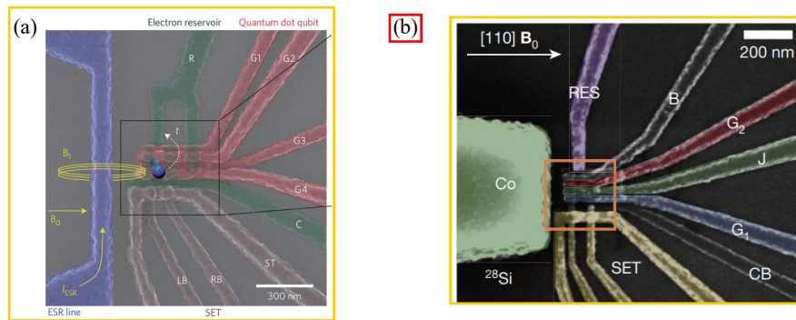
图 1.7 硅量子点中实现自旋单比特门操作的两种实验方案 (a) 硅量子点中带有天线结构样品的扫描电子显微镜（SEM）照片，图中右侧上方红色和绿色电极构成量子点，右侧下方棕色电极构成单电子晶体管，左侧蓝色电极为天线；图片摘录自文献 [13] ；(b) 硅量子点中带有微磁体结构样品的扫描电子显微镜（SEM）照片，图中右侧上方的彩色电极构成量子点，右侧下方黄色电极构成单电子晶体管，左侧绿色的为钴制微磁体；图片摘录自文献 [30] 。
