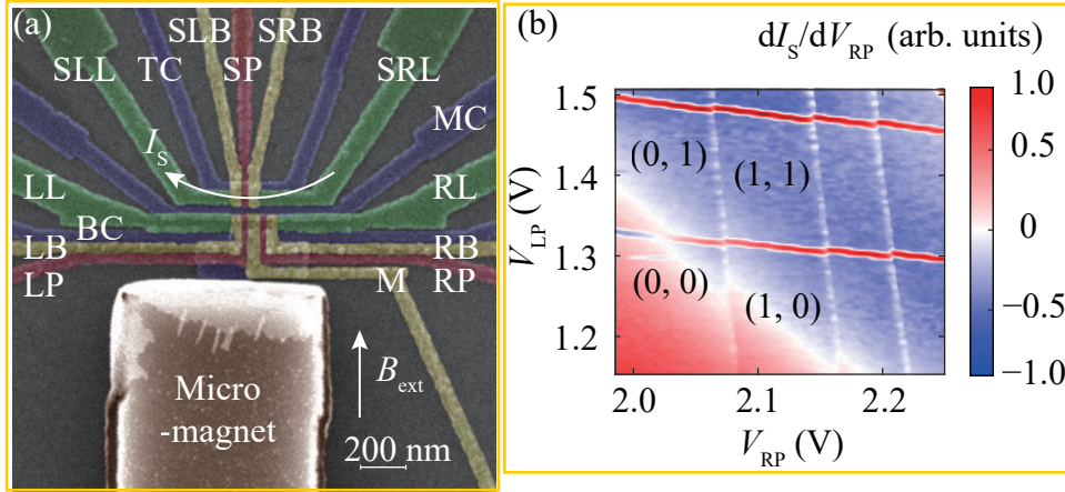
图4.1 (a) MRL-34-3-1 型号样品的 SEM 照片。在电极 LP 和 RP 下方各形成了一个量子点，构成了双量子点结构。 I_s 表示流经 SET 的电流，箭头标识了电流的方向。 B_{ext} 标识了外磁场的大小和方向；(b) 双量子点系统的电荷稳定图。图中不同颜色表示通过单电子晶体管的电流微分信号，括号内的数字表示电极 LP 和 RP 下方量子点中的电子数目。
