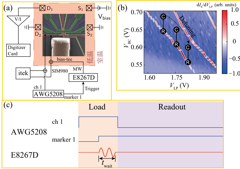
图 5.4 实验中使用的测量翻转模式单自旋量子比特的方式：(a) 测量电路图。我们使用 AWG5208 型号任意波形发生器生成方波脉冲信号，通过对应的 marker 输出端口触发矢量信号发生器 E8267D 生成微波脉冲。其中方波信号与直流电压源 itek 的输出端口在室温下通过叠加器 SIM980 叠加后，施加到电极 LB 上。微波脉冲则在稀释制冷机的 4 K 盘通过 bias-tee 与 itek 的输出的直流电压叠加，最后施加到电极 LP 上；(b) 通过调整读取位置，我们分别对不同能级失谐处的比特进行测量。实际测量过程中，还需要调节电极 LB 的电压以保证隧穿速率稳定，因此图中的读取位置仅为示意图；(c) AWG5208 的 ch 1 端口输出的方波信号、marker 1 输出的触发信号和 E8267D 输出的微波脉冲。
