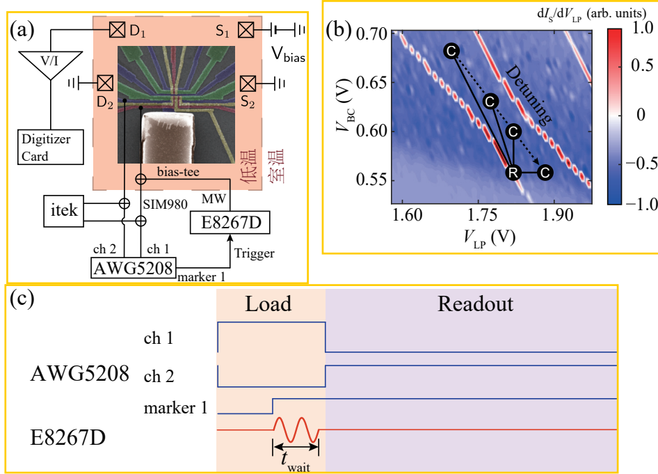
图 5.5 另一种常用的测量翻转模式单自旋量子比特的方式：(a) 测量电路图。我们使用 AWG5208 型号任意波形发生器生成两路方波脉冲信号，并利用 ch 1 的 marker 输出端口触发矢量信号发生器 E8267D 生成微波脉冲。其中 ch 1 的方波信号与直流电压源 itek 的输出端口在室温下通过叠加器 SIM980 叠加后，再在稀释制冷机的 4 K 盘通过 bias-tee 与微波脉冲叠加施加到电极 LP 上。ch 2 的方波信号与直流电压源 itek 的输出端口在室温下通过叠加器 SIM980 叠加后，施加到电极 BC 上；(b) 通过改变两路方波脉冲加载阶段的电压，我们可以分别对不同能级失谐处的比特进行测量；(c) AWG5208 的 ch 1、ch 2 端口输出的方波信号、marker 1 输出的触发信号和 E8267D 输出的微波脉冲。
