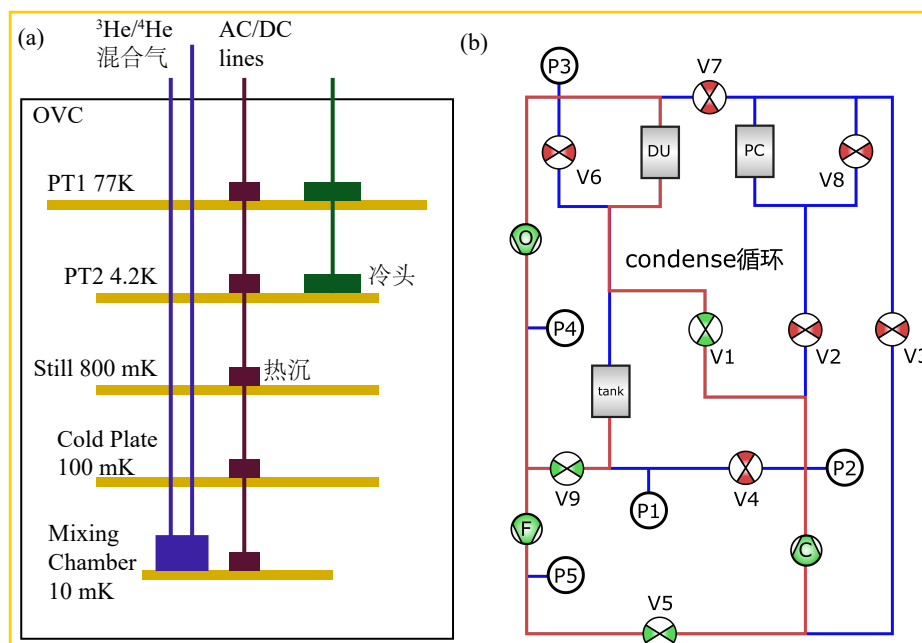
图 2.6 稀释制冷机 (a) 稀释制冷机内部结构示意图，蓝色管路为 ^3\text{He}/^4\text{He} 混合气的循环管路，红色为测量线路，通过热沉与每一层达成热平衡，绿色为脉冲管制冷的管路和冷头；(b) 稀释制冷机控制面板。当系统稳定运行时，外部压缩机帮助 ^3\text{He}/^4\text{He} 混合气完成循环，图中绿色的阀门为开启状态、红色关闭，红色管路为气体循环的管路部分，DU 代表 (a) 图中蓝色的 ^3\text{He}/^4\text{He} 混合气的循环管路。
