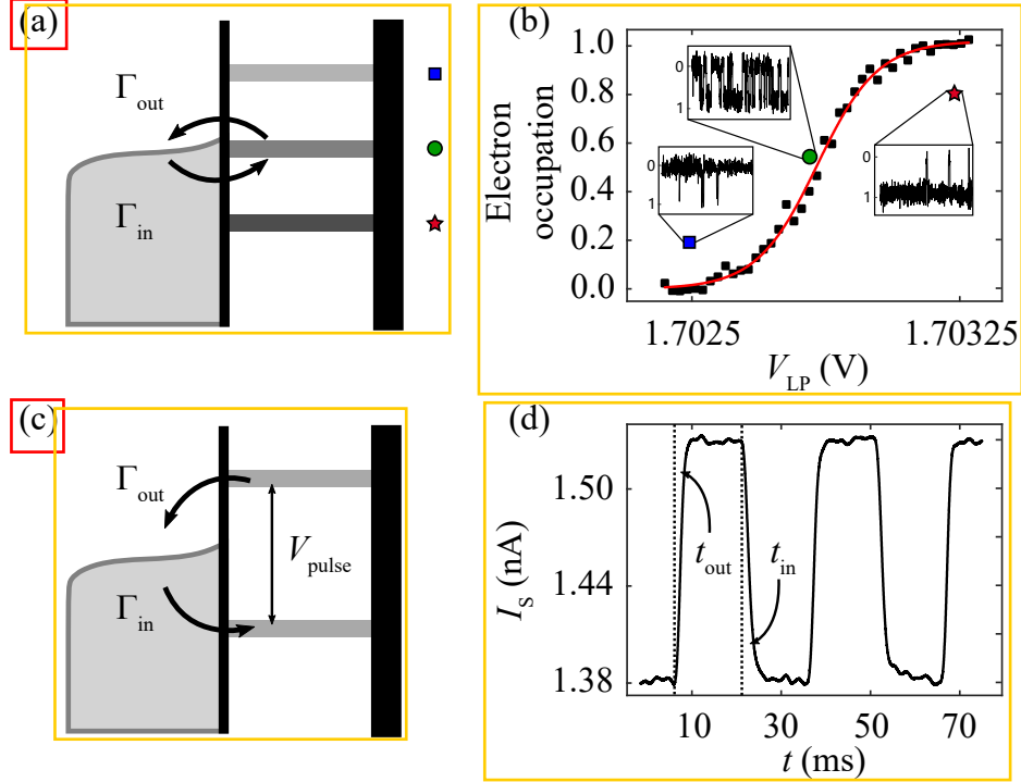
图 4.3 利用随机电报信号测量电子温度和隧穿速率。(a) 硅量子点中在电子隧穿线附近量子点能级和源漏费米面位置的对比示意图；(b) 电极 LP 下方的量子点中电子占据概率随 V_{LP} 的变化。利用臂杆系数，我们可以从中提取出量子点中的电子温度。图中红线对应拟合得到的电子温度是 223.8 \pm 0.8 \text{ mK} 。插图中绿色圆形、蓝色方形和红色星形分别对应 (a) 图中量子点能级对齐、高于和低于源漏费米面的情况；(c) 在电极 LP 上施加周期性的方波，当源漏费米面位于方波高低电平之间时，电子可以在量子点和源漏之间来回隧穿；(d) 施加周期 30 ms 的方波，测量 SET 中响应电流的平均信号，通过拟合波形的上升沿和下降沿，可以得到平均隧穿时间 t_{out} 和 t_{in} ，分别对应隧穿速率 \Gamma_{out} 和 \Gamma_{in} 。
