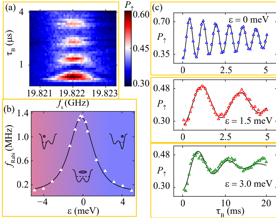
图 5.7 (a) 在双量子点失谐约 0.5 meV 处的自旋比特 Rabi 振荡的 V 形条纹，图中每个点的自旋态概率都是 300 次单发读出结果的平均值，扫描时先固定微波脉冲时间 \tau_B ，扫描微波频率 f_s 。从图中可以得到自旋比特谐振频率约 19.8221 GHz；(b) 自旋比特 Rabi 频率随双量子点能级失谐的变化图。Rabi 振荡在零失谐位置相比 \epsilon = \pm 4.5 meV 处提升了约一个数量级；(c) 不同双量子点能级失谐处的 Rabi 振荡图：上图 \epsilon = 0 meV， f_{\text{Rabi}} = 1.2620 \pm 0.002 MHz， T_2^{\text{Rabi}} = 6.46 \pm 0.39 \mu s；中图 \epsilon = 1.5 meV， f_{\text{Rabi}} = 0.429 \pm 0.003 MHz， T_2^{\text{Rabi}} = 5.53 \pm 0.57 \mu s；下图 \epsilon = 3 meV， f_{\text{Rabi}} = 0.135 \pm 0.003 MHz， T_2^{\text{Rabi}} = 7.01 \pm 0.82 \mu s。
