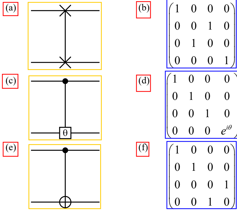
图 1.3 三种常见的两比特门的符号和对应的变换矩阵：(a)(b) SWAP 门符号和对应的变换矩阵；(c)(d) C-Phase 门符号和对应的变换矩阵，当 \theta 取 \pi 、 \pi/2 和 \pi/4 ，分别可以实现 C-Z、C-S 和 C-T 门；(e)(f) C-NOT 门符号和对应的变换矩阵。
