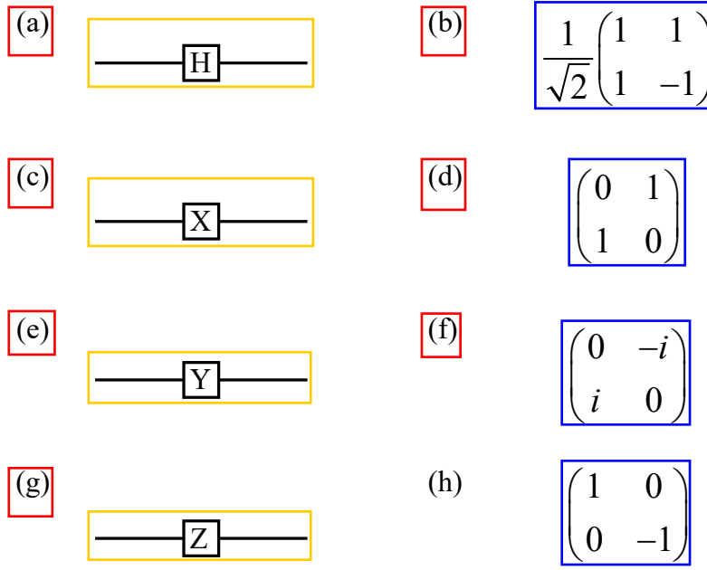
图 1.2 四种常见的单比特门的符号和对应的变换矩阵：(a)(b) Hadamard 门符号和对应的变换矩阵，(a) 图左侧为比特输入，右侧为比特输出，比特经过中间 H 符号表示的 Hadamard 门后，可以将单比特从纯态变换为最大纠缠态，(b) 图为相应的变换矩阵；(c)(d) X 门符号和对应的变换矩阵，绕 X 轴旋转 \pi ；(e)(f) Y 门符号和对应的变换矩阵，绕 Y 轴旋转 \pi ；(g)(h) Z 门符号和对应的变换矩阵，绕 Z 轴旋转 \pi 。
