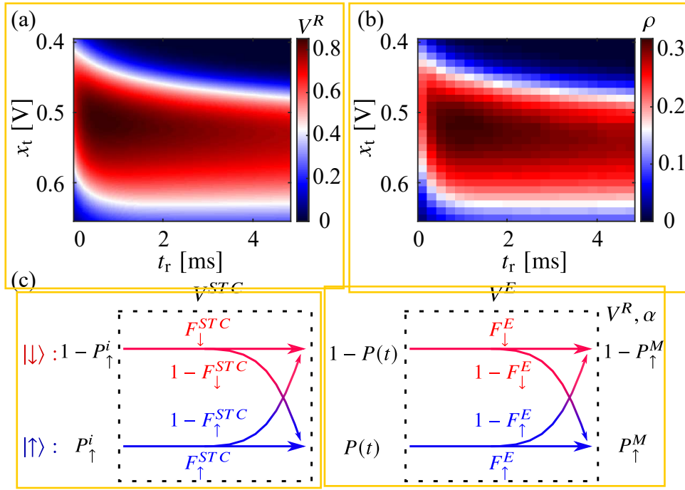
图 3.4 (a) 读取可见度随电压阈值和时间窗口变化的相图，图中读取可见度沿纵轴方向的变化如图 3.3a 中蓝线所示，横轴方向的变化如图 3.3c 中红线所示；(b) 用不同的时间窗口和电压阈值处理读取数据，然后计算自旋弛豫曲线并拟合得到相应的弛豫过程幅值 \rho ；(c) 读取阶段开始时，量子点中电子处于基态的概率为 P^i_{\uparrow} ，经过自旋-电荷转换过程，在时间窗口内，有 P(t) 概率隧穿出量子点；最终经过电荷探测过程，被测量到的激发态概率是 P^M_{\uparrow} 。
