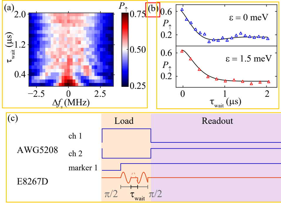
图 5.8 (a) 自旋比特的 Ramsey 实验退相干振荡条纹。对应的双量子点能级失谐 \varepsilon = \pm 0.5 meV; (b) 不同双量子点能级失谐处的退相干振荡图: 上图 \varepsilon = 0 meV, T_2^* = 0.42 \pm 0.31 \mu s; 下图 \varepsilon = 1.5 meV, T_2^* = 0.43 \pm 0.02 \mu s; (c) Ramsey 实验过程中 AWG5208 的 ch 1 端口输出的方波信号、marker 1 输出的触发信号和 E8267D 输出的微波脉冲。其中微波信号由两段相位连续的 \pi/2 脉冲和中间的等待时间 \tau_{\text{wait}} 组成。
