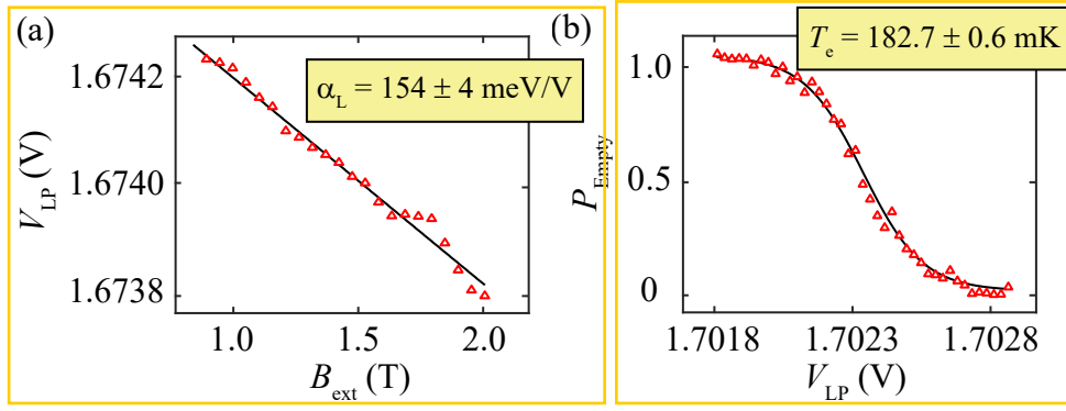
图 5.2 (a) 双量子点中电极 LP 下方量子点中电子填充的能级随磁场的变化，可以提取出臂杆系数 \alpha_{LP} = 154 \pm 4 meV/V；(b) 电极 LP 下方的量子点中电子排空的概率随 V_{LP} 的变化。利用臂杆系数，我们可以从中提取出量子点中的电子温度。图中红线对应拟合得到的电子温度是 182.7 \pm 0.6 mK。
