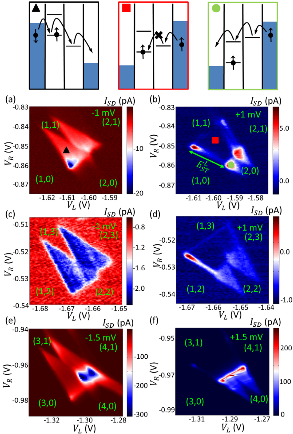
图 5.2 (a)-(b) (1,1)-(2,0) 区域 I_{SD} 在偏压 V_{SD} = -1 mV 和 V_{SD} = +1 mV 时随 V_L 和 V_R 的变化。不同颜色标记的位置处电子隧穿过程由相应颜色的框图示意。(c)-(d) (1,3)-(2,2) 区域 I_{SD} 在偏压 V_{SD} = -1 mV 和 V_{SD} = +1 mV 时随 V_L 和 V_R 的变化。(e)-(f) (3,1)-(4,0) 区域 I_{SD} 在偏压 V_{SD} = -1.5 mV 和 V_{SD} = +1.5 mV 时随 V_L 和 V_R 的变化。
