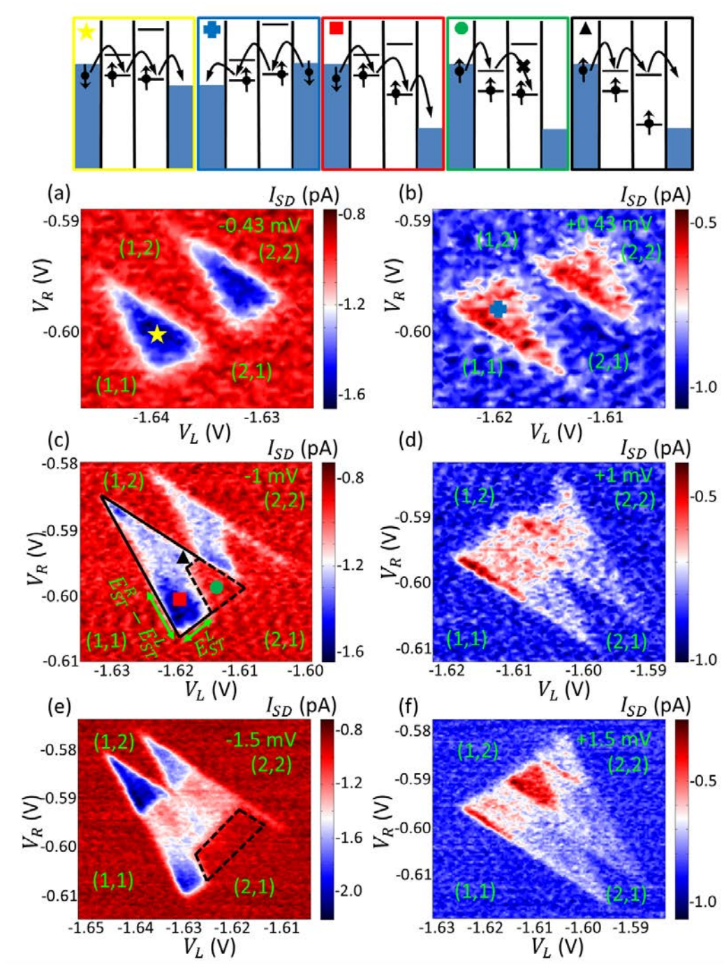
图 5.3 (a)-(f) (1,2)-(2,1) 区域 I_{SD} 在偏压 V_{SD} = -0.43 mV, V_{SD} = +0.43 mV, V_{SD} = -1 mV, V_{SD} = +1 mV, V_{SD} = -1.5 mV 和 V_{SD} = +1.5 mV 时随 V_L 和 V_R 的变化。不同颜色标记的位置处电子隧穿过程由相应颜色的框图示意。
