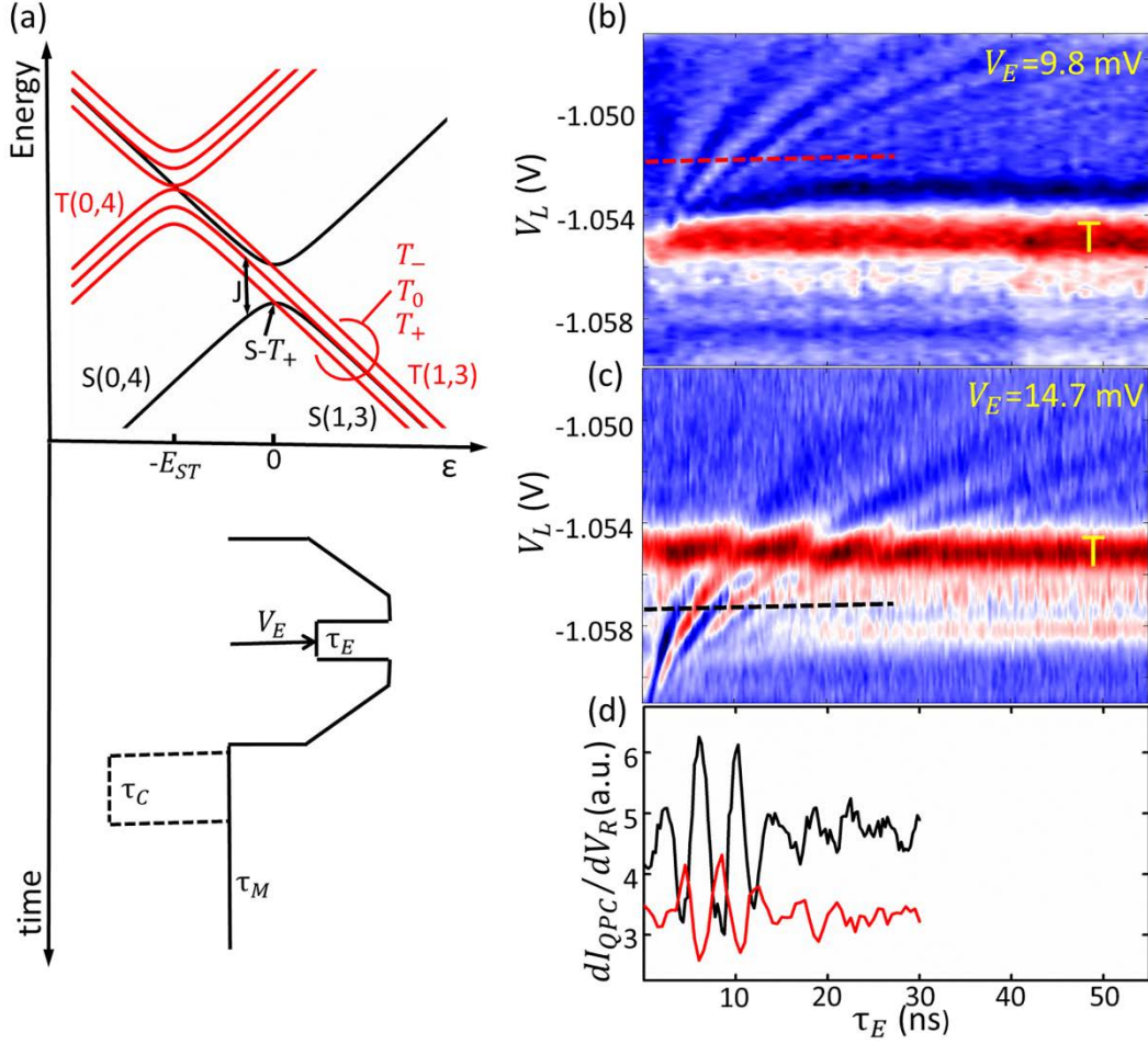
图 4.2 (a) 上部分是能级图, 下部分是用于产生交换振荡的脉冲序列。在采集图 4.4 中数据时, 在操作序列之后添加了一个开关脉冲, 如图中虚线所示。(b) 交换振荡随着交换持续时间 \tau_E 和基准失谐在 V_L 上分量的变化。 V_E = 9.8 mV。(c) 和 (b) 一样, 但是 V_E = 14.7 mV。(d) 中的曲线是 (b) 和 (c) 在相同颜色虚线指示位置处的线切。
