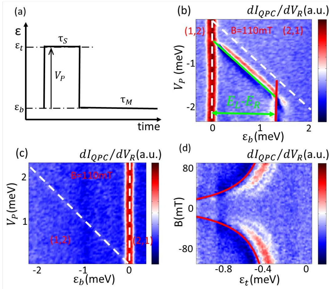
图 3.3 (a)用来观察自旋阻塞和自旋漏斗的失谐脉冲。脉冲宽度 \tau_s = 200 \text{ ns} ，测量时间 \tau_M = 5 \mu\text{s} 。(b) 在沿负失谐轴施加脉冲的情况下，所测得的 QPC 互导 dI_{QPC}/dV_R 随着基准失谐 \varepsilon_b 和脉冲幅度 V_p 的变化。磁场 B = 110 \text{ mT} 。(c)和(b)一样，只不过脉冲是沿着正失谐轴
