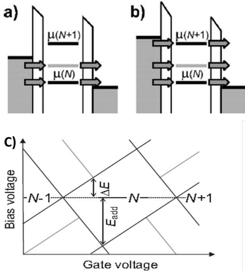
图 1.8 (a) N 个电子的基态和激发态同时处于偏压窗口中，电子可以从任一个态通过量子点。(b) 偏压大于增加能时，允许两个电子同时通过量子点。(c) 量子点的微分电导随着源漏偏压和栅极电压的变化。图中黑线表示电流开始出现。灰色的线表示通过激发态的输运开始出现。(a)(b)引自[37]，(c)引自[5]。
