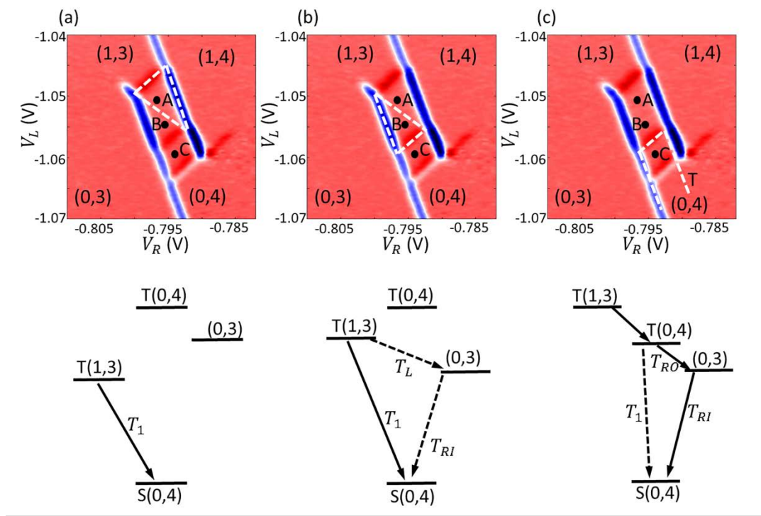
图 4.3 (a)–(c) 中分别用白色虚线标记了不同的测量区域 A, B 和 C。它们对应的能级图画在下边。在能级图中不同跃迁的特征时间被标记了出来。占支配地位的弛豫路径被画为实箭头，其他路径被画为虚箭头。
