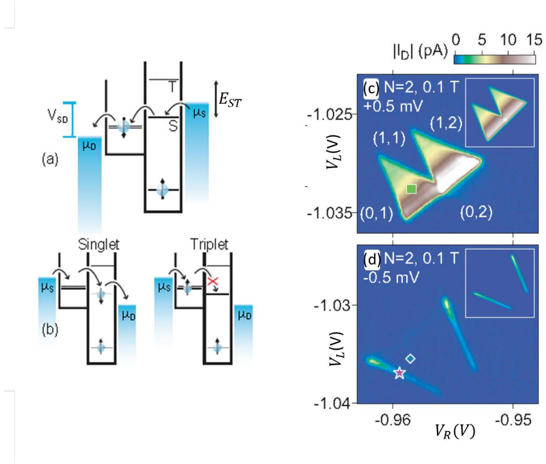
图 2.5 (a) (b) 分别展示了正反偏压下电子隧穿过程。引自[28]。(c) (d) 分别展示了正反偏压下流过量子点的电流。引自[26]。
