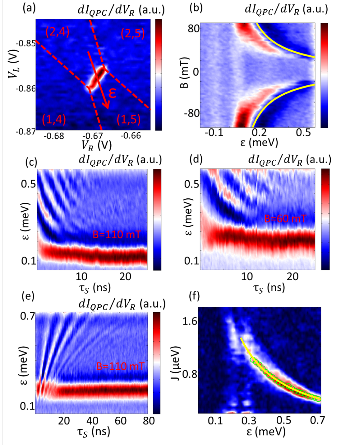
图 4.6 (1, 5)–(2, 4) 区域的测量结果。(a) 相图。(b) 自旋漏斗。实验所用的方脉冲的持续时间为 200 ns, 周期为 10 \mu s。(c) 磁场 B=110 mT 时的 LZS 振荡。(d) 磁场 B=60 mT 时的 LZS 振荡。LZS 振荡实验采用的是梯形波, 上升沿为 5.5 ns, 测量时间为 5 \mu s。(e) 交换振荡。(f) (e) 中数据沿 \tau_S 轴的快速傅里叶变换。黄色的曲线是用两电子 J(\epsilon) 模型所做的拟合, 其
