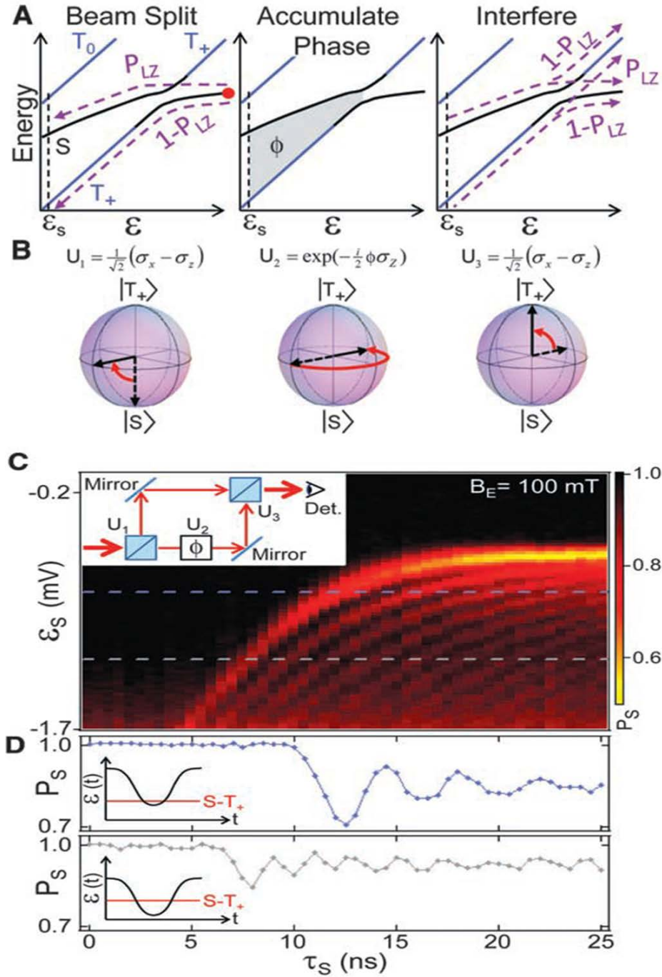
图 2.10 (a) 脉冲过程示意图。(b) 扫描条件满足 P_{LZ} = 1/2 和 \phi = \pi 时的么正变换的布洛赫球表示。(c) 单态概率随着脉冲尖端失谐和脉冲宽度的变化。(d) (c) 中虚线位置处的线切。图片引自[37]
