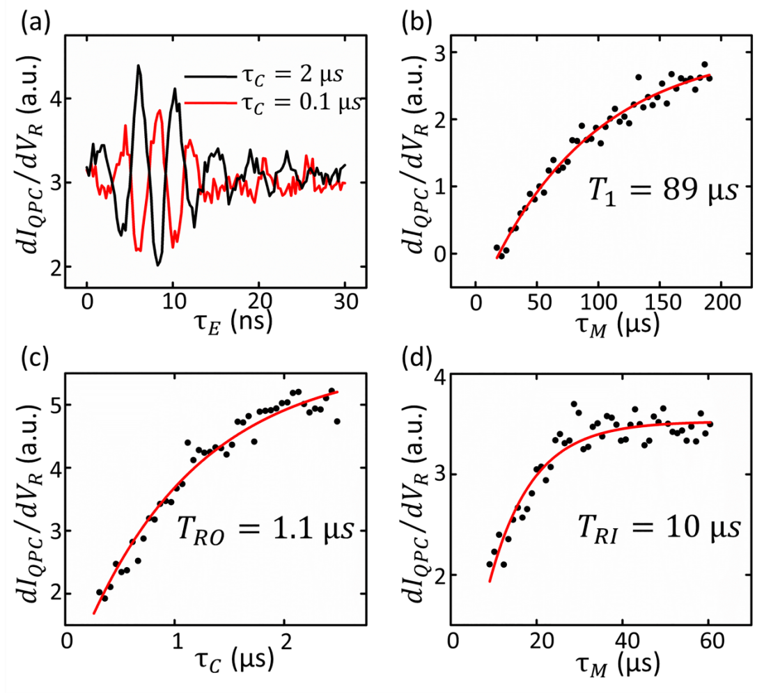
图 4.4 (a) 当 \tau_C = 2 \mu s 和 \tau_C = 0.1 \mu s 时所测得的交换振荡。(b) QPC 互导 dI_{QPC}/dV_R 随 \tau_M 的变化。 \tau_C = 0 。(c) QPC 互导 dI_{QPC}/dV_R 随 \tau_C 的变化。 \tau_M = 10 \mu s 。(b) QPC 互导 dI_{QPC}/dV_R 随 \tau_M 的变化。 \tau_C = 2 \mu s 。(b)-(d) 中的红色曲线是用指数衰减函数 A + B \exp(-\tau/T) 拟合得到的。
