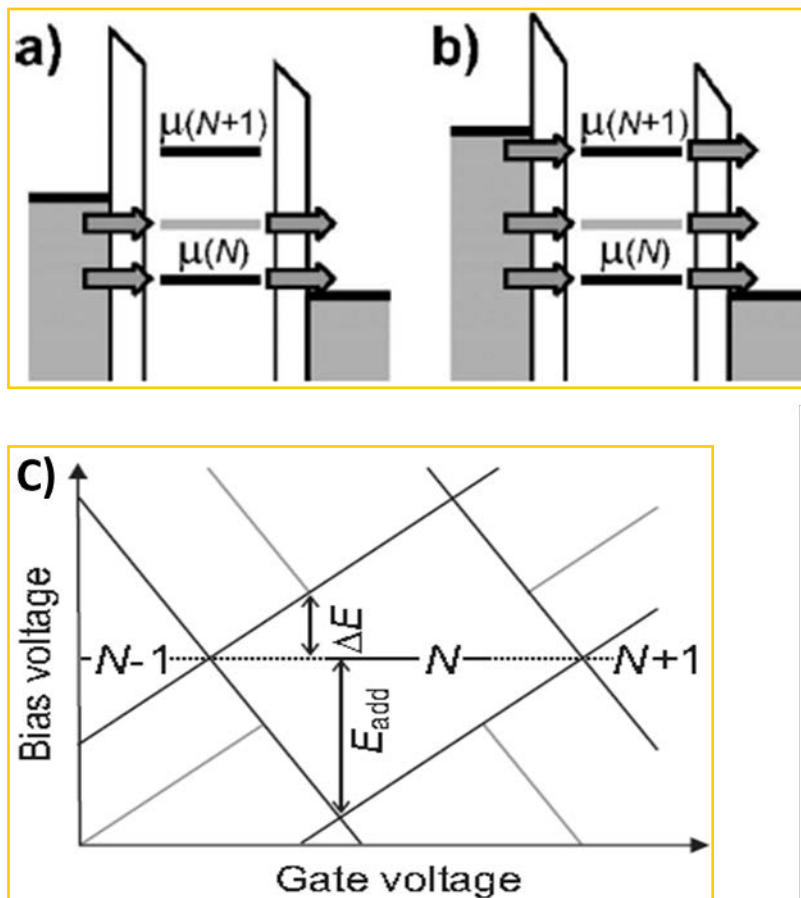
图 1.8 (a) N 个电子的基态和激发态同时处于偏压窗口中，电子可以从任一态通过量子点。(b) 偏压大于增加能时，允许两个电子同时通过量子点。(c) 量子点的微分电导随着源漏偏压和栅极电压的变化。图中黑线表示电流开始出现。灰色的线表示通过激发态的输运开始出现。(a)(b)引自[37]，(c)引自[5]。
