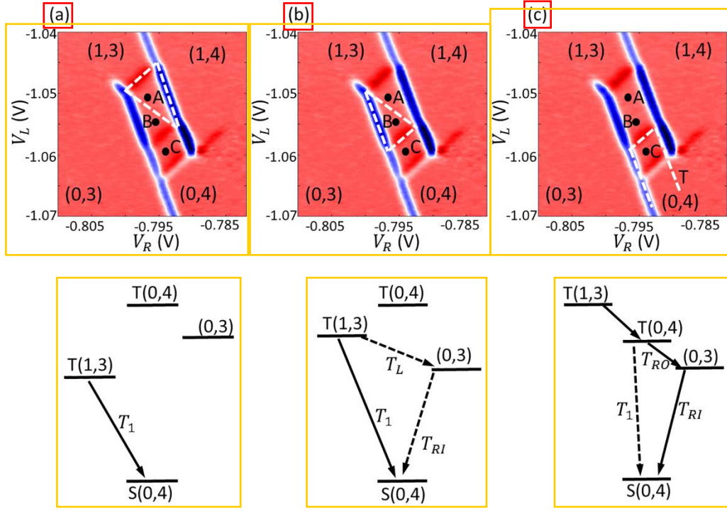
图 4.3 (a)-(c)中分别用白色虚线标记了不同的测量区域 A, B 和 C。它们对应的能级图画在下边。在能级图中不同跃迁的特征时间被标记了出来。占支配地位的弛豫路径被画为实箭头。其他路径被画为虚箭头。
