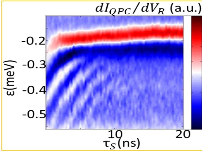
图 2.11 我们组在 (1, 1) - (2, 0) 区域附近测到的 LZS 振荡。
