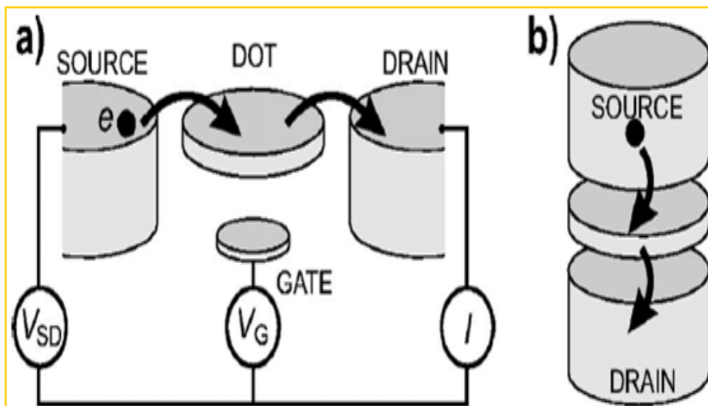
图 1.2 量子点示意图。量子点用圆盘表示，它和源漏通过隧穿势垒耦合，和栅极通过电容耦合。(a)横向量子点结构示意图。(b)纵向量子点结构示意图。图片引自[37]。
