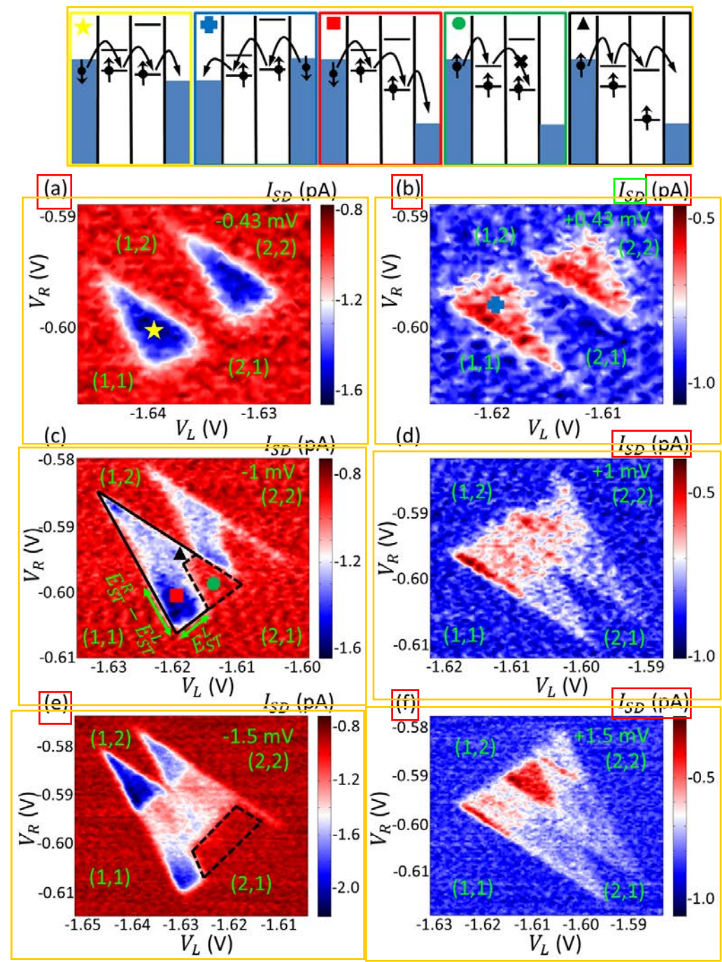
图 5.3 (a)-(f) (1,2)-(2,1) 区域 I_{SD} 在偏压 V_{SD} = -0.43 \text{ mV} , V_{SD} = +0.43 \text{ mV} , V_{SD} = -1 \text{ mV} , V_{SD} = +1 \text{ mV} , V_{SD} = -1.5 \text{ mV} 和 V_{SD} = +1.5 \text{ mV} 时随 V_L 和 V_R 的变化。不同颜色标记的位置处电子隧穿过程由相应颜色的框图示意。
