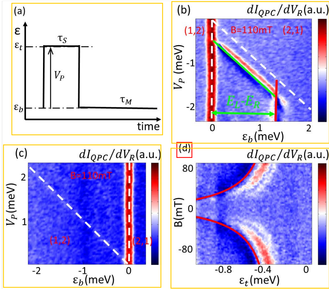
图 3.3 (a) 用来观察自旋阻塞和自旋漏斗的失谐脉冲。脉冲宽度 \tau_S = 200 \text{ ns} , 测量时间 \tau_M = 5 \mu\text{s} 。(b) 在沿负失谐轴施加脉冲的情况下, 所测得的 QPC 互导 dI_{QPC}/dV_R 随着基准失谐 \varepsilon_b 和脉冲幅度 V_P 的变化。磁场 B = 110 \text{ mT} 。(c) 和 (b) 一样, 只不过脉冲是沿着正失谐轴
