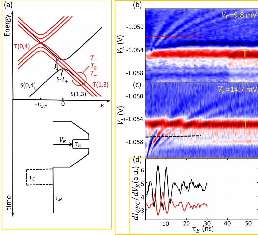
图 4.2 (a) 上部分是能级图，下部分是用于产生交换振荡的脉冲序列。在采集图 4.4 中数据时，在操作序列之后添加了一个开关脉冲，如图中虚线所示。(b) 交换振荡随着交换持续时间 \tau_E 和基准失谐在 V_L 上分量的变化。 V_E = 9.8 \text{ mV} 。(c) 和 (b) 一样，但是 V_E = 14.7 \text{ mV} 。(d) 中的曲线是 (b) 和 (c) 在相同颜色虚线指示位置处的线切。
