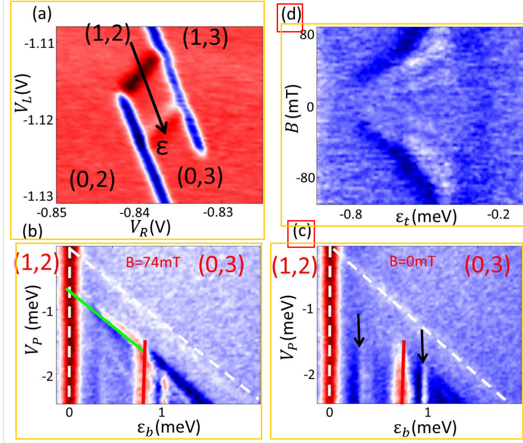
图 3.7 (a) (1,2)-(0,3)电荷跃迁区域附近的相图。不同区域的电子数目也已在图中标出。黑色箭头定义了失谐轴。施加在电极 L 和 R 上的两个同步脉冲经过校准后沿着此轴改变失谐量。 (b) 在沿负失谐轴施加脉冲的情况下，所测得的 QPC 互导 dI_{QPC}/dV_R 随着基准失谐 \varepsilon_b 和脉冲幅度 V_P 的变化。磁场 B = 74 \text{ mT} 。(c)和(b)一样，只不过磁场 B = 0 \text{ mT} 。(d) 在沿负失谐轴施加脉冲的情况下，所测得的 QPC 互导 dI_{QPC}/dV_R 随着脉冲尖端的失谐 \varepsilon_t 和磁场 B 的变化。图像呈现出一个漏斗形状的特征。在测量的过程中，基准失谐 \varepsilon_b 设置在阻塞窗口内。 在(a)-(d)中脉冲宽度 \tau_s = 200 \text{ ns} ，测量时间 \tau_M = 5 \mu\text{s} 。
