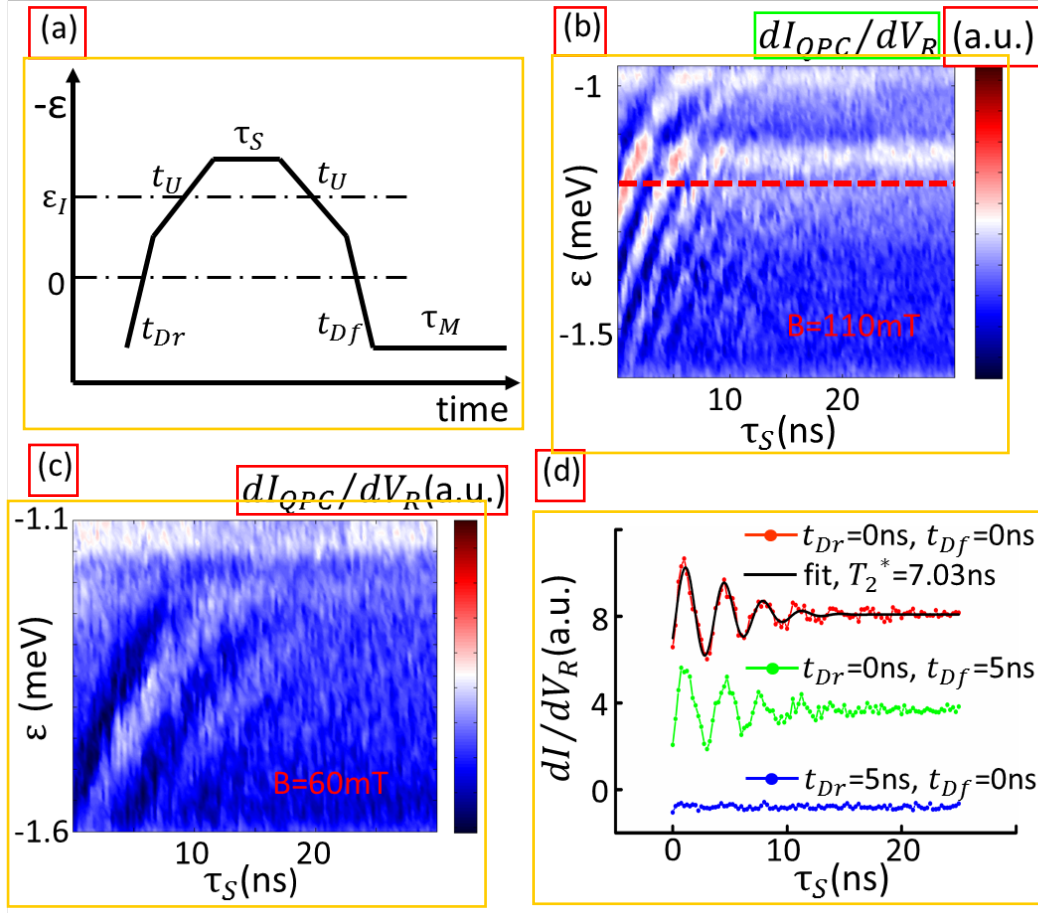
图 3.4 (a)用于测量 LZO 振荡的失谐脉冲。(b)LZO 振荡随着 \varepsilon 和 \tau_s 的变化。磁场 B = 110 \text{ mT} 。(c)和(b)一样，但是磁场 B = 60 \text{ mT} 。(d)在与 D_s - D_s 反交叉相关脉冲参数设为不同值时所测得的 LZO 振荡随 \tau_s 的变化。脉冲尖端失谐 \varepsilon 设在(b)中红色虚线所指示的位置上。对所有情况 t_U 都设为 5 \text{ ns} 。用高斯衰减余弦函数拟合最上边的红色曲线给出 T_2^* = 7 \text{ ns} 。
