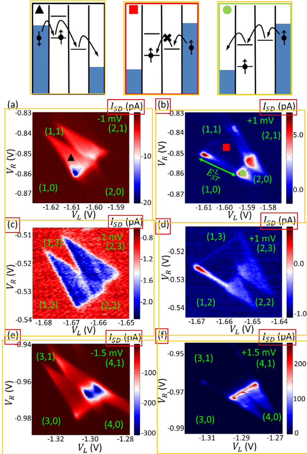
图 5.2 (a)-(b) (1,1)-(2,0) 区域 I_{SD} 在偏压 V_{SD} = -1\text{ mV} 和 V_{SD} = +1\text{ mV} 时随 V_L 和 V_R 的变化。不同颜色标记的位置处电子隧穿过程由相应颜色的框图示意。(c)-(d) (1,3)-(2,2) 区域 I_{SD} 在偏压 V_{SD} = -1\text{ mV} 和 V_{SD} = +1\text{ mV} 时随 V_L 和 V_R 的变化。(e)-(f) (3,1)-(4,0) 区域 I_{SD} 在偏压 V_{SD} = -1.5\text{ mV} 和 V_{SD} = +1.5\text{ mV} 时随 V_L 和 V_R 的变化。
