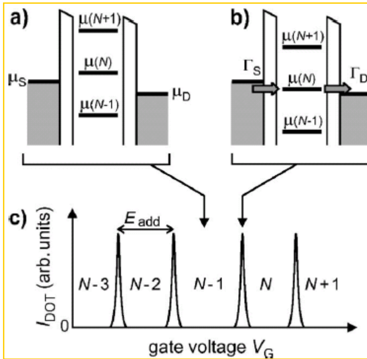
图 1.7 小偏压下的量子点。(a)没有化学势处在由源漏化学势设置的窗口内。量子点的电子数目固定为 N-1 ，库伦阻塞发生。(b) \mu(N) 处在偏压窗口内，量子点的电子数在 N 和 N-1 之间振荡，库伦阻塞解除。(c)通过量子点的电流随栅极电压的变化，呈现出库伦振荡。图片引自[37]。
