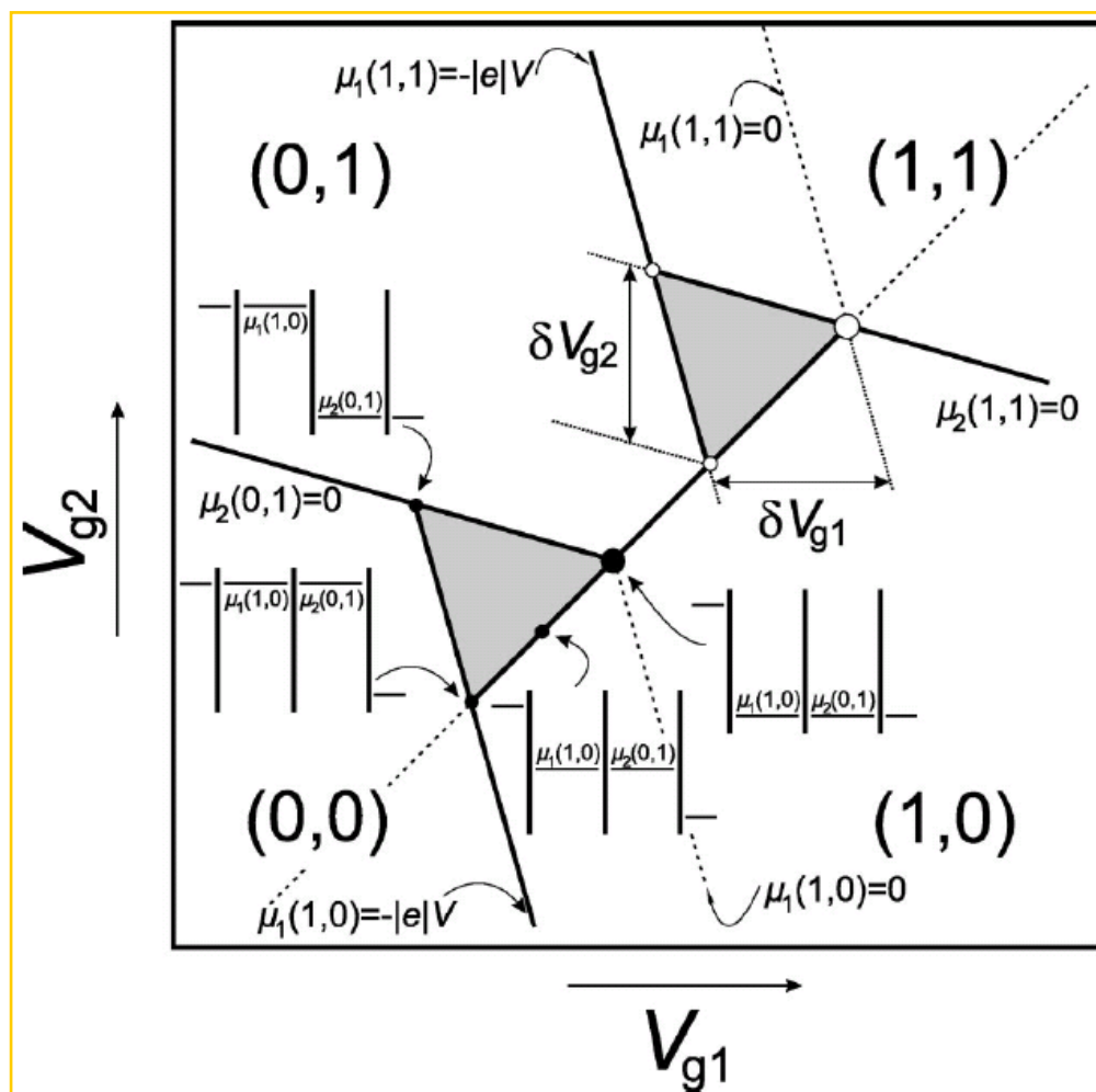
图 1.11 大偏压下，三相点变成偏压三角形。图片引自[40]。
