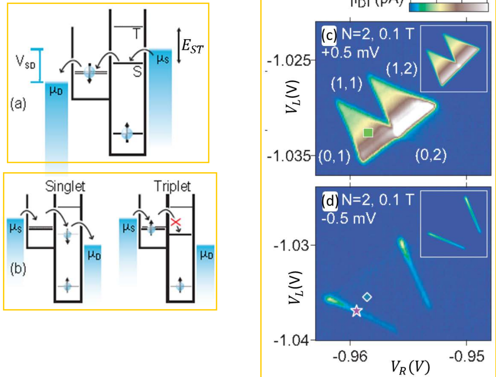
图 2.5 (a) (b) 分别展示了正反偏压下电子隧穿过程。引自[28]。(c) (d) 分别展示了正反偏压下流过量子点的电流。引自[26]
