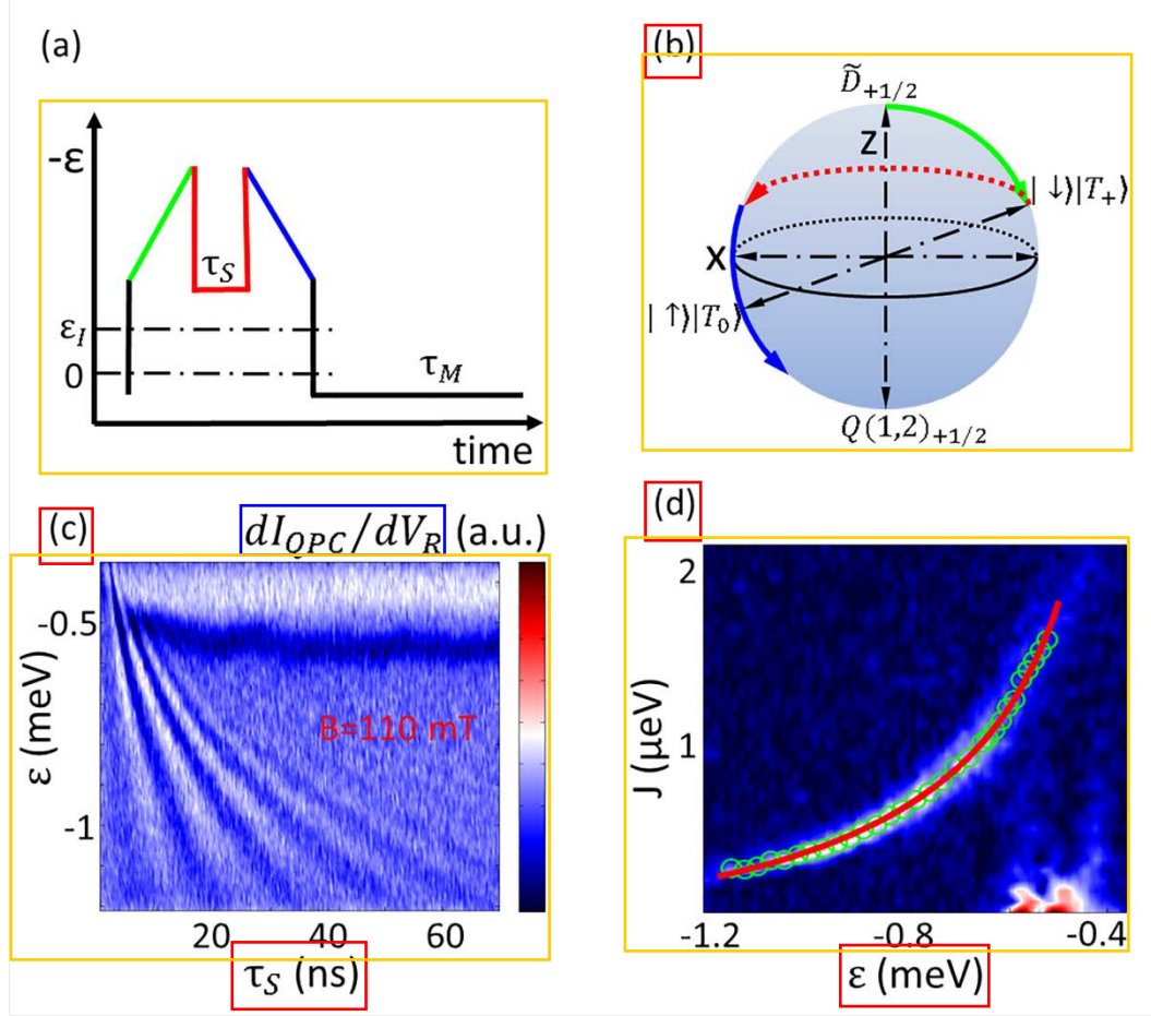
图 3.5 (a) 用于测量交换振荡的失谐脉冲。(b) 态矢量演化的布洛赫球表示。不同颜色的演化轨迹对应着(a)中相应颜色的脉冲阶段。(c) 交换振荡随着交换阶段的失谐 \varepsilon 和持续时间 \tau_S 的变化。磁场 B = 110 \text{ mT} 。(d) (c) 中数据沿 \tau_S 轴的快速傅里叶变换。纵轴已经通过乘以普朗克常数从频率转换为能量。绿色的圆圈是用高斯拟合得到的峰中心。红色曲线是用 J(\varepsilon) 的模型对这些数据做的拟合。拟合结果给出 E_R = 0.27 \text{ } \mu\text{eV} 和 \Delta_s = 21 \text{ } \mu\text{eV} 。
