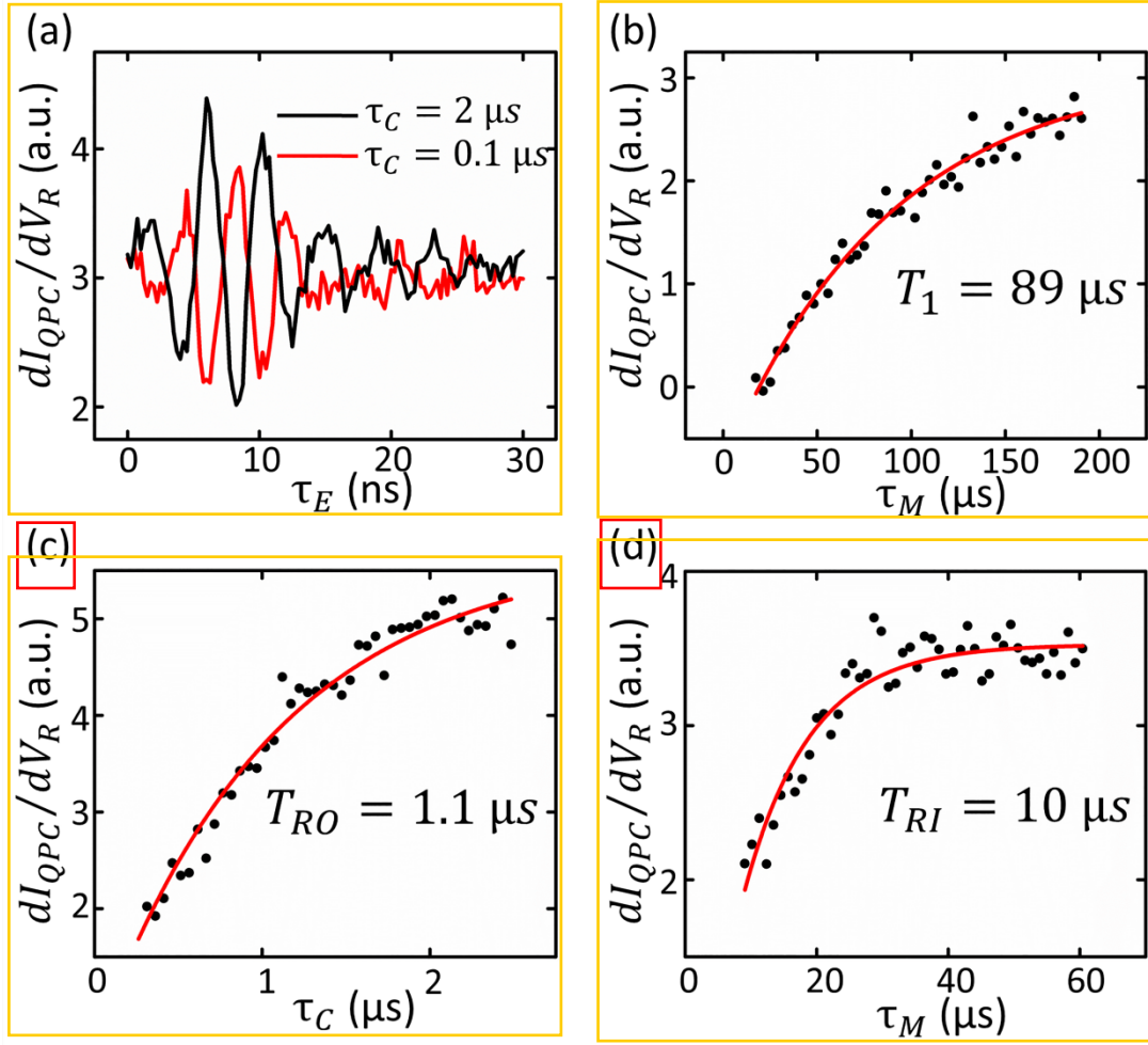
图 4.4 (a) 当 \tau_C = 2 \mu s 和 \tau_C = 0.1 \mu s 时所测得的交换振荡。(b) QPC 互导 dI_{QPC}/dV_R 随 \tau_M 的变化。 \tau_C = 0 。(c) QPC 互导 dI_{QPC}/dV_R 随 \tau_C 的变化。 \tau_M = 10 \mu s 。(d) QPC 互导 dI_{QPC}/dV_R 随 \tau_M 的变化。 \tau_C = 2 \mu s 。(b)-(d) 中的红色曲线是用指数衰减函数 A + B \exp(-\tau/T) 拟合得到的。
