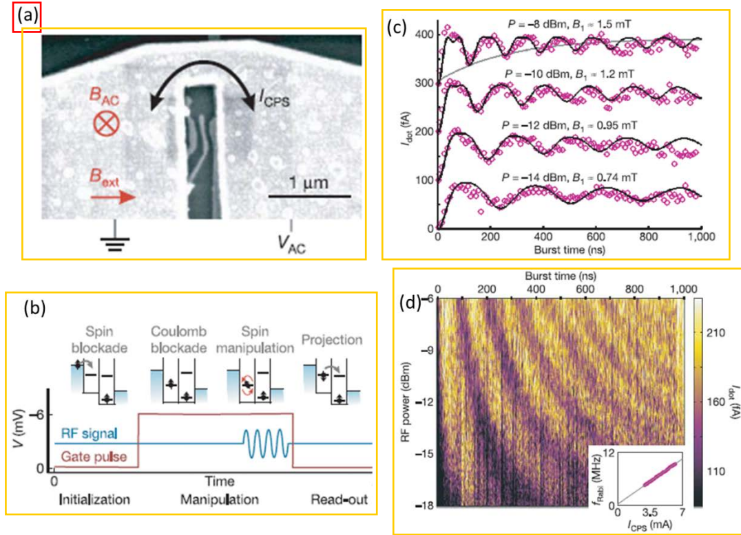
图 2.1 (a) 样品的扫描电镜图片。(b) 操作脉冲序列。(c) 在不同磁场和功率下，通过量子点的电流，随微波脉冲持续时间的变化。(d) 在更大范围功率下，通过量子点的电流，随微波脉冲持续时间的变化。插图显示振荡频率随功率的变化。图片引自 [3]
