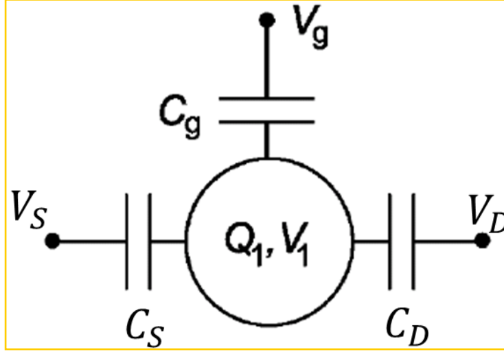
图 1.6 单量子点的等效电路图。量子点和源漏以及栅极的耦合电容分别为 C_S, C_D 和 C_g 。图片引自[40]。
