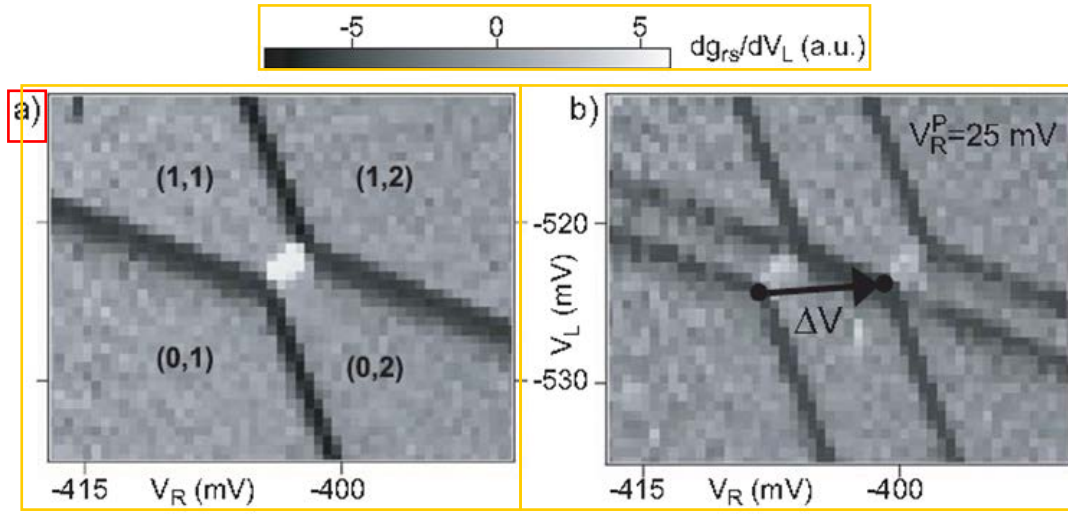
图 2.6 (a) 没有施加脉冲的相图。(b) 在电极 R 上施加一个 25mV, 50% 占空比, 10 \mu s 周期的方波后的相图。图片引自 [29]。
