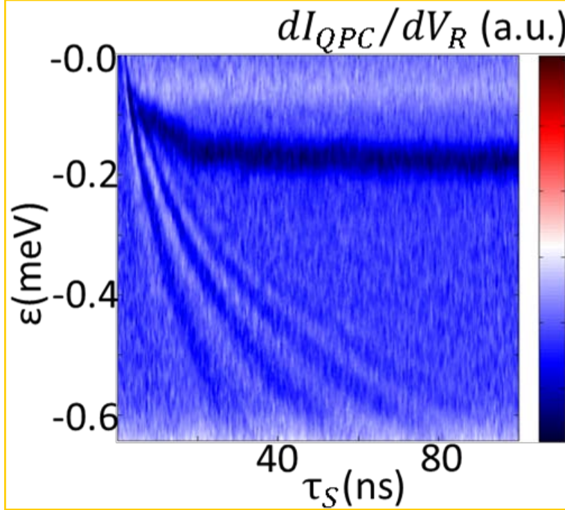
图 2.9 (a) 我们组在 (1, 1)–(2, 0) 区域附近测到的交换振荡。
