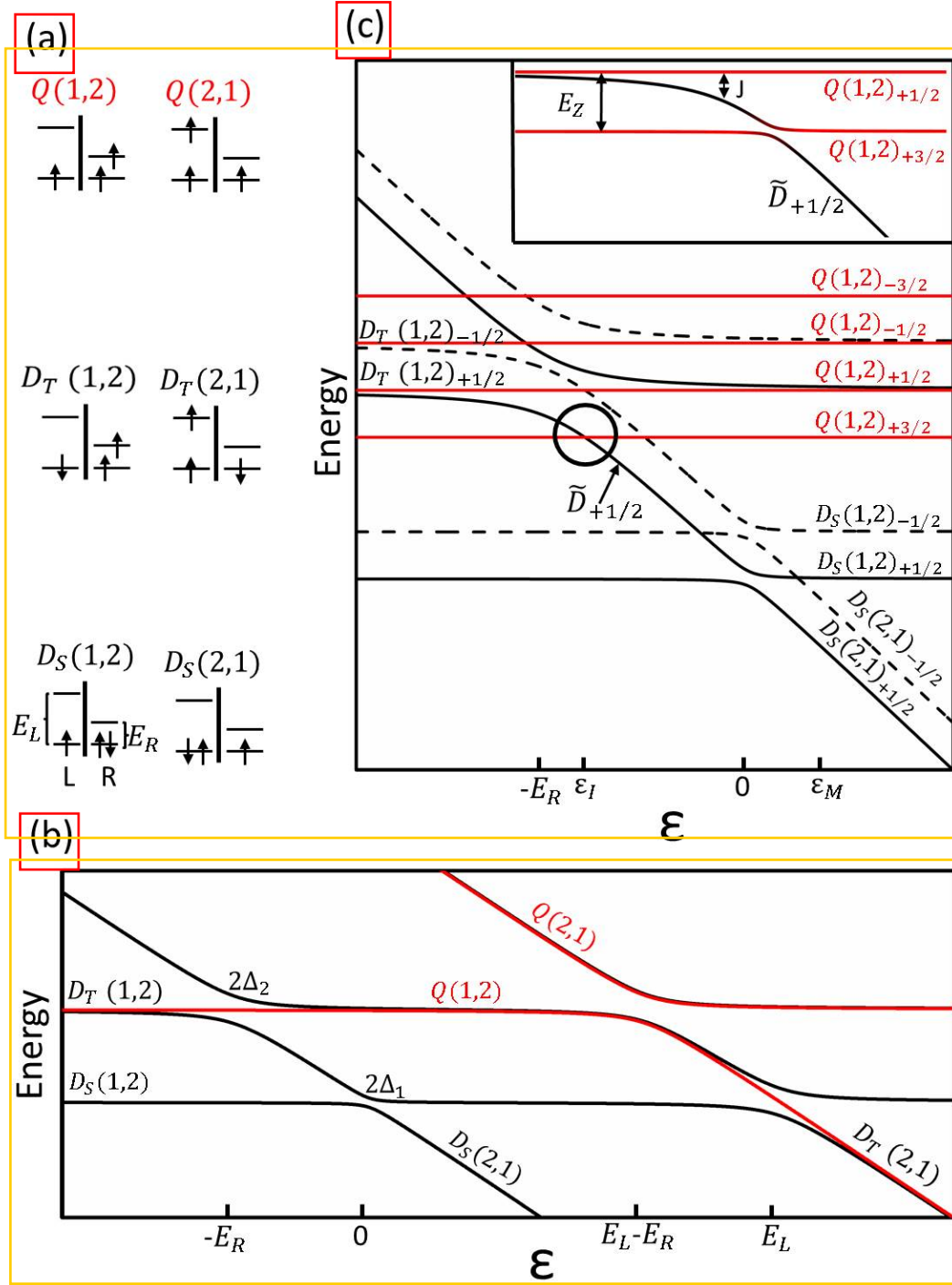
图 3.2 (a)不同自旋和电荷状态的电子轨道填充示意图。只考虑能量最低的状态。(b)磁场 B=0 时，相关能级随失谐变化的示意图。(c) 磁场 B>0 时，相关能级随失谐变化的示意图。只显示失谐 E_L - E_R 左边的区域。插图放大显示了主图黑色圆圈附近的区域，突出了用于相干操作的态和 \tilde{D}_{+1/2} 与 Q(1,2)_{+3/2} 之间的反交叉。
