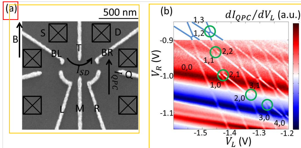
图 5.1 (a) 双点样品的扫描电镜照片。(b) 相图
