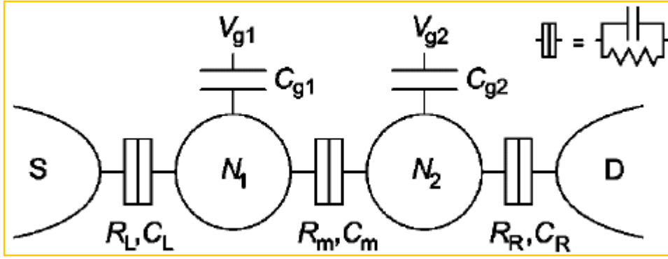
图 1.9(a) 串联双量子点的等效电路图。图片引自[40]。
