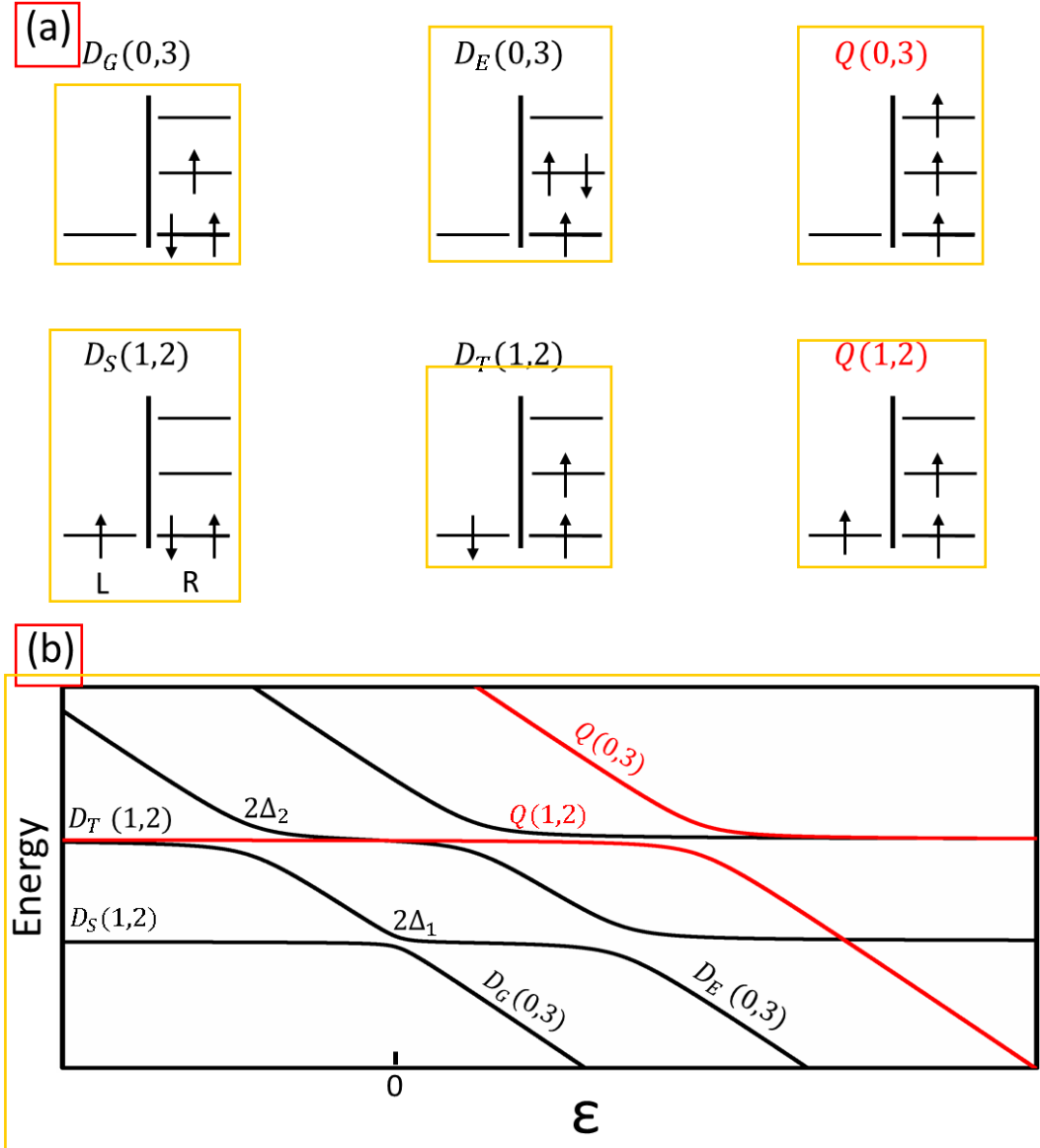
图 3.6 (a)不同自旋和电荷状态的电子轨道填充示意图。(b)磁场 B=0 时, 相关能级随失谐变化的示意图。
