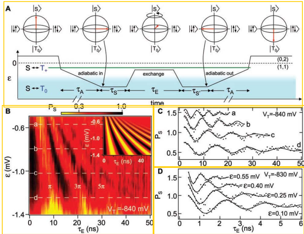
图 2.8 (a) 脉冲序列。(b) 单态概率随脉冲持续时间 \tau_E 和失谐 \varepsilon 的变化。(c) 沿图(b)中白色虚线处的横切，呈现出清晰的振荡。(d) 增大隧穿耦合后所测得的更快频率的振荡。图片引自[5]。
