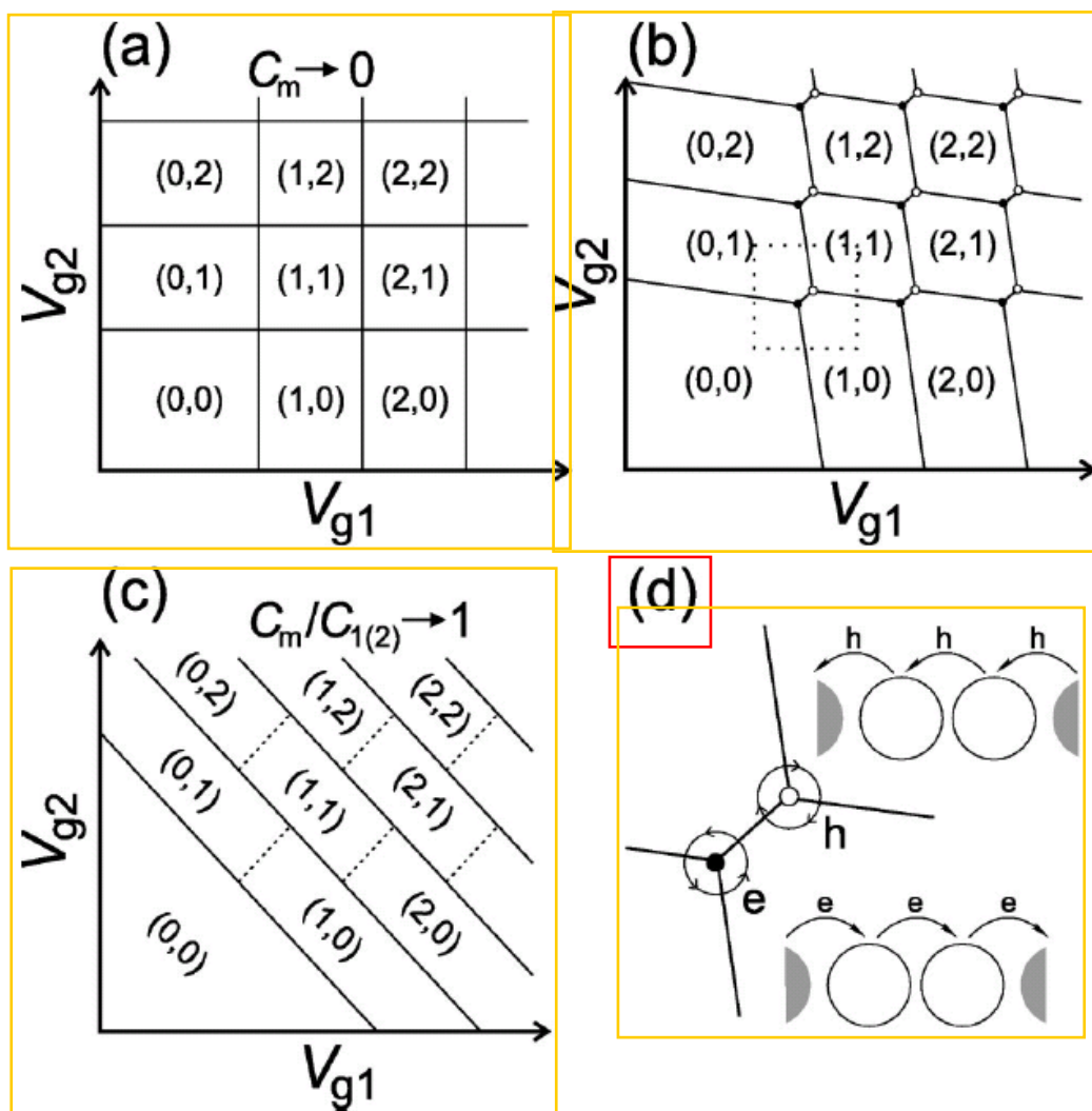
图 1.10 双量子点相图。(a)耦合很弱，双点变成两个孤立的点。(b)耦合中等，也是实验中经常用到的。(c)耦合很大，两个点合并成一个大点。(d)电子和空穴输运过程示意图。图片引自[40]。
