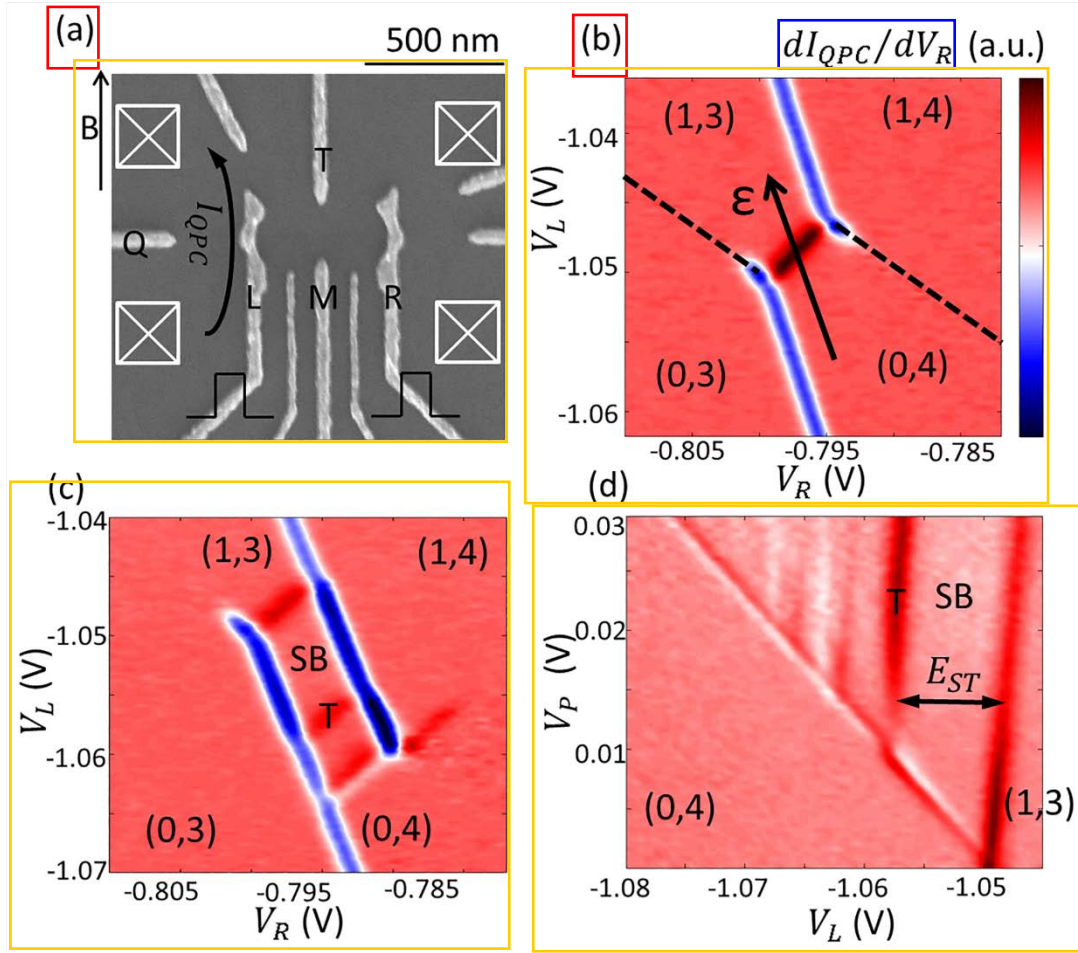
图 4.1 (a) 双点样品的扫描电镜图片。(b) (1,3)-(0,4)区域的相图。(c) 在施加一个方波失谐脉冲时的相图。(d) QPC 互导 dI_{QPC}/dV_R 随着脉冲幅度 V_P 和基准失谐在 V_L 上的分量的变化。
