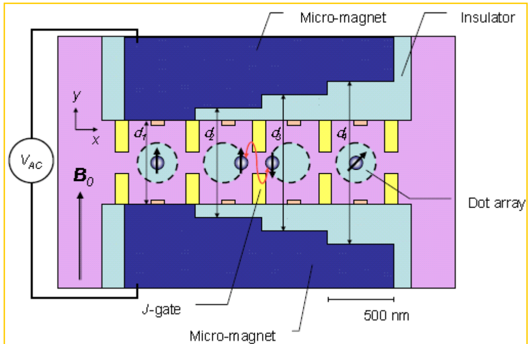
图 2.2 采用微磁体的单自旋比特集成方案。图片引自 [20]
