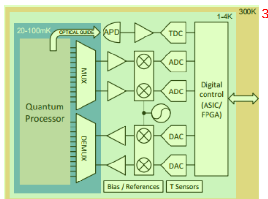
图 5.2: 量子计算机经典单个通道接口的构想图。图片引用于[5]
