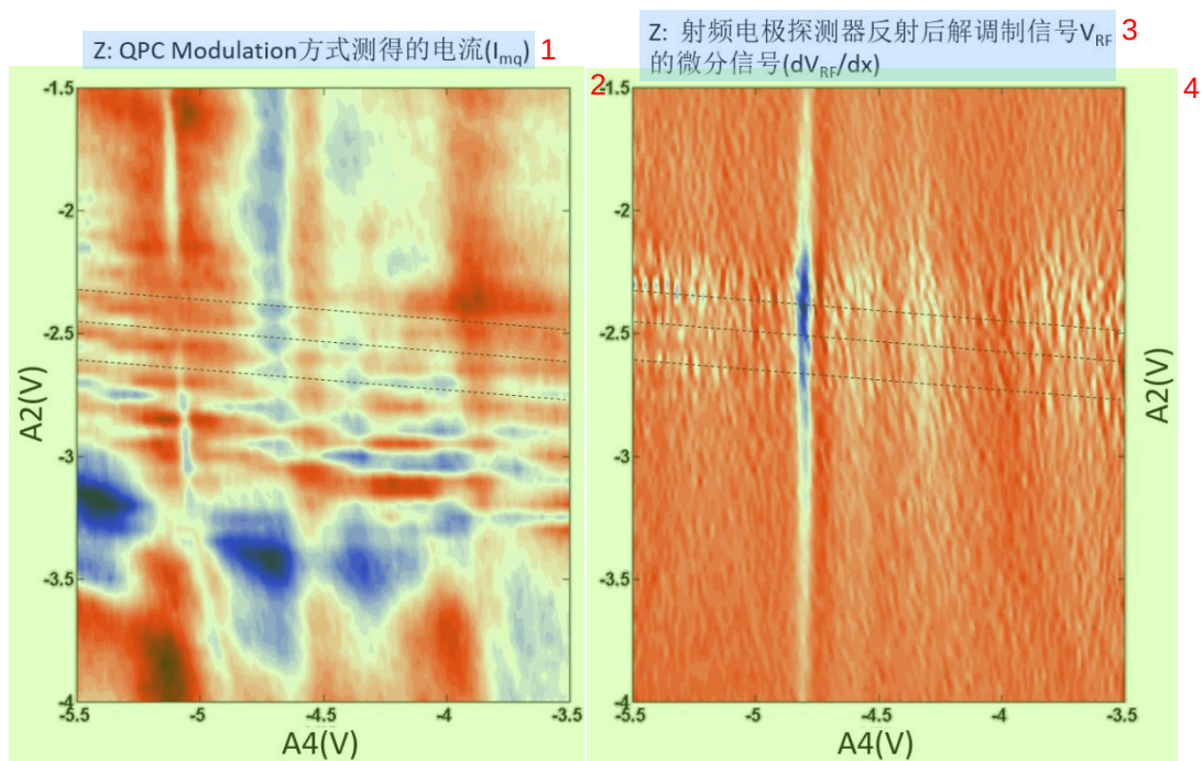
图 3.20: 调节背栅电极, 测量量子点接触输运信号和网分测得的信号, 归一化处理之后 5
