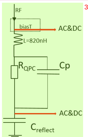
图 3.22: 射频反射式测量电路示意图。 4
