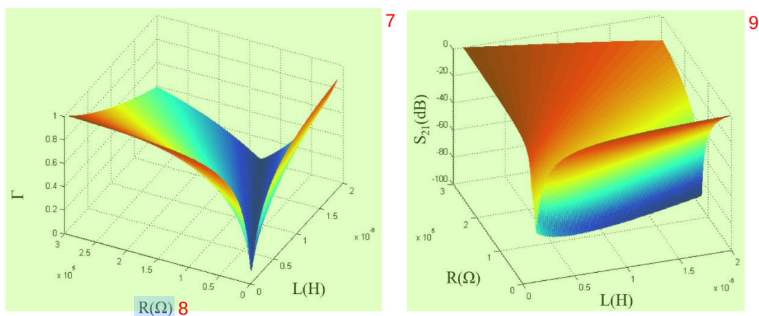
图 3.24: C_p=0.3\text{pF} , 不考虑 C_{\text{reflect}} 时, QPC 电阻 R 、电感 L 与反射系数 \Gamma 和 S 参数的三维关系图。
