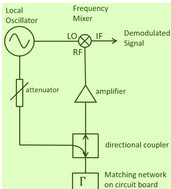
图 3.3: 测量系统信号放大、调制解调示意图。
