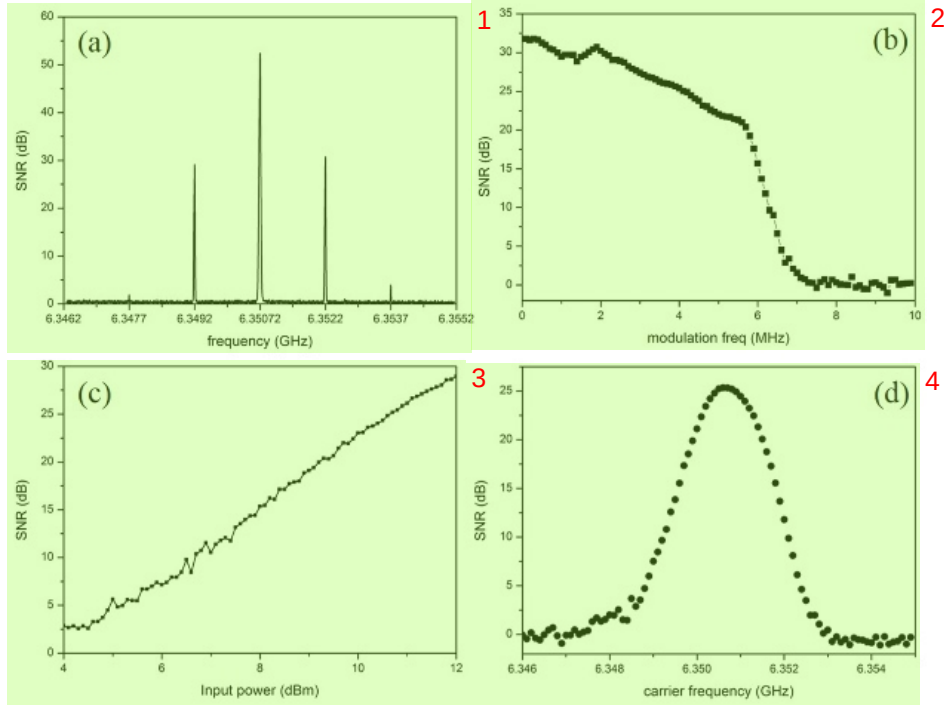
图 4.5: 反射式超导谐振腔作为探测器的性质表征图。
