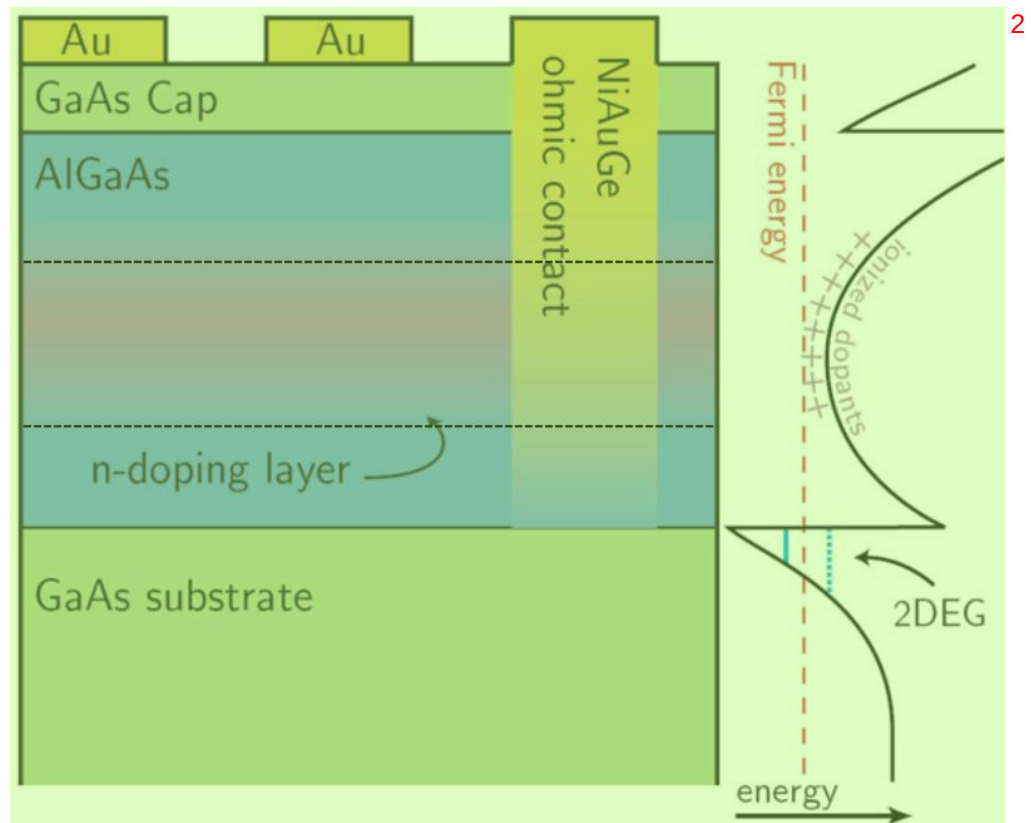
图 1.3: GaAs/AlGaAs 结构和对应的能带结构图。 3
