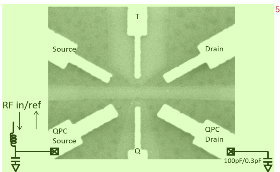
图 3.12: 石墨烯单量子点样品图。实际上是两个单量子点，下面的量子点作为量子点接
