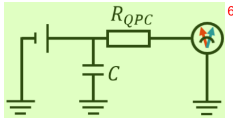
图 3.1: 量子点接触探测的等效电路示意图。 7
