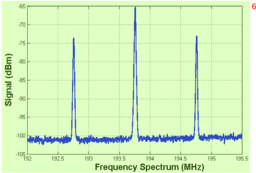
图 3.9: 在量子点的电极 LB 上叠加 1MHz 幅度 20mV 的方波形, 在未解调之前使用频谱仪探测的反射射频信号频谱。频谱仪的分辨带宽设为常用的 10kHz。
