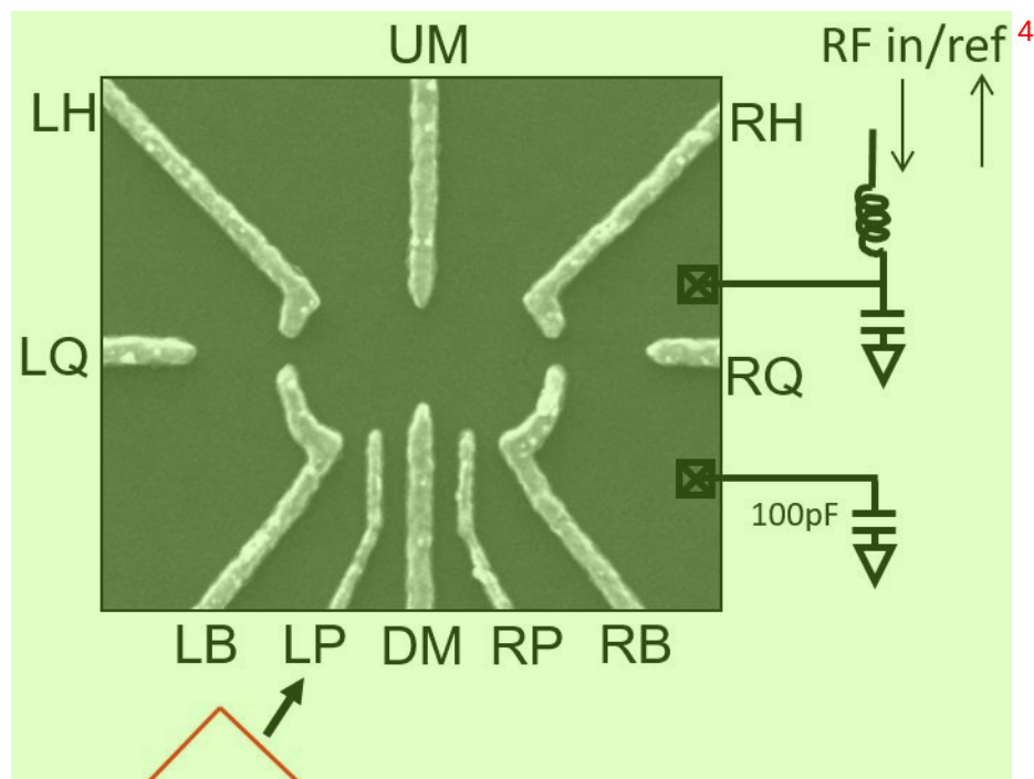
图 4.1: 快速测量样品连接示意图，红色的三角波叠加在电极 LP 上。 5
