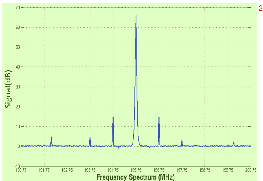
图 3.13: 在电极 Q 上施加了 1MHz, 1Vpp 的方波进行调制, 测得的频谱。 3
