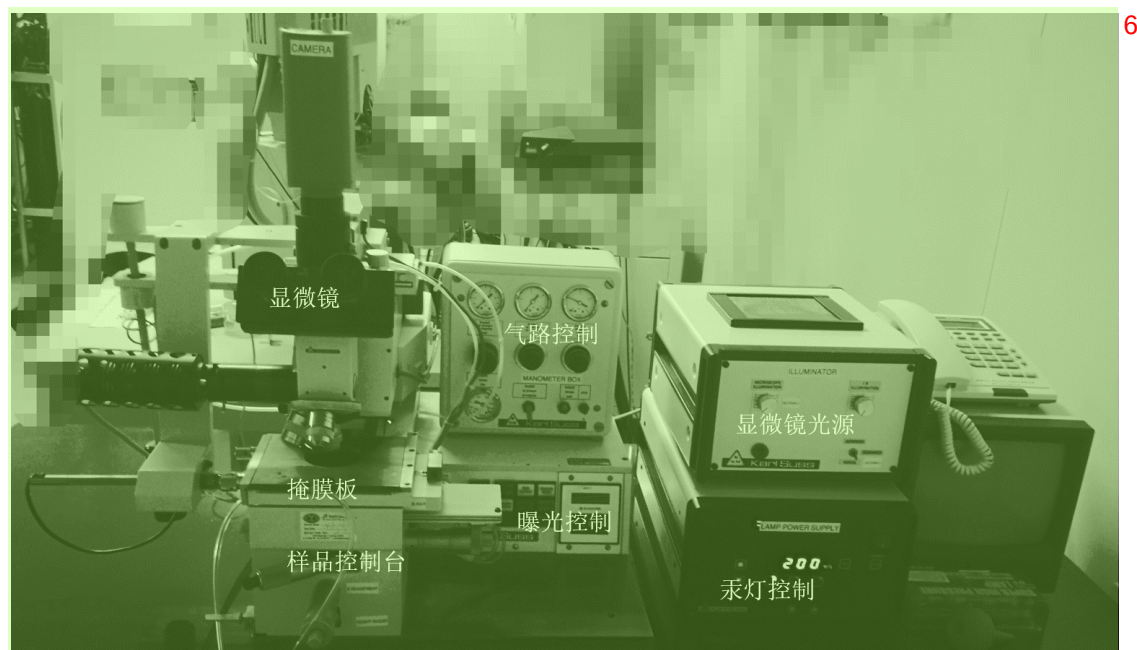
图 A.1: MJB3 型接触式紫外光刻机。 7
