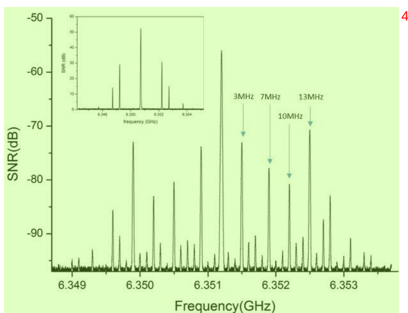
图 4.8: 在 4 个电极输入不同频率的三角波进行调制。内置图为电极 V_{1L} \sim 1\text{MHz} , 300\text{mV}_{pp} 的三角波, V_{2L} \sim 1.5\text{MHz} , 300\text{mV}_{pp} 的三角波时, 所得到的的频谱图。 5
