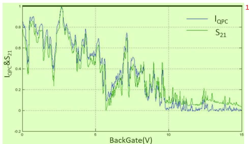
图 3.16: 调节背栅电极, 测量量子点接触输运信号和网分测得的信号, 归一化处理之后得到的对比图。 2
