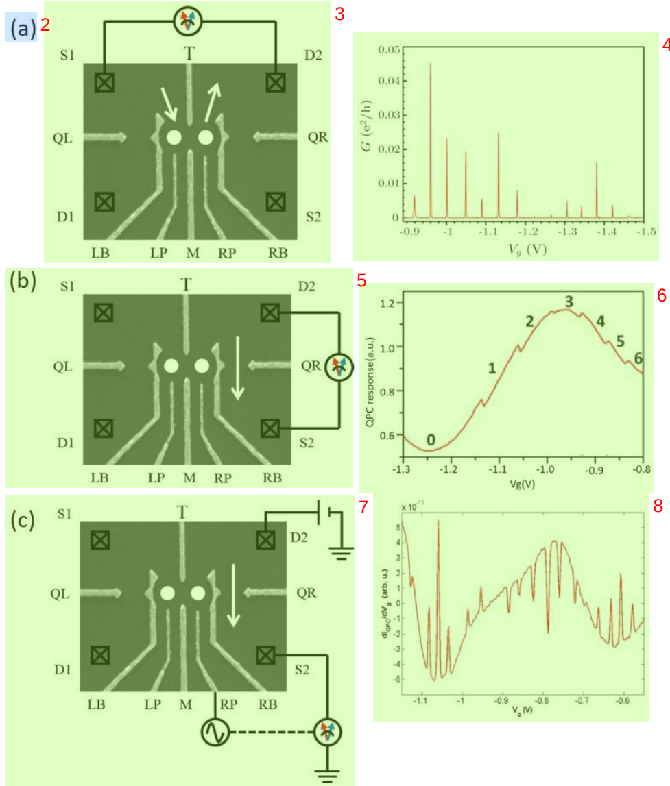
图 2.5: (a) 量子点通道输运测量电路、样品连接示意图和测得信号示意图, (b) 量子点接触输运测量电路、样品连接示意图和测得信号示意图, (c) 量子点接触调制测量电路、样品连接示意图和测得信号示意图。
