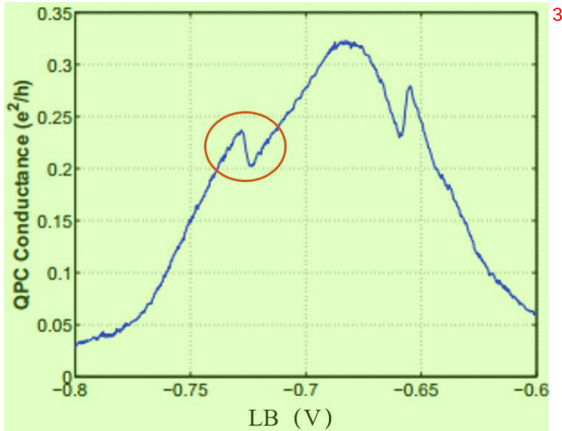
图 3.10: 调节电极 LB，测量 QPC 的电导变化。 4
