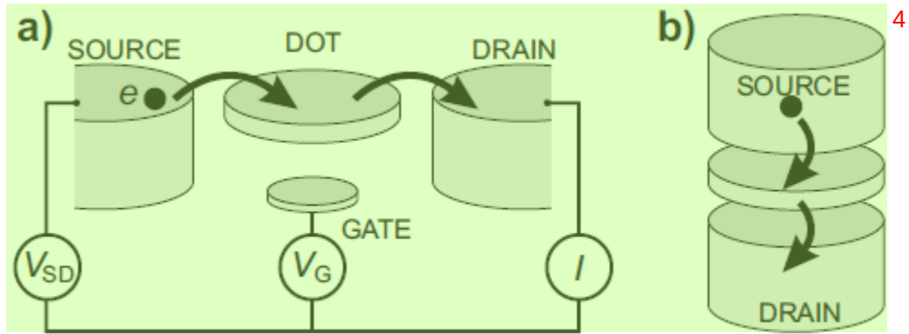
图 1.4: (a)横向量子点, (b)纵向量子点。图片引自文献[58]。 5
