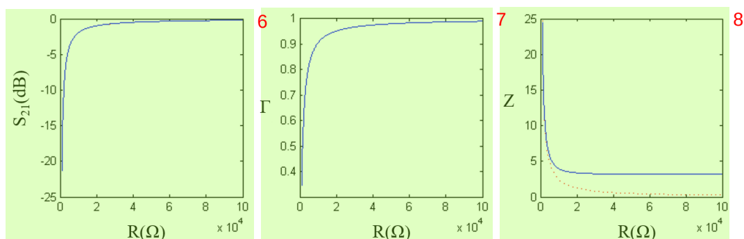
图 3.26: C_p=4\text{pF} , L=820\text{nH} 时 QPC 电阻 R 与 S 参数、反射系数 \Gamma 和阻抗 Z 的关系图。(蓝线为第一种模型, 红色虚线为第二种模型)
