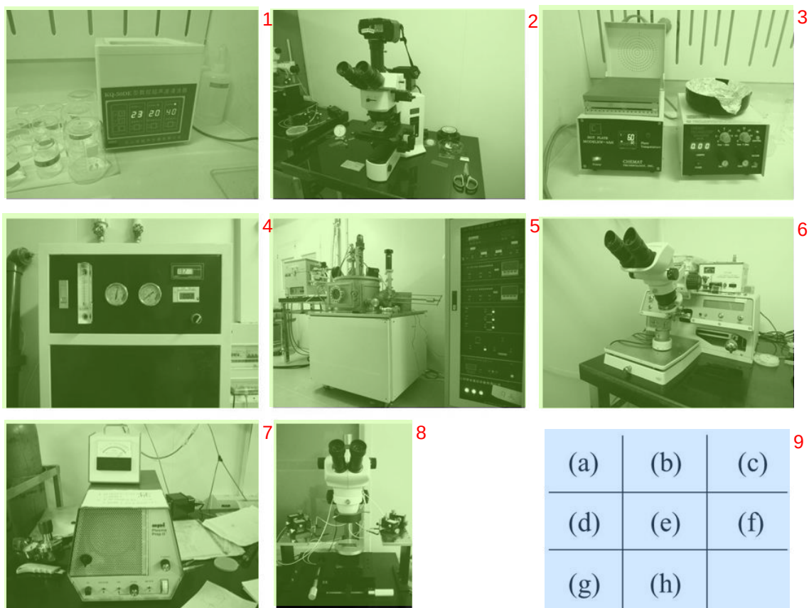
图 A.7: (a)超声清洗, (b)奥林巴斯光学显微镜, (c)烤胶机和匀胶机, (d)去离子水过滤器, (e)快速退火炉, (f)West Bond 焊线机, (g)等离子体清洗机, (h)探针台。
