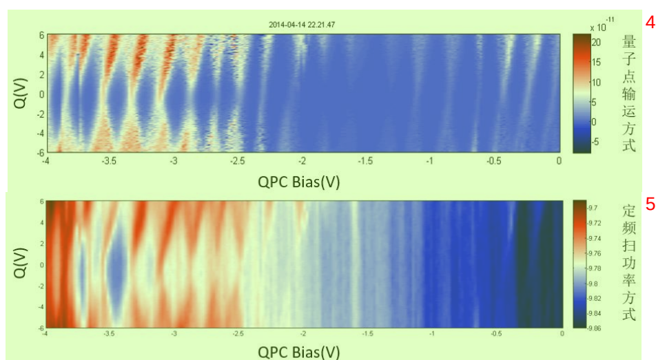
图 3.17: 使用传统量子点输运方式和网络分析仪定频扫功率方式分别得到的库仑菱形图。 6
