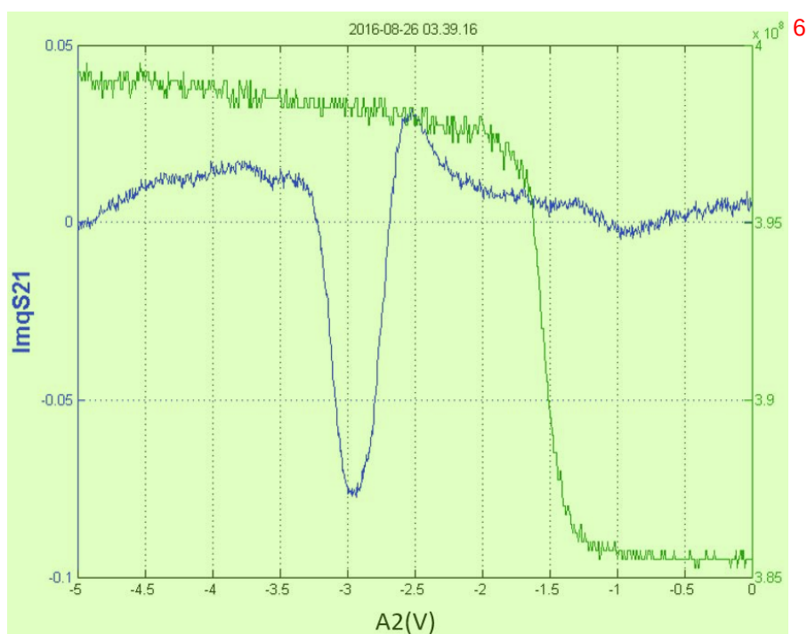
图 3.21: 调节连接在射频反射式电路上的电极 A2 , 测量量子点接触 modulation 信号和射频反射后网络分析仪测得的信号对应的响应范围。 7
