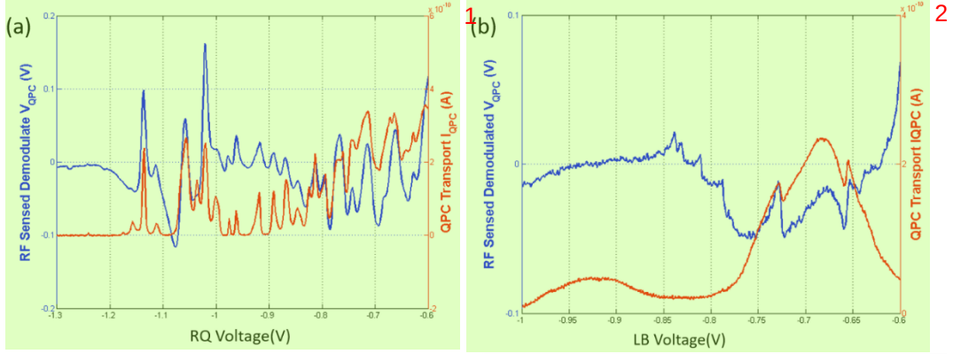
图 3.8: 检测反射射频信号经过解调之后的电压 V_{rf} 与量子点接触的电流 I_{QPC} 是否可以一一对应。(a) 调节直接影响量子点接触的电极 RQ, 测量两种信号。(b) 调节非直接影响量子点接触的电极 LB, 测量两种信号。
