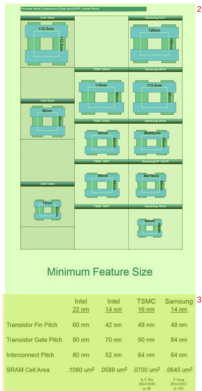
图1.1 近些年各大厂商所使用的不同工艺的晶体管面积对比 (Intel因特尔, TSMC台积电, Samsung三星)
