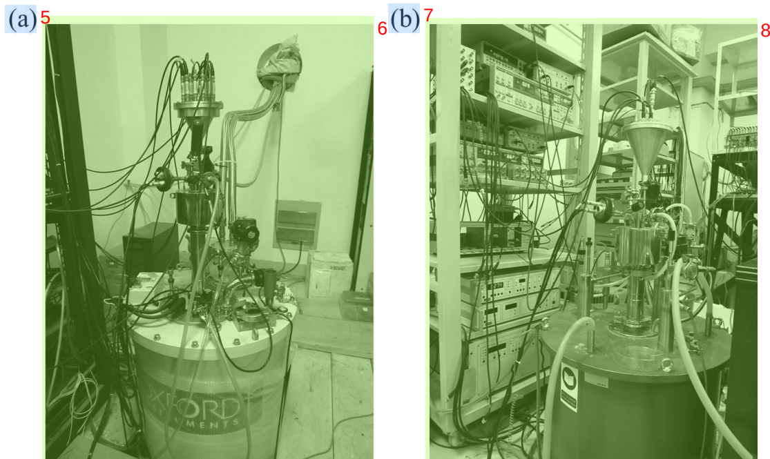
图 2.2: (a)自冷凝 He3 制冷剂(b)液氮夹层 He3 制冷机。 9
