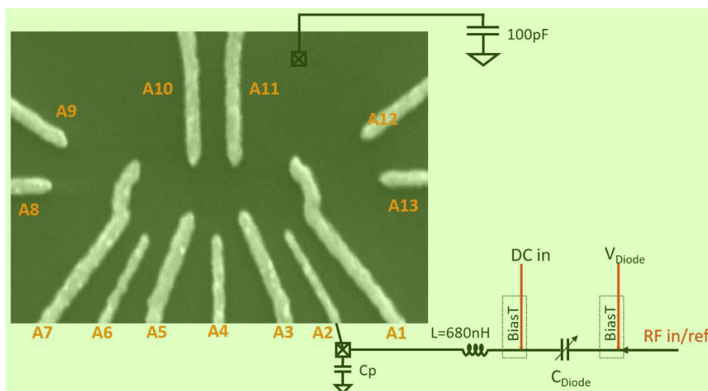
图 3.18: 射频反射式电路与量子点电极连接的示意图。 4
