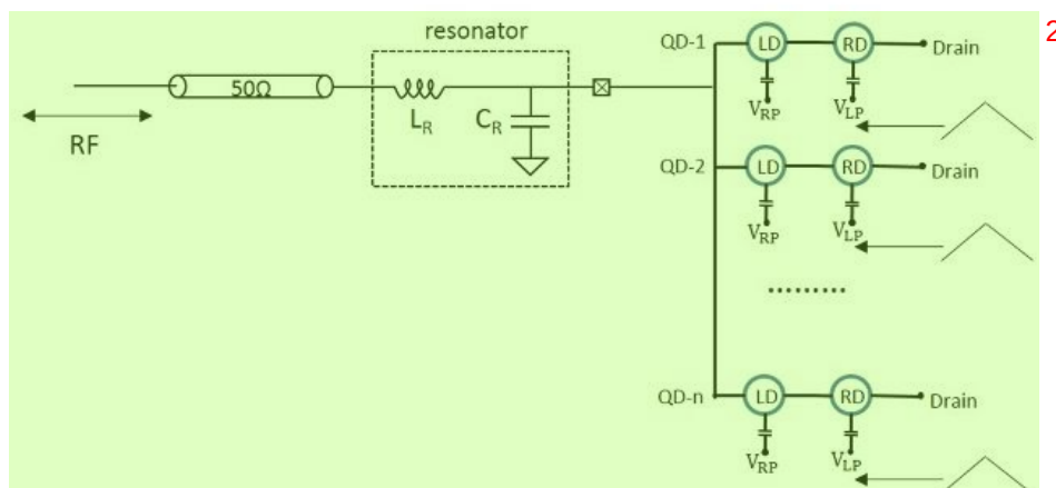
图 4.7: 多通道 Multiplex 读取示意图。 3
