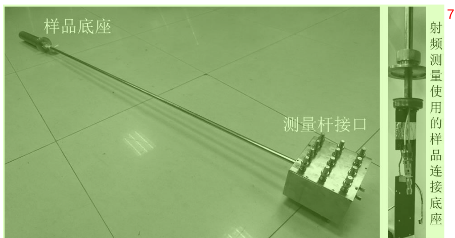
图 2.1: 4.2K 射频测量使用的初步测量杆。 8
