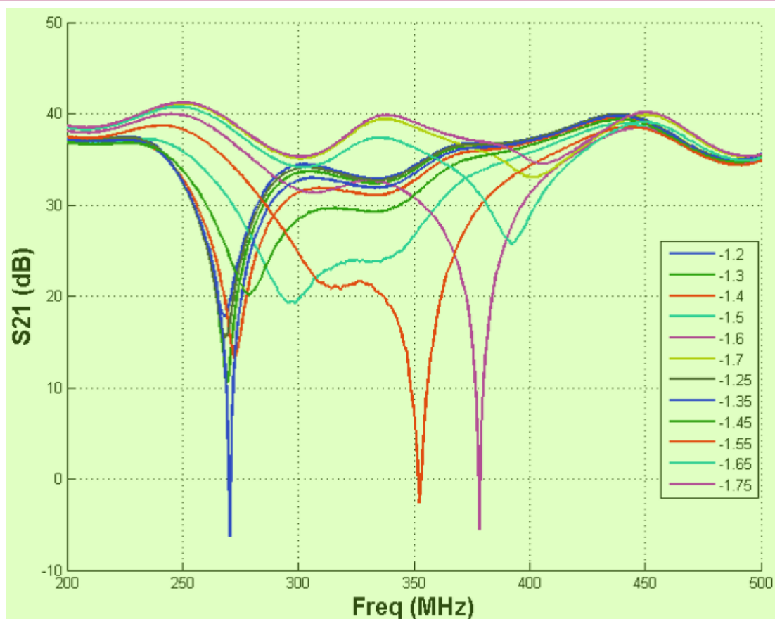
图 3.19: 改变电极 A1 的电压，从 -1.2V ~ -1.75V，我们得到的 S 参数曲线。 4
