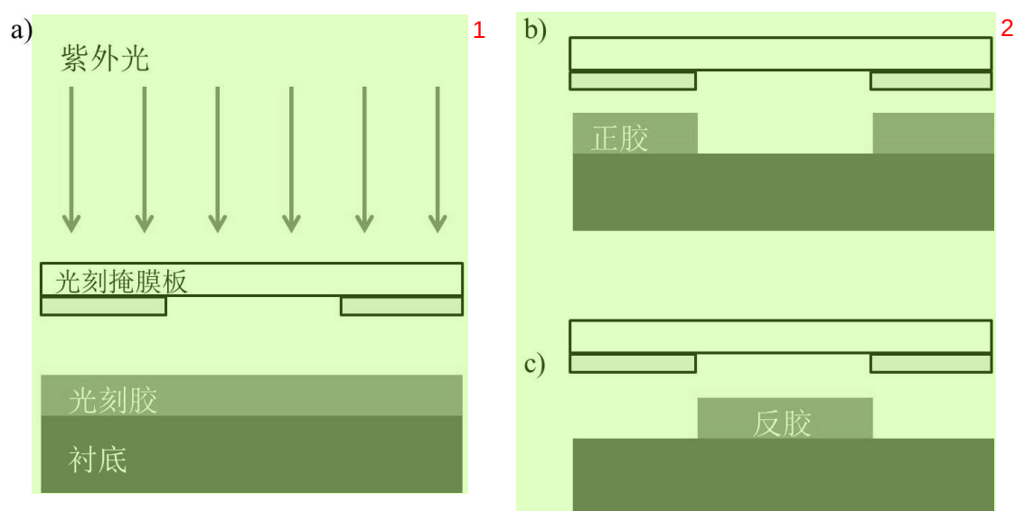
图 A.2: 光刻的基本原理。(a)紫外曝光；(b)正胶曝光示意图；(c)反胶曝光示意图。
