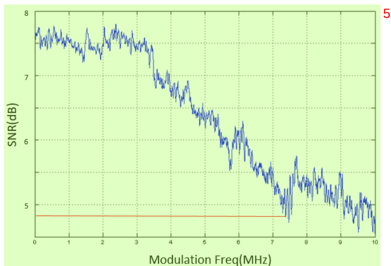
图 3.14: 扫描施加在电极 T 上调制信号的调制频率, 测量其中一个边带的信噪比, 得到的关系图。 6
