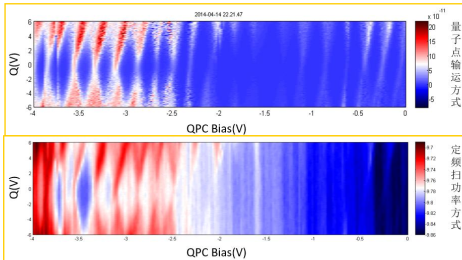
图 3.17: 使用传统量子点输运方式和网络分析仪定频扫功率方式分别得到的库仑菱形图。
