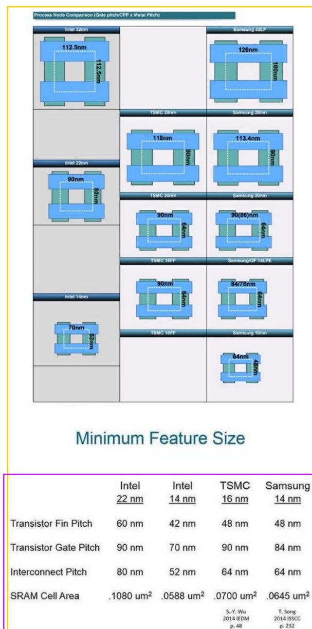
图1.1 近些年各大厂商所使用的不同工艺的晶体管面积对比 (Intel因特尔, TSMC台积电, Samsung三星)
