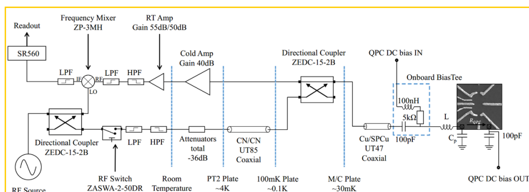
图 3.4: 在干式稀释制冷机中所搭建的射频反射式测量系统的电路示意。
