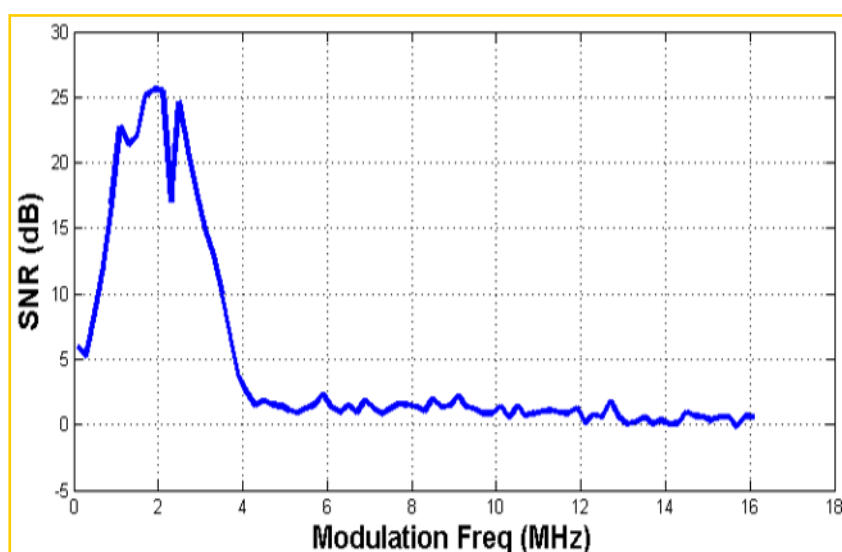
图 3.11: 其中一个边带(Sideband)的信噪比随施加在电极 LB 上的方波调制频率的变化关系
