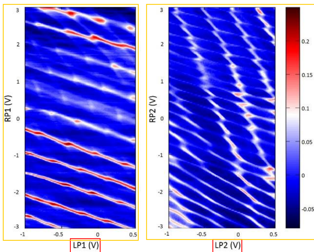
图 4.6: 在每个量子点的电极上施加不同频率的三角波: V_{1L} \sim 17\text{Hz} , 300\text{mV}_{pp} 的三角波, V_{2L} \sim 247\text{Hz} , 300\text{mV}_{pp} 的三角波。解调并滤波放大之后由示波器两个不同通道同时采集得到的相图。
