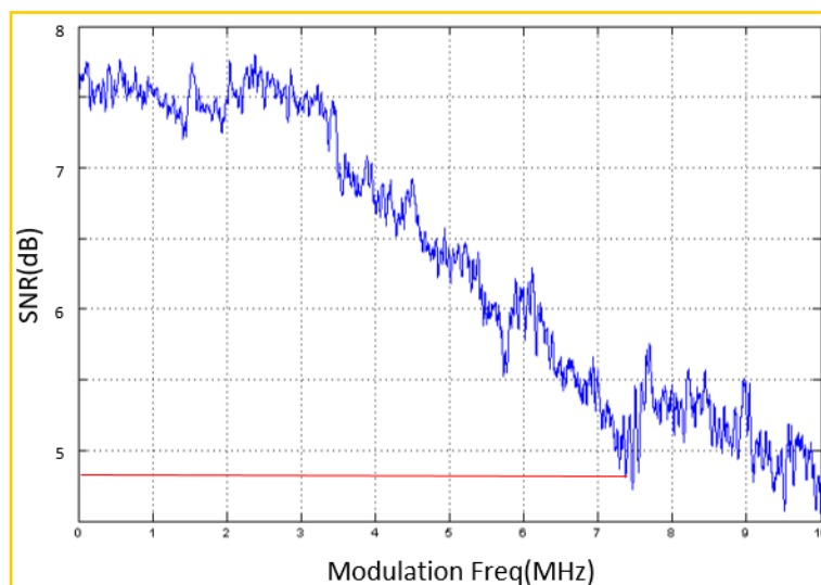
图 3.14: 扫描施加在电极 T 上调制信号的调制频率, 测量其中一个边带的信噪比, 得到的关系图。
