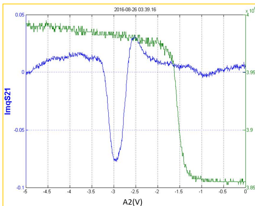
图 3.21: 调节连接在射频反射式电路上的电极 A2, 测量量子点接触 modulation 信号和射频反射后网络分析仪测得的信号对应的响应范围。
