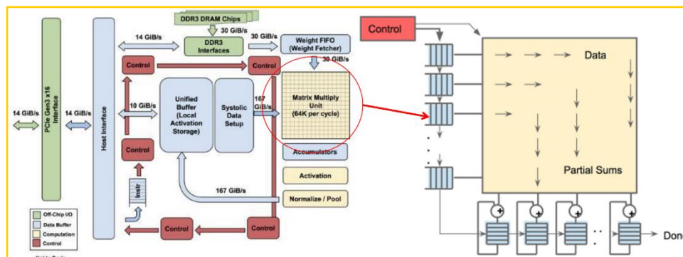
图 5.3: 谷歌生产的 TPU 的架构图，其中左面画红圈的部分在右边有详细的结构，叫乘法矩阵单元 Matrix Multiply Unit。图片引用于[6]。
