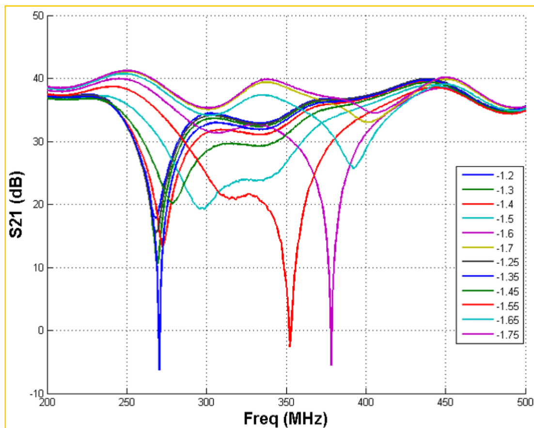
图 3.19: 改变电极 A1 的电压，从 -1.2V ~ -1.75V，我们得到的 S 参数曲线。
