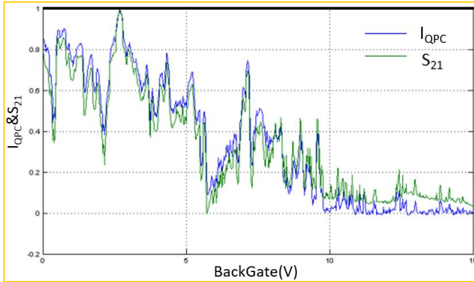
图 3.16: 调节背栅电极，测量量子点接触输运信号和网分测得的信号，归一化处理之后得到的对比图。
