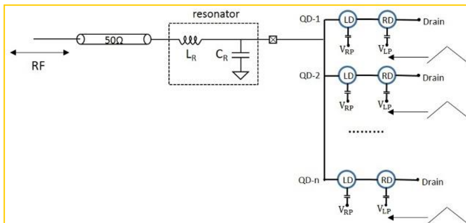
图 4.7: 多通道 Multiplex 读取示意图。
