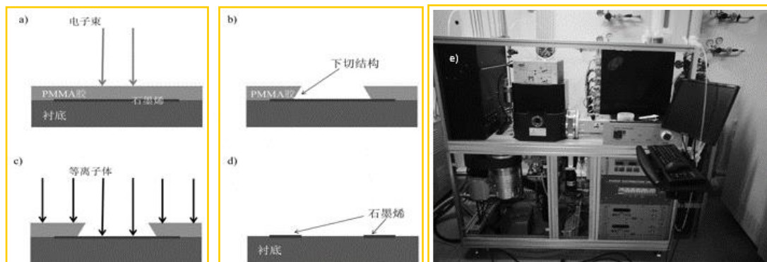
图 A.6: (a) 电子束曝光示意图; (b) 显影之后示意图; (c) 等离子体刻蚀; (d) 清洗之后, 得到图形化的石墨烯; (e) 等离子体刻蚀机系统照片。
