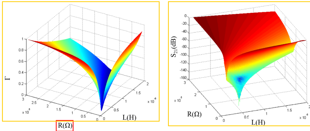
图 3.25: C_p=0.3\text{pF} , 考虑 C_{\text{reflect}} 时, QPC 电阻 R 、电感 L 与反射系数 \Gamma 和 S 参数的三维关系图。
