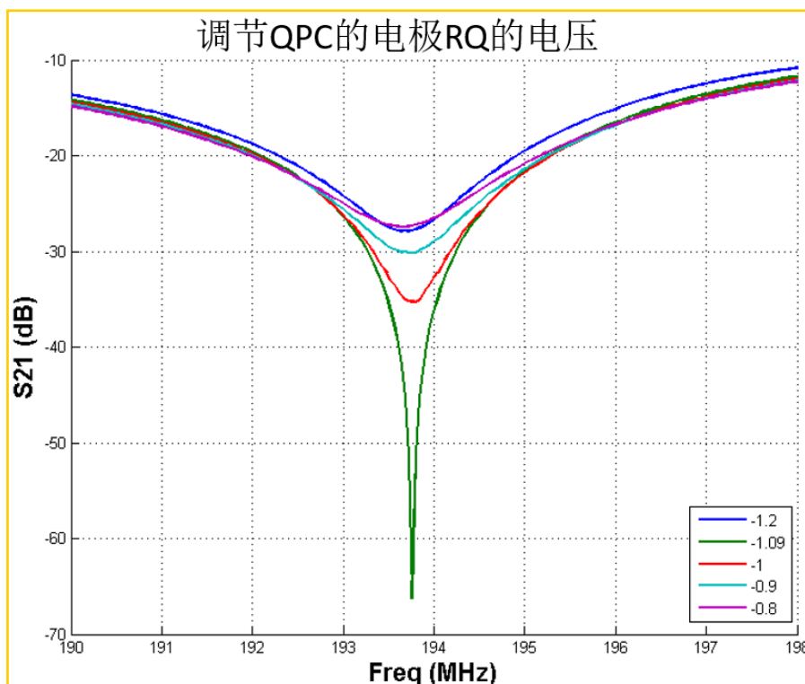
图 3.7: 调节量子点接触的电极 RQ 的电压，测得 S 参数曲线随电极 RQ 电压的变化趋势。电路的谐振频率 f_0 = 193.8\text{MHz} 。
