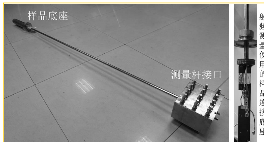
图 2.1: 4.2K 射频测量使用的初步测量杆。
