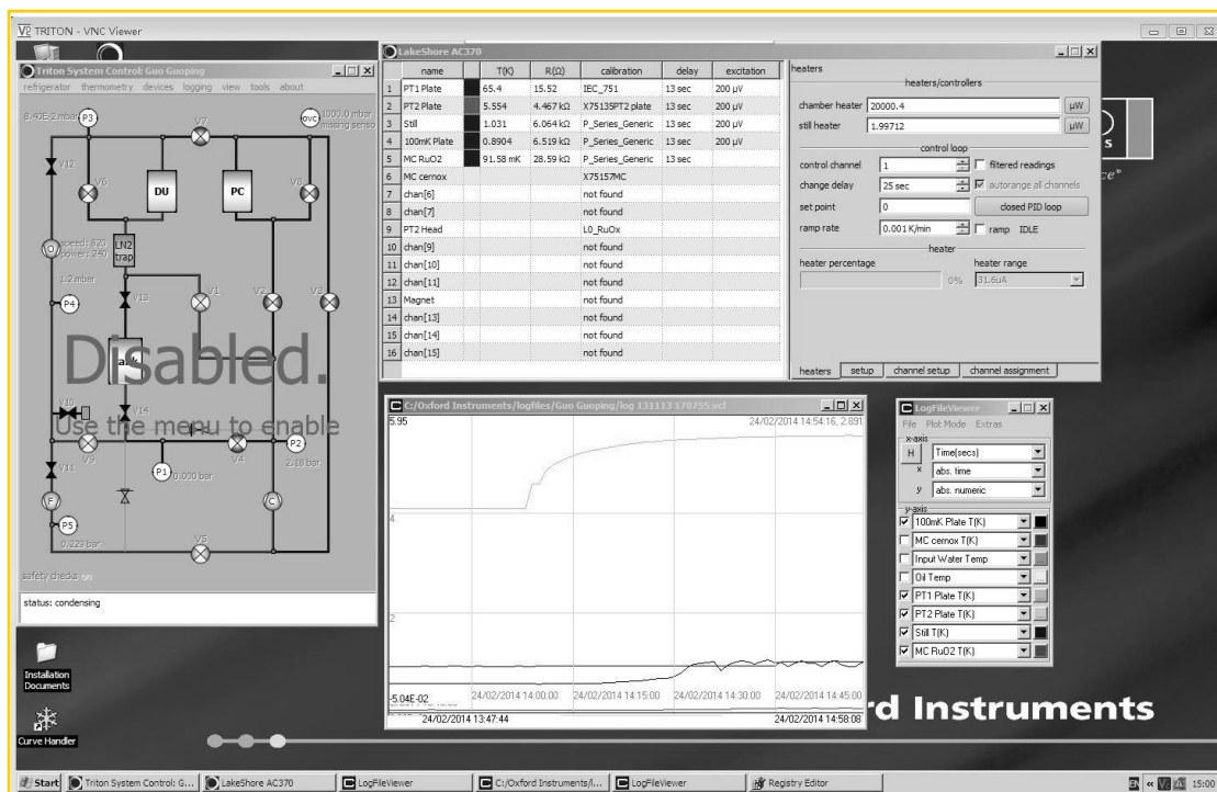
图 2.4: Triton2 进行线路改造，并打开 0.5W 的低温放大器后，无液氮稀释制冷机系统的运行状态。
