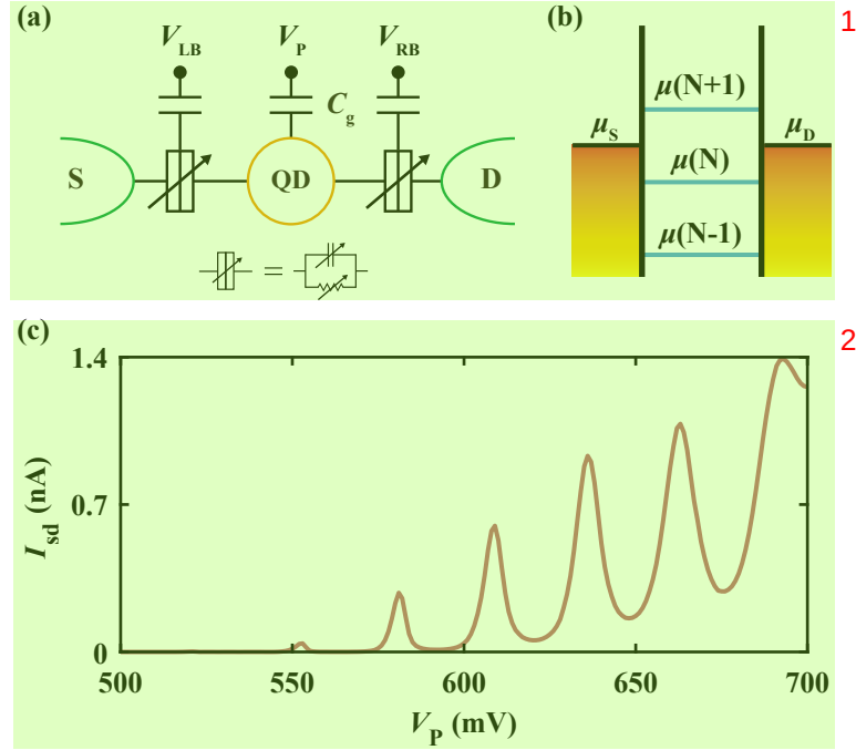
图 2.5 (a) 单量子点电路模型示意图 (b) 单量子点电化学势示意图。(c) 实验测量得到的量子点的库仑峰。
