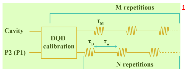
图 5.10 量子比特操作线路示意图，在进行操作之前，需要对量子点进行校准。这里可以通过施加不同的微波序列来实现对量子比特的不同操作。这里的等待时间 \tau_w ，测量时间 \tau_M ，以及施加微波 \tau_B 的时间根据不同的实验需求而确定。图中 M 和 N 表示当前循环的执行次数，也会根据实际情况选取合适的值。
