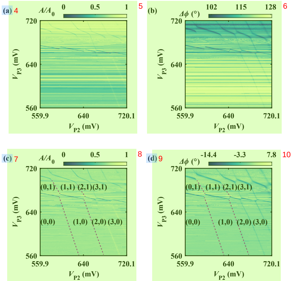
图 4.6 用谐振腔测量得到的 RDQD 稳定性图谱。(a) 谐振腔归一化幅值 A/A_0 与量子点电极电压 V_{P2} 和 V_{P3} 的关系。(b) 谐振腔相位响应 \Delta\phi 与量子点电极电压 V_{P2} 和 V_{P3} 的关系。(c) - (d) 为去除本底后的谐振腔响应信号，数字标识了该区域的电子数目。
