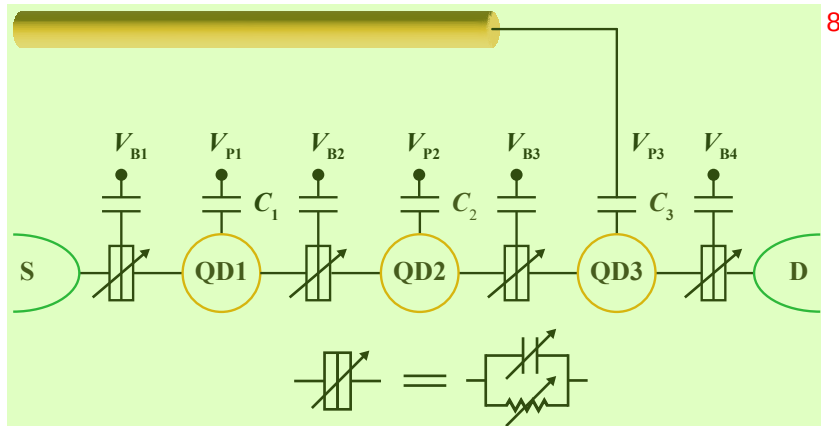
图 6.3 量子点与谐振腔耦合示意图。 9
