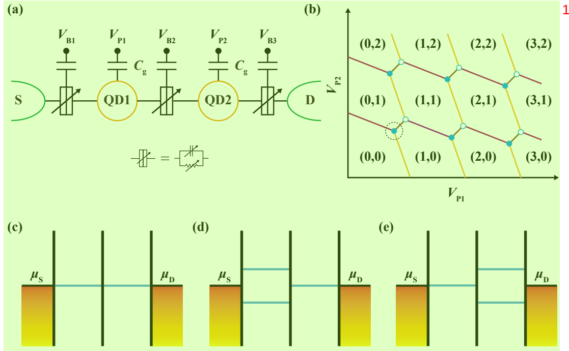
图 2.6 (a) 由 QD1 和 QD2 串联组成的双量子点的电路模型示意图。(b) 双量子点电荷稳定性图谱示意图, 量子点中的电子数目受到电极电压 V_{P1} 和 V_{P2} 的控制。(c) 三相点处的量子点能级示意图。(d) 量子点 QD2 与源漏对齐的能级示意图, 在 (a) 中用紫色线表示。(e) 量子点 QD1 与源漏对齐的能级示意图, 在 (a) 中用橙色线表示。
