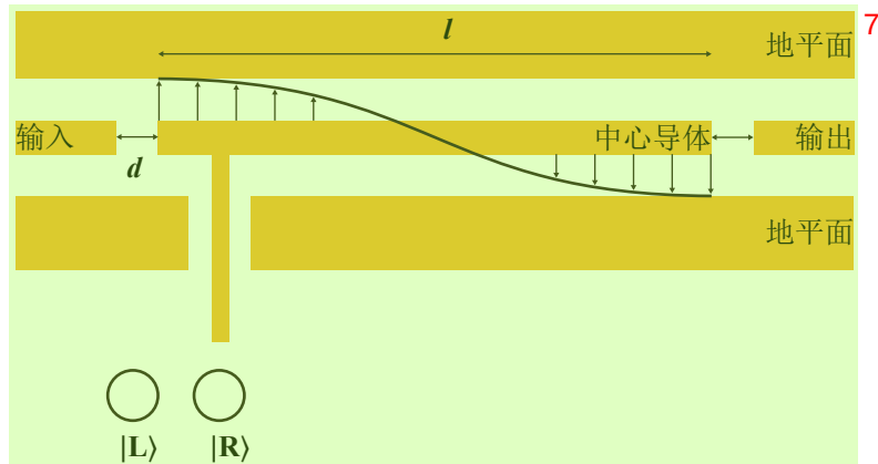
图 2.9 双量子点与谐振腔耦合的结构示意图
