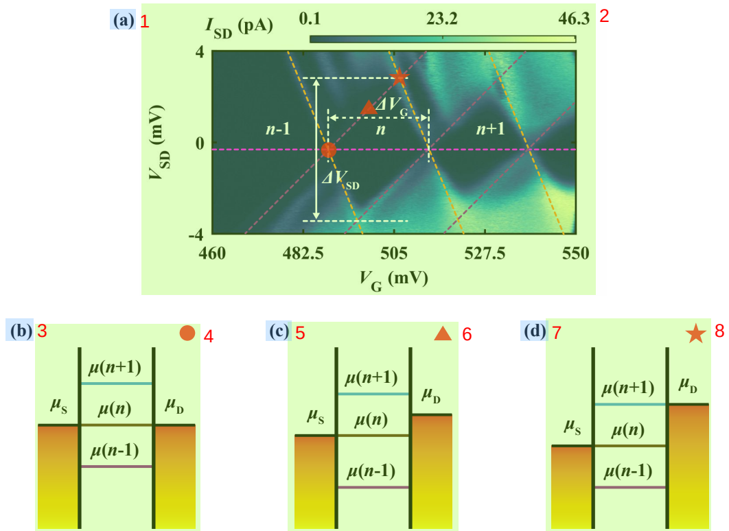
图 4.4 利用库仑菱形测量量子点电极的 lever arm。 n 表示量子点中的电子数目， \Delta V_G 和 \Delta V_{SD} 分别表示栅极和源漏偏置电压的变化量。紫色和橙色虚线标识出了量子点的电化学势和源漏电化学势对齐的情况。(b) - (d) 分别给出了 (a) 中红色圆形、三角形、五角星标识位置的电化学势情况。
