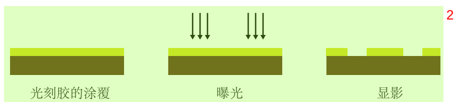
图 3.2 光刻工艺过程示意图，包括光刻胶的涂覆、曝光以及显影三个步骤。 3
