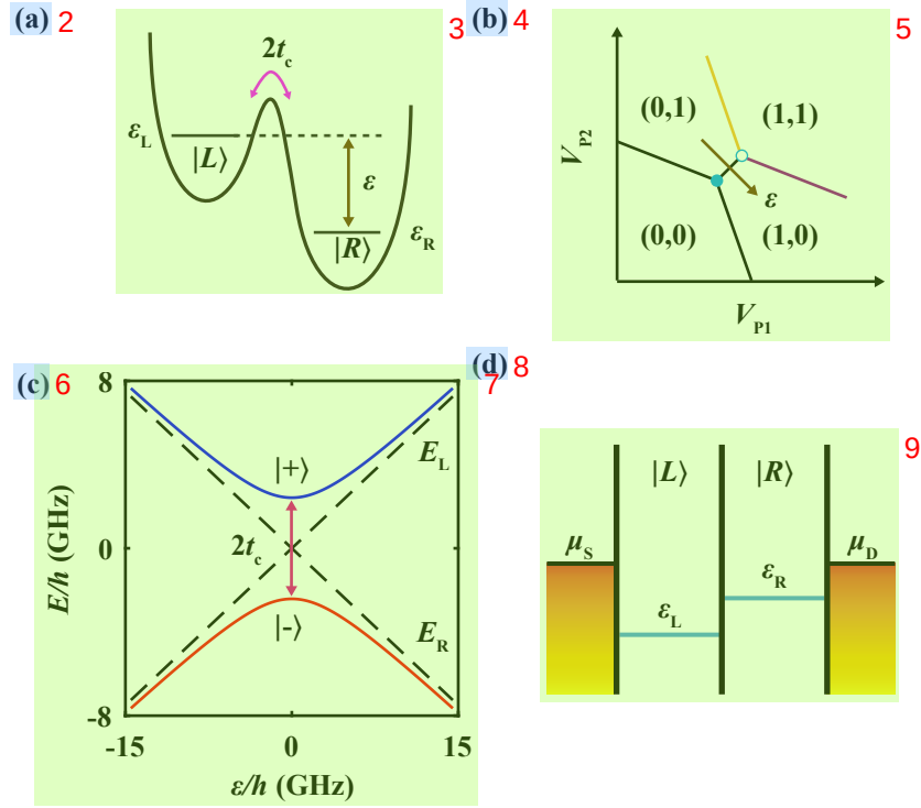
图 2.7 电荷量子比特示意图。(a) 双量子点势阱示意图，其中电荷态 |L\rangle 和 |R\rangle 之间存在速率为 2t_c 的隧穿耦合。电荷态的能量 E_L 和 E_R 分别对应于频率 \omega_L 和 \omega_R 。电荷态之间的失谐量由双点间的能量差 \varepsilon = \omega_L - \omega_R 决定。(b) 双量子点局部的电荷稳定性图，棕色箭头给定了失谐量 \varepsilon 的变化。(c) 电荷量子比特的能级图，本征态 |+\rangle 和 |-\rangle 存在免交叉 (d) 在进行量子比特编码情况下的双量子点电化学势示意图。
