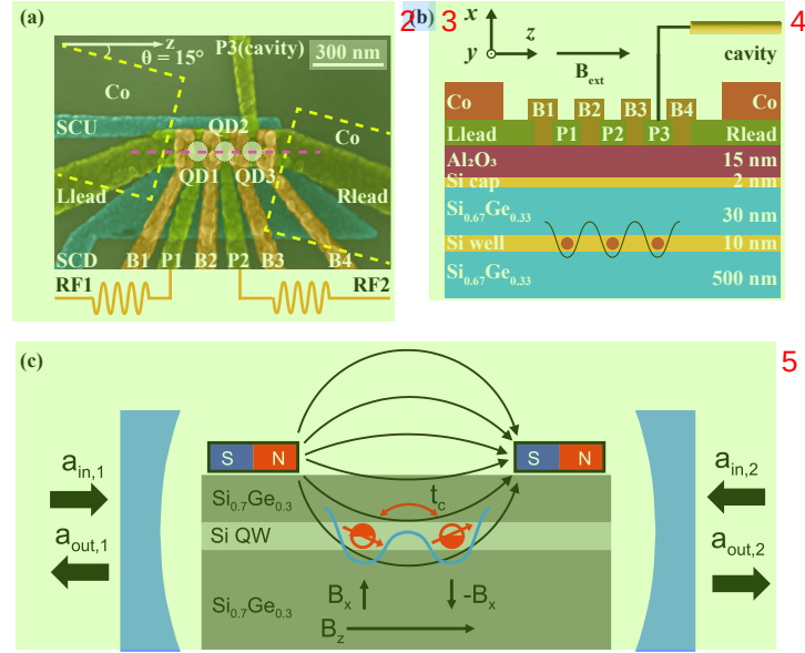
图 5.1 量子器件结构示意图。(a) 三层结构量子点器件 SEM 照片图, 黄色虚线的区域标识了微磁体的位置。(b) 图 (a) 中粉色曲线处的截面图, 外磁场沿着量子点方向。(c) 使用谐振腔耦合双点中翻转模式自旋量子比特的示意图, 这里电子自旋通过微磁体产生的梯度磁场与电荷态产生杂化。图片引自文献 [110] 。
