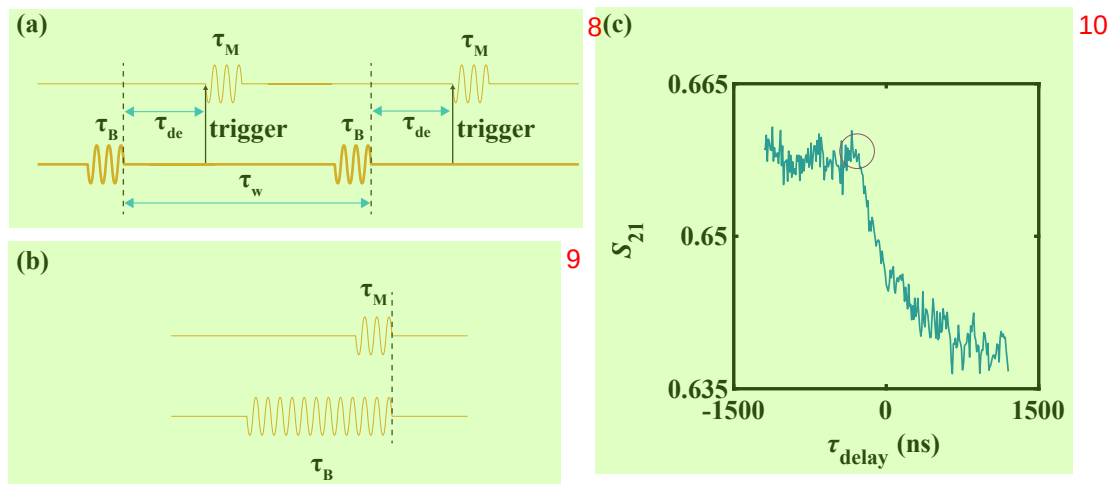
图 5.12 微波时序同步示意图。(a) 延时校准线路。下方线路表示驱动微波持续时间为 \tau_B ，上方线路则表示谐振腔的探测微波持续时间为 \tau_M 。黑色箭头标识出了驱动微波发出的触发信号位置，其与微波结束时间时刻的延时记作 \tau_{de} 。 \tau_w 则表示两次微波的时间间隔。(b) 测量微波结束位置与驱动微波结束位置对齐。(c) 谐振腔幅值信号关于触发延迟的关系，圆圈所示幅值下降位置对应 (b) 中所展示的情况。
