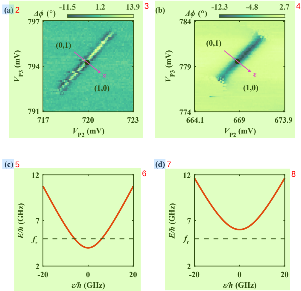
图4.7 使用谐振腔探测量子点间隧穿线 (1, 0) \leftrightarrow (0, 1) 。(a) 谐振腔相位响应关于电极电压 V_{P2} 和 V_{P3} 的关系，对应于隧穿耦合速率 2t_c < \omega_q 。(b) 隧穿耦合速率满足 2t_c > \omega_q 时，谐振腔的相位响应。(c) - (d) 量子比特和谐振腔的能量关系，虚线代表谐振腔能量，当 2t_c < \omega_q 时 (c) 存在两个交点，当 2t_c > \omega_q 时不存在交点。
