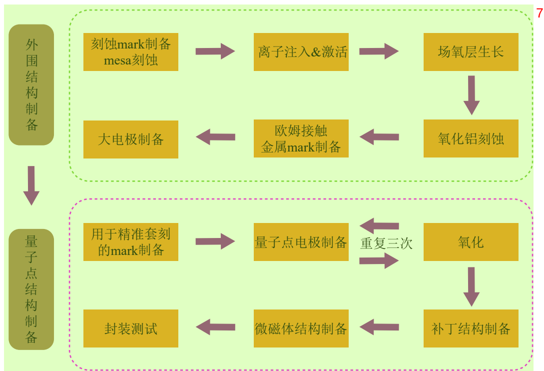
图 3.4 量子点的制备流程示意图，共分为外围结构制备和量子点结构制备两个主要模块。
