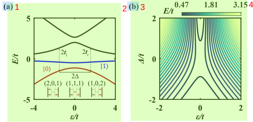
图 6.2 RX 量子比特的能级图。(a) 哈密顿量 H_{\text{eff}} 中各能级与 \varepsilon 的关系，此处我们保持了 \Delta 为固定值，且 t_l = t_r 。RX 量子比特定义在能量最低的两个能级上，在图中分别用红色和蓝色表示。(b) RX 量子比特能量与 \Delta 和 \varepsilon 的等高线关系，这里的能量是 (a) 两个能级的能量差。
