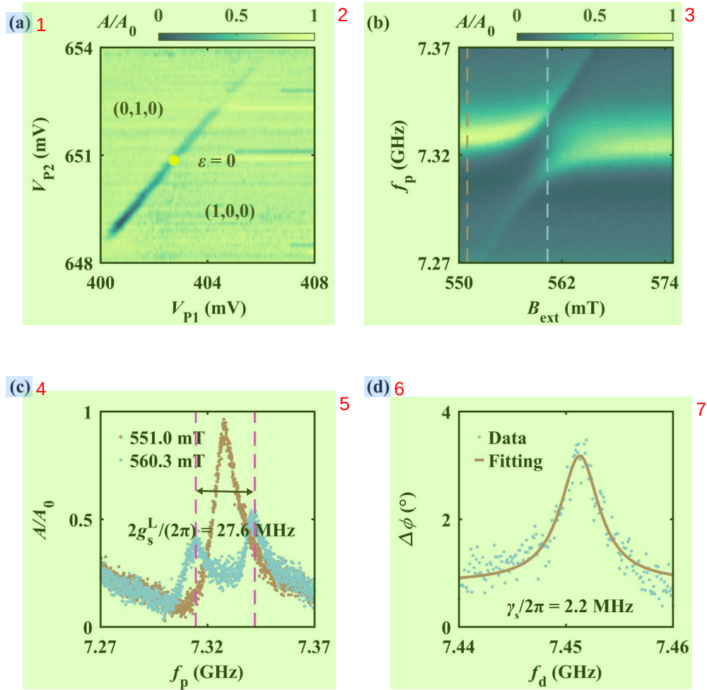
图 5.8 LDQD 中自旋量子比特与谐振腔的强耦合。(a) LDQD 单电子区域电荷稳定性图谱，黄色圆圈表示 \varepsilon = 0 的工作位点，在这里我们排空了 QD3 中的电子。(b) 谐振腔幅值信号关于外磁场和谐振腔探测频率的关系。(c) 对应于 (b) 中虚线所示的两个不同磁场，棕色 B_{\text{ext}} = 551.0 \text{ mT} 以及蓝色 B_{\text{ext}} = 560.3 \text{ mT} ，给出了谐振腔的响应谱线。(d) 通过双色调制谱测量得到的 LDQD 中翻转模式自旋比特展宽以及量子比特频率。
