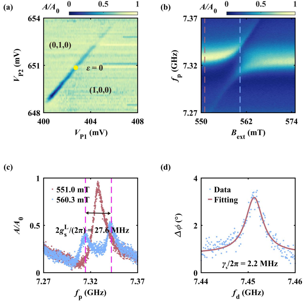
图 5.8 LDQD 中自旋量子比特与谐振腔的强耦合。(a) LDQD 单电子区域电荷稳定性图谱，黄色圆圈表示 \epsilon = 0 的工作位点，在这里我们排空了 QD3 中的电子。(b) 谐振腔幅值信号关于外磁场和谐振腔探测频率的关系。(c) 对应于 (b) 中虚线所示的两个不同磁场，棕色 B_{\text{ext}} = 551.0 mT 以及蓝色 B_{\text{ext}} = 560.3 mT，给出了谐振腔的响应谱线。(d) 通过双色调制谱测量得到的 LDQD 中翻转模式自旋比特展宽以及量子比特频率。
