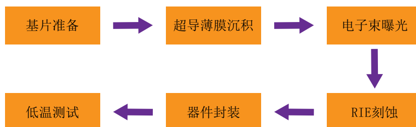
图 3.3 单独制备谐振腔的工艺流程图。
