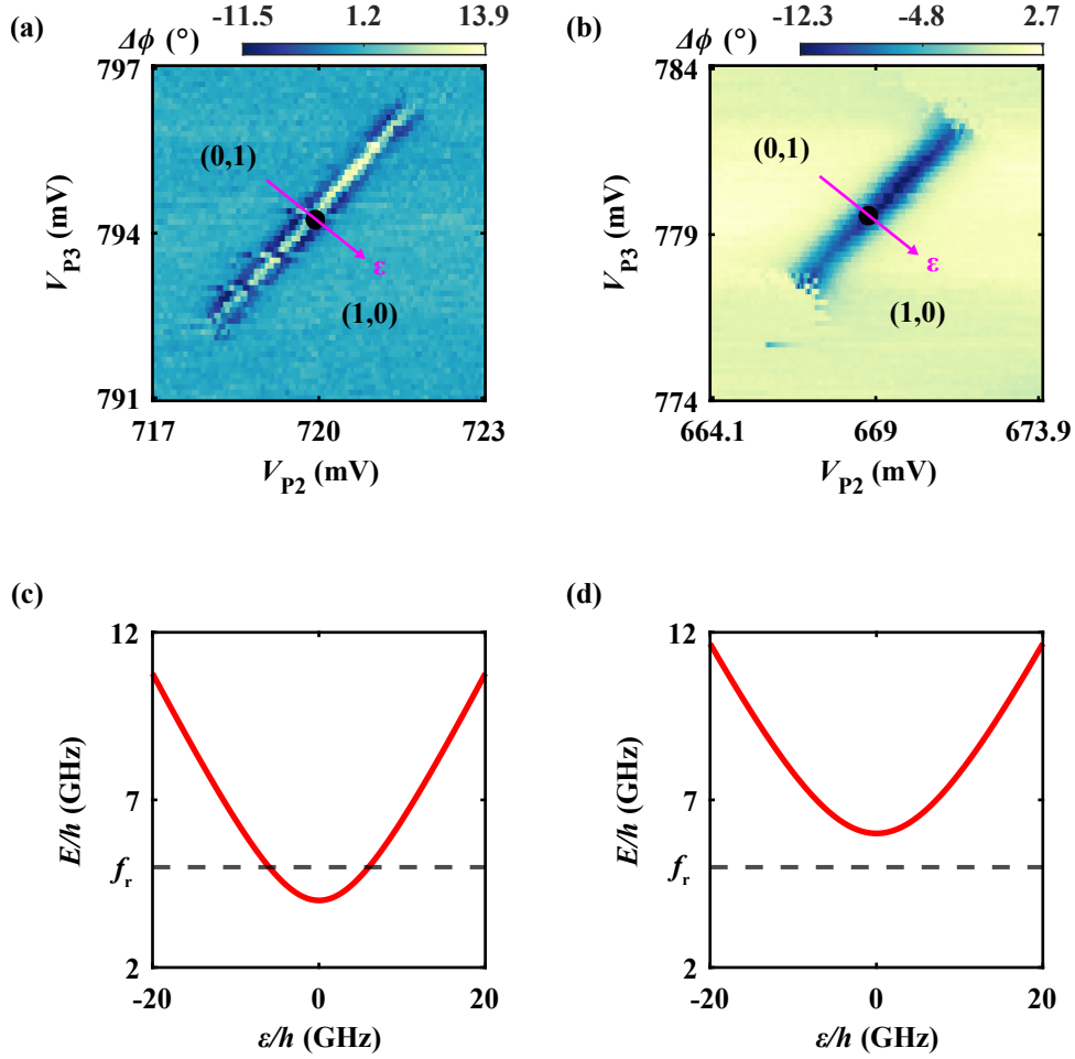
图 4.7 使用谐振腔探测量子点点隧穿线 (1, 0) \leftrightarrow (0, 1) 。(a) 谐振腔相位响应关于电极电压 V_{p2} 和 V_{p3} 的关系，对应于隧穿耦合速率 2t_c < \omega_q 。(b) 隧穿耦合速率满足 2t_c > \omega_q 时，谐振腔的相位响应。(c) - (d) 量子比特和谐振腔的能量关系，虚线代表谐振腔能量，当 2t_c < \omega_q 时 (c) 存在两个交点，当 2t_c > \omega_q 时不存在交点。
