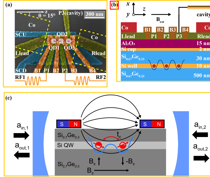
图 5.1 量子器件结构示意图。(a) 三层结构量子点器件 SEM 照片图, 黄色虚线的区域标识了微磁体的位置。(b) 图 (a) 中粉色曲线外的截面图, 外磁场沿着量子点方向。(c) 使用谐振腔耦合双点中翻转模式自旋量子比特的示意图, 这里电子自旋通过微磁体产生的梯度磁场与电荷态产生杂化。图片引自文献 [110] 。
