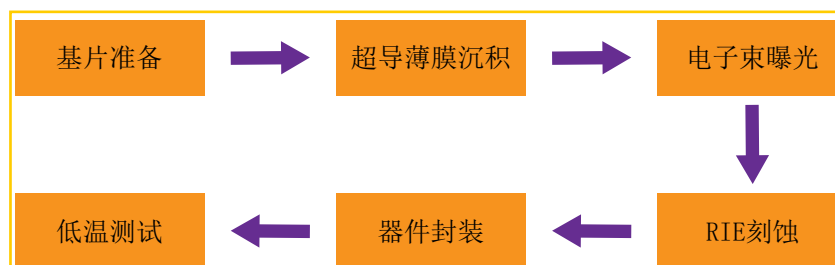
图 3.3 单独制备谐振腔的工艺流程图。
