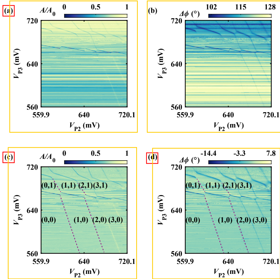
图 4.6 用谐振腔测量得到的 RDOD 稳定性图谱。(a) 谐振腔归一化幅值 A/A_0 与量子点电极电压 V_{P2} 和 V_{P3} 的关系。(b) 谐振腔相位响应 \Delta\phi 与量子点电极电压 V_{P2} 和 V_{P3} 的关系。(c) - (d) 为去除本底后的谐振腔响应信号，数字标识了该区域的电子数目。
