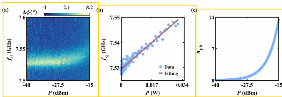
图 5.16 AC Stark shift 实验。(a) 谐振腔相位响应关于驱动功率和一体机输出功率 P 的关系，这里使用 dBm 作为单位。(b) 从 (a) 中提取的量子比特频率关于一体机输出功率 P 的关系，这里使用瓦特作为单位，呈现出明显的线性关系，棕色实线是对数据的拟合。(c) 绘制出的我们实验线路配置下一体机的输出功率和谐振腔光子的对应关系，对于 -30 dBm，我们预计谐振腔中存在 0.4 个光子。
