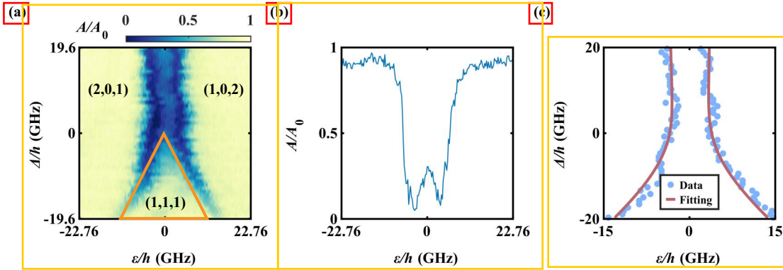
图 6.5 RX 量子比特的能谱。(a) 谐振腔幅值响应和两个失谐参数 \varepsilon 以及 \Delta 的关系，橙色三角形区域标记了 RX 量子比特的工作位置。(b) \Delta=0 时，谐振腔幅值响应关于失谐参数 \varepsilon 的关系。(c) 从 (a) 中提取的比特—谐振腔共振点，棕色实线是对数据的拟合。
