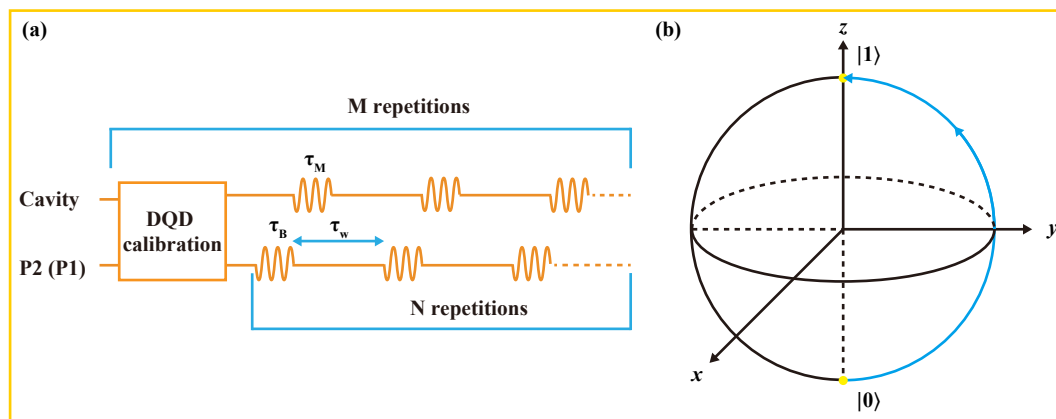
图 5.13 Rabi 操作示意图。(a) 用于 Rabi 操作的波形示意图, 在 Rabi 实验中, 对 RDQD (LDQD) 我们设定等待时间 \tau_w = 3(4) \mu s 。(b) Bloch 球, Rabi 操作过程中量子比特状态沿着图中蓝色曲线进行演化。
