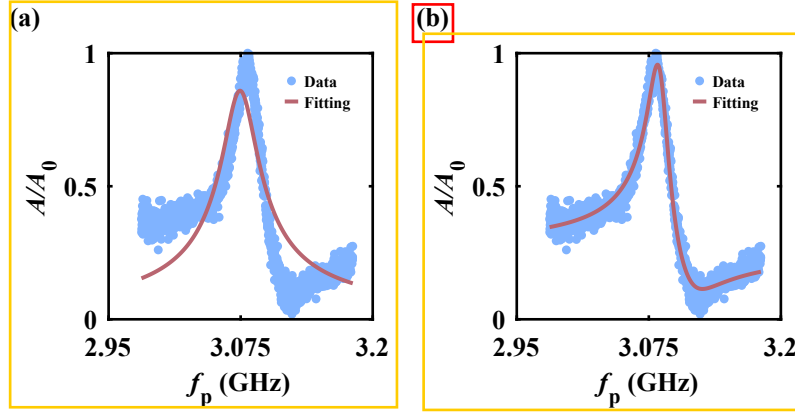
图 2.3 谐振腔拟合示意图。(a) 归一化幅值响应 A/A_0 随探测频率 f_p 的变化关系。蓝色圆点表示实验测量数据，棕色曲线为使用标准 Lorentzian 线型进行拟合的结果。在实验数据存在明显不对称性的情况下，拟合效果较差。(b) 棕色曲线表示基于带有 Fano 因子的公式拟合的结果。在数据不对称性较为显著的情况下，Fano 因子修正的公式能够更好地与实验数据吻合。
