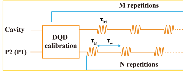
图 5.10 量子比特操作线路示意图，在进行操作之前，需要对量子点进行校准。这里可以通过施加不同的微波序列来实现对量子比特的不同操作。这里的等待时间 \tau_w ，测量时间 \tau_M ，以及施加微波 \tau_B 的时间根据不同的实验需求而确定。图中 M 和 N 表示当前循环的执行次数，也会根据实际情况选取合适的值。
