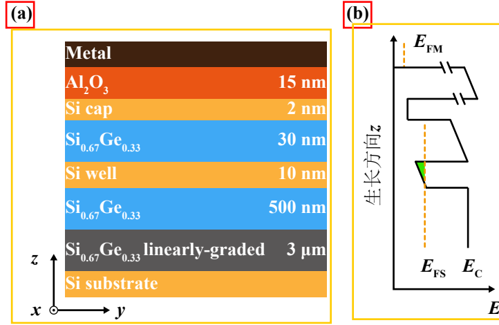
图 2.4 (a) 实验使用的 Si/SiGe 异质结构示意图。(b) 基片的能带结构，在三角形区域其导带底低于费米面。
