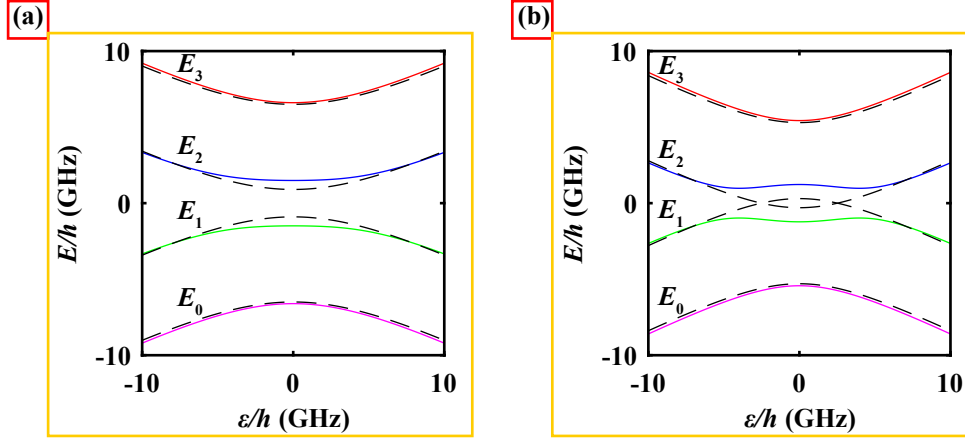
图 5.2 存在外磁场情况下的单个电子能级 E_i 示意图。这里取 B_z = 200 mT, \Delta B_x = 80 mT, 为了观察到梯度磁场的影响, 我们采用了显著高于实验的 \Delta B_x 值 (a) t_c = 3.7 GHz 时翻转模式量子比特能级结构, 满足 2t_c > E_c/h 。灰色虚线显示了 \Delta B_x = 0 的情况。(b) t_c = 2 GHz 时翻转模式量子比特能级结构, 满足 2t_c < E_c/h 。
