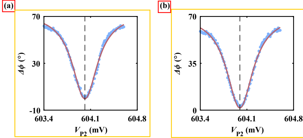
图 5.11 量子比特工作位点的校准。(a) 谐振腔相位响应随 V_{p2} 的变化关系。通过 Lorentz 曲线拟合，得到失谐零点对应的电压 V_{p2} = 604.01 \text{ mV} 。(b) 与 (a) 中相同条件下测量的数据，但测量时间为 (a) 测量结束后的 30 分钟。
