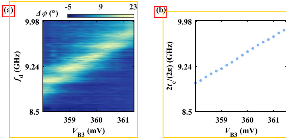
图 5.5 隧穿耦合速率和电极电压的关系。(a) 谐振腔相位响应信号与驱动频率和电极电压 V_{B3} 之间的关系，具有明显的峰值信号。(b) 隧穿耦合速率和 V_{B3} 之间的关系。每个 V_{B3} 对应的数据点都是通过对 (a) 中相应曲线进行洛伦兹拟合得到的，数据呈现出非常好的线性特征。
