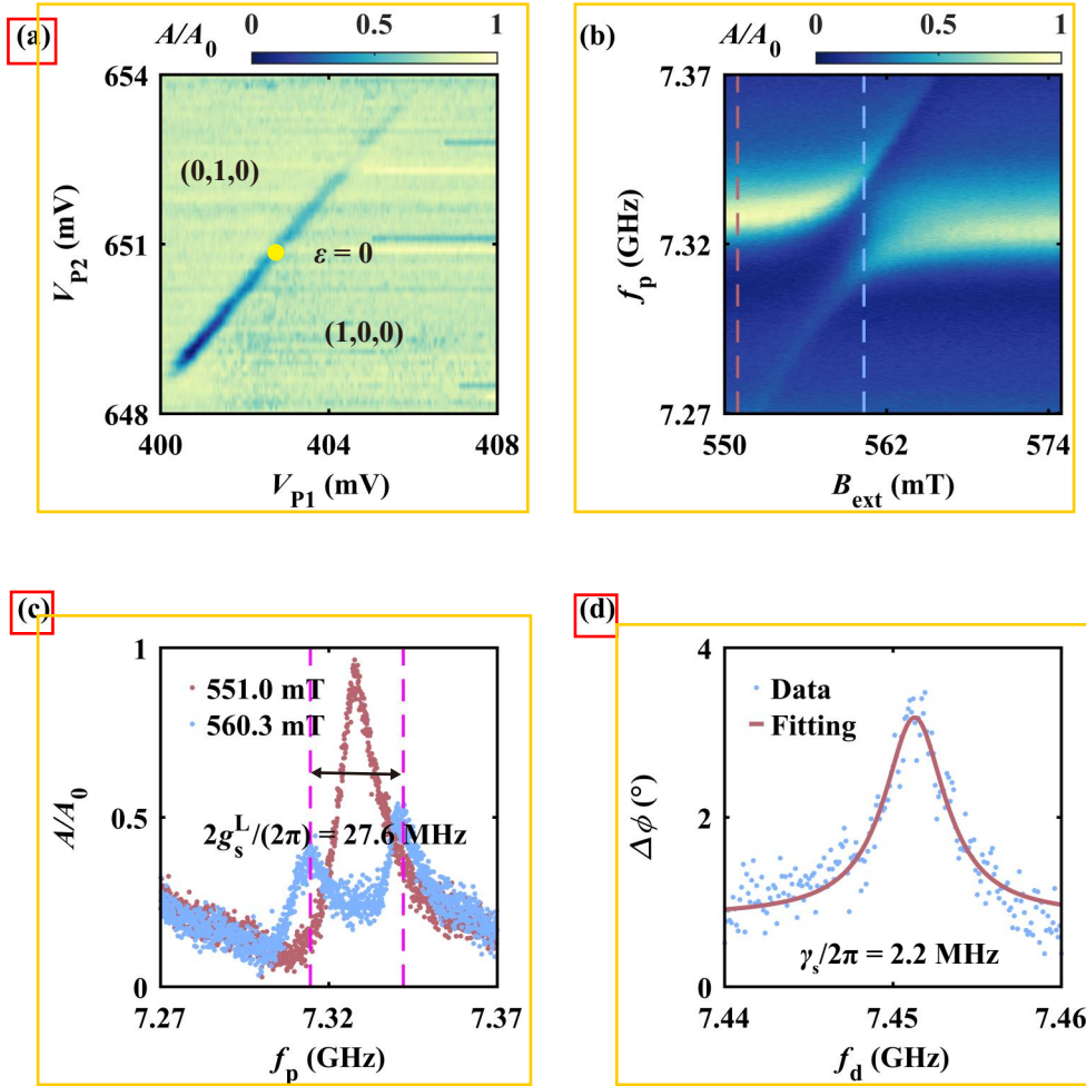
图 5.8 LDQD 中自旋量子比特与谐振腔的强耦合。(a) LDQD 单电子区域电荷稳定性图谱，黄色圆圈表示 \varepsilon=0 的工作位点，在这里我们排空了 OD3 中的电子。(b) 谐振腔幅值信号关于外磁场和谐振腔探测频率的关系。(c) 对应于 (b) 中虚线所示的两个不同磁场，棕色 B_{\text{ext}} = 551.0 \text{ mT} 以及蓝色 B_{\text{ext}} = 560.3 \text{ mT} ，给出了谐振腔的响应谱线。(d) 通过双色调制谱测量得到的 LDQD 中翻转模式自旋比特展宽以及量子比特频率。
