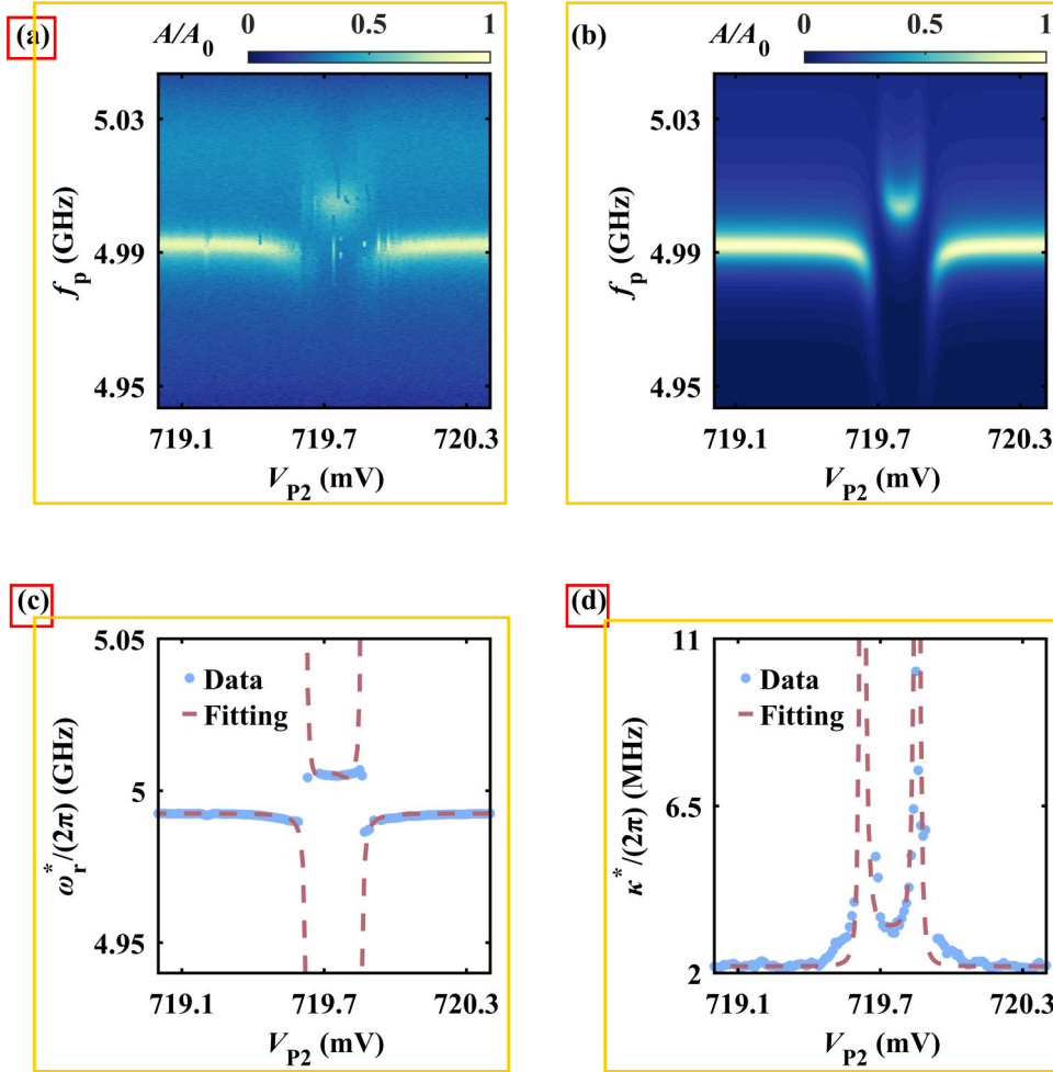
图 4.8 量子点耦合强度的测量。(a) 谐振腔透射信号 A/A_0 关于探测频率 f_p 和电极电压 V_{p2} 之间的关系, 能够观测到清晰的真空 Rabi 劈裂图谱。(b) 使用输入-输出理论对谐振腔透射信号进行模拟。(c) - (d) 对图 (b) 中每个电压对应的谐振腔信号进行拟合, 并提取谐振频率和展宽。再对这些数据进行拟合得到通过拟合得到耦合强度 g_0/(2\pi) = 175 \text{ MHz} 和量子点退相干 \gamma_c/(2\pi) = 99 \text{ MHz} 。
