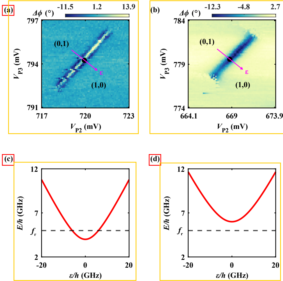
图 4.7 使用谐振腔探测量子点点间隧穿线 (1, 0) \leftrightarrow (0, 1) 。(a) 谐振腔相位响应关于电极电压 V_{p2} 和 V_{p3} 的关系，对应于隧穿耦合速率 2t_c < \omega_q 。(b) 隧穿耦合速率满足 2t_c > \omega_q 时，谐振腔的相位响应。(c) - (d) 量子比特和谐振腔的能量关系，虚线代表谐振腔能量，当 2t_c < \omega_q 时 (c) 存在两个交点，当 2t_c > \omega_q 时不存在交点。
