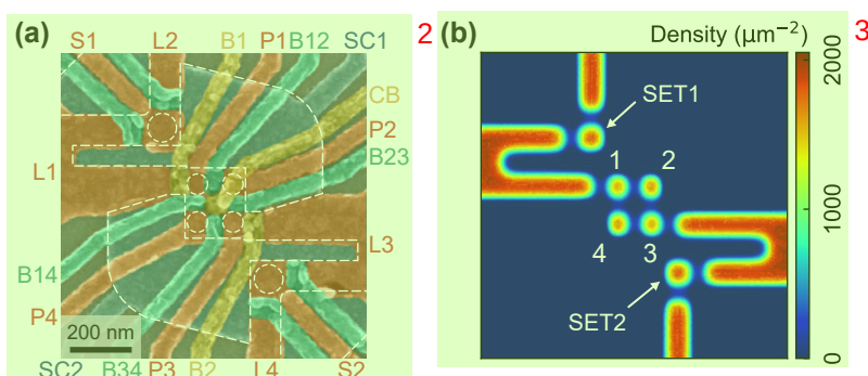
图4.1 基于Si/SiGe异质结的 2 \times 2 量子点阵列。(a)硅基二维量子点阵列的伪彩色扫描电子显微镜图像。该阵列包含位于中心的四个量子点和位于左上及右下的两个用作电荷探测器的大量子点。四个量子点分别位于电极P1-P4（橙色）下方，其中QD1和QD3直接与源漏电子库耦合，隧穿速率分别由势垒电极B1和B4调控。此外，势垒电极 B_{ij} （绿色）控制最近邻量子点之间的隧穿耦合，中心势垒（CB）电极（黄色）则控制次近邻量子点之间的隧穿耦合。(b)基于COMSOL模拟的电子密度分布图，其中标记出了四个量子点以及SET的位置，分别对应(a)中的白色圆圈。
