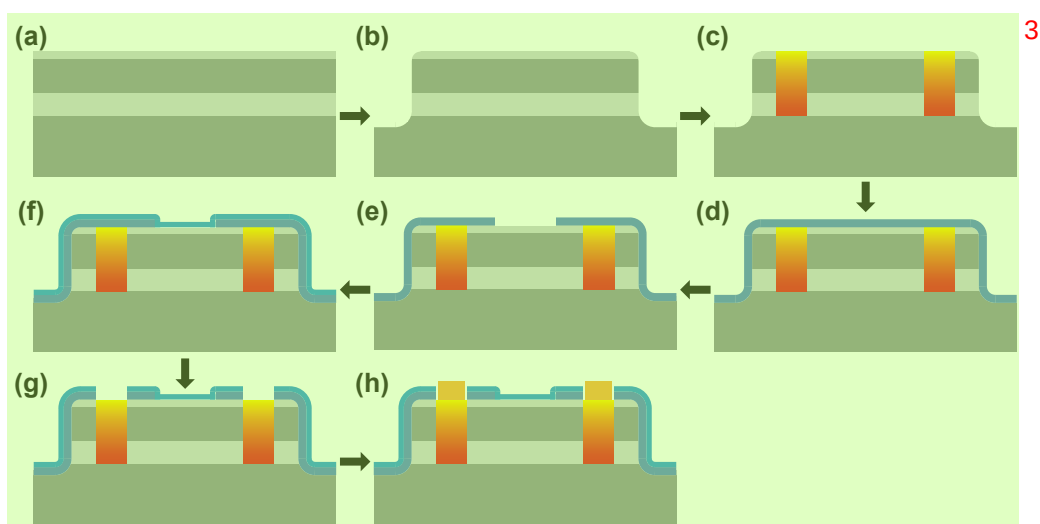
图 2.6 基片前处理过程。(a) Si/SiGe 异质结衬底。(b) Mesa 刻蚀。(c) 离子注入及激活。(d) 场氧层生长及 (e) 刻蚀。(f) 栅氧层生长及 (g) 刻蚀。(h) 氧化硅刻蚀及欧姆接触。
