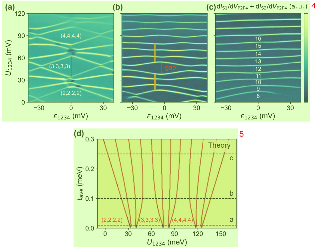
图 5.4 量子点阵列的电子填充谱随点间隧穿耦合的变化情况，分别对应 (a) 弱耦合、(b) 中等耦合，以及 (c) 强耦合。中等耦合下 (b) 呈现出集体库仑阻塞现象，其中橙色线段对应上、下 Hubbard 能带形成的位置，红色箭头线段对应莫特能隙。图中的数字代表电子数目。(d) 基于二维 Fermi-Hubbard 模型模拟的电子填充谱随最近邻点间隧穿耦合强度平均值的变化关系，其中 a、b 和 c 处的耦合强度对应实验中的弱耦合、中等耦合，以及强耦合。模拟参数如下：平均充电能 3 meV，最近邻点间库仑相互作用 0.4 meV，次近点间库仑相互作用为零。 6
