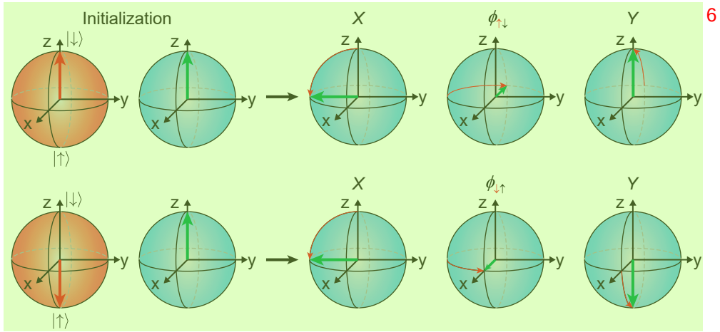
图 3.13 CZ 门实现过程的直观展示。控制比特（红色）分别被初始化为自旋下态和自旋上态时，目标比特（绿色）在布洛赫球上的演化过程。两种情况下的演化速度均为 J/2 ，但演化方向完全相反。通过控制 J 的演化时间使相位积累满足 \phi_{\uparrow\downarrow\uparrow} = \pi/2 时可实现 CZ 门。图片修改自 [27]。
