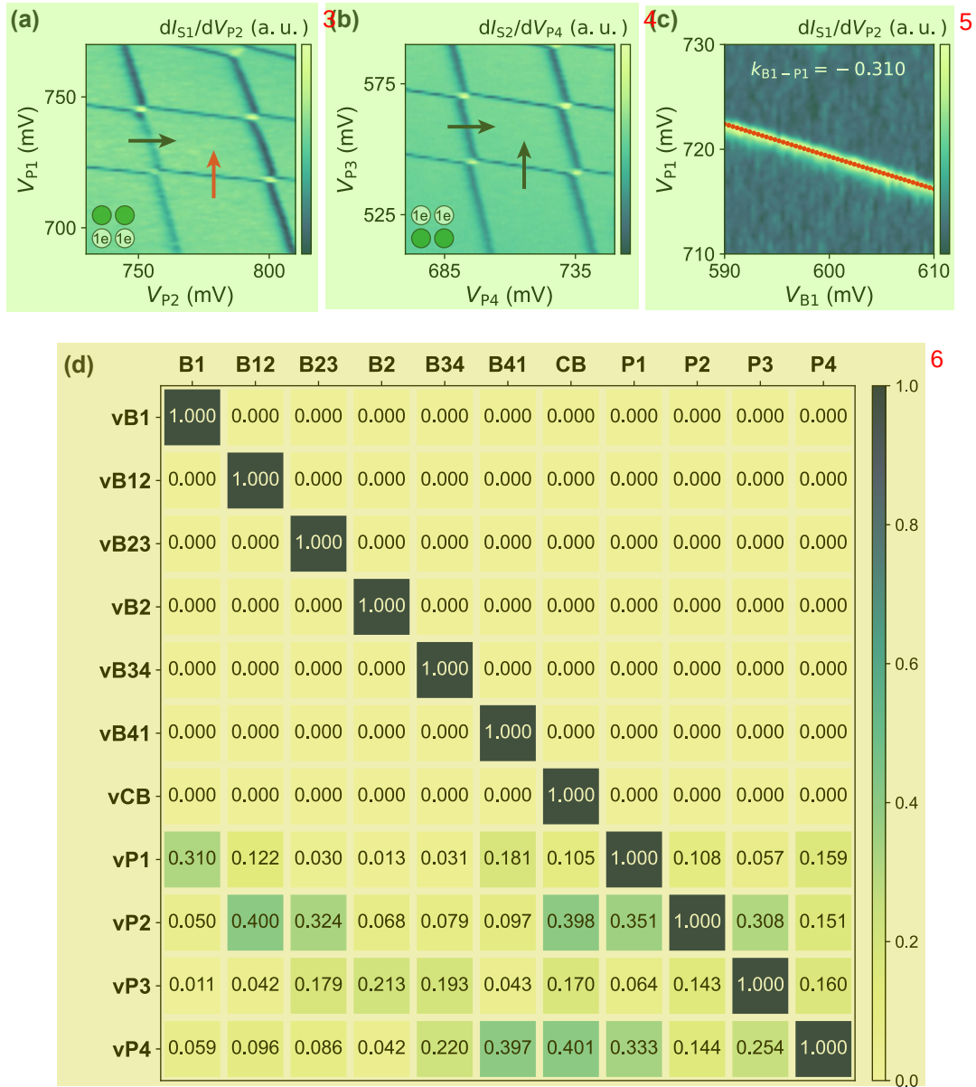
图 4.6 虚拟栅极的建立。(a) 和 (b) 分别为 QD1-QD2 和 QD3-QD4 的电荷稳定图。左下角绿色圆圈代表当前正在测量的量子点，白色圆圈代表闲置的量子点，其中 1e 表示点内有一个电子。在测量 QD1-QD2 时，QD3 和 QD4 均处于深阻塞区避免产生干扰；对于 QD3-QD4 亦然。(c) QD1 的电荷隧穿线随栅极 B1 电压的变化情况，由于电容串扰，隧穿线变得倾斜，其斜率可以通过拟合每个 B1 电压下的峰值位置（红色数据点）来得到。(d) 2 \times 2 量子点阵列的串扰矩阵。最后四行矩阵元分别为四个量子点电化学势（P1-P4）的电容串扰系数。 7
