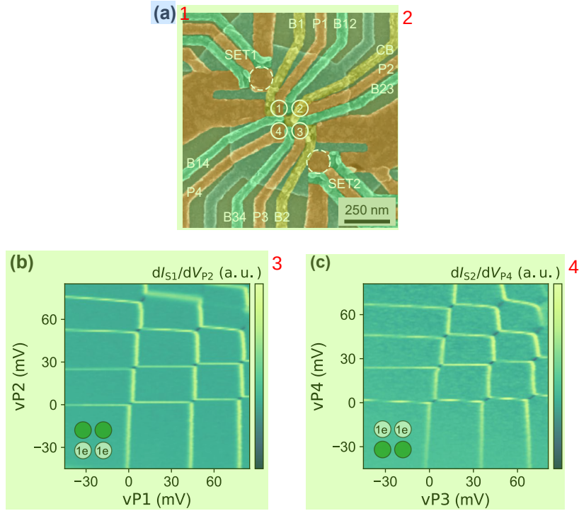
图 5.2 2 \times 2 量子点阵列及其电荷稳定图。(a) 器件的 SEM 图，包含四个量子点和两个电 5 荷探测器。(b) 和 (c) 分别为 QD1-QD2 和 QD3-QD4 的电荷稳定图。量子点阵列可以被调 6 节至单电子占据状态。
