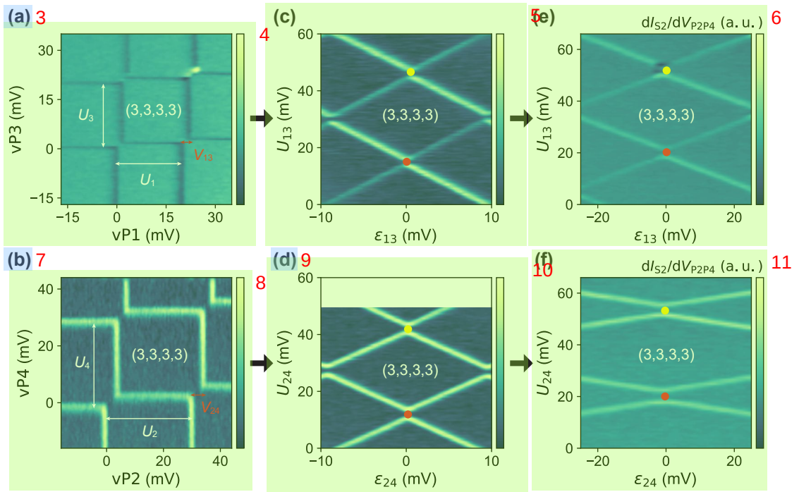
图 5.3 均匀同步填充的实现过程。(a) 和 (b) 分别为 QD1-QD3 和 QD2-QD4 在三个电子区的电荷稳定图。根据电荷隧穿线的间距可以提取四个点的充电能大小。(c) 和 (d) 分别为 QD1-QD3 和 QD2-QD4 在失谐-能量轴下的电荷稳定图。两个相图中反交叉的间距相同。(e) 和 (f) 为添加失谐轴扫描系数后测得的电荷稳定图，分别对应 QD1-QD3 和 QD2-QD4。红和黄色点代表讲四个量子点电势对齐的参考点。
