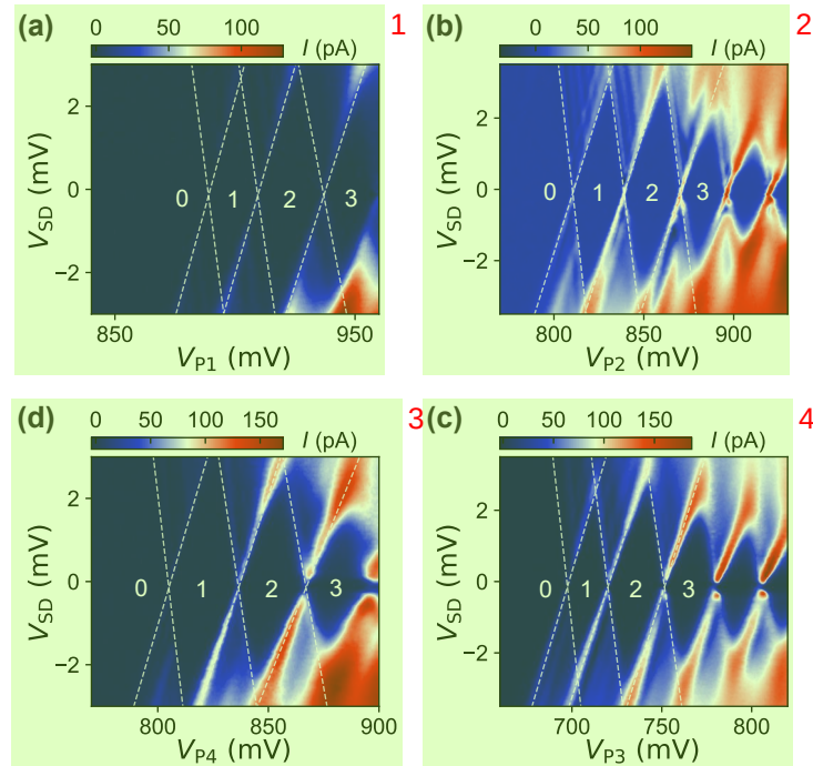
图 4.2 单量子点的库仑菱形图，分别对应 (a) QD1, (b) QD2, (c) QD3 和 (d) QD4, 每个点中电子都可以被排空，其中数字代表电子数目。
