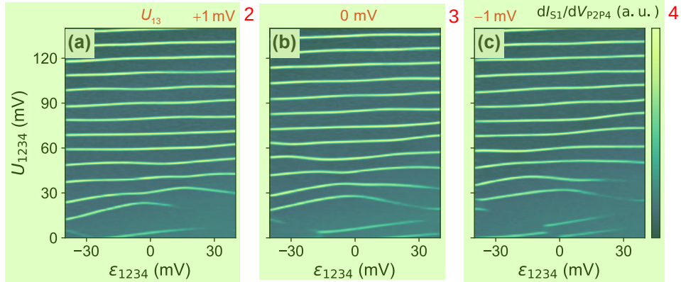
图 5.5 强耦合下电子填充谱随 U_{13} 的变化情况。(a) 和 (c) 相对 (b) 分别增加 1 mV 和减少 1 mV。
