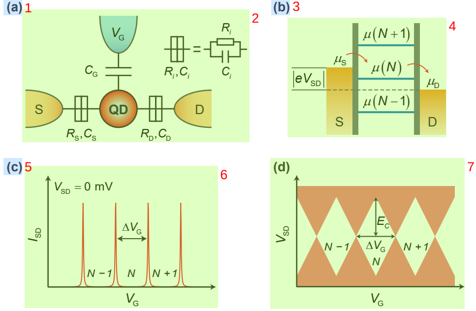
图 1.3 单量子点模型及其基本性质。(a) 单量子点的等效电路模型示意图，其中隧穿势垒等效为电阻 R_{S(D)} 和电容 C_{S(D)} 的并联。图片修改自文献 [80] 。(b) 单量子点能级示意图，只有 \mu(N) 落入源漏偏压窗口时，电子才能够连续隧穿产生电流。(c) 零偏压下的库仑振荡示意图，相邻库仑峰的间距对应量子点充电能大小（需要用杠杆臂系数进行换算）。(d) 库仑菱形示意图，从中可以提取量子点的充电能及杠杆臂系数。
