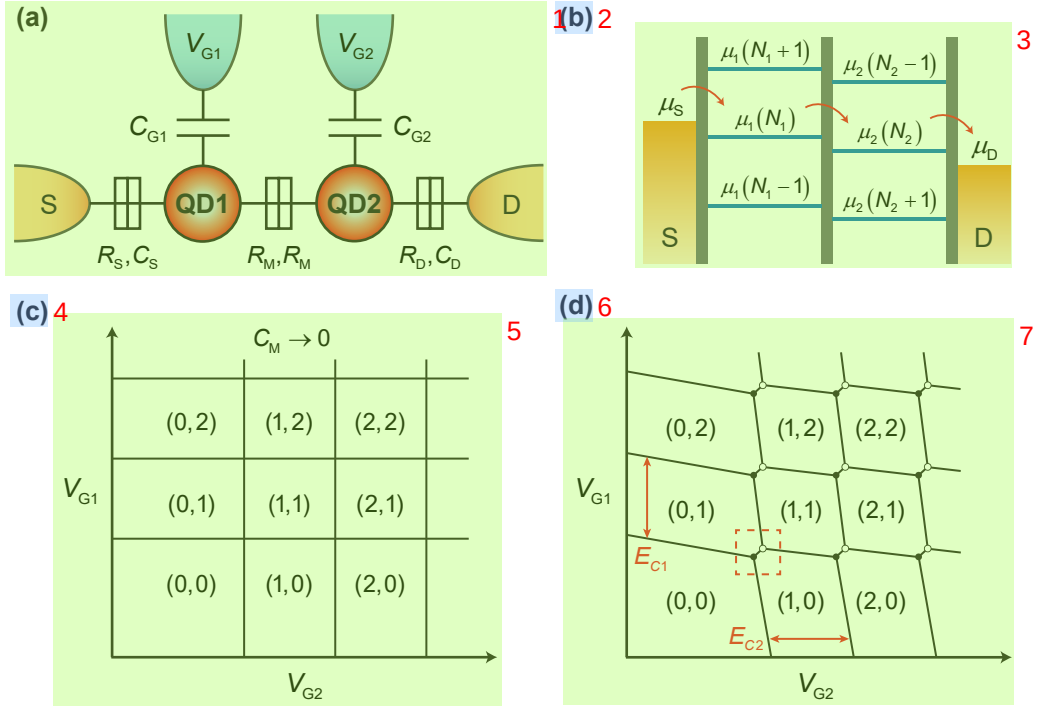
图 1.4 双量子点模型及其基本性质。(a) 双量子点的等效电路模型示意图，其中 C_M 为两个量子点间的耦合电容。(b) 双量子点的能级结构示意图，此时电子可以依次从源极跳入 QD1 和 QD2，最后进入漏极。(c) 耦合能接近零时的电荷稳定图。(d) 弱耦合状态下的电荷稳定图。根据电荷隧穿线的间距可提取充电能大小。注意，以上为常相互作用模型描述下的电荷稳定图。图片修改自文献 [80] 。
