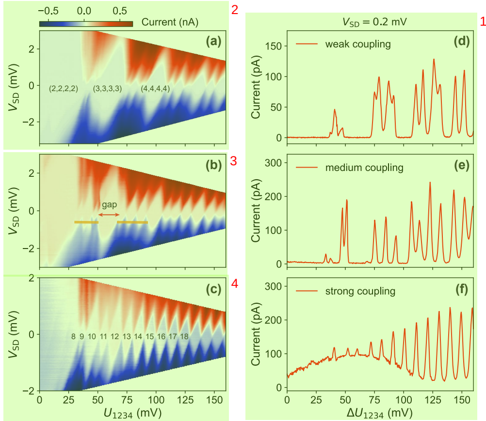
图 5.6 量子点阵列的电流输运测量结果。(a) - (c) 分别为弱耦合, 中等耦合和强耦合下的库仑菱形图, 以及相应 (d) - (f) 源漏偏压 V_{SD} = 0.2 \text{ mV} 时的电流曲线。
