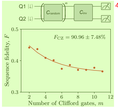
图 3.14 两比特门随机基准测试。Q1 和 Q2 的联合测量概率随两比特 RB 序列长度 m 的变化关系。图片上方为两比特标准 RB 的波形序列示意图。每个数据点为 25 个随机序列测量结果的平均，其中每个序列重复测量了 20 次，每次包含 200 组 single-shot 数据。 5
