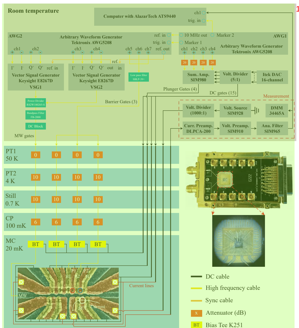
图 2.8 两比特操控的测量线路图。
