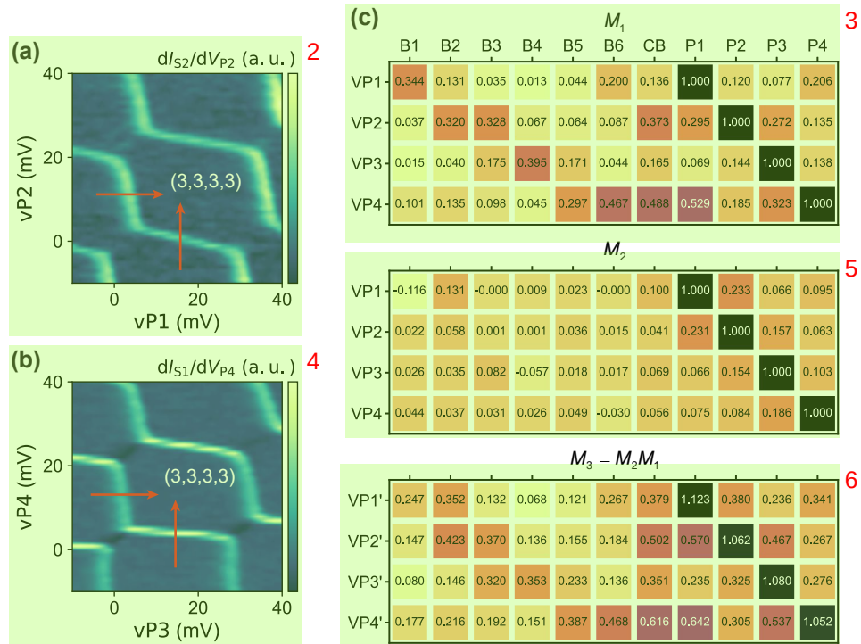
图 5.7 虚拟电极的更新。(a) QD1-QD2 和 (b) QD3-QD4 的电荷稳定图，用于提取新的串扰矩阵。红色带箭头的线代表扫描的具体位置。(c) 电容串扰矩阵，其中 M_1 、 M_2 和 M_3 = M_2 M_1 分别对应原始矩阵、新测量得到的矩阵和更新后的矩阵。 7
