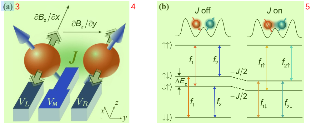
图 1.10 两比特门的实现原理。(a) 基于交换相互作用耦合的双自旋系统，其中磁场梯度由微磁体提供。图片修改自文献 [118] 。(b) 交换相互作用关闭和打开时的能级图。交换相互作用的打开会使反自旋态的能级向下移动 J/2 ，使得一个比特的频率依赖于另外一个比特的状态。图片修改自文献 [107,119] 。
