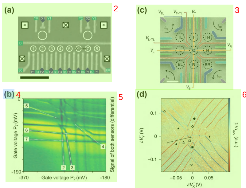
图 1.6 基于 GaAs 的一维和二维量子点阵列。(a) 一维八量子点阵列及其 (b) 电荷稳定图, 7 其中电荷隧穿线难以有效区分。图片引自 [62] 。(c) 3 \times 3 量子点阵列及其 (d) 电荷稳定图, 其调控过程非常复杂。图片引自 [66] 。
