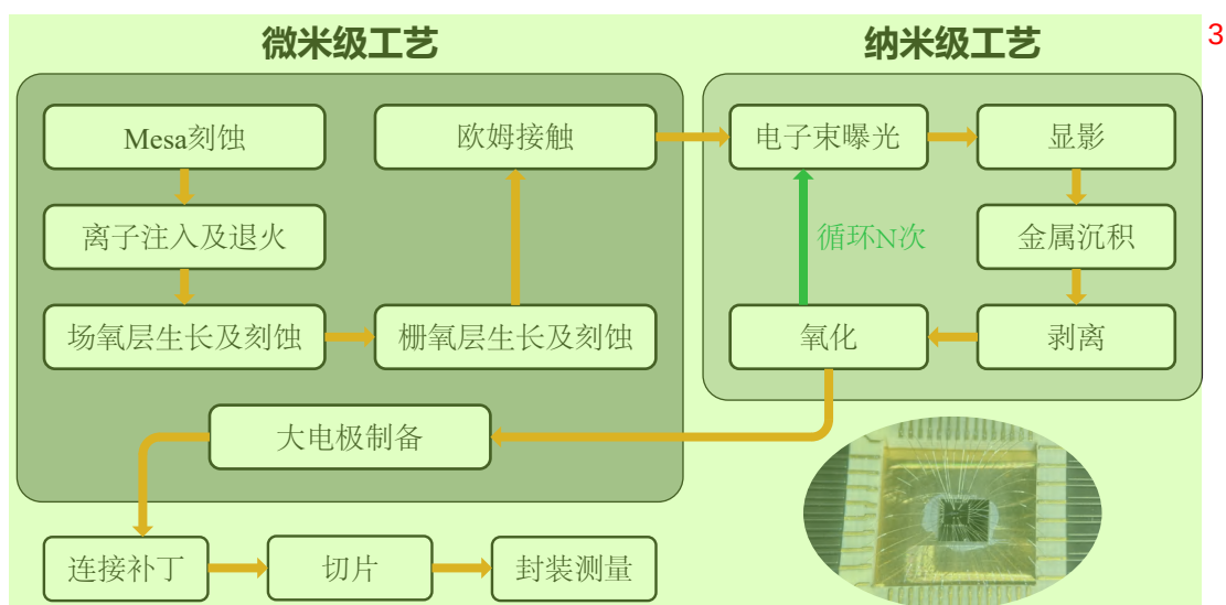
图 2.5 Si/SiGe 量子点的制备流程，包括微米级、纳米级制造工艺和后续封装过程。右下角 4 为键合封装后的芯片照片。
