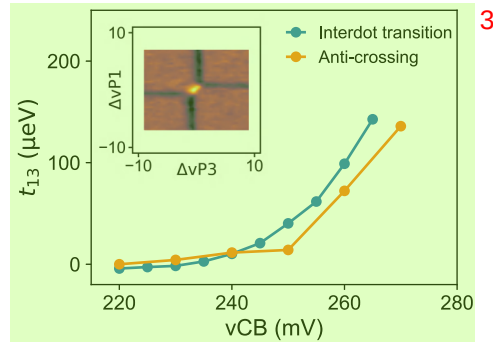
图 4.14 点间隧穿线与反交叉拟合的对比。为了便于比较，点间隧穿线拟合的数据向下平移了 25\text{ }\mu\text{eV} 。插图为 QD1-QD3 的电荷稳定图。 3
