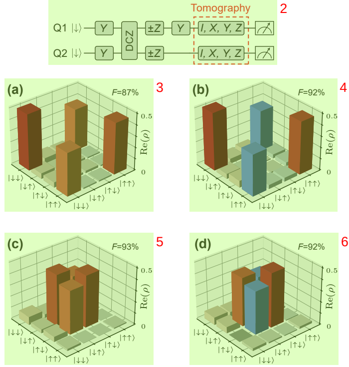
图 3.16 基于 DCZ 门的 Bell 态制备。(a) |\Phi^+\rangle = (|\downarrow\downarrow\rangle + |\uparrow\uparrow\rangle)/\sqrt{2} , (b) |\Phi^-\rangle = (|\downarrow\downarrow\rangle - |\uparrow\uparrow\rangle)/\sqrt{2} , (c) |\Psi^+\rangle = (|\downarrow\uparrow\rangle + |\uparrow\downarrow\rangle)/\sqrt{2} , (d) |\Psi^-\rangle = (|\downarrow\uparrow\rangle - |\uparrow\downarrow\rangle)/\sqrt{2} 的重构密度矩阵（实部）。读出误差移除前（后）的保真度分别为 84%（87%），85%（92%），86%（93%）和 86%（92%）。图片上方为制备 Bell 态及态层析的波形序列示意图。 7
