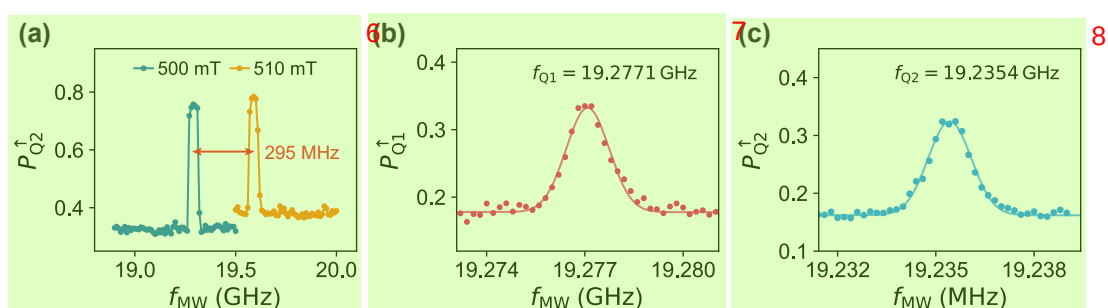
图 3.3 寻找电子自旋共振峰。(a) 采用 Chirp 波形分别在外磁场 500 mT 和 510 mT 下测得的电子自旋共振峰 (Q2), 其中 Chirp 波形宽度为 50 MHz。(b) Q1 和 (c) Q2 在低微波功率下的自旋共振峰。通过高斯函数拟合 (实线), 可以确定 Q1 和 Q2 的比特频率分别为 19.2771 GHz 和 19.2354 GHz。
