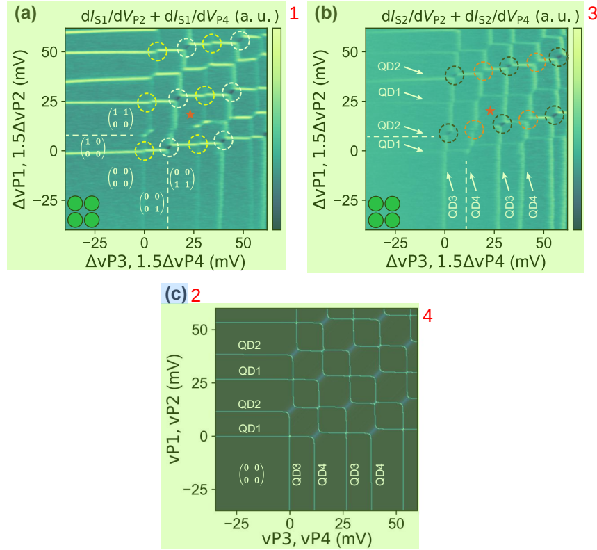
图 4.8 基于同步扫描测得的电荷稳定图，分别对应 (a) SET1 和 (b) SET2 的信号。由于 QD1 和 QD3 的电化学势相对于 QD2 和 QD4 略低，因此呈现出交错排列的电荷隧穿线。虚线圆圈标记了不同双量子点的反交叉点：白、黑、黄和橙色圆圈分别对应 QD1-QD4，QD2-QD3，QD1-QD3 和 QD2-QD4。受到 SET 与量子点之间相位位置和距离的影响，QD1-QD4 的点间隧穿线在 (a) 中更明显，而 QD2-QD3 则在 (b) 中更突出。红色五角星位置对应 (1, 1, 1, 1) 电荷区。(c) 基于 Hubbard 模型模拟得到的电荷稳定图，与实验结果相符。模拟参数如下：平均充电能为 3 meV，最近邻点间隧穿耦合和库仑相互作用分别为 0.1 meV 和 0.2 meV，次近邻点间隧穿耦合和库仑相互作用为 0 meV 和 0.05 meV，lever arm 为 0.12 eV/V。
