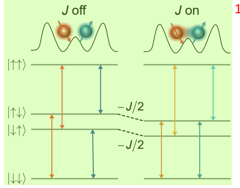
图 3.8 双电子自旋系统的能级示意图。当塞曼能级差远大于交换相互作用时，系统本征态近似为自旋直积态，打开 J 会导致自旋反平行能级向下移动 J/2 。图片修改自文献 [107,119] 。
