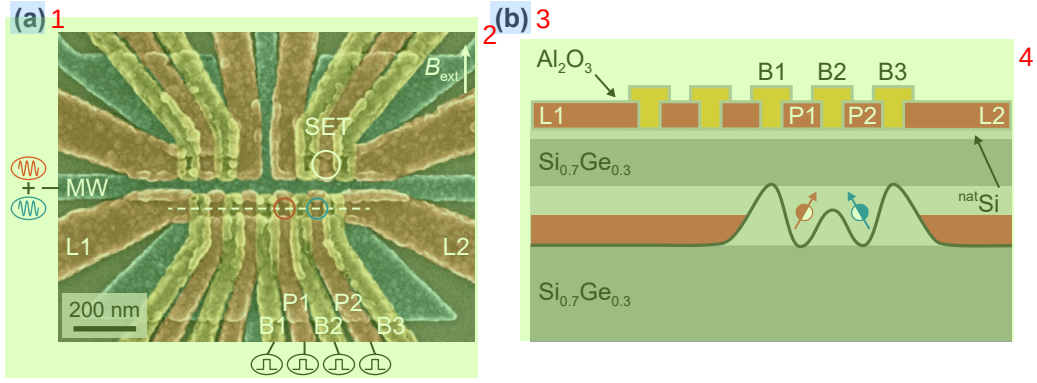
图 3.1 一维四量子点器件结构。(a) 量子点器件的伪彩色 SEM 图。两个量子点分别位于栅极 P1 和 P2 下方，其间隧穿耦合由势垒栅极 B2 控制。量子点对面为电荷探测器 (SET)，用于探测自旋比特的状态。微波电场施加到栅极 MW 上，用于驱动自旋比特翻转；低频与高频电压脉冲分别施加到能级栅 (P1 和 P2) 和势垒栅 (B2 和 B3) 上，用于调控电势及交换相互作用。(b) 双量子点的横截面示意图，对应 (a) 中的虚线方向。每个量子点中各有一个电子，其自旋用于编码形成量子比特。最左侧两个量子点的栅极电压与 L1 相同，用作源极电子库。
