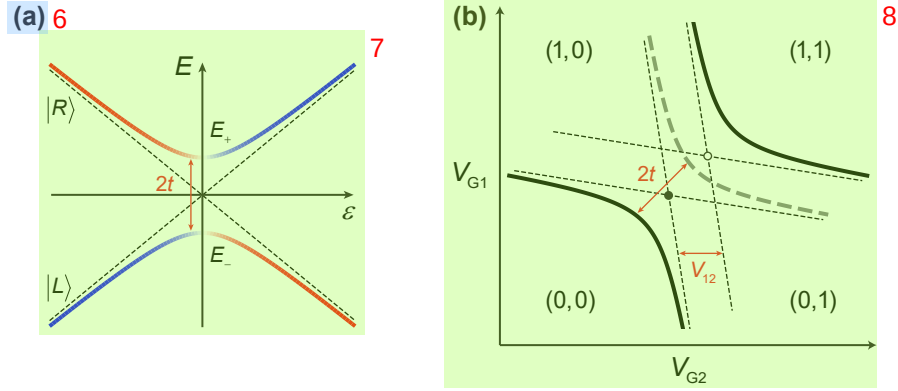
图 1.5 电荷二能级系统。(a) 能级示意图, 其中失谐零处的能级劈裂为 2t 。(b) 电荷隧穿线的反交叉示意图, 其中反交叉的弯曲程度取决于 2t 大小。虚线代表右上角反交叉沿对角线向下平移 V_{12} 的结果。图片修改自文献 [80] 。
