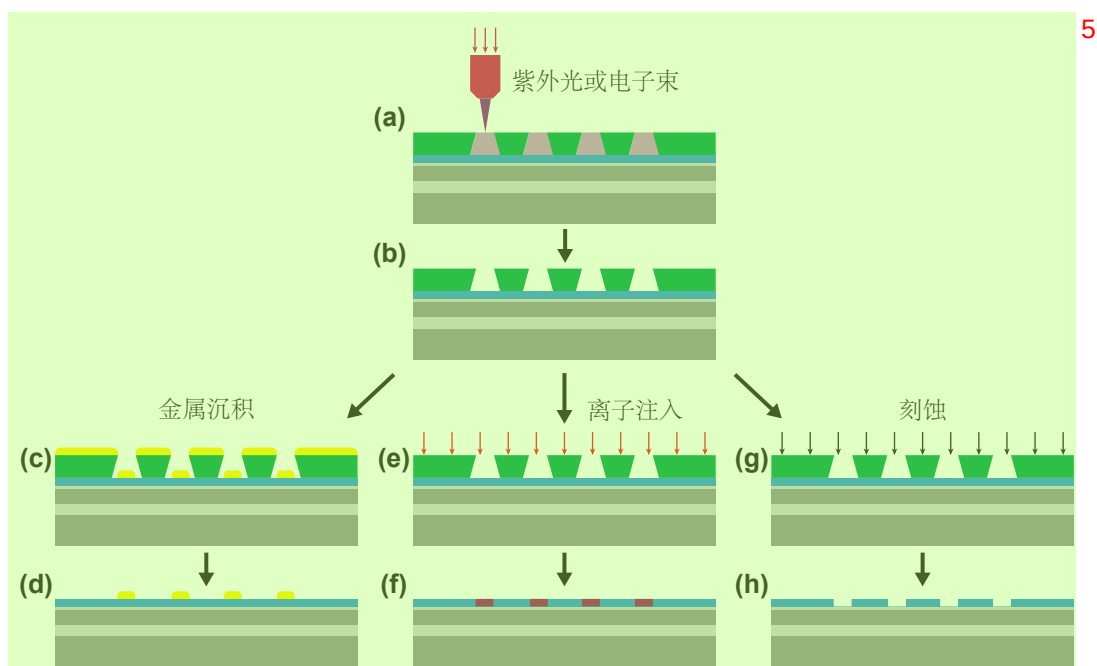
图 2.3 基于无掩模光刻技术的图形转移工艺。(a) 图形发生，采用紫外或电子束光刻。(b) 显影工艺。(c) 金属沉积及 (d) lift-off 工艺。(e) 离子注入及 (f) 去胶。(g) 刻蚀工艺（包括干法和湿法）及 (h) 去胶。 5
