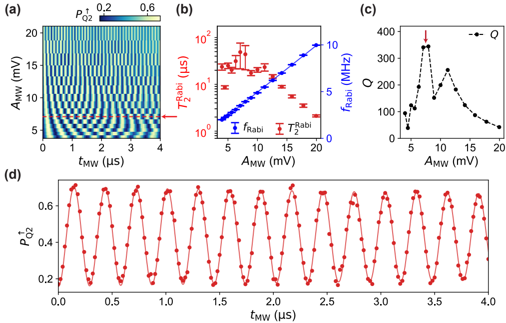
图 3.6 Rabi 振荡的品质因子。(a) Rabi 振荡与微波幅值和脉冲时间的变化关系。(b) 不同 A_{MW} 下拟合得到的 T_2^{\text{Rabi}} 和 f_{\text{Rabi}} , 其中 f_{\text{Rabi}} 随 A_{MW} 呈线性增加(实线为线性拟合结果)。(c) 不同 A_{MW} 下计算得到的 Q 值。(d) A_{MW} \approx 7 \text{ mV} 时的 Rabi 振荡, 对应 (a) 中的红色虚线位置, 其中 f_{\text{Rabi}} = 3.5 \text{ MHz} , T_2^{\text{Rabi}} = 27.6 \mu\text{s} 。每个数据点为 2500 次 single-shot 测量的平均。
