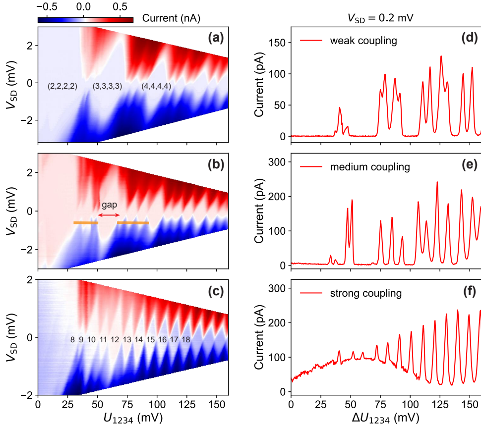
图 5.6 量子点阵列的电流输运测量结果。(a) - (c) 分别为弱耦合，中等耦合和强耦合下的库仑菱形图，以及相应 (d) - (f) 源漏偏压 V_{SD} = 0.2 mV 时的电流曲线。
