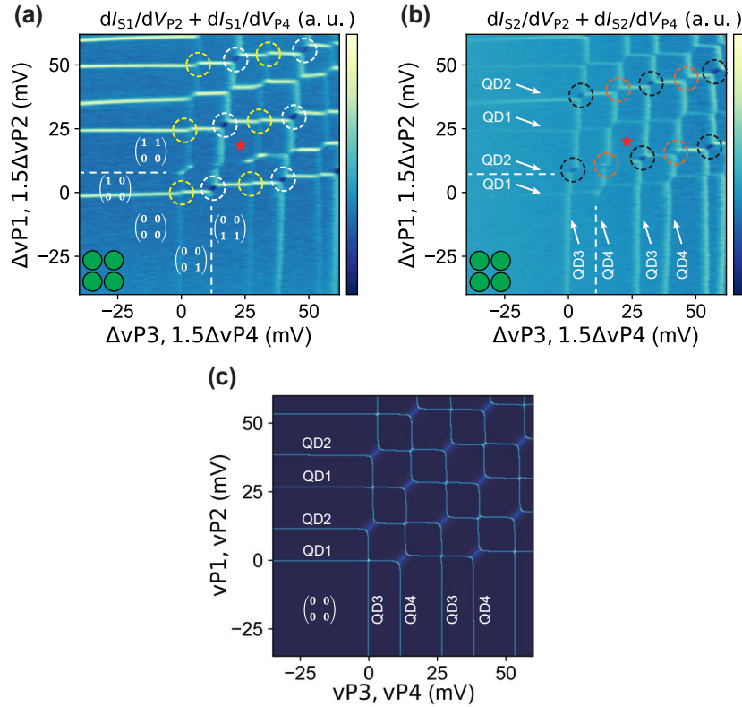
图 4.8 基于同步扫描测得的电荷稳定图，分别对应 (a) SET1 和 (b) SET2 的信号。由于 QD1 和 QD3 的电化学势相对于 QD2 和 QD4 略低，因此呈现出交错排列的电荷隧穿线。虚线圆圈标记了不同双量子点的反交叉点：白、黑、黄和橙色圆圈分别对应 QD1-QD4, QD2-QD3, QD1-QD3 和 QD2-QD4。受到 SET 与量子点之间相位位置和距离的影响，QD1-QD4 的点间隧穿线在 (a) 中更明显，而 QD2-QD3 则在 (b) 中更突出。红色五角星位置对应 (1, 1, 1, 1) 电荷区。(c) 基于 Hubbard 模型模拟得到的电荷稳定图，与实验结果相符。模拟参数如下：平均充电能为 3 meV，最近邻点间隧穿耦合和库仑相互作用分别为 0.1 meV 和 0.2 meV，次近邻点间隧穿耦合和库仑相互作用为 0 meV 和 0.05 meV，lever arm 为 0.12 eV/V。
