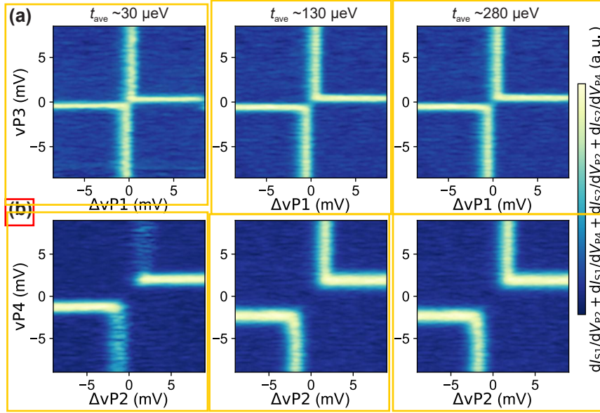
图 4.15 (a) QD1-QD3 和 (b) QD2-QD4 的电荷稳定图随最近邻隧穿耦合的变化情况, 分别对应 30 \mu\text{eV} 、130 \mu\text{eV} 和 280 \mu\text{eV} 。图中为两个 SET 信号的叠加。
