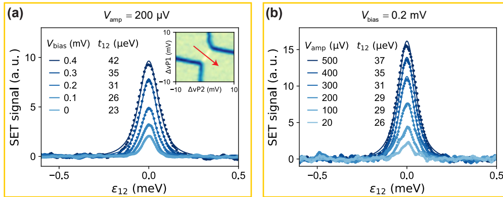
图 4.13 t_{12} 的拟合值随 (a) SET 直流偏置电压 V_{\text{bias}} 及 (b) lockin 的交流激励幅值 V_{\text{amp}} 的变化情况。插图 of QD1-QD2 的电荷稳定图，其中红色箭头代表失谐扫描的方向和位置。
