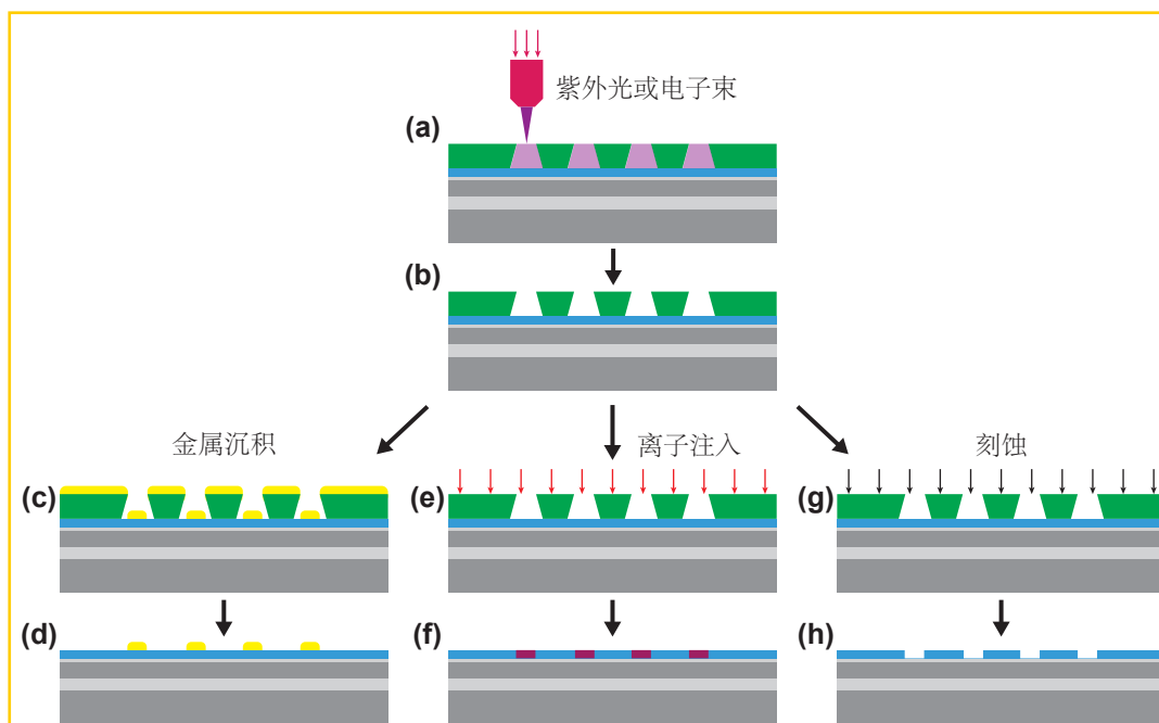
图 2.3 基于无掩模光刻技术的图形转移工艺。(a) 图形发生，采用紫外或电子束光刻。(b) 显影工艺。(c) 金属沉积及 (d) lift-off 工艺。(e) 离子注入及 (f) 去胶。(g) 刻蚀工艺（包括干法和湿法）及 (h) 去胶。
