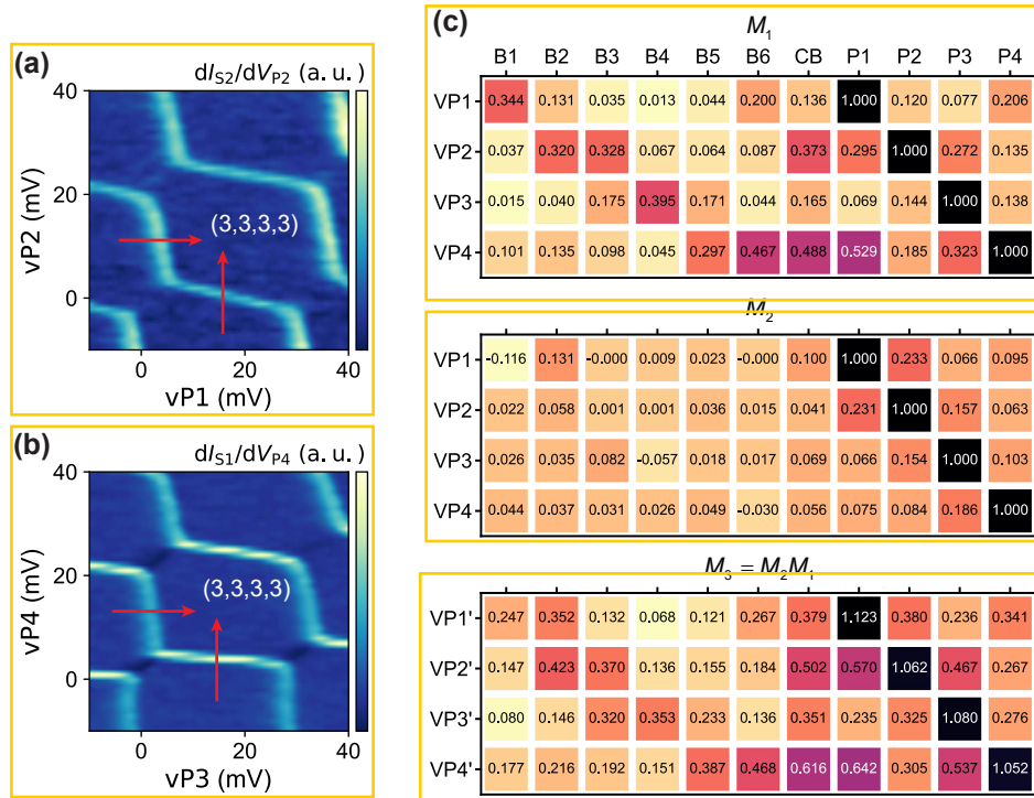
图 5.7 虚拟电极的更新。(a) OD1-OD2 和 (b) OD3-OD4 的电荷稳定图，用于提取新的串扰矩阵。红色带箭头的线代表扫描的具体位置。(c) 电容串扰矩阵，其中 M_1 、 M_2 和 M_3 = M_2 M_1 分别对应原始矩阵、新测量得到的矩阵和更新后的矩阵。
