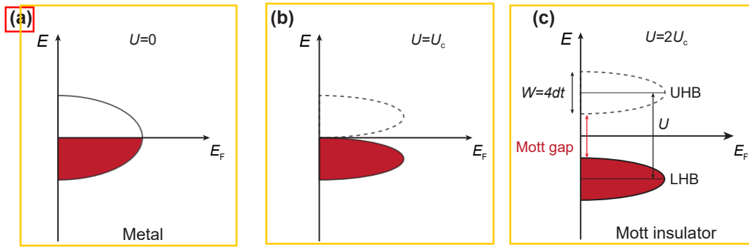
图 5.1 莫特金属到绝缘体转变的物理图像。系统能带结构随 U 变化的示意图：(a) U = 0 的情况，表现出金属态；(b) U = U_c 时，对应临界状态，即 U 恰好等于带宽 W ；(c) U = 2U_c ，表现出莫特绝缘态。图片修改自文献 [202] 。
