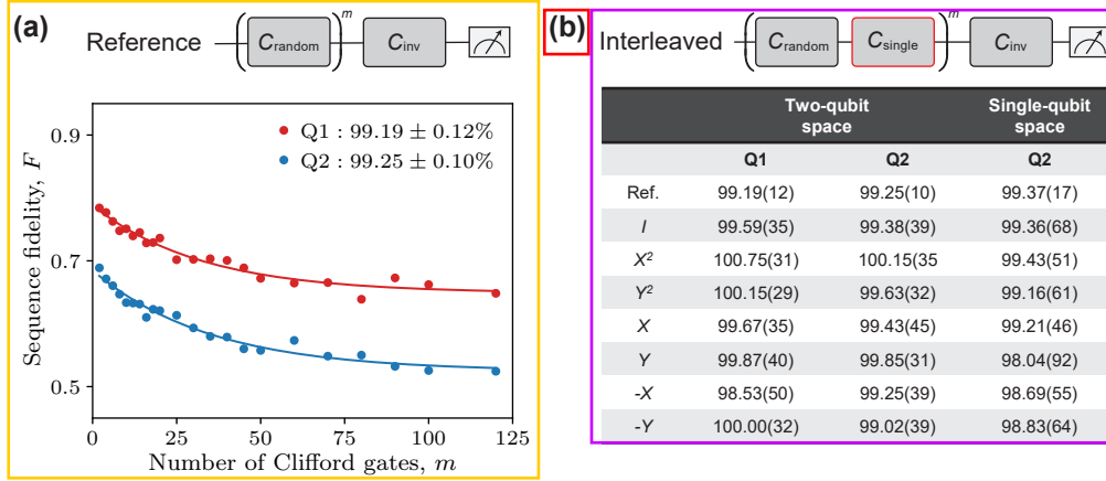
图 3.7 单比特随机基准测试。(a) 基于标准 RB 序列测得的初态保持概率随序列长度的衰减曲线，分别对应 Q1（红色数据点）和 Q2（蓝色数据点），其中实线为拟合结果。(b) 单比特和两比特空间中的 IRB 测量结果。每个数据点包含 15 个随机 Clifford 门序列，每个序列重复测量了 30 组，每组包含 200 次 single-shot 测量。
