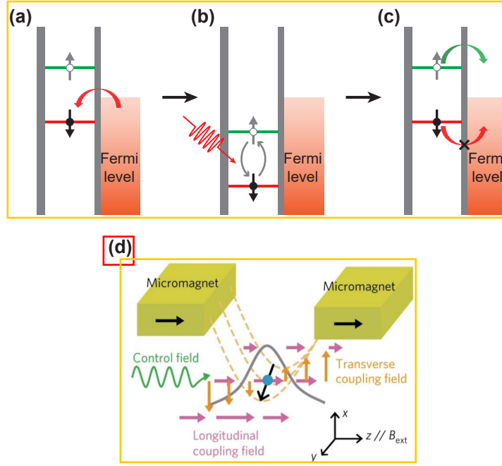
图 1.9 自旋量子比特的初始化与读出、操控原理图。(a) 利用源漏电子库将电子自旋初始化至 |\downarrow\rangle 态。(b) 通过微波驱动实现自旋量子比特的操控。(c) 能量选择性读出机制，自旋 |\uparrow\rangle 态的电子可以跳出量子点，而 |\downarrow\rangle 态则无法跳出。图片修改自文献 [107] 。(d) 基于微磁体的 EDSR 操控示意图，微波电场驱动电子在横向梯度磁场中振荡，从而产生一有效交变磁场。图片修改自文献 [33] 。
