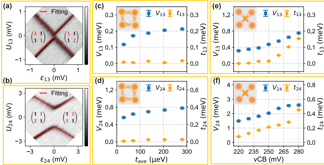
图 4.10 次近邻点间隧穿耦合。(a) 和 (b) 分别为 QD1-QD3 和 QD2-QD4 在失谐-能量坐标系下的电荷稳定图, 对应 (1,2)-(2,1) 反交叉。红色实线为采用双曲线函数对滤波后的数据 (90% 数据被过滤掉) 拟合的结果。(c) 和 (d) t_{ij} 和 V_{ij} 随最近邻隧穿耦合平均值 t_{ave} 的变化情况, 分别对应对角和反对角双点。左上角插图为量子点阵列耦合状态的示意图。(e) 和 (f) t_{ij} 和 V_{ij} 随中心势垒栅极电压 vCB 的变化情况, 分别对应角和反对角双点。在调控 vCB 时, 最近邻隧穿耦合均被置于弱耦合状态。
