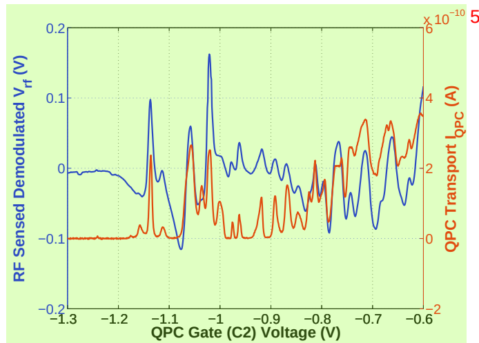
图 4.8 反射的射频信号解调制之后的电压 V_{rf} ，输运测得的量子点接触电流 I_{QPC} 分别与量子点接触的栅极 (C2) 电压的关系。
