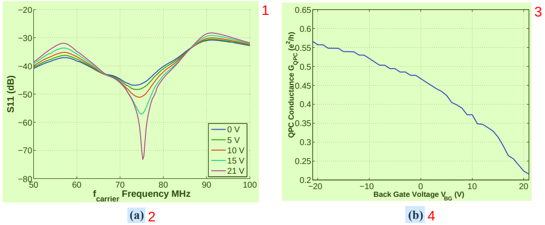
图 4.17 编号 WDCZ 的样品测量结果。(a) 量子点接触在不同的背电极电压下，功率反射系数与载波频率的关系。(b) 量子点接触在不同的背电极电压下的电导。
