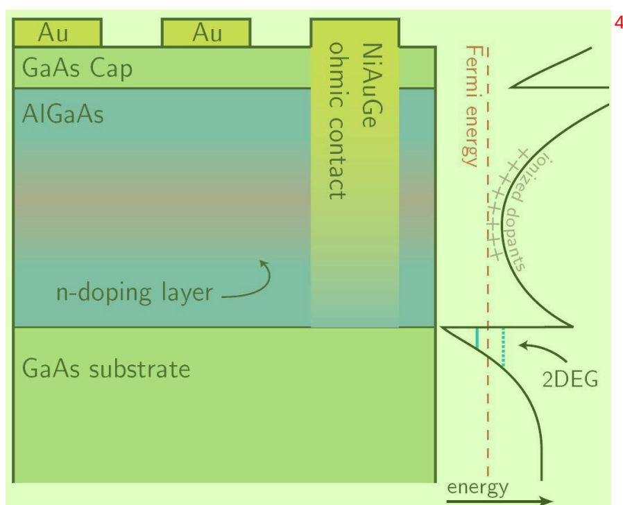
图 1.1 砷化镓/砷化镓铝异质结及其能带结构示意图。图片引自 5 (Switkes, 1999)。
