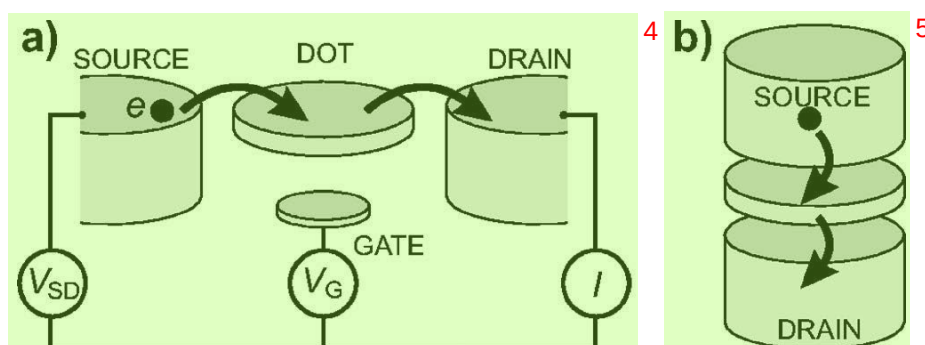
图 1.2 半导体量子点示意图。(a) 横向量子点。(b) 纵向量子点。图片引自 (Hanson et al., 2007)。
