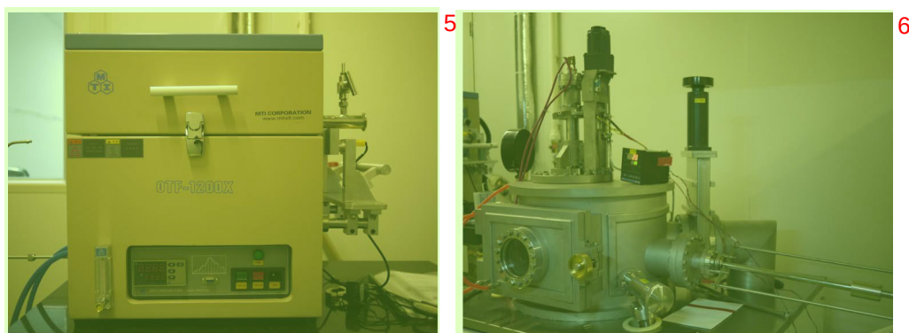
图 2.9 实验中所用到的快速退火炉。左为合肥科晶公司生产的 OTF-1200X 型快速退火炉。右为沈阳某企业生产的快速退火炉。 5 6
