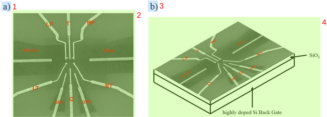
图 4.14 石墨烯量子点的扫描电子显微镜图像，包含一个双量子点及一个与之耦合的量子点接触结构。
