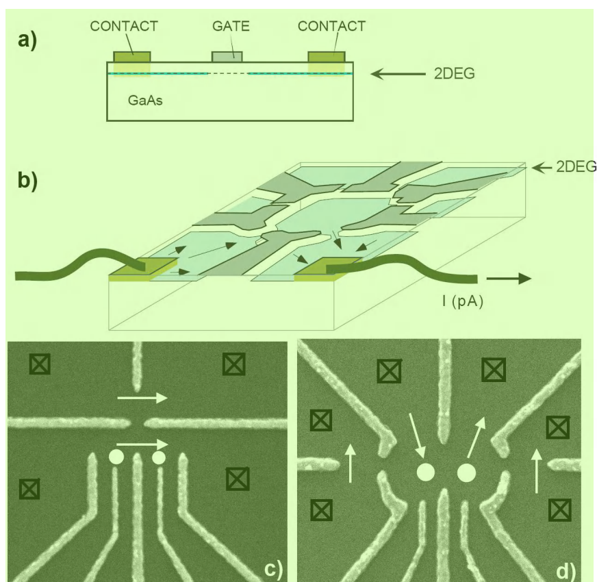
图 1.3 由金属表面电极形成的半导体门控型量子点示意图。(a) 侧视视角示意。(b) 透射视角示意。(c)(d) 扫描电子显微镜 (SEM) 下的双量子点, 由我们研究组自行制备。(a)(b) 图引自 (Huibers, 1999)。
