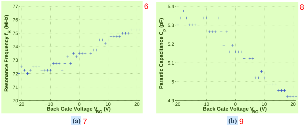
图 4.18 随着背电极电压改变，编号 WDCZ 的样品的寄生电容与谐振频率会发生改变。
