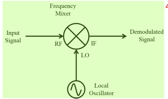
图 4.3 混频器解调制示意图。从谐振电路中反射的信号是由反射的参考信号与量子点接触的信号混频而成，经过混频器解调后可以得到解调之后的中频信号，而这个中频信号实时反应了量子点接触的电导。
