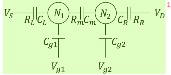
图 1.6 串联双量子点系统中等效隧穿电阻，电容示意图。
