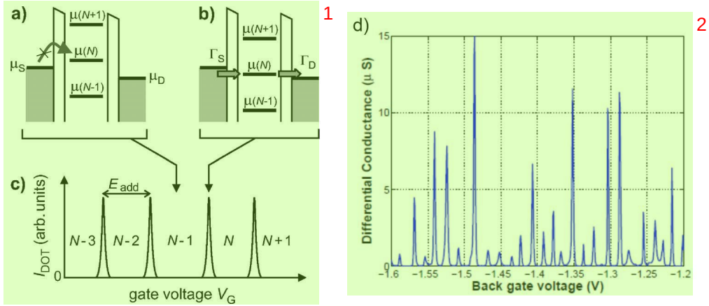
图 1.4 量子点的输运与库仑阻塞示意图。(a) 库仑阻塞现象。(b) 单电子隧穿现象。(c) 库仑阻塞电流示意。(d) 实验测得的库仑阻塞。(a)(b)(c) 图引自 (Hanson et al., 2007)。
