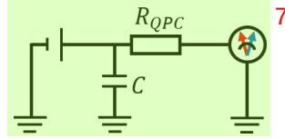
图 4.1 利用量子点接触作为电荷探测器进行测量的等效电路示意图。 8
