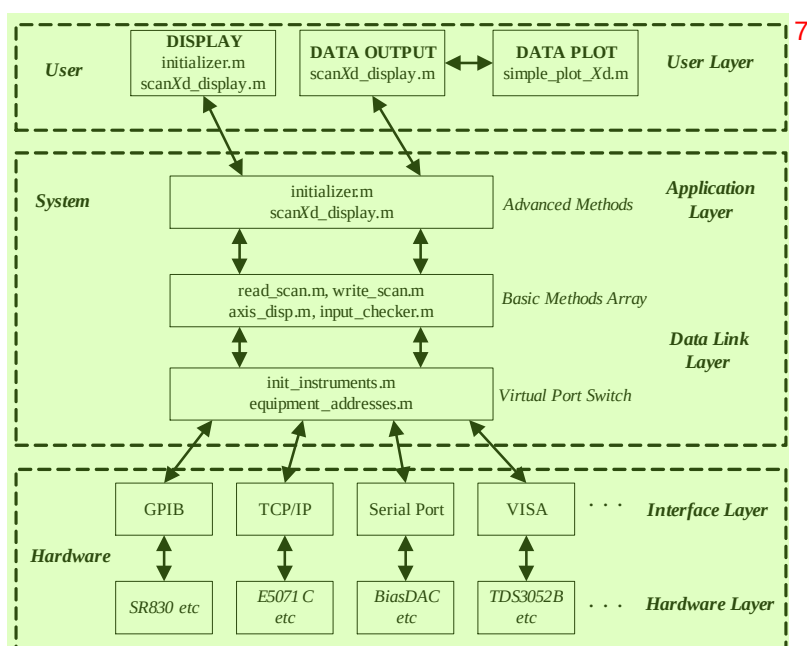
图 B.2 MATLAB 平台架构设计。
