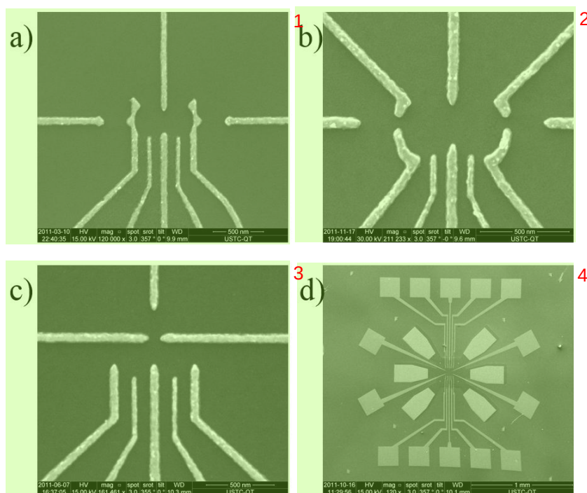
图 2.14 扫描电子显微镜所拍摄的由电子束曝光制版制成的量子点。 5 (a)(b)(c) 量子点中经过电子束曝光制版制备的小电极，每幅图的右下角展示了 500 nm 的长度标尺。(d) 量子点的整体图，右下角展示的长度标尺为 1 mm
