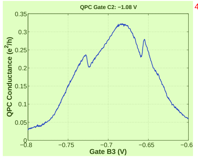
图 4.10 量子点接触的电导与量子点栅极 B3 上的电压的关系。电导台阶处说明量子点中电子的数目改变了 1。
