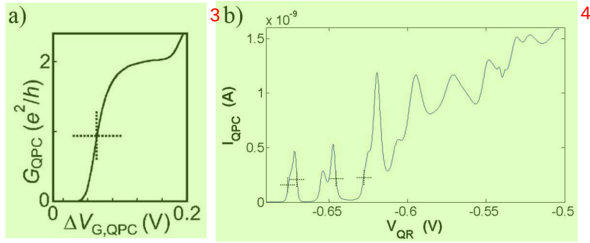
图 3.7 作为电荷探测器的量子点接触。(a) 调节电极 QR，量子点接触 5 的电导会出现量子化的电导平台。当其电导为最后一个平台的最陡峭处 G_{QPC} \sim e^2/h 时，其对与之耦合的量子点中的电子隧穿最为敏感。(b) 往往量子点接触在形成的过程中，不能理想的形成单调的量子化电导平台，而是形成类似与单量子点的结构，调节电极 QR，会出现于单量子点类似的库仑阻塞，这时将量子点接触的电导调至库仑峰两侧最陡，斜率最大的位置(十字叉标识的位置)，同样也是对与之耦合的量子点的电子隧穿最为敏感之处。(a) 图引自 (Hanson et al. , 2007)。
