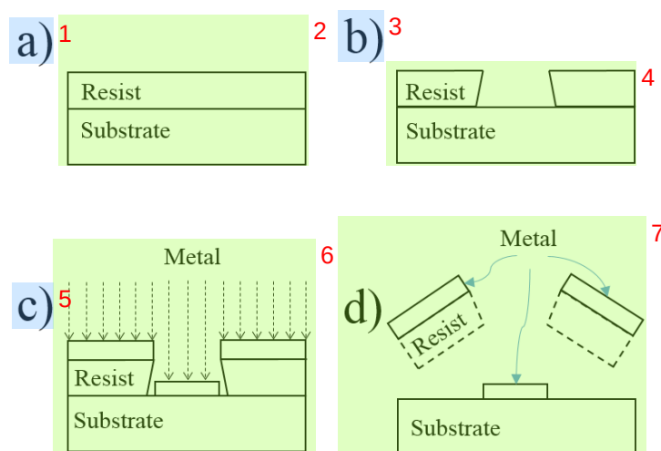
图 2.6 金属电极制备的剥离工艺。(a) 甩胶。(b) 显影之后的形态。(c) 金属镀膜。(d) 剥离。
