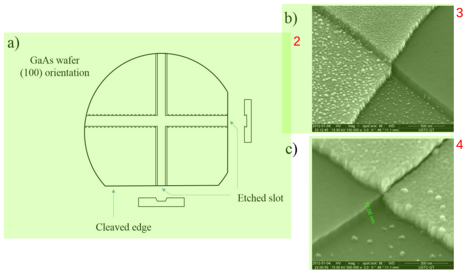
图 2.2 砷化镓晶体刻蚀结果示意。晶圆出厂时就带有一个沿晶面分解的缺口，当然我们也可以通过分解晶圆，来制造这个缺口。 5 (a) 刻蚀示意图，仅刻蚀晶圆上垂直于切割线的十字形区域，可以发现刻蚀边界一边呈坡面，与之垂直的一边呈凹面。 6 (b) 通过坡面刻蚀边界的表面金属电极。 3 (c) 通过凹面刻蚀边界的表面金属电极。 4
