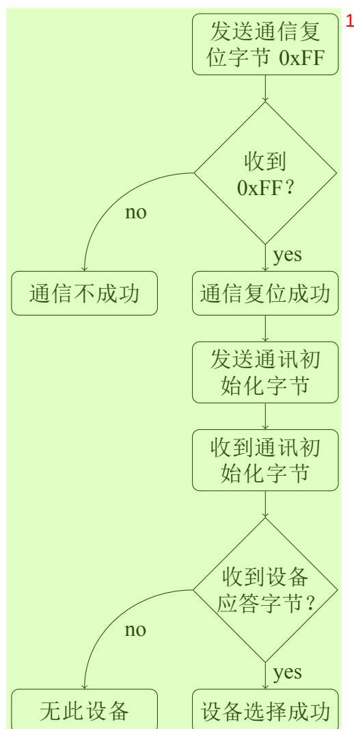
图 A.8 通信初始化的流程。
