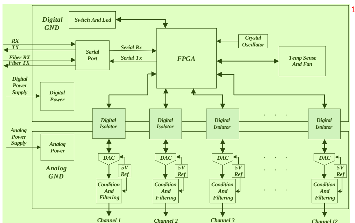
图 A.1 多通道高精度偏置电压源的电路结构示意图。 2
