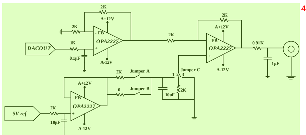
图 A.5 输出调理电路的结构示意图。 5
