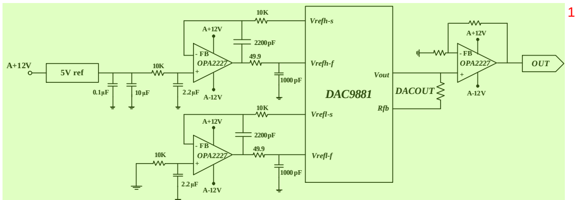
图 A.4 采用 TI DAC9881 芯片的模拟电路部分的结构示意图。 2
