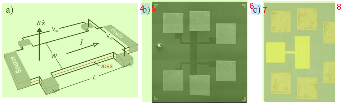
图 3.3 用于磁输运测量的霍尔棒样品示意图与照片。(a) 长度 L 宽度 W 的霍尔棒样品示意图，暗色区域表示欧姆接触，电流在二维电子气上流动，磁场垂直于样品。(b) 扫描电子显微镜下的霍尔棒样品。(c) 光学显微镜下的霍尔棒样品，在其上方额外制作了顶栅级。(a) 图引自 (赵勇杰, 2009)。 9
