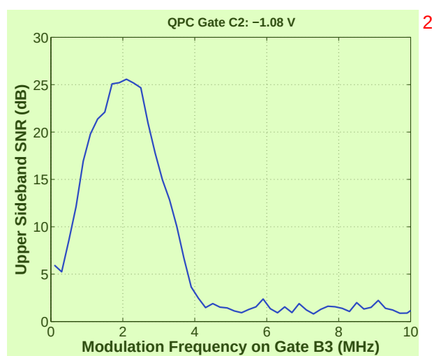
图 4.13 上边频带的信噪比，与叠加在量子点栅极 B3 上方波调制信号频率的关系
