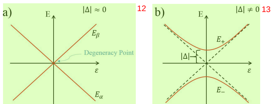
图 1.9 二能级体系能级示意图。(a) 无耦合或者耦合可以忽略时，能级交叉，出现简并点。 14 (b) 耦合相互作用时，能级反交叉。 15
