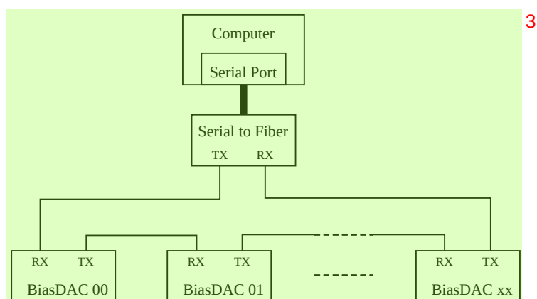
图 A.3 通过一根光纤链路形成的光纤环拓扑结构，同时控制多台偏置电压源。 4
