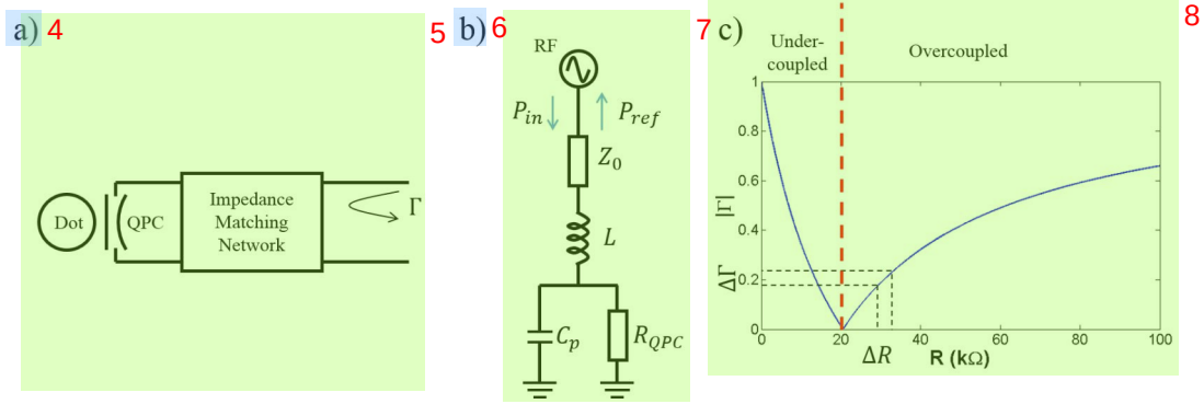
图 4.2 射频反射式测量阻抗匹配电路与等效电路示意图。(a) 阻抗匹配电路，作为电荷探测器的量子点接触与阻抗匹配电路相连接，将其阻抗转化为接近射频电路的特征阻抗 ( 50 \Omega )，加入一个射频信号后可以测量其反射的功率，从而得到反射系数 \Gamma 。(b) 等效电路，来源于引线电极，导线等的寄生电容 C_p 与电感 L 共同构成了阻抗匹配电路，这两者与量子点接触电阻 R_{QPC} 共同决定了电路的振荡频率 f_R 。当往电路中施加固定功率 P_{in} 的射频信号，反射的射频信号的功率 P_{ref} 由量子点接触电阻 R_{QPC} 决定。(c) 理论上的反射系数 \Gamma 与量子点接触电阻 R_{QPC} 的依赖关系。量子点接触电阻的改变 \Delta R 将导致反射系数的改变 \Delta \Gamma ，所以测量 \Delta \Gamma 可以反推出 \Delta R 。 9
