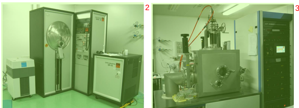
图 2.8 实验中所用到的镀膜机。左为 CHA 公司生产的 Mark 40 型电子束蒸发镀膜机。右为沈阳某企业生产的热蒸发镀膜机。
