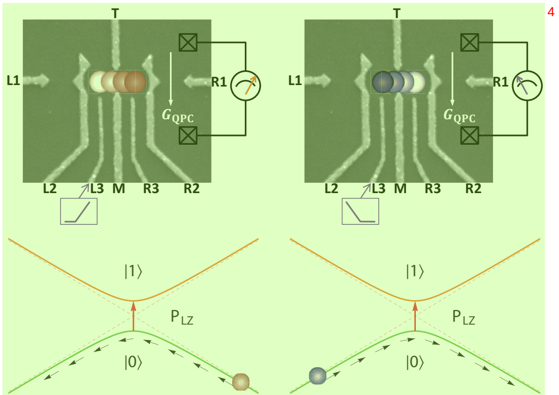
图 6.3 用双量子点中的电荷量子比特实现 Landau-Zener 跃迁过程。上：扫描电子显微镜下的带有量子点接触的双量子点，图中示意了价电子的占据状态，同时标明了脉冲叠加的栅极。下：受控的二通道 Landau-Zener 跃迁过程。
