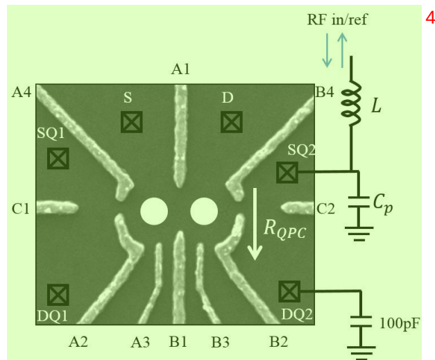
图 4.6 实验中使用的砷化镓量子点的扫描电子显微镜图像。图中标注了射频反射探测的电路原理示意。
