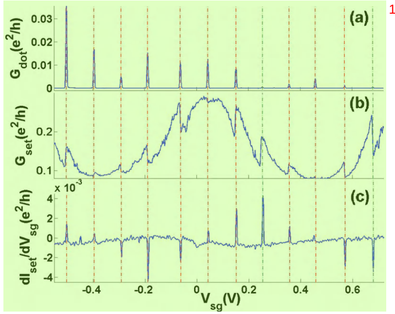
图 3.9 三种测量方式的结果比较，结果是一一对应的。(a) 3.3.1 节中介绍的量子点输运测量。(b) 3.3.2 节中介绍的利用量子点接触的输运性质对量子点进行测量。(c) 本节介绍的利用量子点接触对量子点的充电感应进行测量。图片引自 (Wang et al. , 2010)。
