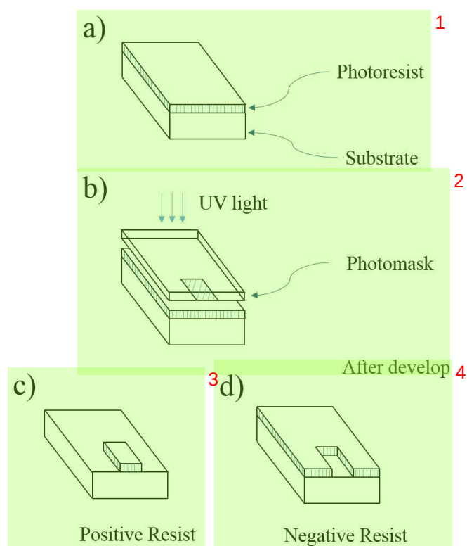
图 2.3 光刻曝光示意图。(a) 覆盖了光刻胶的基片。(b) 在基片上方放置光刻掩模版，然后用紫外光照射。(c) 显影之后，正胶留下与光刻掩模版相同的图案。(d) 显影之后，反胶留下与光刻掩模版互补的图案。
