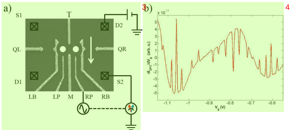
图 3.8 利用量子点接触对量子点的充电感应进行测量。(a) 在栅极 RP 5 上叠加一个微弱的低频交流或者方波激励信号，并将该低频交流或者方波信号与锁相放大器锁定，用锁相放大器直接从量子点接触的漏极上探测锁定的电流。通常我们会在量子点接触的源极上施加一个微小的直流偏置，使量子点接触上有一个微小的直流电流，但是锁相放大器并不会读出这个直流电流，而是会读出与低频交流激励同频同相的感应到的电流。(b) 实际的测量结果，其实读出的是微分电流信号 dI_{QPC}/dV_{RP} 。
