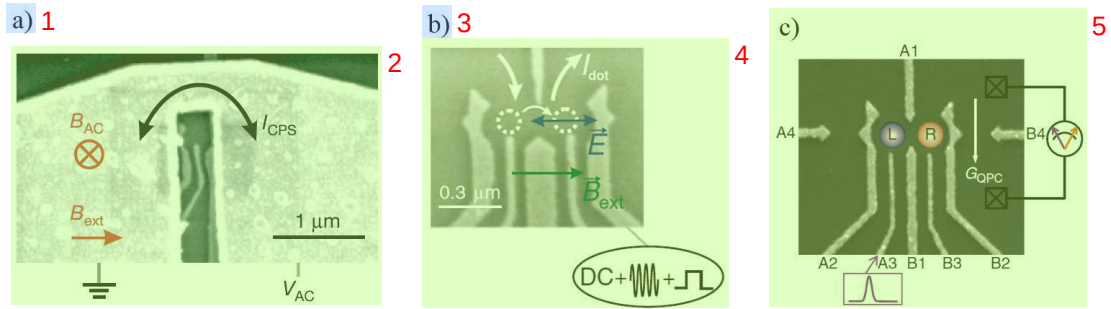
图 1.11 半导体门控型量子比特的几个物理实现。(a) 通过在双量子点上加工一个共面微带线，当射频电流通过其时，交变电流产生交变磁场 B_{AC} ，通过电子自旋共振 (Electron Spin Resonance, ESR)，翻转电子自旋，从而实现对自旋量子比特的操作。(b) 通过在双量子点电极上施加预设的脉冲序列与射频场的组合，通过电偶极自旋共振 (Electric Dipole Spin Resonance, EDSR)，影响其束缚电子的轨道自由度，并通过自旋轨道耦合相互作用 (Spin-Orbit Coupling)，翻转电子自旋，从而实现对自旋量子比特的操作。(c) 通过在双量子点电极上施加超快脉冲，改变电子在量子点中的束缚状态，从而实现对电荷量子比特的操作。(a) 图引自 (Koppens et al. , 2006)，(b) 图引自 (Nowack et al. , 2007)，(c) 图引自 (Cao et al. , 2013)。
