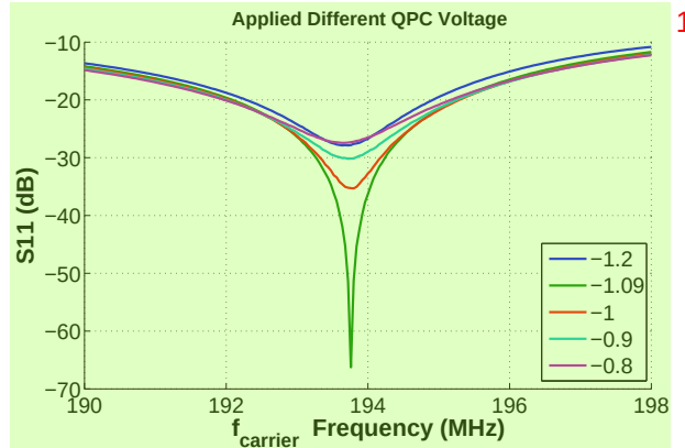
图 4.7 量子点接触的不同栅极电压下，测得的功率反射系数与载波频率的关系，振荡电路的谐振频率为193.8 MHz。
