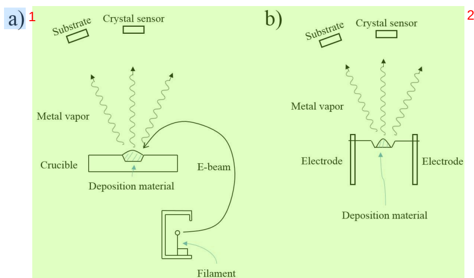
图 2.7 金属蒸发镀膜机示意图。(a) 电子束蒸发镀膜。(b) 热蒸发镀膜。
