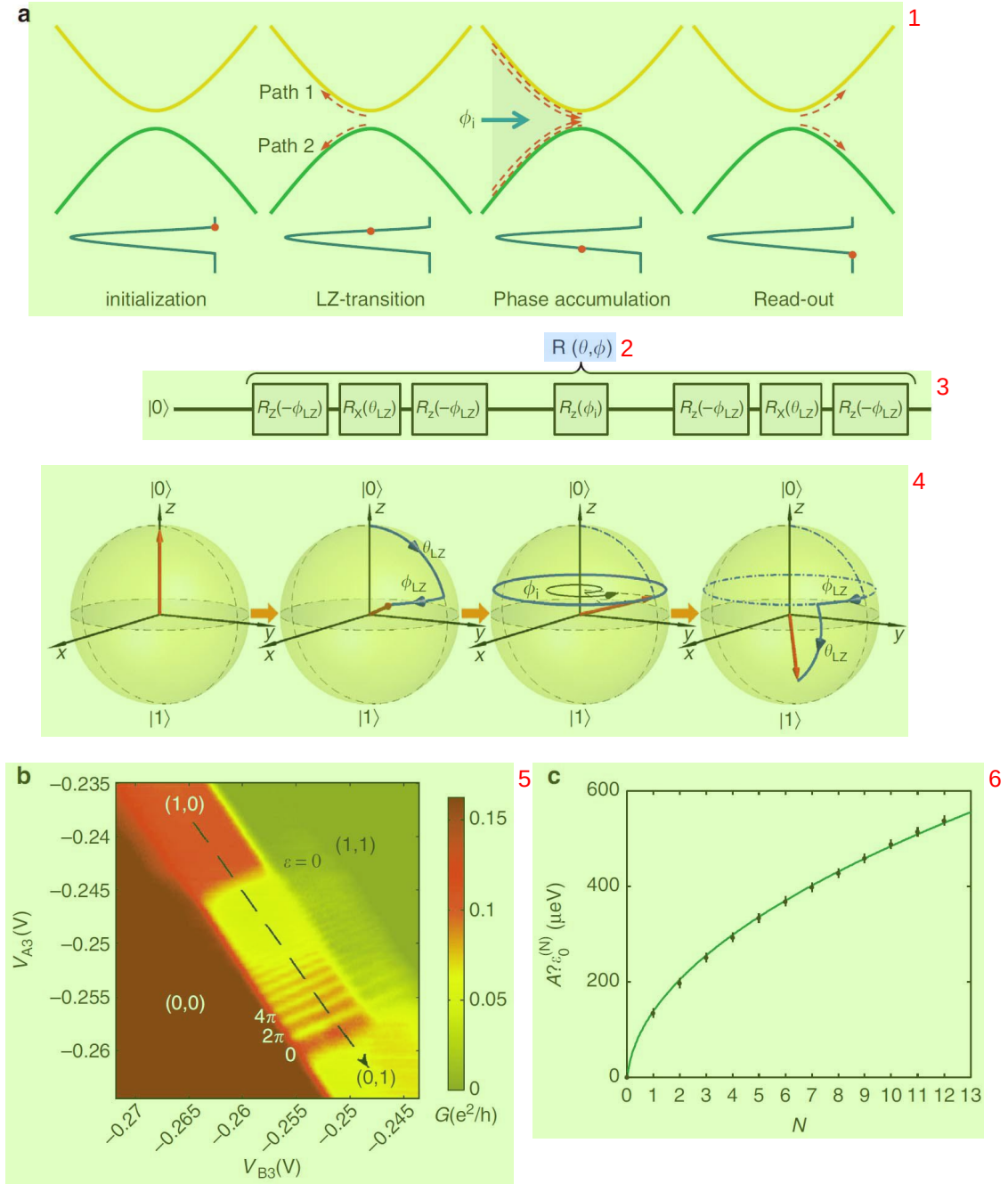
图 5.4 施加脉冲信号，实验中观察到电荷量子比特的 Landau-Zener-Stückelberg 干涉过程。(a) 施加脉冲时，电荷量子比特的能级演化，及其对应的在 Bloch 球面上的受控演化过程，包括绕 X 轴旋转的 R_x(\theta) 过程，和绕 Z 轴旋转的 R_z(\phi) 。(b) 在脉冲的驱动下，图 5.3(c) 所示的电荷分布相图发生改变，形成了一系列的干涉条纹。(c) 生成性干涉条纹的能量失谐的位置，与干涉次数 N 的关系，实线为理论算得。图片引自 (Cao et al. , 2013)。
