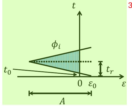
图 5.5 施加脉冲信号使体系的能量失谐随时间的演化示意。初始时体系的能量失谐为 \varepsilon_0 ，经过 t_0 时间的演化后，到达 \varepsilon = 0 的能级反交叉点，然后开始进行绝热演化，带来相位累积，最后再次穿越能级反交叉点，回到 \varepsilon_0 处。 4
