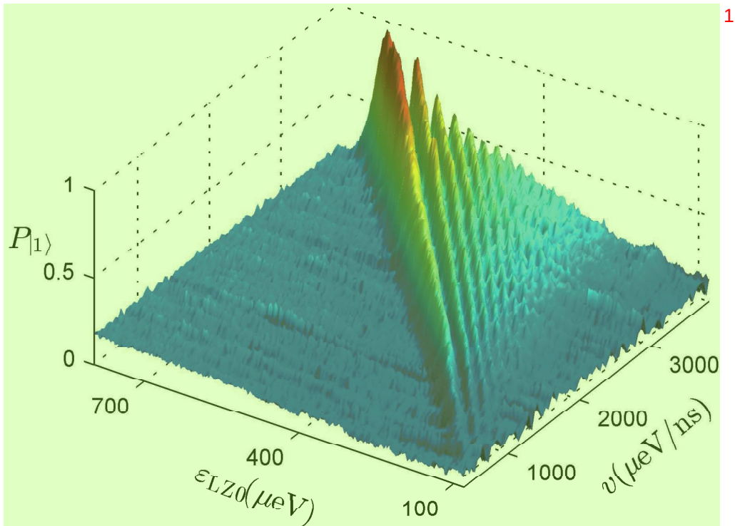
图 6.4 受控的 Landau-Zener 跃迁。电荷量子比特中 |1\rangle 态的占据情况与能级位置 \epsilon_{LZ0} ，及扫描速率 v 的关系，这是一个二通道的 Landau-Zener 跃迁过程。
