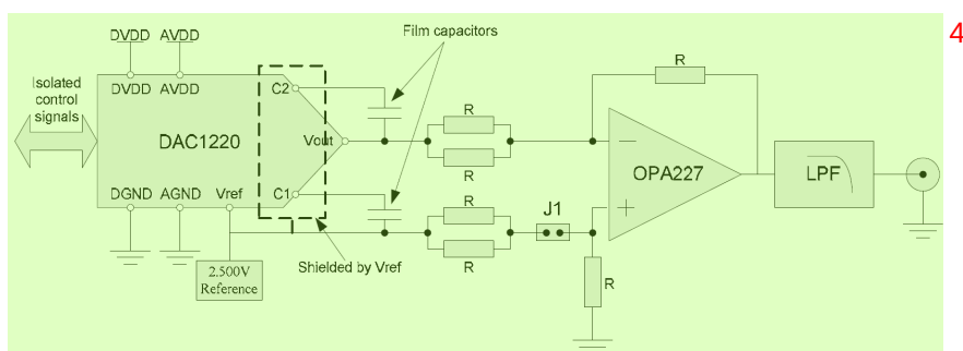
图 A.2 采用 TI DAC1220 芯片的模拟电路部分结构示意图。引自 (Huang et al., 2009)。 5
