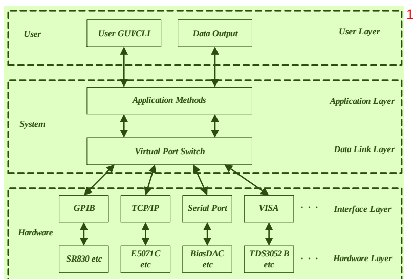
图 B.1 总体设计架构。
