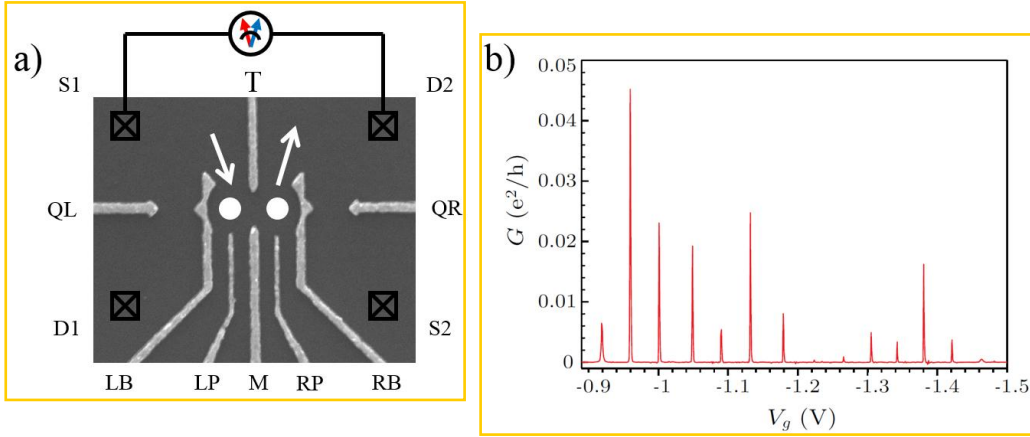
图 3.5 量子点输运测量。(a) 简要测量电路，通过量子点输运性质直接测量量子点中电荷的状态。(b) 实验实际测得的量子点输运的库仑阻塞图。
