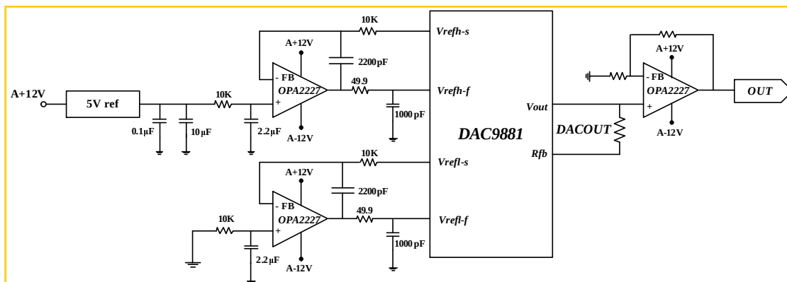
图 A.4 采用 TI DAC9881 芯片的模拟电路部分的结构示意图。
