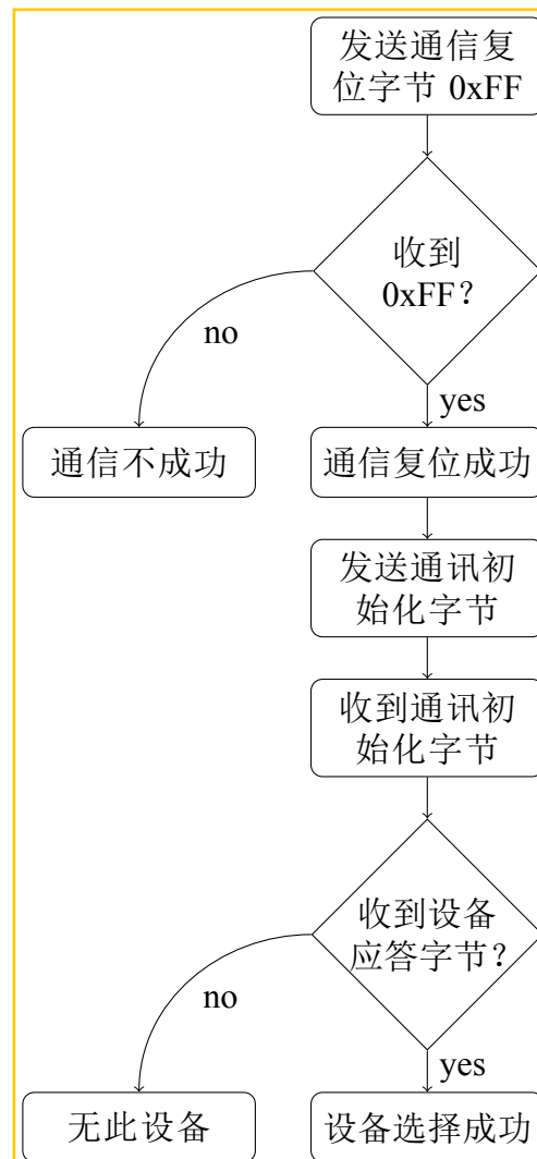
图 A.8 通信初始化的流程。
