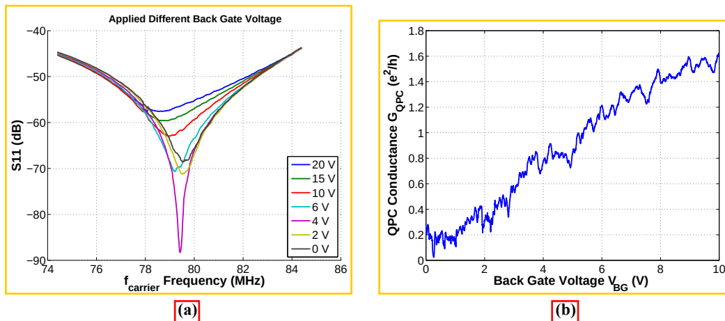
图 4.15 编号 SXX0307A 的样品测量结果。(a) 量子点接触在不同的背电极电压下，功率反射系数与载波频率的关系。(b) 量子点接触在不同的背电极电压下的电导。
