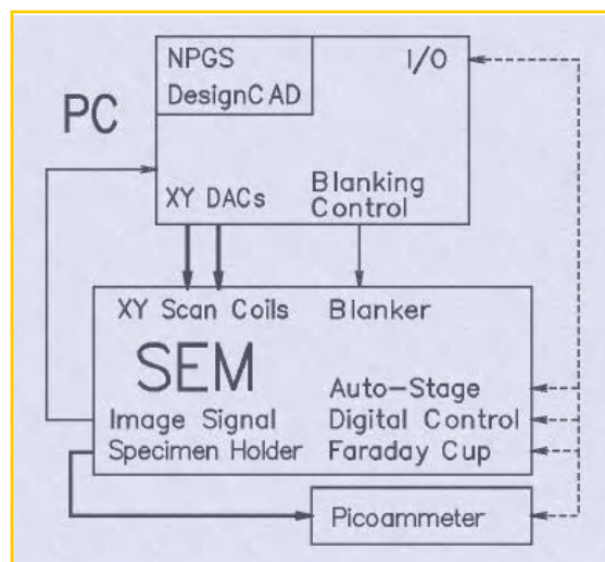
图 2.10 NPGS 系统原理框图，来源于 NPGS 软件帮助文件。
