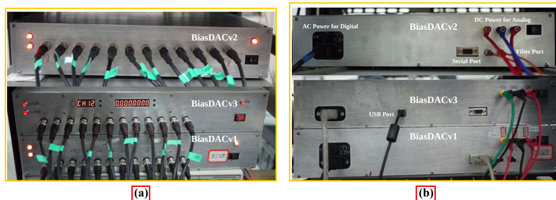
图 A.6 三个版本的比较。(a) 正面, v3 添加了通道与设定电压的显示。 (b) 背面, v3 省略了光纤接口, 添加了 USB 接口。
