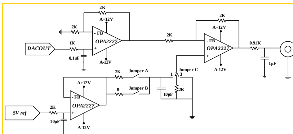
图 A.5 输出调理电路的结构示意图。
