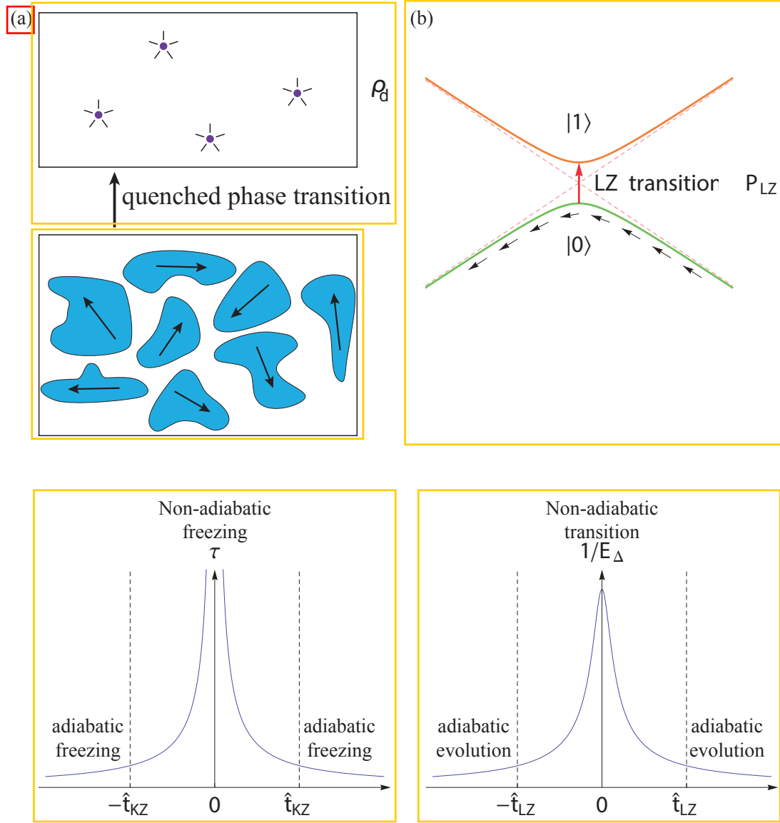
图 6.2 比较 Kibble-Zurek 机制与 Landau-Zener 跃迁。(a) 上：淬至对称性破缺的相变示意图，会产生拓扑缺陷 \rho_d ；下：Kibble-Zurek 机制中的两个区域：绝热冻结区域和非绝热冻结区域。在绝热冻结区域 [-\hat{t}_{KZ}, \hat{t}_{KZ}] 中(外)，弛豫时间 \tau 比淬火时间 \tau_Q 长(短)，所以此时的相被固定(演化)。(b) 上：二能级体系的 Landau-Zener 演化，以一定速度进行；下：由第 5 章 5.1 节中介绍的 Landau-Zener 跃迁的绝热-脉冲模型，我们也可以将跃迁过程分为两个区域：绝热演化区和非绝热跃迁区。在非绝热跃迁区中(外)，能量间隔的倒数 1/E_\Delta 小于(大于)扫描速度 v ，所以导致了非绝热跃迁 P_{LZ} (绝热演化)。
