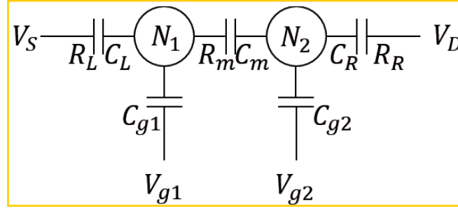
图 1.6 串联双量子点系统中等效隧穿电阻，电容示意图。
