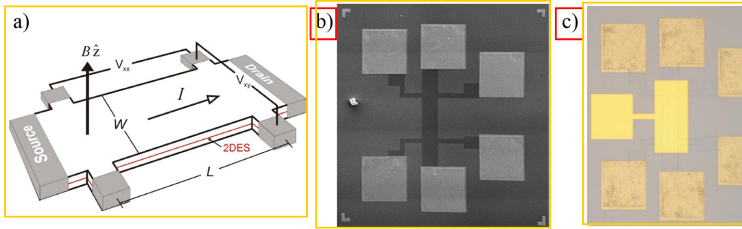
图 3.3 用于磁输运测量的霍尔棒样品示意图与照片。(a) 长度 L 宽度 W 的霍尔棒样品示意图，暗色区域表示欧姆接触，电流在二维电子气上流动，磁场垂直于样品。(b) 扫描电子显微镜下的霍尔棒样品。(c) 光学显微镜下的霍尔棒样品，在其上方额外制作了顶栅级。(a) 图引自 (赵勇杰, 2009)。
