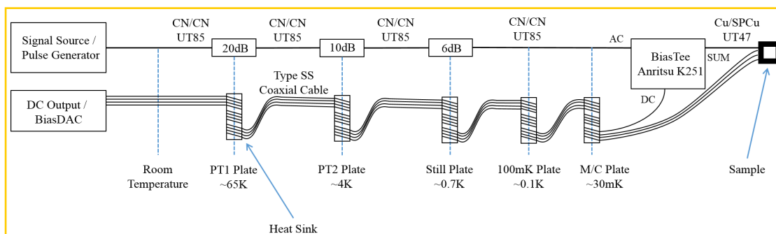
图 3.2 Triton 400 型无液氦稀释制冷机中直流与射频引线的设计示意。
