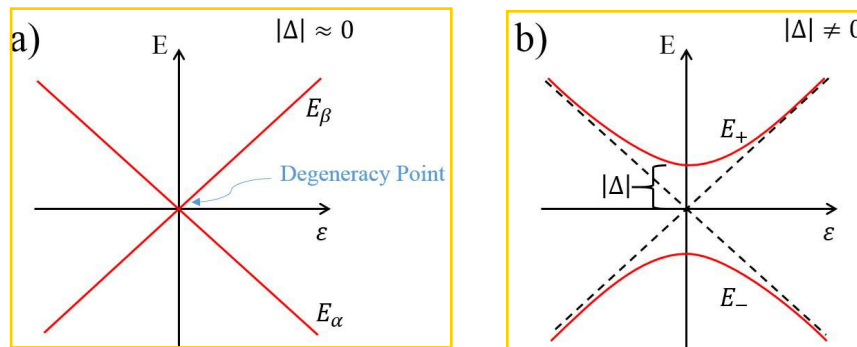
图 1.9 二能级体系能级示意图。(a) 无耦合或者耦合可以忽略时，能级交叉，出现简并点。(b) 耦合相互作用时，能级反交叉。
