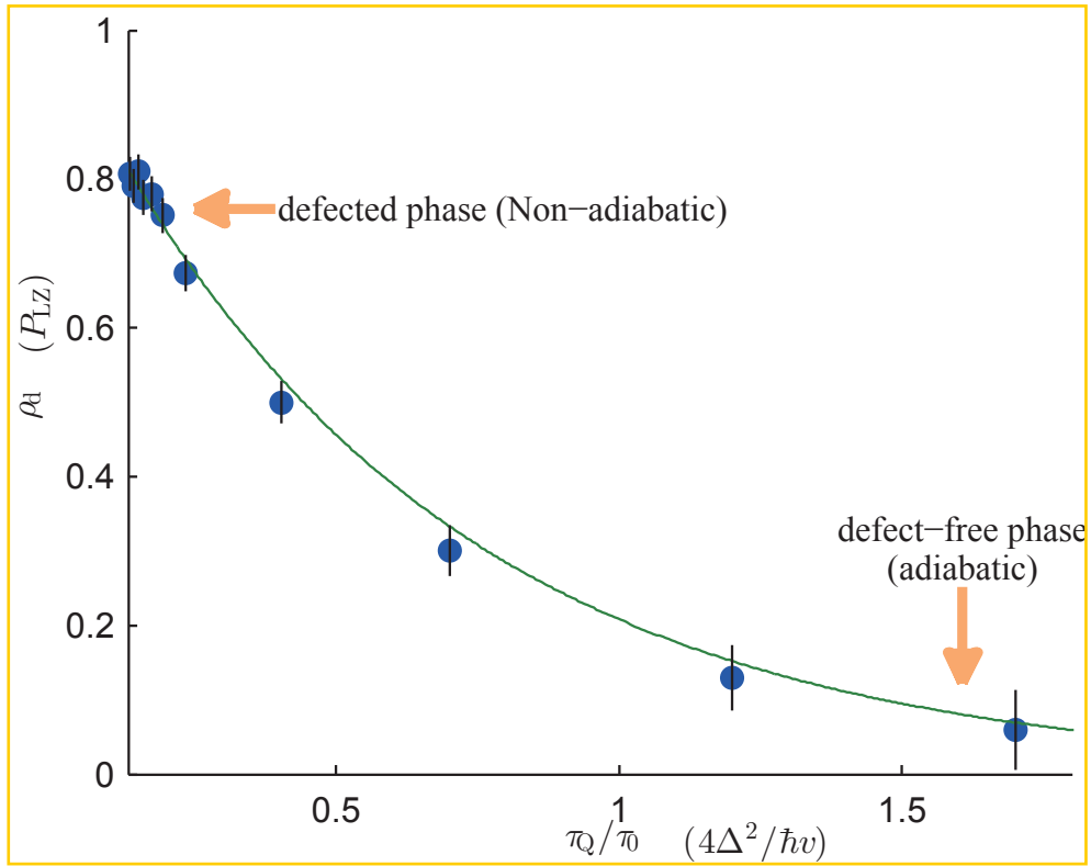
图 6.5 Kibble-Zurek 机制的量子模拟，拓扑缺陷密度与淬火速率相关。图中的点为归一化缺陷密度与淬火速率的关系，而曲线为式 6.23 的理论模拟。图中的坐标轴标注了对应的 Landau-Zener 跃迁中相对应的量。
