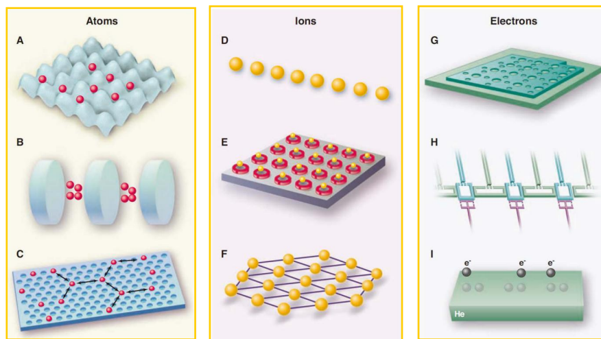
图 1.13 实现量子模拟的各种系统方案。(A) 光晶格束缚冷原子系统。(B) 一维光学腔阵列束缚冷原子系统。(C) 二维光学腔阵列束缚冷原子系统。(D) 离子链系统。(E) 二维共面离子阱系统。(F) 二维库仑晶体离子系统。(G) 量子点阵列束缚电子系统。(H) 超导电路阵列系统。(I) 液氦表面束缚电子系统。图片引自 (Buluta and Nori, 2009)。
