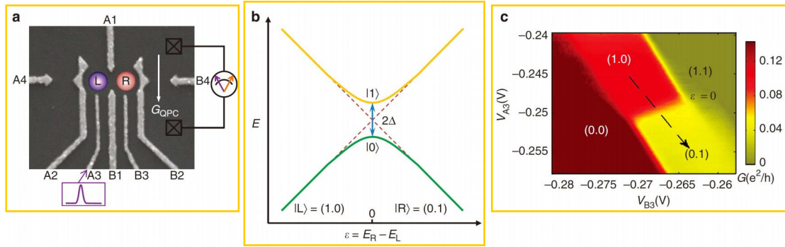
图 5.3 电荷量子比特实验中单电荷的控制与测量。(a) 扫描电子显微镜下的实验中所用到的带量子点接触的半导体双量子点。(b) 由双量子点构成的电荷量子比特能级示意图。(c) 由量子点接触作为电荷探测器测得的双量子点中的电荷分布。图片引自 (Cao et al. , 2013)。
