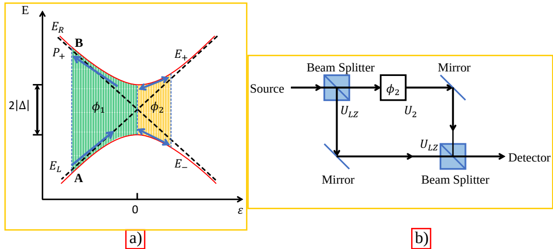
图 5.2 体系随时间经过能级反交叉点的演化示意图。(a) 体系从 A 点出发，经过能级反交叉点，在能级反交叉点的另一边累积了 \phi_1 的相位后，再次经过能级反交叉点，在 B 点测量。(b) 这一过程可以很形象的视作光学里的 Mach-Zehnder 干涉仪。
