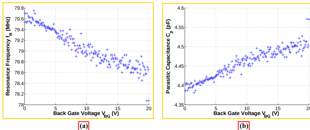
图 4.16 随着背电极电压改变，编号 SXX0307A 的样品的寄生电容与谐振频率会发生改变。
