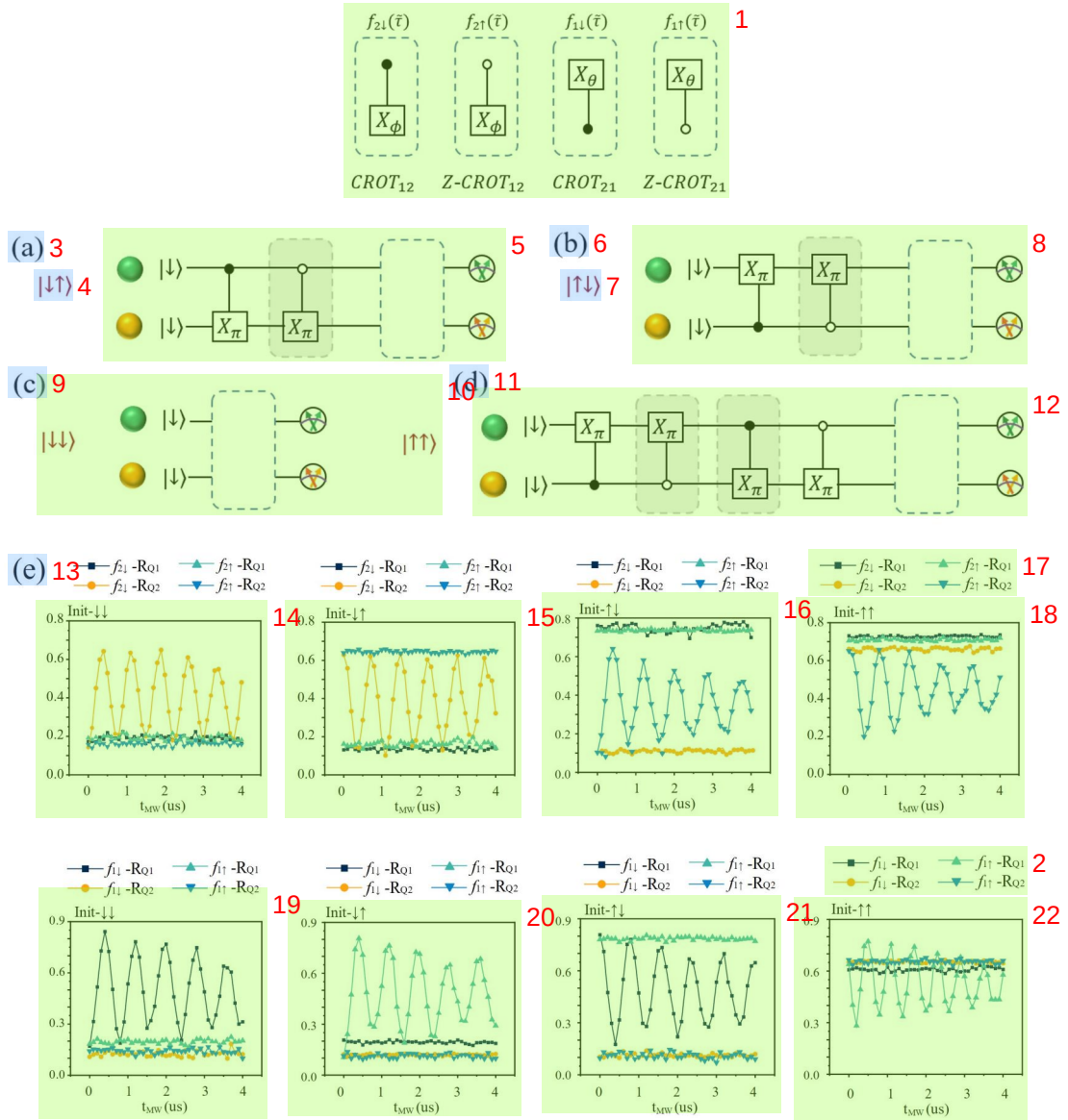
图 5.8 不同微波频率状态下的受控驱动。(a-d) 对两比特体系进行四种近似直积态的初始化，电子刚抵达电荷稳定图 E 位置时为 \downarrow\downarrow ，经过受控旋转门的操作将自旋初始化到不同的状态，然后对每种不同的初始化态进行四种受控旋转门的操作，改变持续的时间，其中 Q_2 比特的旋转角度为 \phi ， Q_1 比特的旋转角度为 \theta 。灰色框为在实际实验中未施加的操作，因为在确定开始为 \downarrow\downarrow 的情况下可以直接进行对应的受控旋转操作，每个白色虚线框中的操作为四种不同的 CROT_{ij} 和 ZCROT_{ij} 门 ( i, j = 1, 2 )。(a) 为初始化到 \downarrow\uparrow ，(b) 为初始化到 \uparrow\downarrow ，(c) 为初始化到 \downarrow\downarrow ，(d) 为初始化到 \uparrow\uparrow 。(e) 不同初始状态对不同受控旋转的测试结果，其中 R_{Qi} 为对第 i 个量子比特的读取。黄色的数据为不同初始化状态对 f_{2\downarrow}(\tau) 操作的结果，由于对应的 CROT_{12} 仅会在第二个量子比特上进行驱动，所以只会在初始化为 \downarrow\downarrow 或者 \uparrow\downarrow 的状态下进行旋转。同理的，蓝色的数据为不同初始化状态进行 ZCROT_{12} 操作之后的结果，也只会初始化为 \uparrow\downarrow 或者 \uparrow\uparrow 的状态下进行旋转。绿色的数据只会在 \downarrow\uparrow 或者 \uparrow\uparrow 的状态下进行旋转。黑色的数据只会在 \downarrow\downarrow 或者 \uparrow\downarrow 的状态下进行旋转。图中除了上述对应状态下发生的旋转以外，没有其它受控旋转门使初始态发生振荡（每张图中只有一个振荡），即没有发生非共振驱动。
