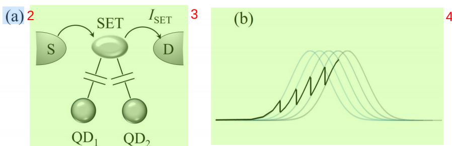
图 1.8 SET 探测原理 (a) 单电子晶体管 (SET) 探测量子点内电子数电路示意图，其中作为 SET 的单量子点通过输运电流的方式与被探测量子点产生电容耦合。(b) 量子点内电子数的变化使得 SET 电流产生偏移，产生锯齿信号，转化为电导信号即为一个信号峰或者谷，图中显示在 \text{QD}_1 中前五个填充电子的探测信号。
