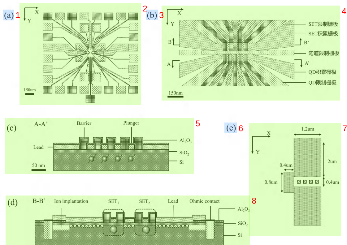
图 3.1 四量子点芯片结构图。(a) 四比特芯片整体平面图，电极的作用以及具体名称参照后续章节不同的具体的芯片。(b) 中间量子点区域的电极，指出了不同电极的功能。(c) 沿图 (b) 中 A-A' 的切面图，其中在四个柱塞栅极下定义了四个量子点。(d) 沿图 (b) 中 B-B' 的切面图，显示了两个 SET 的切面。SET 1 用来探测左侧的两个量子点状态，SET 2 用来探测右侧的两个量子点状态。(e) 微磁体形貌以及尺寸参数。
