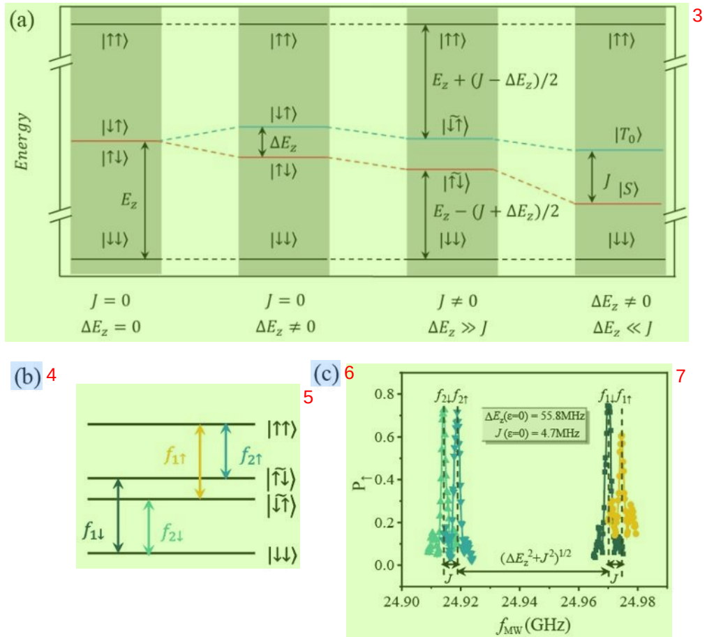
图 5.3 两比特体系的能谱。(a) 随着塞曼劈裂能级差大小和量子点间交换耦合相互作用的变化，两比特体系的能谱演化过程。(b) CROT 门操作所参考的能谱。(c) 两量子比特系统的 ESR 谱。我们在 |\downarrow\downarrow\rangle 、 |\downarrow\uparrow\rangle 或 |\uparrow\downarrow\rangle 中制备了 |Q_1, Q_2\rangle ，并测量了 Q_1 和 Q_2 的自旋上升概率作为应用微波频率的函数。由于有限交换耦合 J 和塞曼的能量差 \Delta E_z ，出现了四个不同的 ESR 峰。每个共振峰代表目标量子比特的状态（CROT 信号）的旋转。能级图将每个峰映射到一对双量子比特特征态之间的相应跃迁。
