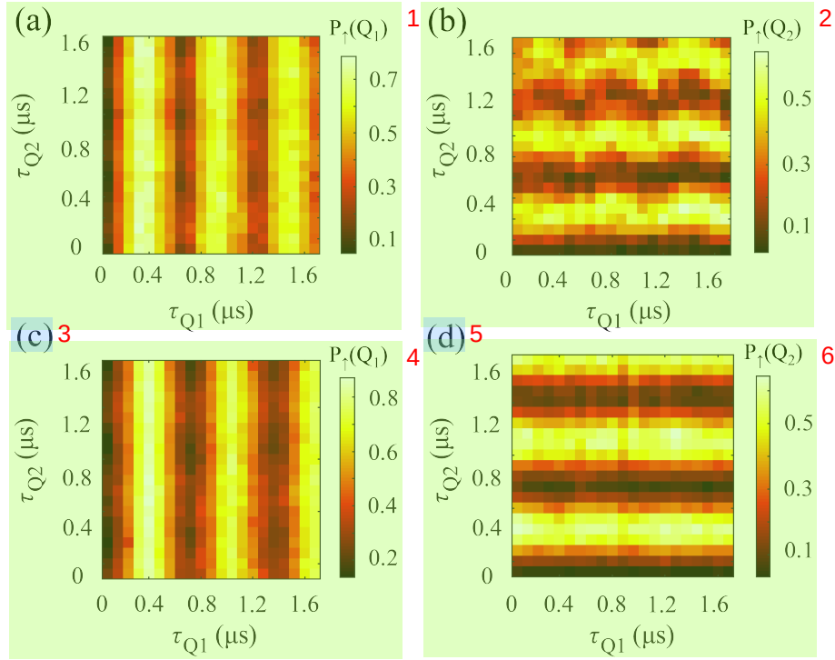
图 5.9 微波功率校正对合成单比特操控的影响。(a,b) 未对 ZCROT 门进行 AWG 幅度的校准的独立单比特操作, (a) 为 Q_1 比特的振荡, (b) 为 Q_2 比特的振荡, 会发生振荡的不均匀。(c,d) 对 ZCROT 门进行 AWG 幅度的校准的独立单比特操作, (c) 为 Q_1 比特的振荡, (d) 为 Q_2 比特的振荡, 振荡均匀。
