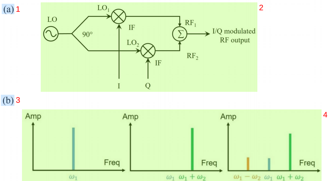
图 3.6 IQ 混频。(a)IQ 混频器的原理图。(b)微波源的本振输出。(c)理想情况下的上变频。(d)有相位误差以及偏置误差时的输出频率。
