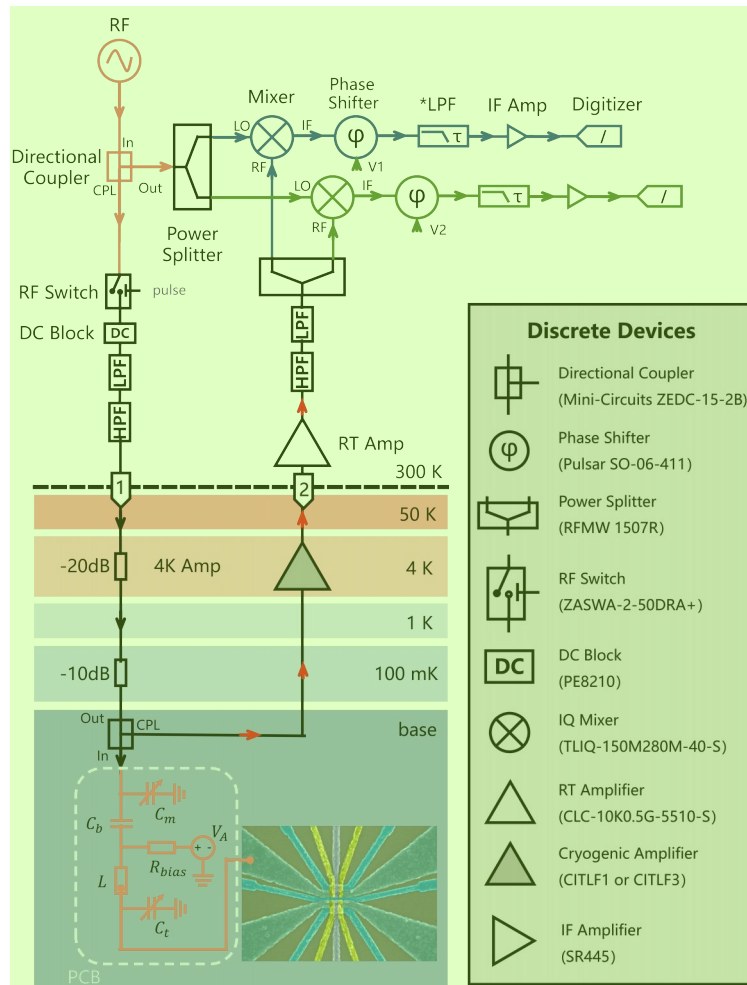
图 6.9 射频测量装置的示意图。一个栅极定义的单量子点耦合到包含电感 L (860 nH)、可变电容 C_t 和 C_m 以及固定电容 C_b (100 nF) 的阻抗匹配网络。载波频率设定为 160.1 MHz。为了探测匹配网络，射频信号在通过 30 dB 衰减器和定向耦合器后注入端口 1。信号在反射和放大后到达端口 2。反射信号在室温下通过与本地振荡器混合进行解调。通过改变 V_1 和 V_2 以调整移相器的相位，可以通过数字化仪检测信号的不同正交分量。射频开关的目的是在除读出阶段外的其他阶段保持静默。偏置电阻 R_{bias} 允许我们测量器件的直流传输电流。灰色框中是示意图中使用的器件类型。
