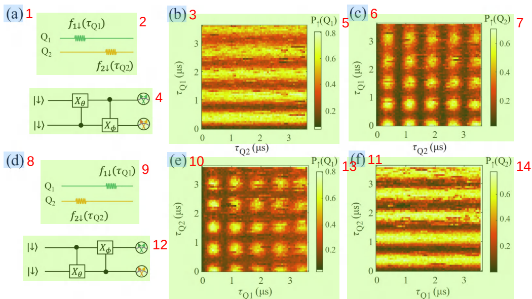
图 5.7 控制旋转门操作。(a) Q_1 作为控制比特, Q_2 作为目标比特的控制旋转操作的波形图以及量子线路图。(b) 控制比特 Q_1 产生的独立振荡。(c) 目标比特随着控制比特相干状态的变化而产生周期振荡的消失与出现。(d,e,f) 将控制比特与目标比特交换之后的控制旋转门操作结果。
