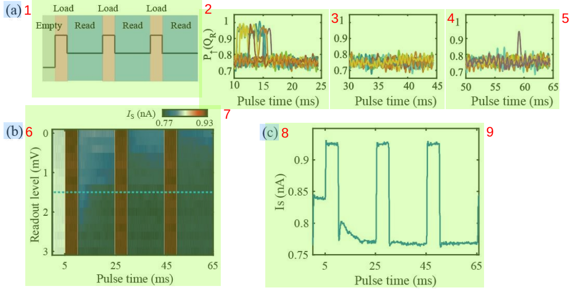
图 2.2 单发读出位置标定。(a) 用于旋转读出的三级脉冲序列。Empty 和 Load 电压水平保持不变，而 Read 级别则从高到低进行扫描，后续跟的加载和读出过程用来进行读出正确与否的判断。(b) SET 的输运电流 I_s ，平均 200 次 d 单发读出的轨迹，作为在读取阶段的电压水平的图像变化。用应用磁场 B=0.7T 采集的数据。(c) 在 (b) 中蓝色切线位置处的电信号，①区域为读取的窗口阶段，在合适的区域中会产生 spin-bump 的信号。②③为判断读取位置合适的监视，如果这两个监视窗口的单发读出高电平比例过高 ( >0.2 )，则说明暗计数太多，需要重新矫正读取位置。
