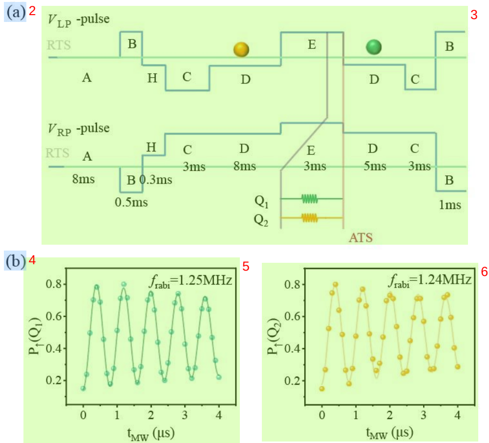
图 5.2 两比特测试区域对两个单比特的控制。(a) 对 LP 和 RP 使用的波形序列, 在 V_{LP} -pulse 中给出了每个阶段的持续时间, H 为 (2,1) 和 (3,0) 电荷区中间处, 理论上这两种不同的能级在此处产生 anti-crossing, 会出现弛豫的热点, 适合于自旋的快速初始化, 在后续的实验中为了加快测量速率, 我们将这个 H 点省去了。绿色的 RTS 线表示设置的波形零点位置, 红色 ATS 表示触发采集卡采集的位置, 整体的单发读出的时间为 28\ \text{ms} 。(b) 在两比特区域两个比特的各自的 Rabi 振荡, 显示了两个比特平均 1000 次后的读出信号轨迹。通过调节两个微波源的功率使得两个比特的 Rabi 频率相同, 为 f_{rabi} = 1.25(1)\ \text{MHz} , 这样在后续的操作中可以固定单比特旋转 \pi 角度的持续时间为 400\ \text{ns} 。
