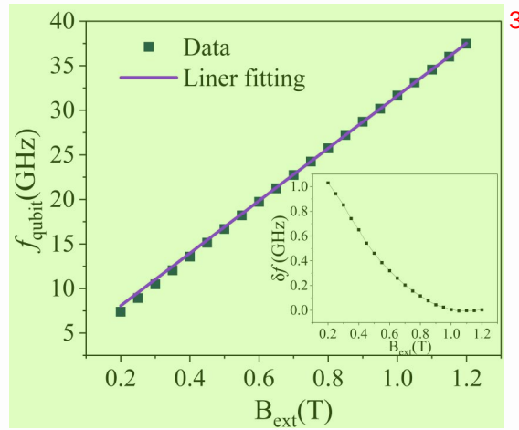
图 4.12 微磁体饱和极化。拉莫尔进动频率随外部磁场强度的变化趋势，紫色线为线性拟合，插图为实验数据与拟合数据的差值。 4
