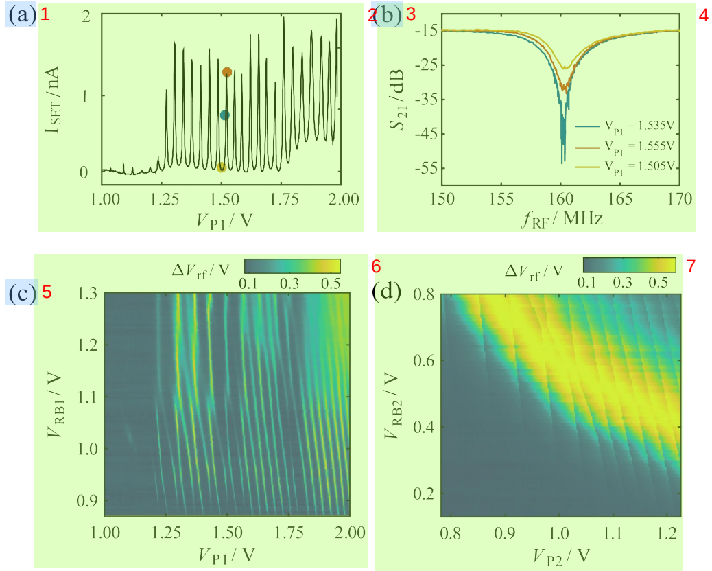
图 6.7 Si-MOS 中的射频探测。(a) SET 直流电流 I_{\text{SET}} 随栅极电压 V_{P1} 变化的示意图。对一 8 个欧姆接触施加 500 \mu\text{V} 的直流偏置电压，另一个欧姆接触通过放大器连接到电压表。同时， 被探测的量子点 \text{QD}_2 的两个欧姆接触均接地。SET 的传输电流依赖于柱塞栅极电压 V_{P1} 和 偏置电压。(b) 在 (a) 面板中不同颜色的三个圆圈位置观察到反射信号。单电子晶体管的反 射系数 S_{21} 随着柱塞栅极电压的变化而变化。当实现阻抗匹配时（用蓝色表示），灵敏度达 到最大。 -15 \text{ dB} 的背景反映了从定向耦合器的耦合端口到输入端口的衰减，并考虑了额外的 电路衰减。(c) 通过射频反射计测量的 \text{QD}_1 的电荷稳定性图，图中显示了解调后的电压信号。 (d) \text{QD}_1 用作检测器来测试 \text{QD}_2 的信号。锯齿状信号表明电子的跃迁。黄色背景表示 (a) 中 的库仑峰。图片来源于文献 [200] 。
