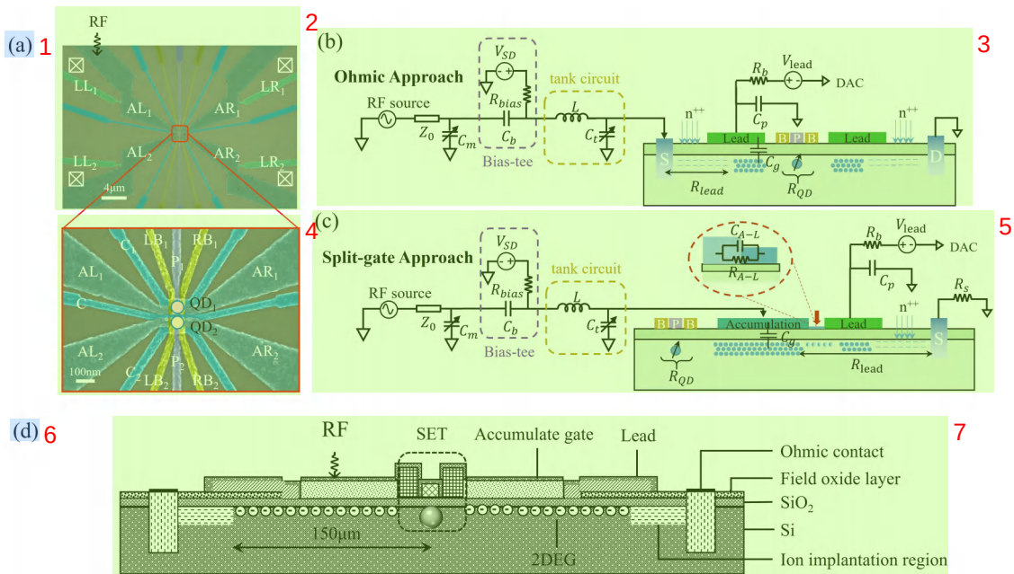
图 6.5 Si-MOS 中的劈裂栅极结构。 (a) Si-MOS 器件的伪彩色 SEM 图像。为了便于相互检测，我们设计了一个对称结构。下标 1 和 2 表示上下两侧具有完全相同的结构。两个量子点 QD_1 和 QD_2 分别位于栅极 P_1 和 P_2 下方（紫色），并在栅极 LB_1 、 LB_2 、 RB_1 和 RB_2 下方形成势垒（黄色）。限制栅极 C_1 、 C_2 和 C 用于控制量子点的横向尺寸。先前的大引线栅极被分为两层：引线栅极（LL 和 LR）和劈裂累积栅极（AL 和 AR）。在测试中，我们利用上方的量子点作为 SET 来检测来自下方量子点的信号，射频电路连接到 AL1 栅极。(b) 欧姆方法。在欧姆设计中，偏置三通（紫色虚线）和储能电路（黄色虚线）在 PCB 上实现。 R_{lead} 表示累积在引线栅极下方的二维电子气的电阻，它阻止了射频信号的泄露。 C_g 表示引线栅极与二维电子气之间的电容，它导致射频信号的泄露。 C_p 是来自键合线和累积栅极到 PCB 接地平面的寄生电容。 R_b 是 PCB 上的电阻，用于防止射频信号泄露到直流线路中。匹配电容 C_m 可以将射频电路与高阻抗的 SET 匹配。 n^{++} 是离子注入区域。(c) 劈裂栅极方法。射频信号施加到累积栅极。引线栅极和累积栅极被分成两部分，减少它们的重叠以最小化电阻 R_{A-L} 和电容 C_{A-L} 。重叠区域的长度为 0.1\ \mu\text{m} ，宽度为 0.3\ \mu\text{m} 。为方便起见， R_{A-L} 包含在引线栅极至欧姆接触电阻 R_{lead} 中。(d) 劈裂栅结构的横截面图。离子注入区位于距 SET 中心 150\ \mu\text{m} 处。 \text{Al}_2\text{O}_3 层厚度为 30\ \text{nm} ，芯片中心 100\ \mu\text{m} \times 100\ \mu\text{m} 区域中的氧化铝已被蚀刻掉。图片来源于网络文献 [200] 。
