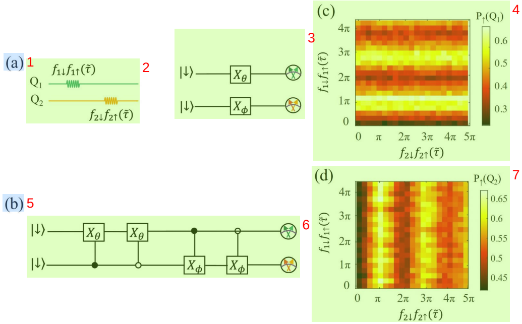
图 5.6 受控旋转合成单比特。(a) 在恒定交换相互作用 J 的存在下，通过在两个条件频率 8 上同时施加微波脉冲，可以实现独立的量子比特控制。第一个脉冲 f_{1\downarrow}f_{1\uparrow}(\tau) 施加到 Q_1 上，第二个脉冲 f_{2\downarrow}f_{2\uparrow}(\tau) 施加到 Q_2 上。右图为两个单比特实现的线路，其中 \theta 为第一个脉冲所对自旋的 bloch 球上产生的极相位， \phi 为第二个脉冲所对自旋的 bloch 球上产生的极相位。(b) 两个独立单比特控制的详细控制线路。(c,d) 两个独立量子比特控制的结果，(c) 为 Q_1 比特单独控制的读出，(d) 为 Q_2 比特单独控制的读出。
