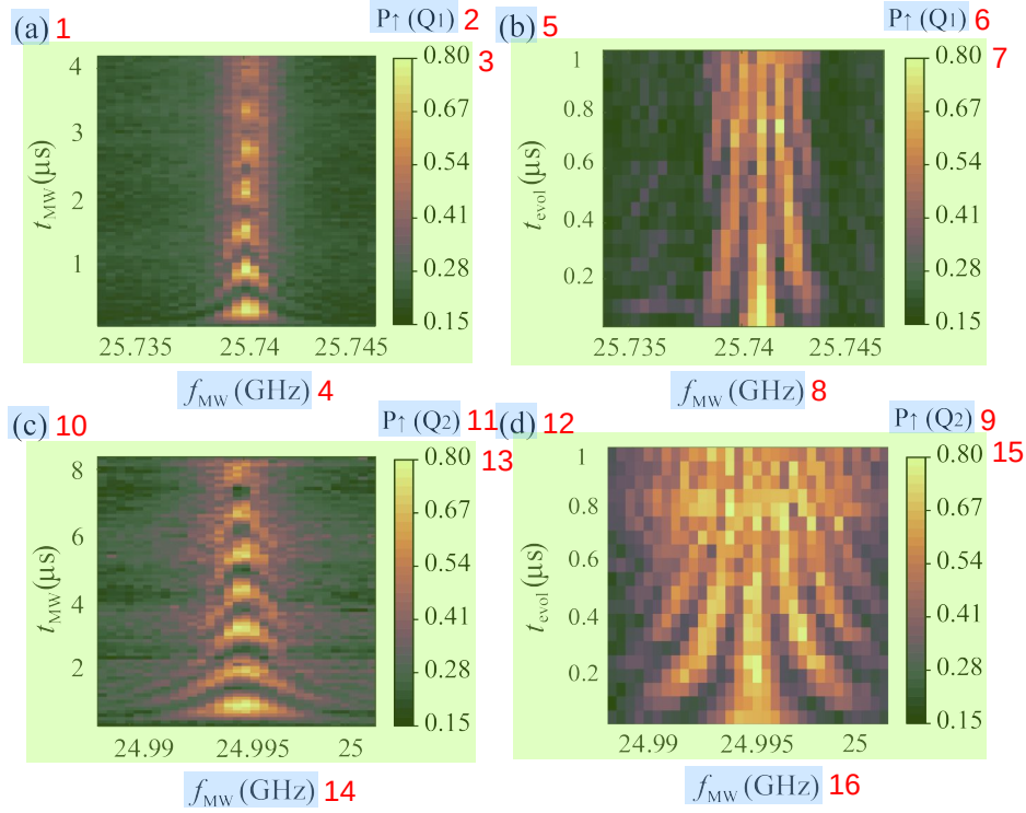
图 5.24 两个单比特的 chevron 图。(a) Q_L(Q_1) 量子比特自旋向上的概率 P_{\uparrow}(Q_1) 绘制为微波频率 f_{MW} 和驱动时间 t_{MW} 的函数，显示相干拉比振荡。(b) Q_L 比特在拉姆齐序列下测试的结果，横轴为微波频率，纵轴 t_{evol} 表示两个 \pi/2 之间的自由演化时间。(c) Q_R(Q_2) 量子比特的 Rabi-chevron。(d) Q_R(Q_2) 量子比特的 Ramsey-chevron。
