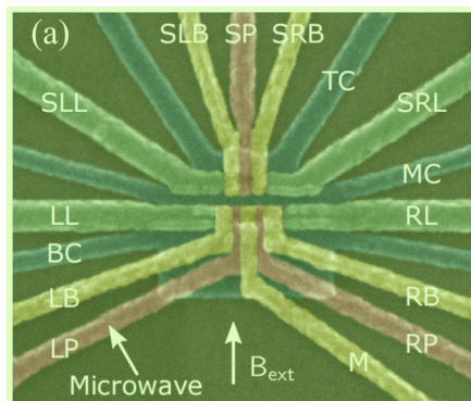
图 1.6 Si-MOS 样品的三维结构以及纵切面。(a) Si-MOS 上样品结构的示意图，蓝色电极为第一层，绿色与粉色栅极为第二层，黄色栅极为第三层。(b) 在衬底上，电极上的电压束缚出一个双量子点 (DQD) 和一个单电子晶体管 (SET) [59] 。
