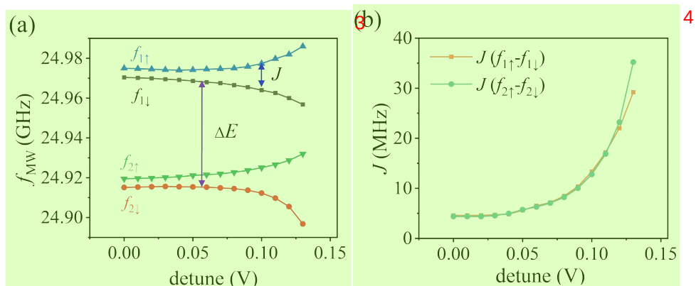
图 5.4 交换相互作用常开情况下的能谱。(a) 四种共振峰随失谐量变化。(b) 提取出的交换相互作用强度随失谐量的变化，近似于指数上升，其中在零失谐的位置 J 为 4.8(4) MHz。
