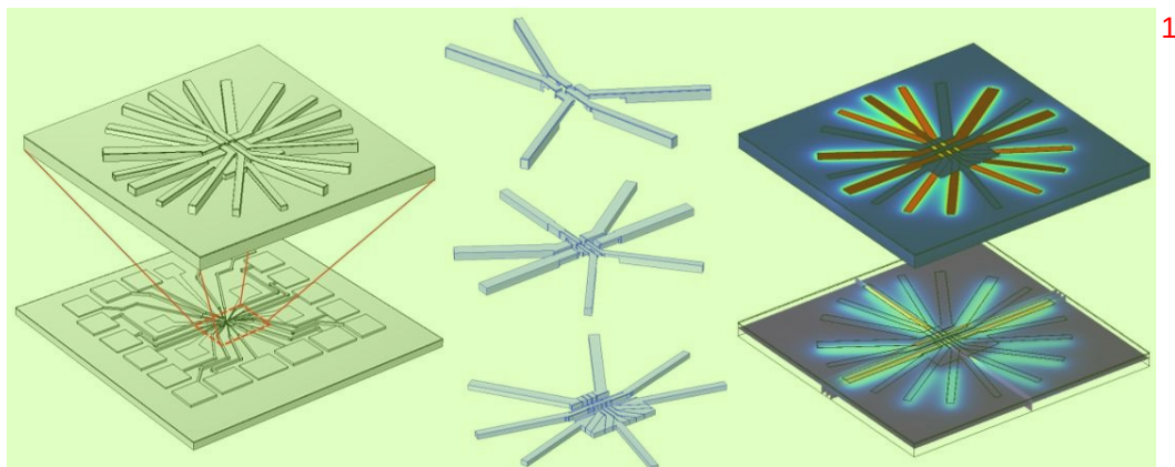
图 3.2 双量子点芯片立体结构图。(left) 芯片不同尺度下的示意图。(middle) 从下往上是第一层的限制栅极(厚度 35 nm), 第二层的引线 and 柱塞栅极(厚度 55 nm), 第三层的势垒栅极(厚度 75 nm)。(right) 上方基片表面(后续称为表面)上的电场和下方的纯化硅与氧化硅界面(后续称为界面)的电场图, 做了切面。图片由 COMSOL 软件进行电场模拟, 图片仅为示意图, 目的是模拟表面和界面电场, 而电极厚度实际是叠加的, 为了不影响观察, 我们对厚度做了调整, 但仍可以保证表面所受的电压是实验上施加的实际电压。
