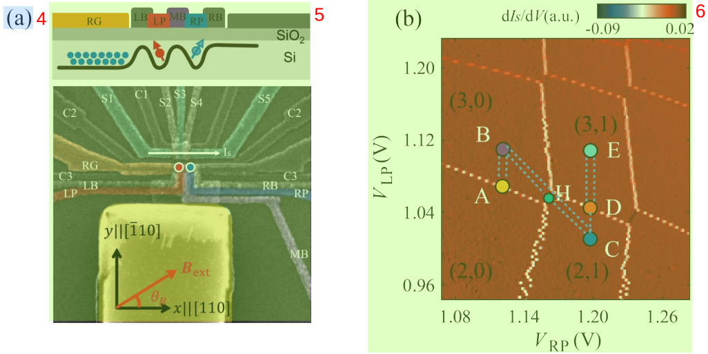
图 5.1 两量子比特器件以及两比特体系的操控波形。 7 (a) 两量子比特设备原理图和假彩色扫描显微镜图像。两个比特分别位于栅极 LP (红色) 和 RP (蓝色) 的下方，它们之间的约束势垒在栅极电极 MB (紫色) 的下方形成，右侧的势垒栅极 RB 和引线栅极都关闭。单电子晶体管位于 S3 下，量子点状态的变化通过影响 SET 的电流 I_S 进行探测。实验上施加的磁场为 B_{\text{ext}}=777 \text{ mT} ， \theta_B = -90^\circ 。(b) 在 LP 和 RP 下形成的两个量子点的电荷稳定性图。这些点中的电子数用 (N_L, N_R) 表示。在 A 点进行 Q_L 比特的初始化，通过 B 点和 C 点的过程将初始化之后的 Q_L 转移到 Q_R 去，然后在 D 点再进行 Q_L 比特的初始化，最后到 E 点，此时在完成初始化的 E 点进行两个量子比特的操控。而读出阶段为初始化阶段的反过程，即在 D 点进行 Q_L 比特的读出，然后通过左右量子点中电子的隧穿之后，将 Q_R 的自旋状态通过 A 点进行读出
