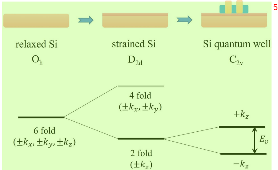
图 4.2 硅中的点群对称性。上图为 Si-MOS 在制备过程中点群对称性逐步减小的过程，从体晶硅的 O_h 到应变硅的 D_{2d} ，再到电极施加电势导致的 C_{2v} 。下图为硅中的六个简并谷态在不同结构下的简并和劈裂。
