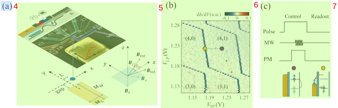
图 4.3 样品以及测试。(a) 实验中测量的器件的示意图和假彩色扫描电子显微镜图像。标出了栅极电极和微磁体。通过 SET 的电流 I_s 用白色箭头表示。外部磁场 B_{\text{ext}} 与 x 轴之间的角度为 \theta_B 。SEM 图像下方是说明微磁体和 Q_R 量子点之间几何关系的示意图，其中对微磁体结构进行了几何建模。插图：不同磁场的笛卡尔坐标和标签。(b) 图中显示了在 LP 和 RP 下方形成的两个量子点的电荷稳定性图。这些点中的电子数表示为 (Q_L, Q_R) 。橙色圆圈表示读出位置，而紫色圆圈表示控制位置。(c) 测量方案的示意图，说明如何通过偏置器将直流电压以及脉冲和微波 (MW) 波形施加到 RP 电极。在控制阶段 (10 ms)，量子比特由微波脉冲驱动，脉冲调制 (PM) 有助于控制微波开关，从而实现更高的微波开关比。在读出阶段 (10 ms)，执行能量选择性读出。如果电子处于自旋向上状态，它可以隧穿到电子储存器中并加载自旋向下的电子，从而完成初始化过程。相反，如果电子处于自旋向下状态，则不会发生跃迁。图片来源于文献 [174] 。
