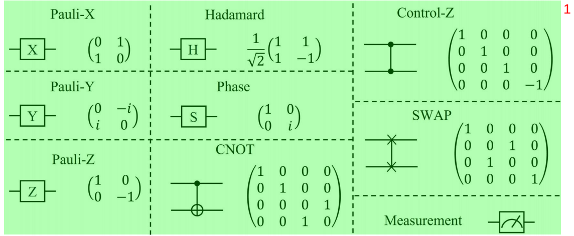
图 2.5 比特门 2
