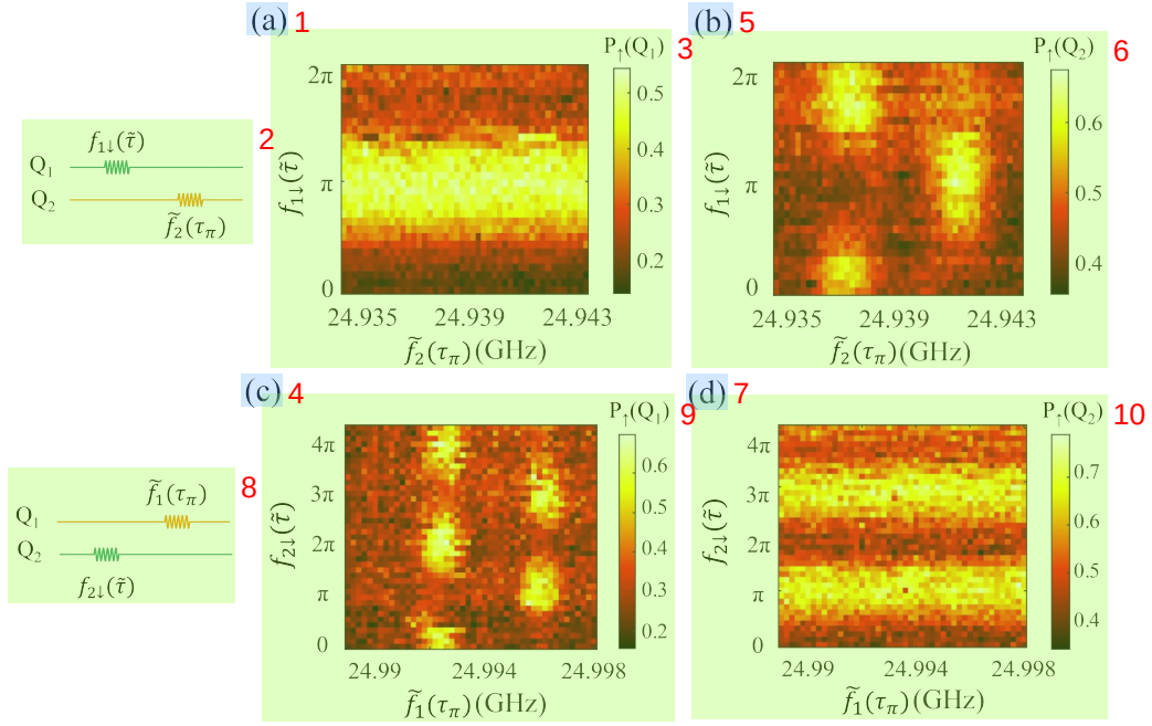
图 5.5 不同控制比特状态下受控比特共振频率的偏移。(a,b) 受控的量子比特旋转是通过在个别共振频率上的脉冲来自然实现的。第一个脉冲 f_{1\downarrow}(\tilde{\tau}) 在 Q_1 上进行 Rabi 旋转，导致 Q_2 的共振频率在 f_{2\downarrow} 和 f_{2\uparrow} 之间振荡，(a) 图为对 Q_1 比特的测试结果，(b) 图为对 Q_2 比特的测试结果。(c,d) Q_2 为控制比特， Q_1 为受控比特的旋转，第一个脉冲 f_{2\downarrow}(\tilde{\tau}) 在 Q_2 上进行 Rabi 旋转，导致 Q_1 的共振频率在 f_{1\downarrow} 和 f_{1\uparrow} 之间振荡。左侧线路为对两个比特施加的波形。
