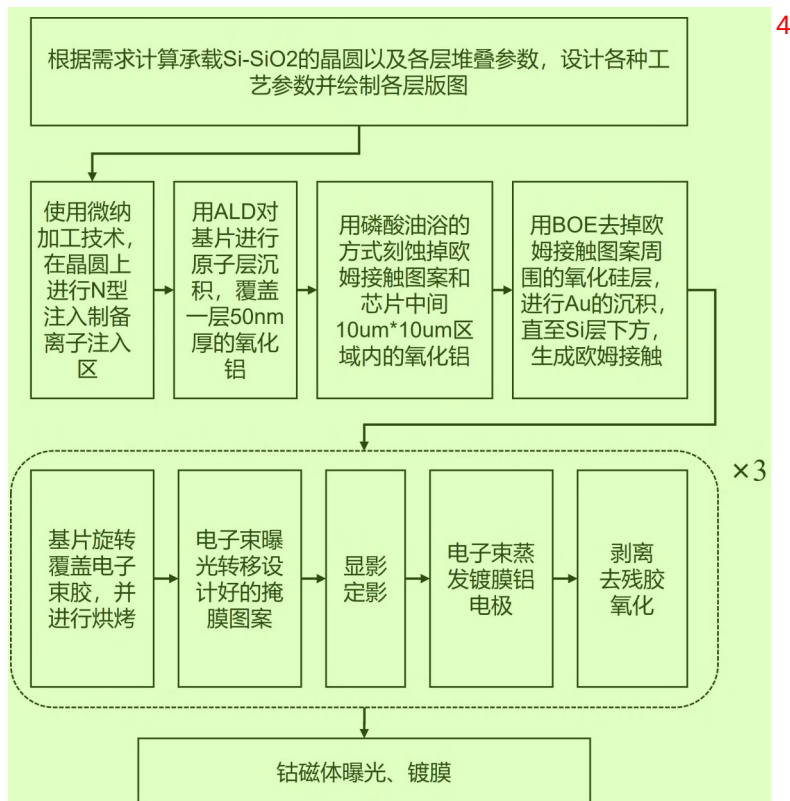
图 3.4 加工流程。对上述过程绘制的流程图
