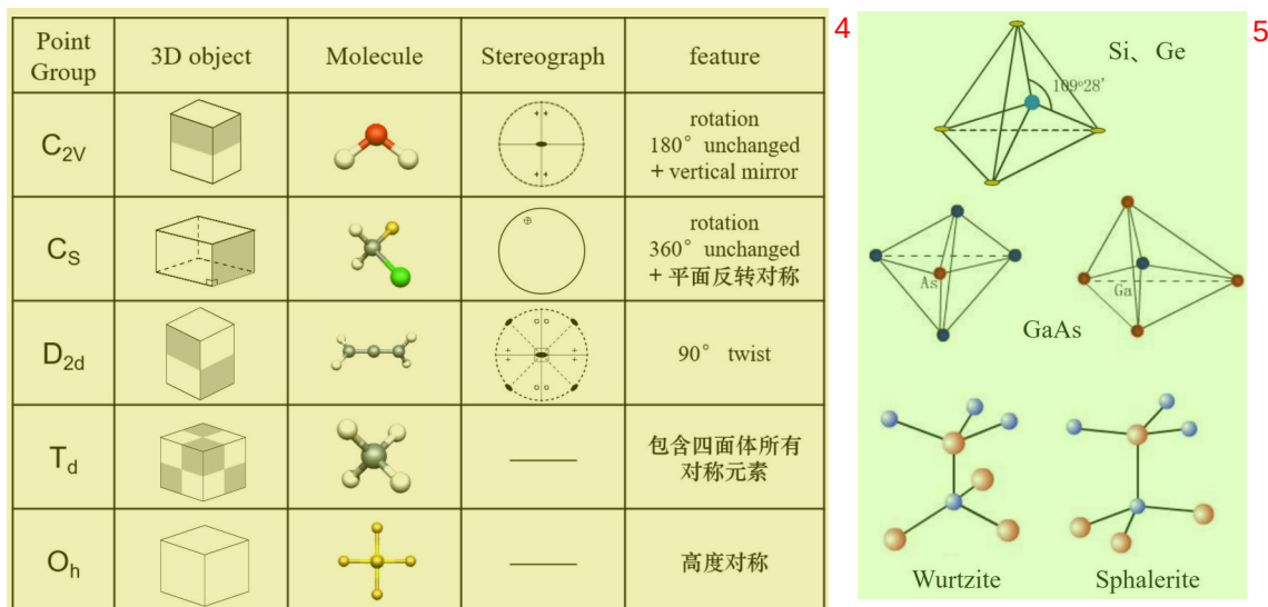
图4.1 点群对称性。左表格中列出了几种常用的点群，我们用三维模型、分子结构、立体图以及特征的方式进行详细说明。右图显示了硅锗以及砷化镓半导体中的晶体结构以及纤锌矿和闪锌矿的结构。
