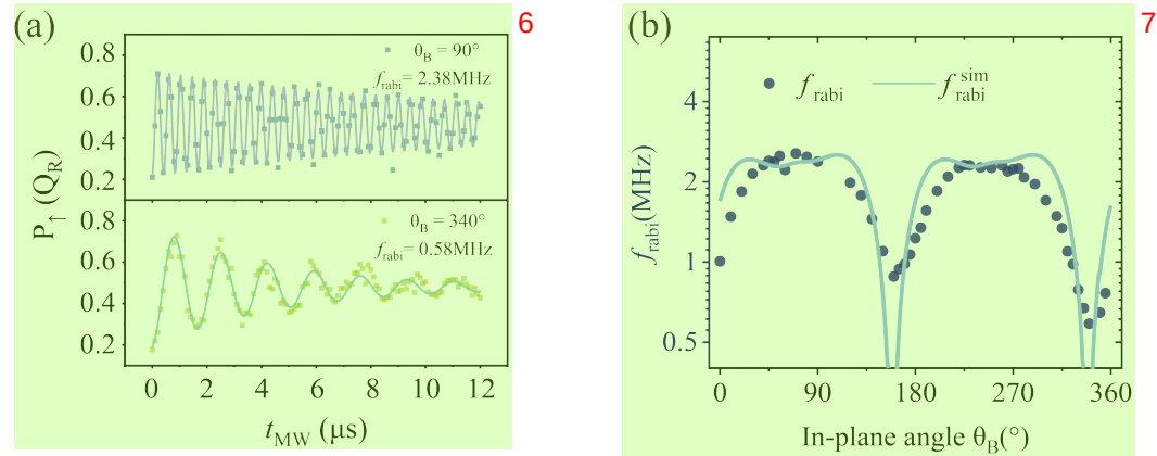
图 4.5 拉比频率的各向异性。(a) 上图： \theta_B = 90^\circ 处的拉比振荡（外部磁场沿 y 轴方向），拉比频率为 f_{rabi} = 2.38(3) MHz。下图： \theta_B = 340^\circ 处的拉比振荡， f_{rabi} = 0.58(6) MHz。拉比频率的最大值和最小值相差约 4.1 倍。(b) 测量的（深蓝色圆圈）和计算的（浅蓝色线）拉比频率 f_{rabi} 是平面磁场角度 \theta_B 的函数。微波频率和功率在整个实验过程中保持不变。图片来源于文献 [174] 。
