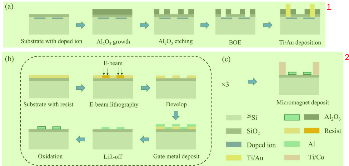
图 3.3 芯片加工流程示意图。(a) 在已经做好离子注入区的基片上进行欧姆接触的制备，并且生长 50 nm 厚的 \text{Al}_2\text{O}_3 作为场氧，中间暴露出的 \text{SiO}_2 作为栅氧。(b) 金属栅极制备的过程，每一层都需要按照这个流程循环一遍，对三层电极各重复一次。(c) 在量子点附近镀微磁体。
