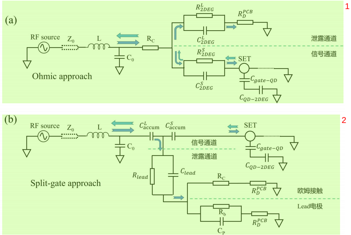
图 6.10 两种不同的适应增强型器件的射频读出的电路方案。(a) 欧姆方法。射频信号从欧姆接触打入，实现的核心是将离子注入区深入量子点中心区域 10\ \mu\text{m} 内以达到尽可能小的 R_c 来抑制耗散，并且与离子注入区搭界到外围大电极区域的电阻 R_{2DEG}^L 要减小需要电极尽可能短，对应电容 C_{2DEG}^L 要抑制可以通过 mesa 刻蚀的方式除掉下方二维电子气。而与离子注入区搭界到内部小电极的电阻 R_{2DEG}^S 尽可能小以保证耗散足够弱，对应的电容 C_{2DEG}^S 也要尽可能小，保证泄露可以抑制。(b) 劈裂栅极方法。射频信号从累积栅极打入，核心是引线栅极与累积栅极之间的重叠面积够小，使得 C_{lead} 可以抑制信号的泄露，而 R_{lead} 的泄露通道的抑制可以通过关闭引线栅极的电压来实现。图中蓝色箭头为入射信号，青色箭头为反射信号。
