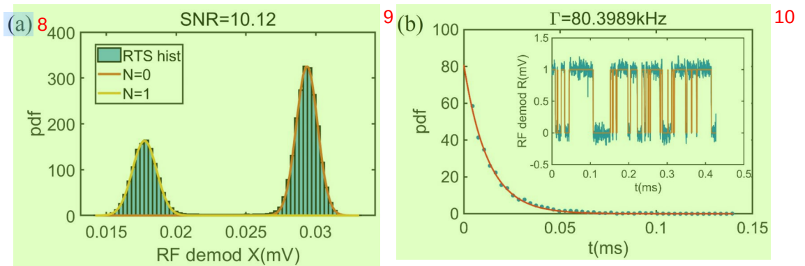
图 6.16 Ge/SiGe 量子点结构中的射频探测结果。(a) 解调反射信号的 X 分量分布，积分时间为 t_{int}=100 ns，信噪比为 10.12，橙色和黄色条包络分别表示在检测到的量子点中电子数为 0 和 1 时，SET 反射的 V_Q 电压分布。(b) 插图中间时间轨迹所获得时间的概率密度，通过射频检测获得的平均 RTS 调谐率高达 80.4 kHz。
