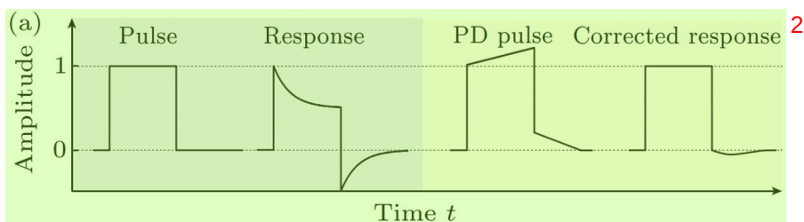
图 5.21 DCZ 门中高频波形的畸变校准。(a) Bias-tee 器内部 RC 滤波线路后的方波脉冲响应示意图。具有线性斜坡上升沿的预失真脉冲可以校正失真。下降沿后的线性斜坡下降脉冲用于将脉冲幅度逐渐减小到零, 并尽可能降低剩余失真的影响 [186] 。
