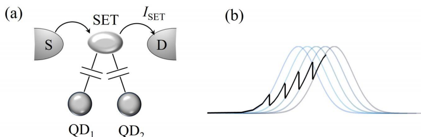
图 1.8 SET 探测原理 (a) 单电子晶体管 (SET) 探测量子点内电子数电路示意图，其中作为 SET 的单量子点通过输运电流的方式与被探测量子点产生电容耦合。(b) 量子点内电子数的变化使得 SET 电流产生偏移，产生锯齿信号，转化为电导信号即为一个信号峰或者谷，图中显示在 \text{QD}_1 中前五个填充电子的探测信号。
