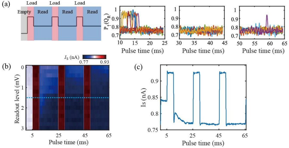
图 2.2 单发读出位置标定。(a) 用于旋转读出的三级脉冲序列。Empty 和 Load 电压水平保持不变，而 Read 级别则从高到低进行扫描，后续跟的加载和读出过程用来进行读出正确与否的判断。(b) SET 的输运电流 I_s ，平均 200 次单发读出的轨迹，作为在读取阶段的电压水平的图像变化。用应用磁场 B=0.7T 采集的数据。(c) 在 (b) 中蓝色切线位置处的电信号，①区域为读取的窗口阶段，在合适的区域中会产生 spin-bump 的信号。②③为判断读取位置合适的监视，如果这两个监视窗口的单发读出高电平比例过高 ( >0.2 )，则说明暗计数太多，需要重新矫正读取位置。
