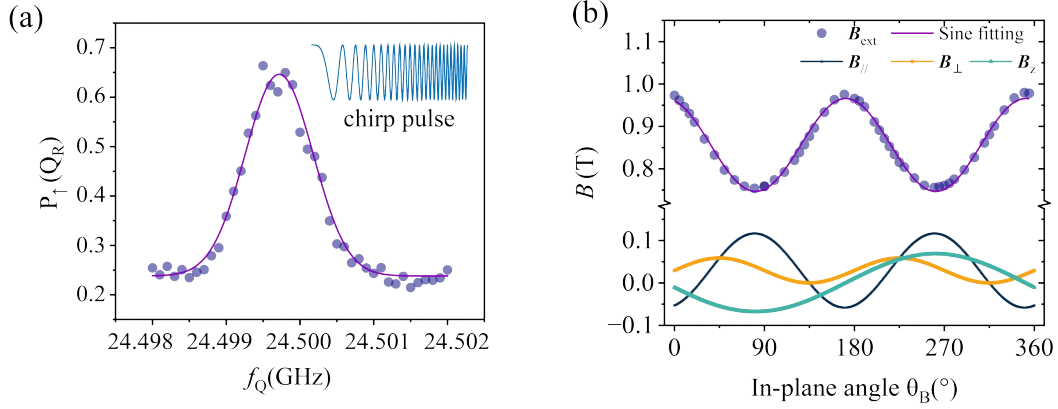
图 4.4 固定拉莫尔频率下的外磁场各向异性。(a) 频率可变的 1MHz 啁啾脉冲微波激励 500 \mu\text{s} 绝热翻转自旋为自旋向上配置。显示了自旋分数与施加的啁啾脉冲的微波频率的关系，其中电子状态初始化为自旋向下，得到的 Q_R 的共振频率为 24.4998 GHz。数据使用高斯峰值函数进行拟合。(b) 测量的谐振磁场强度（紫色圆圈）是平面内磁场角度 \theta_B 的函数，微波频率固定为 24.5 GHz。对数据进行余弦拟合，方程为 A \cos(2\pi\theta_B + \phi) + B ，其中 A 是比例因子，B 是偏移量，相位因子 \phi = 8.3^\circ 可能源于量子点和条形磁铁在空间 y 方向上的不对称性。通过计算微磁体不同磁化方向对应的磁场强度，可以得到分量 B_{//} 、 B_{\perp} 和 B_z 。图片来源于文献 [174] 。
