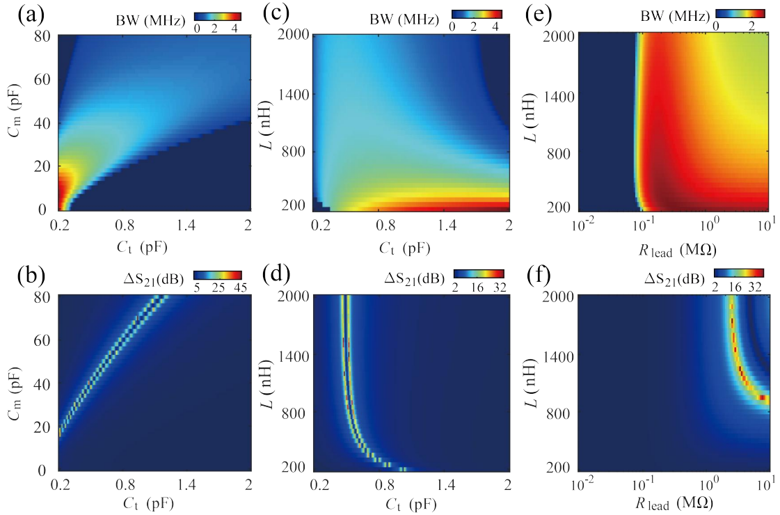
图 6.13 劈裂栅极结构的模拟仿真。假设量子态的变化导致 SET 阻抗在 625 k \Omega 和 500 k \Omega 之间变化，模拟展示了不同参数如何影响测量带宽和信号变化。谐振具有反洛伦兹形状，带宽对应于反射功率的半峰全宽。(a,b) 当电路的阻抗匹配时， C_m 和 C_t 呈正相关。然而， C_t 的增加会降低测量带宽。(c,d) 当 C_m 固定时， C_t 和 L 决定系统的谐振频率。因此， C_t 、 C_m 和 L 需要匹配。(e,f) 当泄漏通道的等效阻抗 R_{lead} 足够大时，系统处于完美的阻抗匹配状态。否则，反射信号的幅度太小而无法读出。模拟的详细参数显示在表格中。
