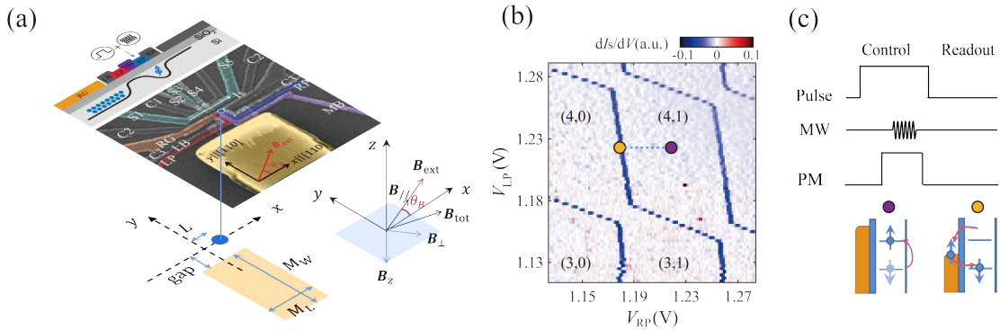
图 4.3 样品以及测试。(a) 实验中测量的器件的示意图和假彩色扫描电子显微镜图像。标出了栅极电极和微磁体。通过 SET 的电流 I_s 用白色箭头表示。外部磁场 B_{\text{ext}} 与 x 轴之间的角度为 \theta_B 。SEM 图像下方是说明微磁体和 Q_R 量子点之间几何关系的示意图，其中对微磁体结构进行了几何建模。插图：不同磁场的笛卡尔坐标和标签。(b) 图中显示了在 LP 和 RP 下方形成的两个量子点的电荷稳定性图。这些点中的电子数表示为 (Q_L, Q_R) 。橙色圆圈表示读出位置，而紫色圆圈表示控制位置。(c) 测量方案的示意图，说明如何通过偏置器将直流电压以及脉冲和微波 (MW) 波形施加到 RP 电极。在控制阶段 (10 ms)，量子比特由微波脉冲驱动，脉冲调制 (PM) 有助于控制微波开关，从而实现更高的微波开关比。在读出阶段 (10 ms)，执行能量选择性读出。如果电子处于自旋向上状态，它可以隧穿到电子储存器中并加载自旋向下的电子，从而完成初始化过程。相反，如果电子处于自旋向下状态，则不会发生跃迁。图片来源于文献 [174] 。
