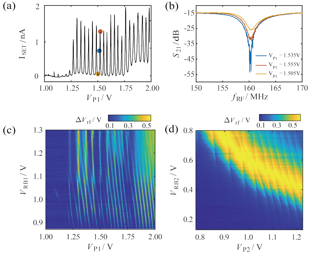
图 6.7 Si-MOS 中的射频探测。(a) SET 直流电流 I_{\text{SET}} 随栅极电压 V_{P1} 变化的示意图。对一个欧姆接触施加 500 \mu\text{V} 的直流偏置电压，另一个欧姆接触通过放大器连接到电压表。同时，被探测的量子点 \text{QD}_2 的两个欧姆接触均接地。SET 的传输电流依赖于柱塞栅极电压 V_{P1} 和偏置电压。(b) 在 (a) 面板中不同颜色的三个圆圈位置观察到反射信号。单电子晶体管的反射系数 S_{21} 随着柱塞栅极电压的变化而变化。当实现阻抗匹配时（用蓝色表示），灵敏度达到最大。 -15 \text{ dB} 的背景反映了从定向耦合器的耦合端口到输入端口的衰减，并考虑了额外的电路衰减。(c) 通过射频反射计测量的 \text{QD}_1 的电荷稳定性图，图中显示了解调后的电压信号。(d) \text{QD}_1 用作检测器来测试 \text{QD}_2 的信号。锯齿状信号表明电子的跃迁。黄色背景表示 (a) 中的库仑峰。图片来源于文献 [200] 。
