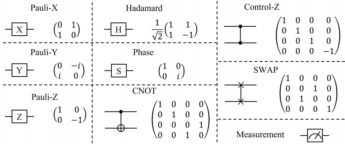
图 2.5 比特门
