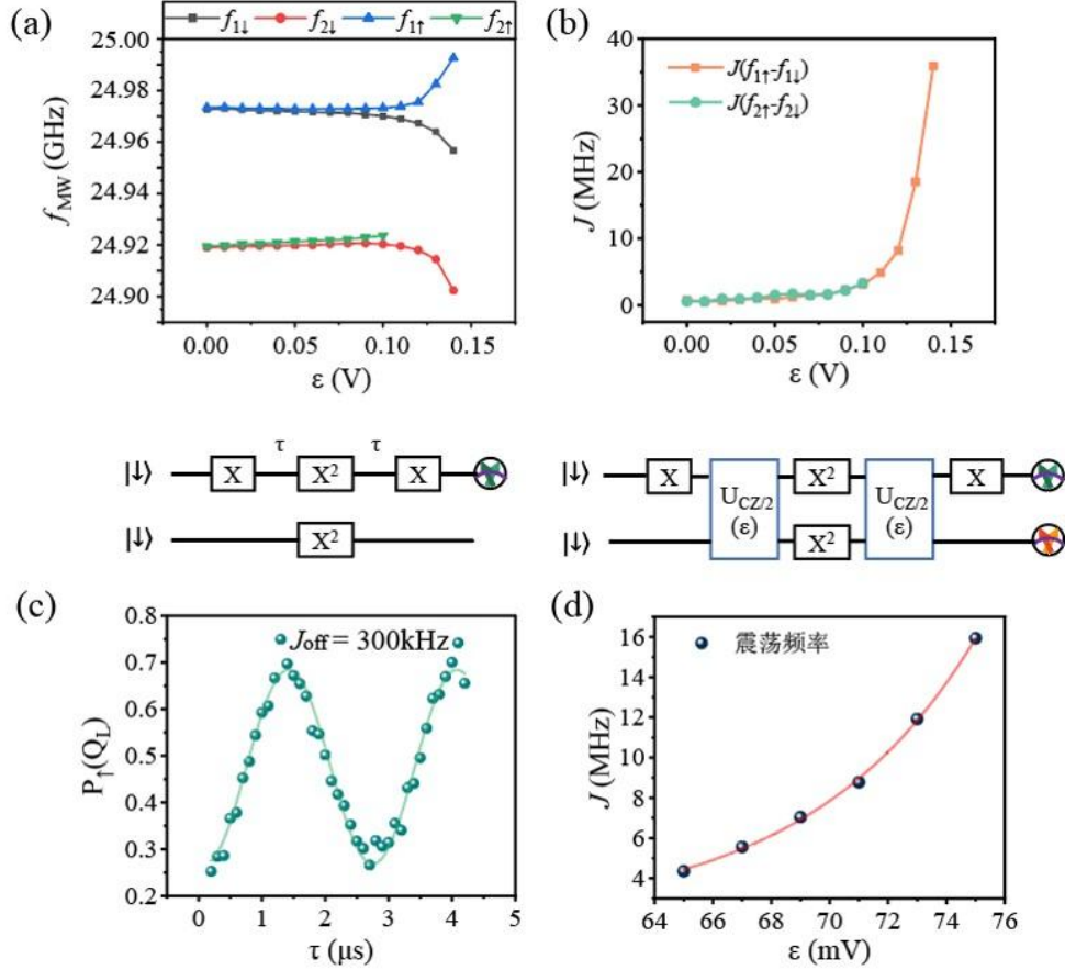
图 5.16 CZ 门操作区域的两比特能谱和交换相互作用的控制。(a) V_{MB} = 1.3 \text{ V} 时的两比特能谱。(b) 提取出的交换相互作用强度随失谐量的变化, 近似于指数上升, 其中 J(\epsilon = 0) < 0.5 \text{ MHz} , 可以保证两个单比特进行同时的高保真度驱动。(c) 使用解耦序列测量 J_{off} 。使用两比特 Hahn echo 序列测量单比特门期间的交换耦合 J_{off} , 该序列可抵消自由演化时间 \tau 期间的 \hat{z} 旋转。使用拟合方程 \sin(2\pi J_{off}\tau) 将自旋向上的概率拟合为自由演化时间 \tau 的函数, 得到的 J_{off} = 300 \text{ kHz} 。(d) 通过设计 DCZ 的线路进行测试, 通过拟合不同失谐 ( \epsilon ) 处的振荡频率, 可以得到 J 随失谐的变化, 其中红色为指数拟合。后续实验中所用到的 J_{on} = 10 \text{ MHz} , 其开关比 J_{on}/J_{off} \sim 30 。
