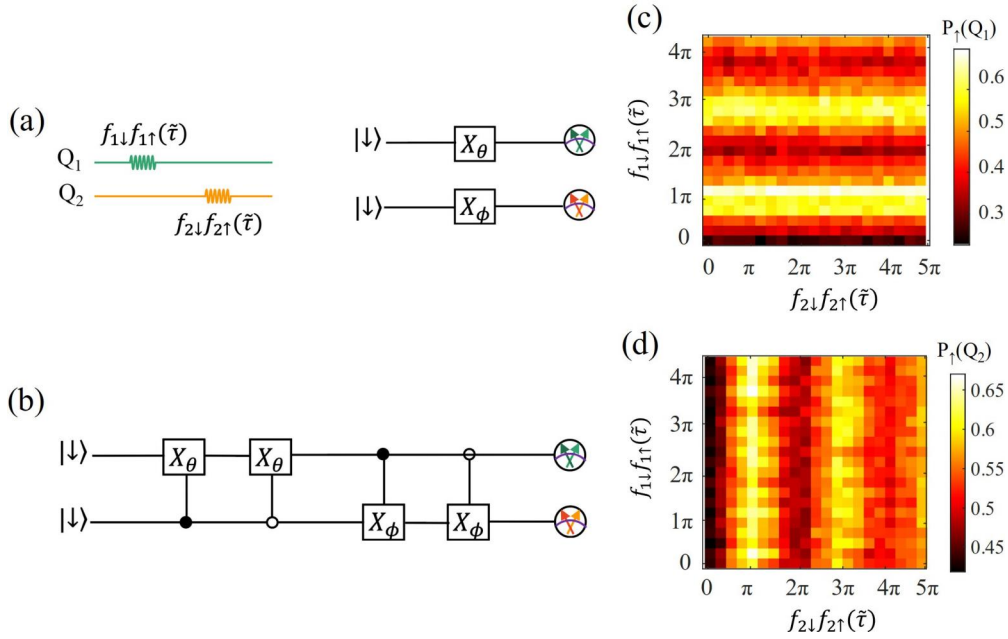
图 5.6 受控旋转合成单比特。(a) 在恒定交换相互作用 J 的存在下，通过在两个条件频率上同时施加微波脉冲，可以实现独立的量子比特控制。第一个脉冲 f_{1\downarrow}f_{1\uparrow}(\tau) 施加到 Q_1 上，第二个脉冲 f_{2\downarrow}f_{2\uparrow}(\tau) 施加到 Q_2 上。右图为两个单比特实现的线路，其中 \theta 为第一个脉冲所对自旋的 Bloch 球上产生的极相位， \phi 为第二个脉冲所对自旋的 Bloch 球上产生的极相位。(b) 两个独立单比特控制的详细控制线路。(c,d) 两个独立量子比特控制的结果，(c) 为 Q_1 比特单独控制的读出，(d) 为 Q_2 比特单独控制的读出。
