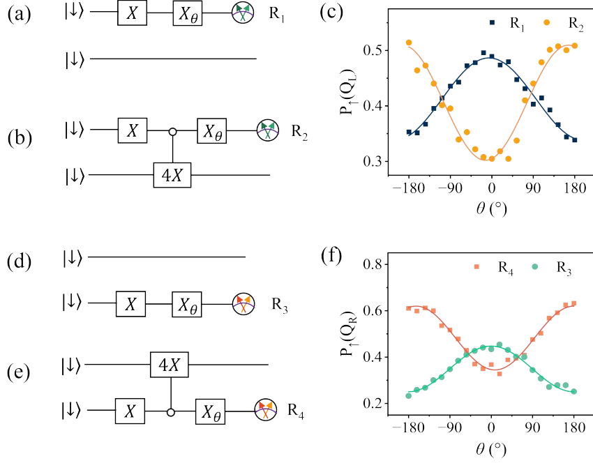
图 5.11 在交换相互作用常开中 CNOT 门的控制比特的额外相位。(a) 对控制比特上进行拉姆齐序列的相位旋转测试， X 表示绕 X 轴旋转 \pi/2 角度，变化第二个 X 门的相位， R_1 为 Q_L 比特的读出结果。(b) 在拉姆齐序列中间插入 ZCROT 2 ，测试其控制比特的相干性以及产生的对应相位， R_2 为 Q_L 比特的读出结果。(c) 控制量子比特在 CROT 操作中获得的相位为 \pi ，即在拉姆齐序列中插入与不插入 ZCROT 2 产生的控制比特相位 out-of-phase。(d,e,f) 交换控制比特与目标比特进行相位旋转测试。
