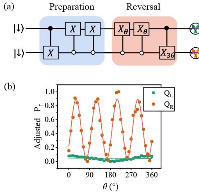
图 5.15 基于 CNOT 门的 Bell 态的相位反转层析。(a) 通过 Preparation 过程制备 Bell 态 \Phi^+ = (|\downarrow\downarrow\rangle + |\uparrow\uparrow\rangle)/\sqrt{2} (蓝色部分)，接下来使用与制备过程相反的操作进行相位反转层析测试。(b) 两个比特的自旋向上概率的振荡作为反转脉冲相位 \theta 的函数，此处我们调整了振荡的振幅来消除态准备和测量 (SPAM) 误差。
