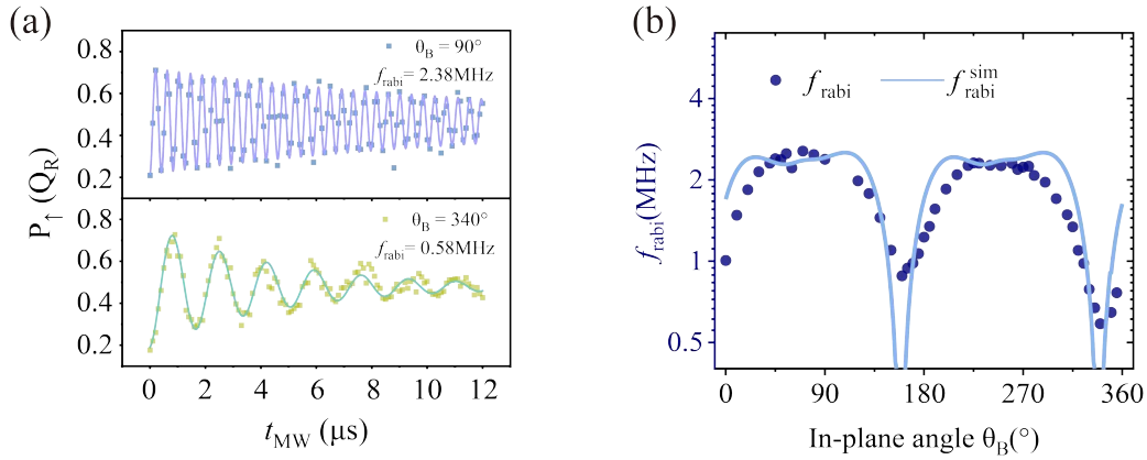
图 4.5 拉比频率的各向异性。(a) 上图： \theta_B = 90^\circ 处的拉比振荡（外部磁场沿 y 轴方向），拉比频率为 f_{rabi} = 2.38(3) MHz。下图： \theta_B = 340^\circ 处的拉比振荡， f_{rabi} = 0.58(6) MHz。拉比频率的最大值和最小值相差约 4.1 倍。(b) 测量的（深蓝色圆圈）和计算的（浅蓝色线）拉比频率 f_{rabi} 是平面磁场角度 \theta_B 的函数。微波频率和功率在整个实验过程中保持不变。图片来源于文献 [174] 。
