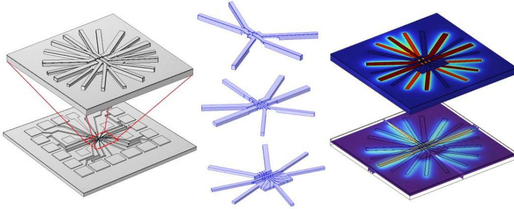
图 3.2 双量子点芯片立体结构图。(left) 芯片不同尺度下的示意图。(middle) 从下往上是第一层的限制栅极(厚度 35 nm), 第二层的引线栅极和柱塞栅极(厚度 55 nm), 第三层的势垒栅极(厚度 75 nm)。(right) 上方基片表面(后续称为表面)上的电场和下方的纯化硅与氧化硅界面(后续称为界面)的电场图, 做了切面。图片由 COMSOL 软件进行电场模拟, 图片仅为示意图, 目的是模拟表面和界面电场, 而电极厚度实际是叠加的, 为了不影响观察, 我们对厚度做了调整, 但仍可以保证表面所受的电压是实验上施加的实际电压。
