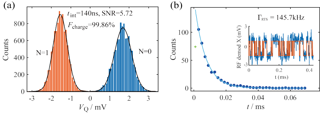
图 6.8 Si-MOS 中的射频高速探测。(a) 解调反射信号的 X 分量在积分时间为 t_{int}=140 ns 下的分布，黑色曲线为两高斯分布之和的拟合结果。通过拟合得到信噪比为 5.72，蓝色和黄色条分别表示在检测到的量子点中电子数为 0 和 1 时，SET 反射的 V_Q 电压分布。(b) 插图中时间轨迹所获得时间的概率密度，通过射频检测获得的平均 RTS 调谐率高达 145.7 kHz。图片来源于文献 [200] 。
