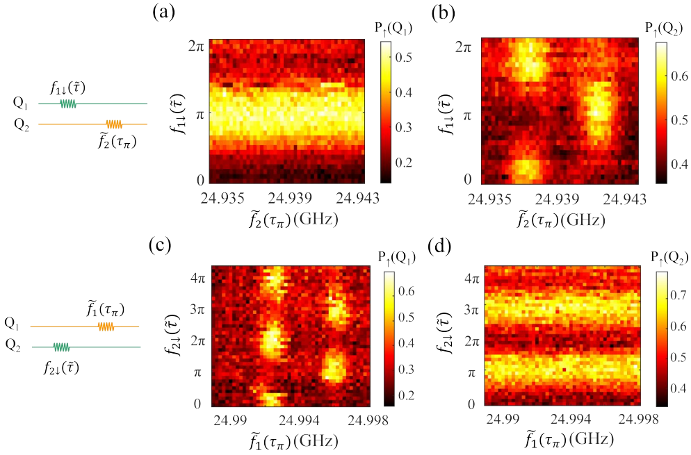
图 5.5 不同控制比特状态下受控比特共振频率的偏移。(a,b) 受控的量子比特旋转是通过在个别共振频率上的脉冲来自然实现的。第一个脉冲 f_{1\downarrow}(\tau) 在 Q_1 上进行 Rabi 旋转，导致 Q_2 的共振频率在 f_{2\downarrow} 和 f_{2\uparrow} 之间振荡，(a) 图为对 Q_1 比特的测试结果，(b) 图为对 Q_2 比特的测试结果。(c,d) Q_2 为控制比特， Q_1 为受控比特的旋转，第一个脉冲 f_{2\downarrow}(\tau) 在 Q_2 上进行 Rabi 旋转，导致 Q_1 的共振频率在 f_{1\downarrow} 和 f_{1\uparrow} 之间振荡。左侧线路为对两个比特施加的波形。
