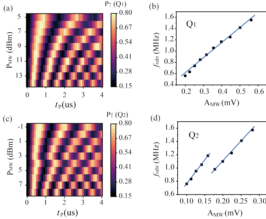
图 5.23 两个单比特门驱动频率随功率变化。(a) Q_L(Q_1) 比特随微波源施加功率的变化。在 14dBm 的微波功率内，我们没看到因为加热效应所导致的拉比频率趋于饱和。(b) 我们将功率的坐标 P_{MW} 转变为幅值 A_{MW} ，变换的公式为 A_{MW}(mV) = (2 \times P(mW) \times 50)^{1/2} 。(c) Q_R(Q_2) 比特随微波源施加功率的变化。(d) Q_R 比特的拉比频率随功率幅值的变化，其中在 3 dBm (0.16 mV) 处有一个断点，我们暂时搞不清这种不连续的来源，我们推测可能是微波源的功率不连续的原因。
