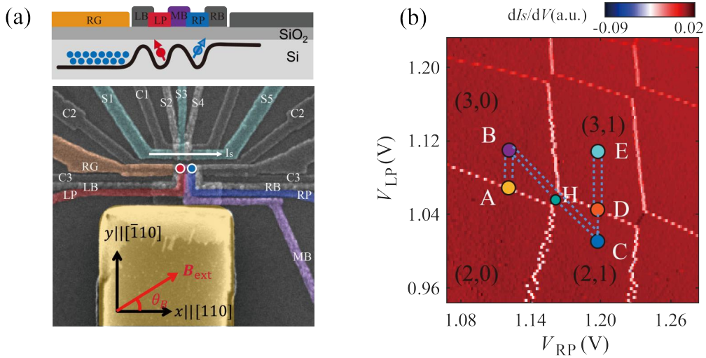
图 5.1 两量子比特器件以及两比特体系的操控波形。(a) 两量子比特设备原理图和假彩色扫描显微镜图像。两个比特分别位于栅极 LP (红色) 和 RP (蓝色) 的下方，它们之间的约束势垒在栅极电极 MB (紫色) 的下方形成，右侧的势垒栅极 RB 和引线栅极都关闭。单电子晶体管位于 S3 下，量子点状态的变化通过影响 SET 的电流 I_S 进行探测。实验上施加的磁场为 B_{\text{ext}}=777 \text{ mT} ， \theta_B = -90^\circ 。(b) 在 LP 和 RP 下形成的两个量子点的电荷稳定性图。这些点中的电子数用 (N_L, N_R) 表示。在 A 点进行 Q_L 比特的初始化，通过 B 点和 C 点的过程将初始化之后的 Q_L 转移到 Q_R 去，然后在 D 点再进行 Q_L 比特的初始化，最后到 E 点，此时在完成初始化的 E 点进行两个量子比特的操控。而读出阶段为初始化阶段的反过程，即在 D 点进行 Q_L 比特的读出，然后通过左右量子点中电子的隧穿之后，将 Q_R 的自旋状态通过 A 点进行读出
