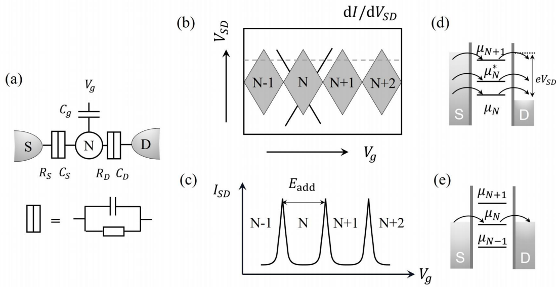
图 1.7 单量子点输运模型 (a) 单量子点的常相互作用模型，栅极与量子点之间的耦合用耦合电容来表示，量子点与源漏之间的隧穿耦合和电容耦合用并联的电容与电阻来表示。(b) 栅极电压与偏压窗口产生的库伦菱形图，菱形内部为库伦阻塞区，外部则有电流，当偏压窗口足够大时，会看到激发态 \mu_N^* 的能谱，继续增大到增加能 E_{add} 会产生双电子隧穿。(c) 零偏置窗口时，运输电流表现为一个个分离的库伦峰，即库伦振荡。(d) 大偏置窗口下多电子隧穿的能级。(e) 小偏置窗口下单电子隧穿的能级。
