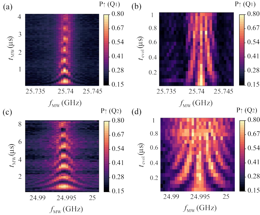
图 5.24 两个单比特的 chevron 图。(a) Q_L(Q_1) 量子比特自旋向上的概率 P_{\uparrow}(Q_1) 绘制为微波频率 f_{MW} 和驱动时间 t_{MW} 的函数，显示相干拉比振荡。(b) Q_L 比特在拉姆齐序列下测试的结果，横轴为微波频率，纵轴 t_{evol} 表示两个 \pi/2 之间的自由演化时间。(c) Q_R(Q_2) 量子比特的 Rabi-chevron。(d) Q_R(Q_2) 量子比特的 Ramsey-chevron。
