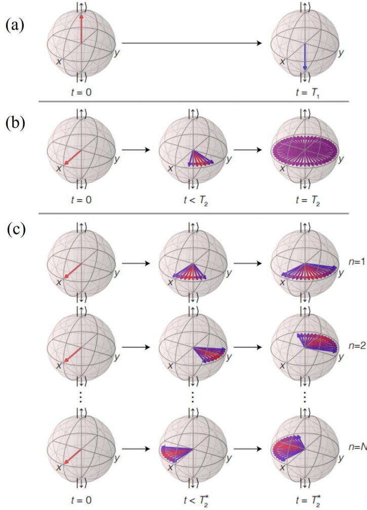
图 2.4 弛豫与退相干。(a) 量子比特激发态弛豫到基态，具有特征时间尺度 T_1 。(b) 自旋去相，初始自旋沿 x 轴，在时间 T_2 后，自旋完全失去了相位相干性，有任意的相位角 \phi 。(c) 自由演化时间 T_2^* 对应于自旋系综。这是 N 次单发测量下退相位的平均结果，由系综所经历的涨落引起。
