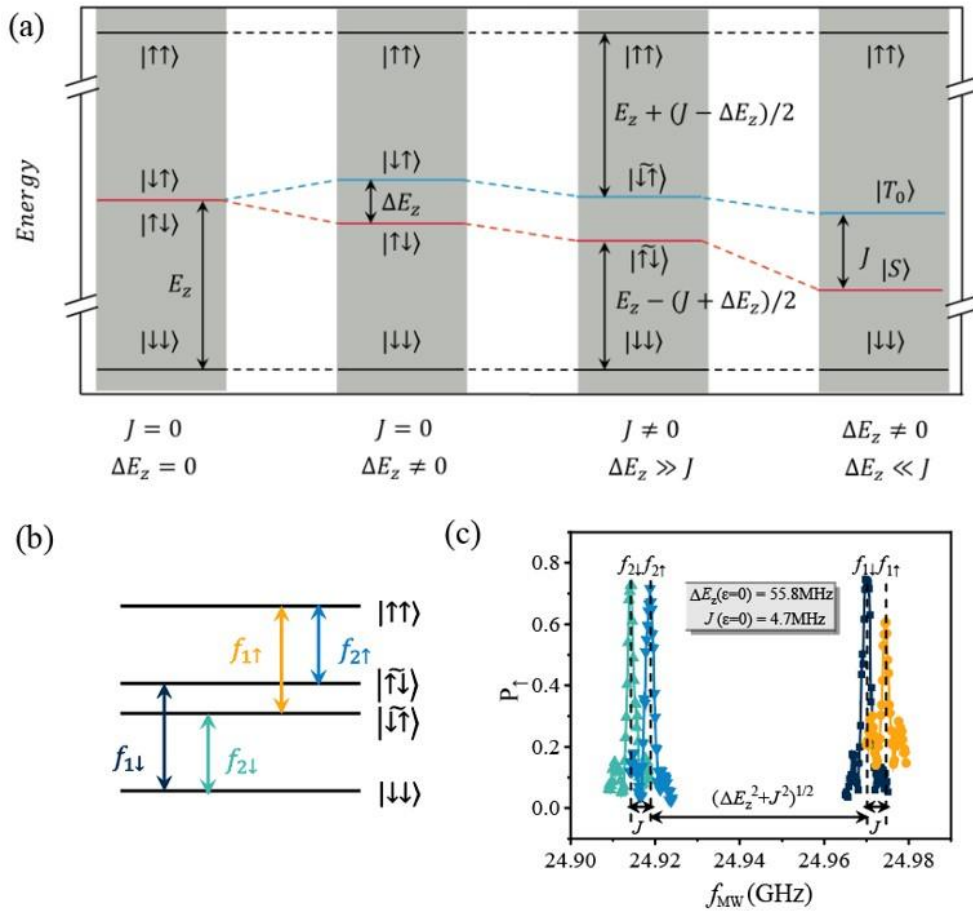
图 5.3 两比特体系的能谱。(a) 随着塞曼劈裂能级差大小和量子点间交换耦合相互作用的变化，两比特体系的本征能级的演化过程。(b) CROT 门操作所参考的能谱。(c) 两量子比特系统的 ESR 谱。我们在 |\downarrow\downarrow\rangle 、 |\downarrow\uparrow\rangle 或 |\uparrow\downarrow\rangle 中制备了 |Q_1, Q_2\rangle ，并测量了 Q_1 和 Q_2 的自旋上升概率作为应用微波频率的函数。由于有限交换耦合 J 和塞曼的能量差 \Delta E_z ，出现了四个不同的 ESR 峰。每个共振峰代表目标量子比特的状态（CROT 信号）的旋转。能级图将每个峰映射到一对双量子比特特征态之间的相应跃迁。
