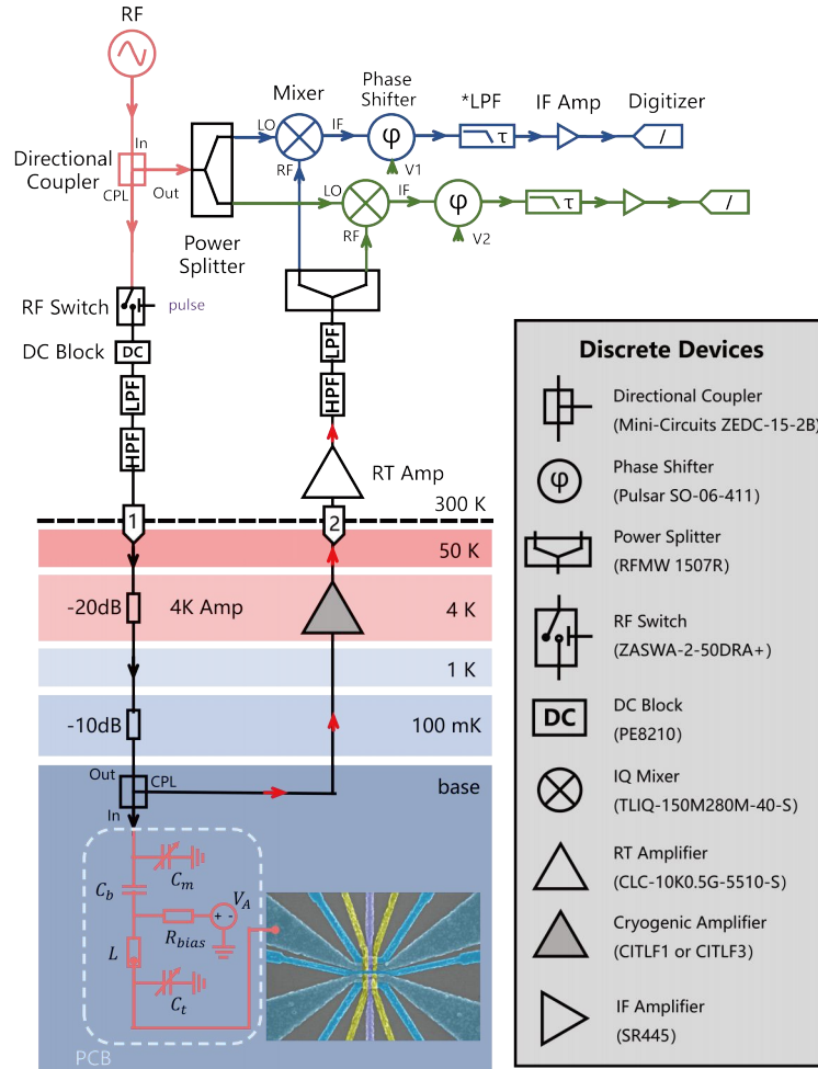
图 6.9 射频测量装置的示意图。一个栅极定义的单量子点耦合到包含电感 L (860 nH)、可变电容 C_t 和 C_m 以及固定电容 C_b (100 nF) 的阻抗匹配网络。载波频率设定为 160.1 MHz。为了探测匹配网络，射频信号在通过 30 dB 衰减器和定向耦合器后注入端口 1。信号在反射和放大后到达端口 2。反射信号在室温下通过与本地振荡器混合进行解调。通过改变 V_1 和 V_2 以调整移相器的相位，可以通过数字化仪检测信号的不同正交分量。射频开关的目的是在除读出阶段外的其他阶段保持静默。偏置电阻 R_{bias} 允许我们测量器件的直流传输电流。灰色框中是示意图中使用的器件类型。
