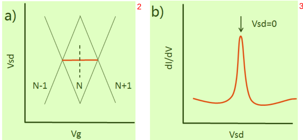
图 5.2 (a) 是一个典型的库伦阻塞。如果出现 Kondo 效应，那么我们能在红线所 4 表示的位置上观察到电导不为 0 的现象。虚线是沿着源漏偏压 V_{sd} 方向 扫描，可以绘制出如 (b) 的图。(b) 上的中央电导峰，一般认为是 Kondo 效应的基本特征。
