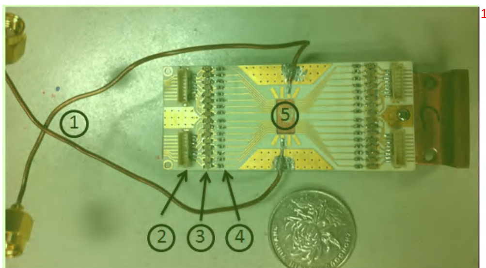
图 2.12 自制 PCB 板载滤波 chip-carrier。1 是软质高频线及接口 2 是普通直流控制测量线路 (lakeshore SS1) 插头 3 是 RC 贴片滤波器 4 铁氧体磁珠滤波器 5 是样品放置的位置。
