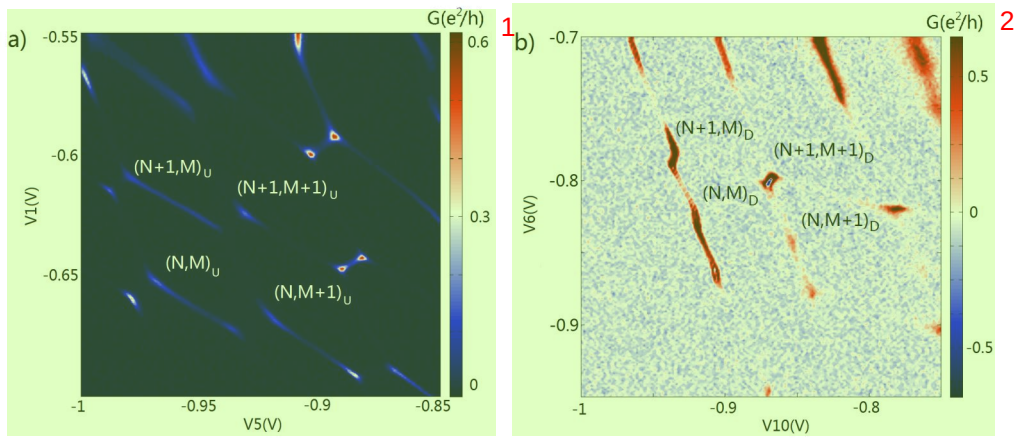
图 5.6 (a) 上面的双量子点，四个不同的电荷态 (N, M)_U , (N+1, M)_U , (N, M+1)_U , (N+1, M+1)_U 。(b) 下面的双量子点，四个不同的电荷态 (N, M)_D , (N+1, M)_D , (N, M+1)_D , (N+1, M+1)_D 。
