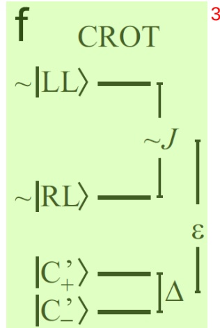
图 4.2 形成 CROT 门时，各个态形成的能谱。图片引自 [87]
