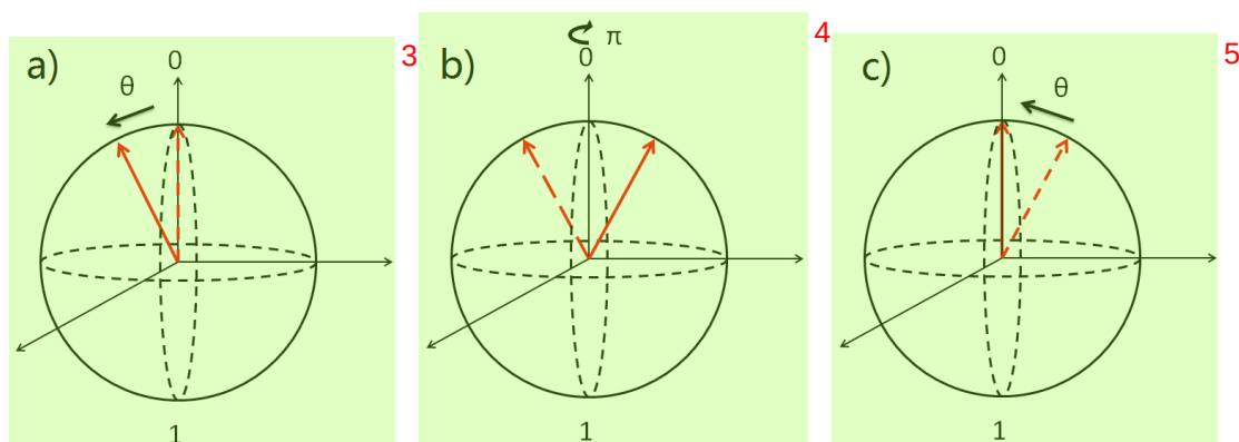
图 1.10 原本在 T = 0 时刻处在 0 位置的 qubit, 收到外界影响, 可能在 T = T_0 时间内沿 x 轴转动了一定角度 \theta , 如果我们对 qubit 做一个操作, 目标是使得 qubit 快速地沿 z 轴转动 \pi , 则它在下一个 T = T_0 时间内继续转动 \theta , 则又重新回到 0。红色虚线和实线分别代表一段时间内起始态和终了态。
