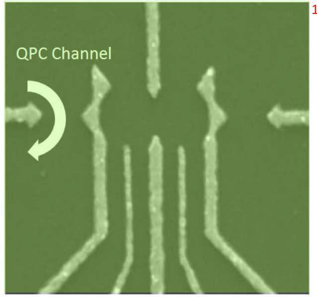
图 1.9 QPC 通道示意图，白色箭头标示了 QPC 电流 2
