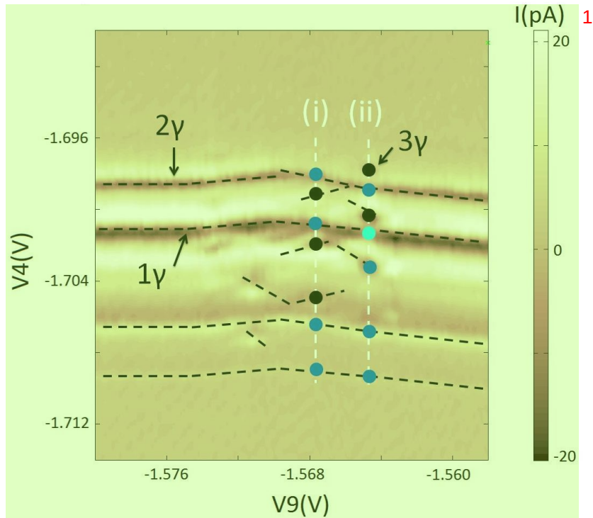
图 4.6 (施加了频率 20GHz, 功率 -10dbm 连续正弦信号, 量子点中呈现出许多微波光子辅助隧穿。为了清晰起见, 我们用黑色虚线来表示。白色虚线 (i) 和 (ii) 分别对应于图 (4.7 a) 和 (4.7 b) 的情况。不同颜色的点对应着不同的跃迁终态
