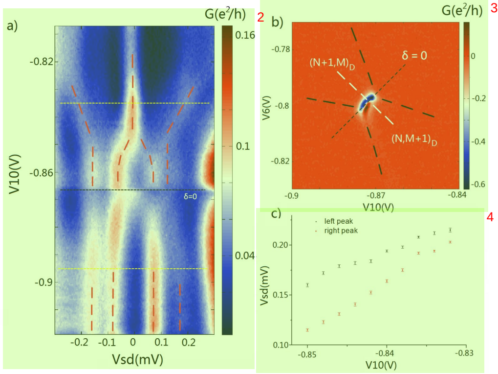
图 5.9 (a) 显示了当沿着 (b) 中白色虚线所示的路径，扫描下面双量子点的相应电压时，上面双量子点源漏通道的微分电导 dI/dV 的变化情况。Kondo 峰用红色虚线标记出来。从 V10=-0.82V 到 V10=-0.85V 阶段，这里出现了中央峰，连同其他两个不断靠拢的侧峰。在 V10=-0.866 的位置，这里出现了一个跳跃 (位置用黑色虚线标记)，对着下面双量子点出现了一个电子态的变化 [从 (N+1, M)_D 到 (N, M+1)_D ]。 (b) 显示了 (N, M)_D 区域附近的细节。黑色虚线标记了库伦峰的位置；较细的虚线标记了失谐量 \delta = 0 的位置；白色虚线标记了扫描路径，从 (V6=-0.855V, V10=-0.807V) 到 (V6=-0.752V, V10=-0.919V) 。 (c) 展示了左右两峰到 V=0 位置的绝对距离。可以发现，随着 V10 从 -0.83V 变化到 -0.85V ，其差距越来越大。
