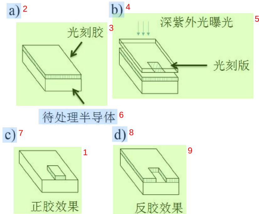
图 2.1 如图 (a) 和 (b)，光刻胶覆盖在待处理半导体表面，画好图案的光刻板覆盖在胶上。(b) 图中是一块反版，有图案处不透光。(c) 和 (d) 分别显示了曝光完成，并显影后显示出的图案。(c) 是正胶的效果，图案处留下了光刻胶，其余被清洗掉；(d) 是反胶效果，图案处被清洗掉，其余部分留下光刻胶。
