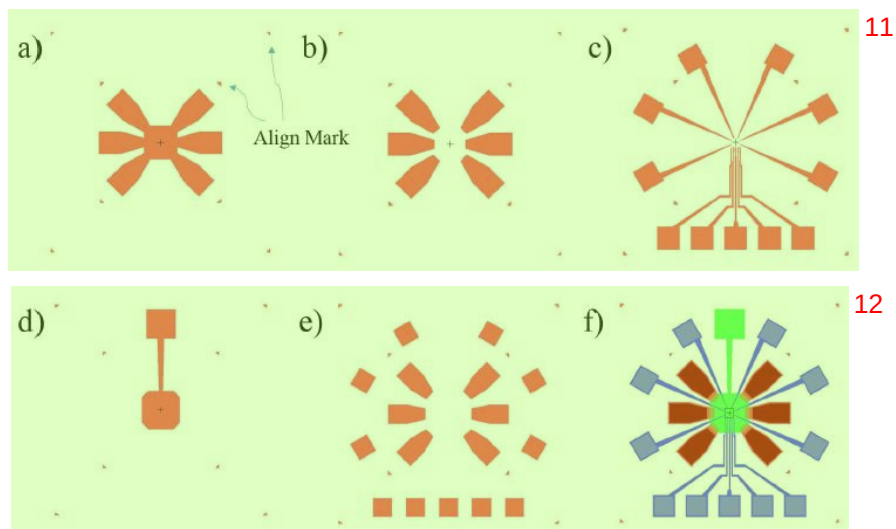
图 2.2 这是一组用 Altium 软件绘制的光刻板 CAD 图样。(a) mesa; 其中虚线箭头处标示了对准位置。(b) 欧姆接触电极; (c) 表面电极; (d) top gate, 在有些样品，比如非掺杂的 GaAs 晶圆上需要使用; (e) 统称为 pad 的大电极; (f) 总体效果。
