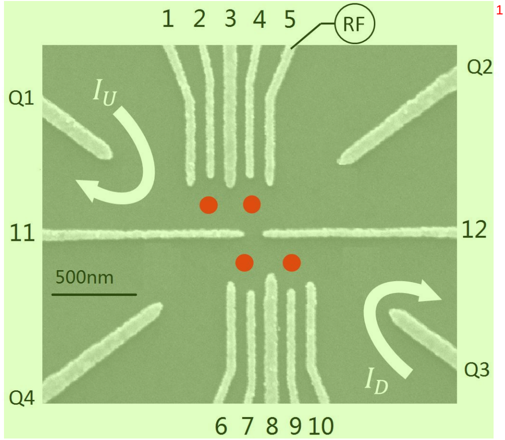
图 4.1 (a)Ti/Au 电极 1-12 定义了一个典型的四量子点结构。在上下两组量子点共用横向电极 11 和 12 的基础上，电极 1-5 定义了一个典型的双量子点；电极 6-10 同样定义了一个典型的双量子点。电极 Q1-Q4 是四个 QPC 电极，用来形成四个 QPC 测量通道。白色箭头表示了测量电流流过的方向。红色的四个圆点表示了四个量子点的假想位置
