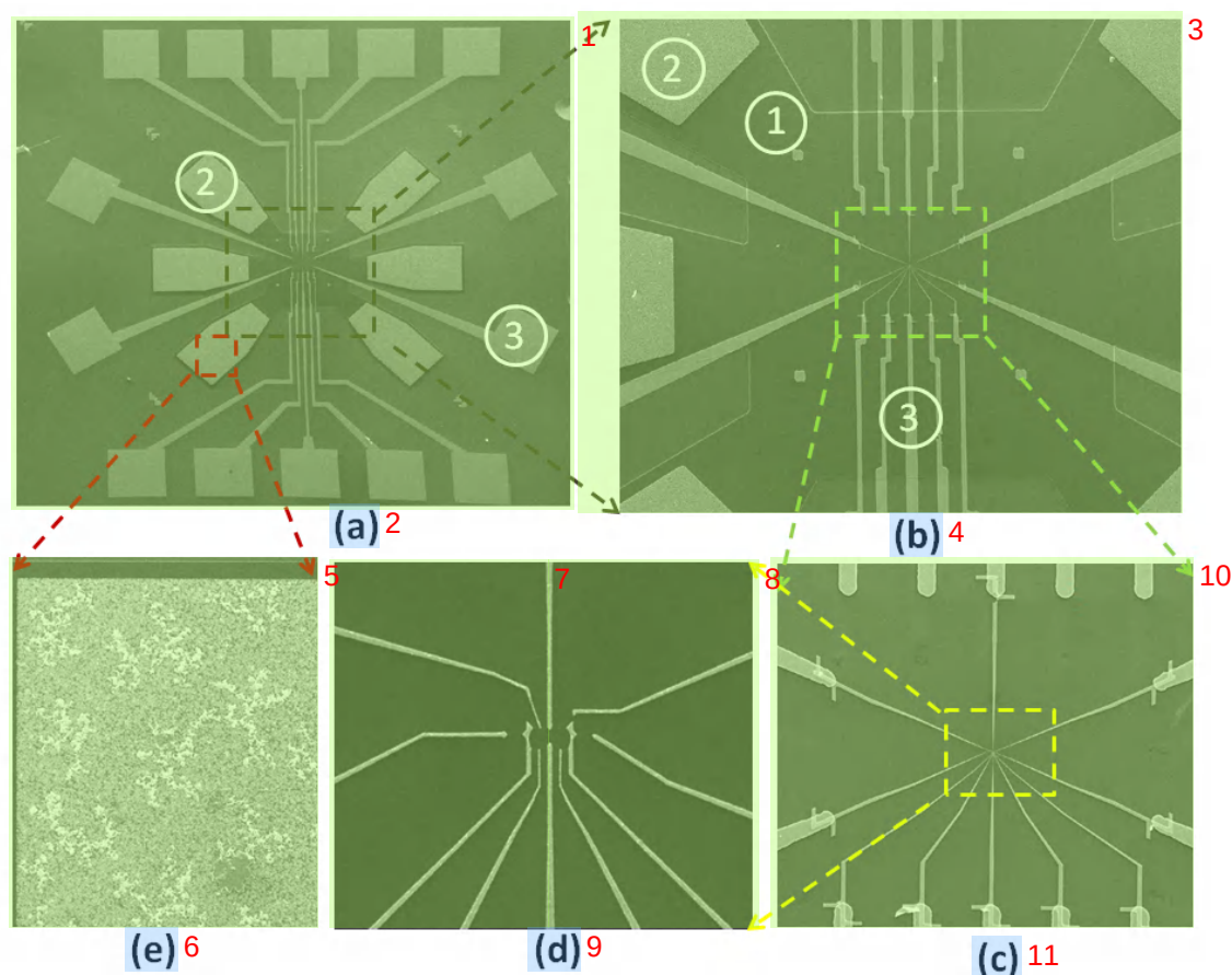
图 2.7 (a) 是整体效果图 (b) 是局部放大图，图中绿色方框外围四个小方形位置，就是电子束曝光对准标记 (c) 是电子束曝光部分图 (d) 是双量子点核心区域电极，最细处大约在 10nm。电子束曝光电极和光刻曝光电极交接处，存在一些 Z 字形图样，目的是防止对准时出现偏差，增加二者接触的可能性 (e) 是欧姆接触电极退货后表面形状，坑洼不平。圆圈内的 1,2,3，分别对应着 Mesa，欧姆接触电极和表面电极。
