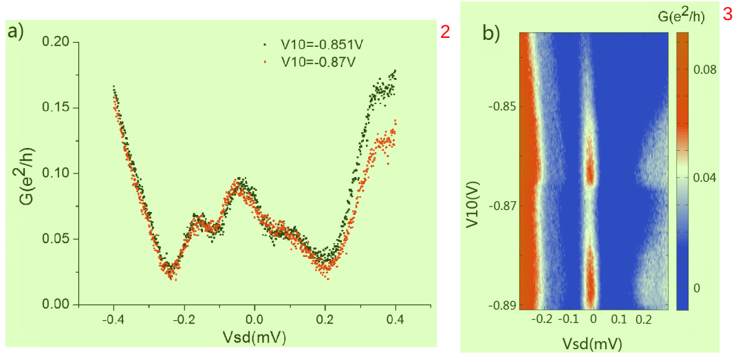
图 5.11 (a) 比较了图 (5.9 a) 中 V10=-0.851 和 V10=-0.87V 两处的曲线，除了最右边的本底以外，几乎完全一致。(b) 将 V11 和 V12 从 -0.8V 改变到 -0.8003V ，观察上面双量子点微分电导 dI/dV 随着 V10(V6) 的变化。中央峰在 V10=-0.866V 处发生了一个明显的跳跃。这里我们可以用下面的双量子点作为控制比特，来实现一个 Kondo 效应开关。
