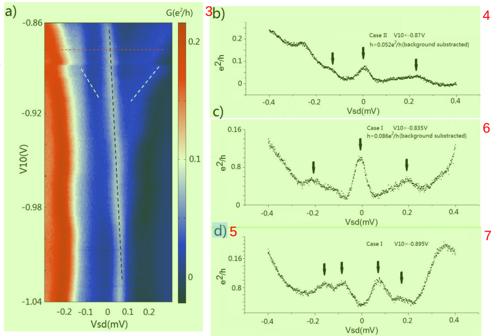
图 5.10 为了证明我们在图 (5.9 a)(情况 1) 中观察的现象是来自于上下两组双量子点之间的耦合，我们将下面双量子点的两个 plunge gate V_7 和 V_9 从 -0.4V 变化到 0V(情况 2)。同时扫描 V_6 和 V_{10} ，读出上面双量子点的微分电导 dI/dV 。(a) 中， V_{10}=-0.875 处的跳跃是一个偶然的随机跳跃，量子点系统中偶尔会出现这种整体的突然移动，可以被忽略。白色虚线标记了中央峰两侧相互靠近的两个“隆起”。它们从 V_{10}=-0.86 V 到 V_{10}=-0.93 V 的区域，依然保持了靠拢的趋势。之后随着 V_{10} 向负方向的增加而消失。(b) 是从 (a) 中抽取的曲线，位置在 ( V_{10}=-0.87 V)，(c) 和 (d) 是从图 (5.9 a) 中抽取的曲线，位置在 ( V_{10}=-0.835 V, -0.895V)。(b) 中，中央峰的高度明显降低了，约在 0.052e^2/h ，而且整个 V_{10} 范围内变化不大。(c) 中的中央峰高度则有 0.086e^2/h 。(d) 图清晰地展示了一个四峰结构 (情况 1)。
