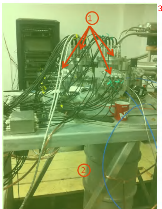
图 2.9 照片中是我们购买的 Triton 300 型稀释制冷实际改装完成照片。1 是我们自制的真空密封法兰，使用真空 BNC 接头与外界相连。2 是稀释制冷机杜瓦。
