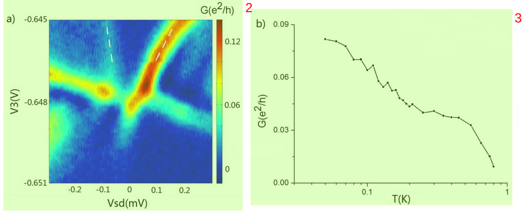
图 5.8 (a) 显示了微分电导 dI/dV 随着上面双量子点中间电极 V_3 的变化关系。 V_3 的调节范围从 -0.651V 到 -0.645V。在 V_3=-0.647V 处，出现了一个单峰到双峰的劈裂现象 (白色虚线标示，此时 V_6=-0.774V ， V_{10}=-0.885V ，其余见正文)。(b) 显示了 Kondo 中央峰随着温度的依赖关系 (本底已扣除)，我们推测 Kondo 温度大约在 900mK
