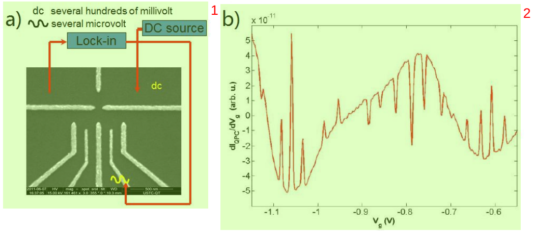
图 3.5 (a) 样品的基本电路图，QPC modulation measurement (b) 展示了实际的测量结果。
