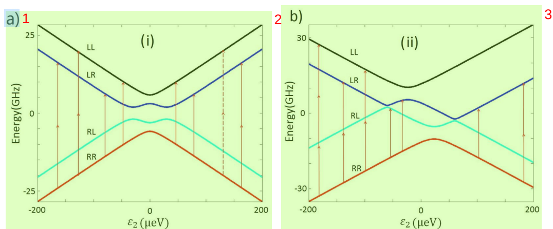
图 4.7 (a) 和 (b) 是四量子点 Hamiltonian 能级的数值模拟结果。红色箭头表示了微波光子辅助下的跃迁过程。红色虚线箭头表示这里应该有一个跃迁，但没有在实验上观察到
