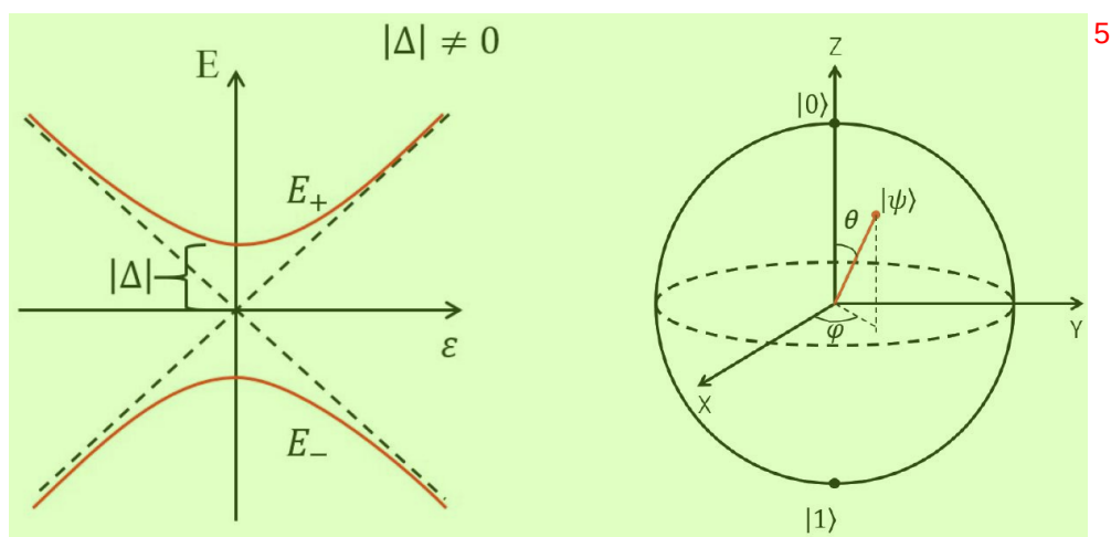
图 1.6 (a) 一个典型的二能级体系的能级图，横轴为失谐量 \epsilon 。 \epsilon = 0 时，上下两个电极之间的差值为 2\Delta 。(b) Bloch 球上的每一点都代表了一个态
