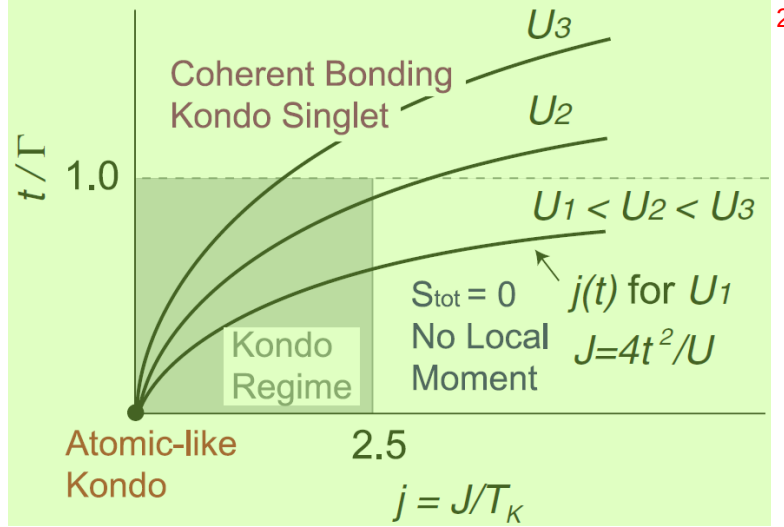
图 5.4 串联双量子点 2-IK 相图。这里， j = J/T_K = 4t^2/U ， J 是两个量子点之间等效反铁磁耦合能， t 是两个量子点之间的隧穿耦合能。 \Gamma 是量子点到源漏电极的隧穿速率。 T_K 是 Kondo 温度。这里假定了整个系统是完全对称的，不再区分左右不同。横纵坐标并不独立。电子充电能 U 不同的条件下，单独调节 t ，在像图上走过的轨迹也不一样。相图的左下角， t 很小时，系统近似为两个独立的 Kondo 过程，称为 atomic Kondo state； t > \Gamma 时，系统的基态是 coherent bonding Kondo 态；当 t < \Gamma 时，如果 j > 2.5 ，则系统的基态是两个自旋杂质绑定成的 Singlet 态。图片摘自 [99]。
