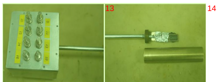
图 2.8 (a) 和 (b) 是我们自制的测量杆。(c) 是我们购买的初测用的 chip-carrier(也就是 plug)。样品用银胶粘在中央，并用 bonding machine 完成 bonding 操作。
