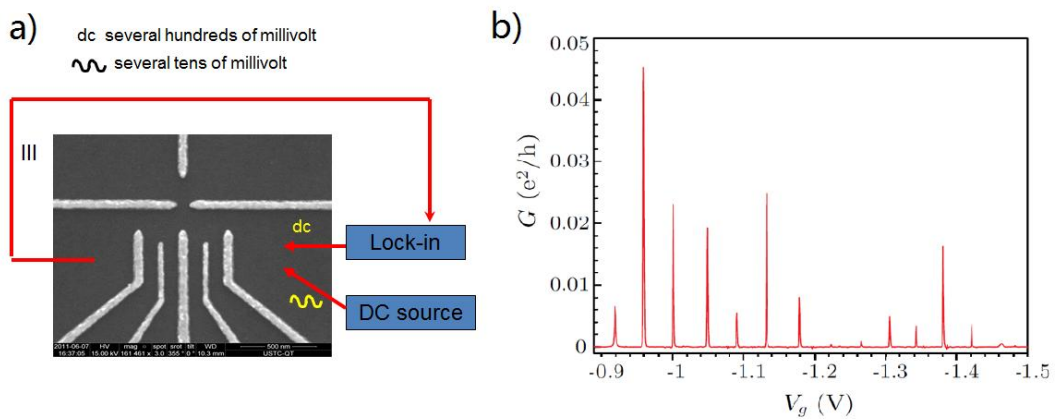
图 3.3 (a) 样品的基本电路图，QD transport measurement (b) 展示了实际的测量结果。
