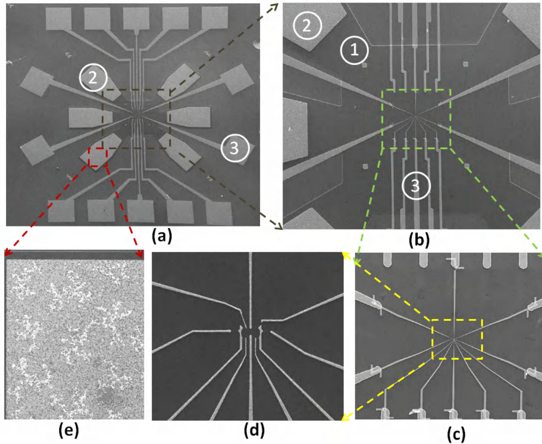
图 2.7 (a) 是整体效果图 (b) 是局部放大图，图中绿色方框外围四个小方形位置，就是电子束曝光对准标记 (c) 是电子束曝光部分图 (d) 是双量子点核心区域电极，最细处大约在 10nm。电子束曝光电极和光刻曝光电极交接处，存在一些 Z 字形图样，目的是防止对准时出现偏差，增加二者接触的可能性 (e) 是欧姆接触电极退货后表面形状，坑洼不平。圆圈内的 1,2,3，分别对应着 Mesa，欧姆接触电极和表面电极。
