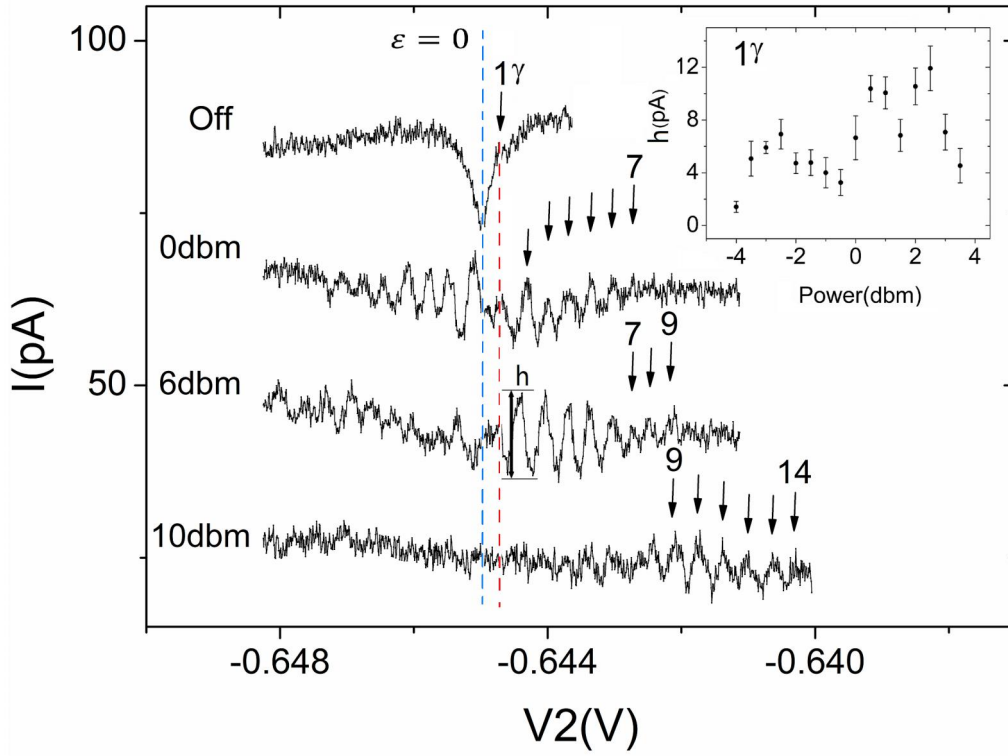
图 3.12 此图展示了一系列不同微波功率下的微分电流 dI/dV 曲线，固定频率在 15GHz。为了提高信噪比，每个点采样 10 次求平均值。蓝色虚线表示了 \epsilon = 0 的位置。曲线表示的功率分别为 off, 0dbm, 6dbm 和 10dbm(从上到下)，曲线在纵轴上连续地移动了 20pA，以便能画在同一张图上。两条平行的短线中间所夹的距离，定义为峰高 h 。Inset 显示了 1\gamma 峰(用红色的虚线标示)的高度在 3pA 和 12pA 之间振荡，大约在 -4dbm, 0dbm, 4dbm 附近达到最小值。 2\gamma - 6\gamma 表现出了同样的行为。在微波功率提高到 10dbm 以后， 7\gamma 直至 14\gamma 过程逐渐展现出来。
