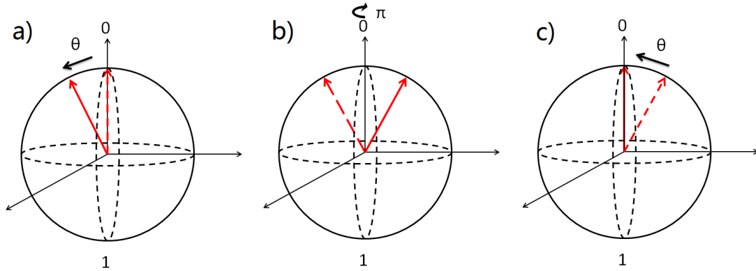
图 1.10 原本在 T = 0 时刻处在 0 位置的 qubit, 收到外界影响, 可能在 T = T_0 时间内沿 x 轴转动了一定角度 \theta , 如果我们对 qubit 做一个操作, 目标是使得 qubit 快速地沿 z 轴转动 \pi , 则它在下一个 T = T_0 时间内继续转动 \theta , 则又重新回到 0。红色虚线和实线分别代表一段时间内起始态和终止态。
