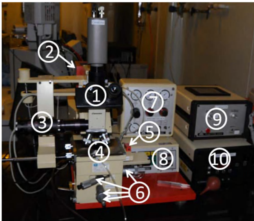
图 2.3 光刻机 KarlSuss MJB-3。各组件为:1 光学显微镜 2 汞灯光源（曝光光源） 3 光学显微镜光源 4 光刻板台，放置光刻版 5 样品台，防止样品 6 样品台控制杆，用于控制样品的位置，以便和光刻版上图案对齐 7 气路控制器 8 光刻控制器，开启曝光，控制曝光时间 9 显微镜光源控制器 10 汞灯光源控制器
