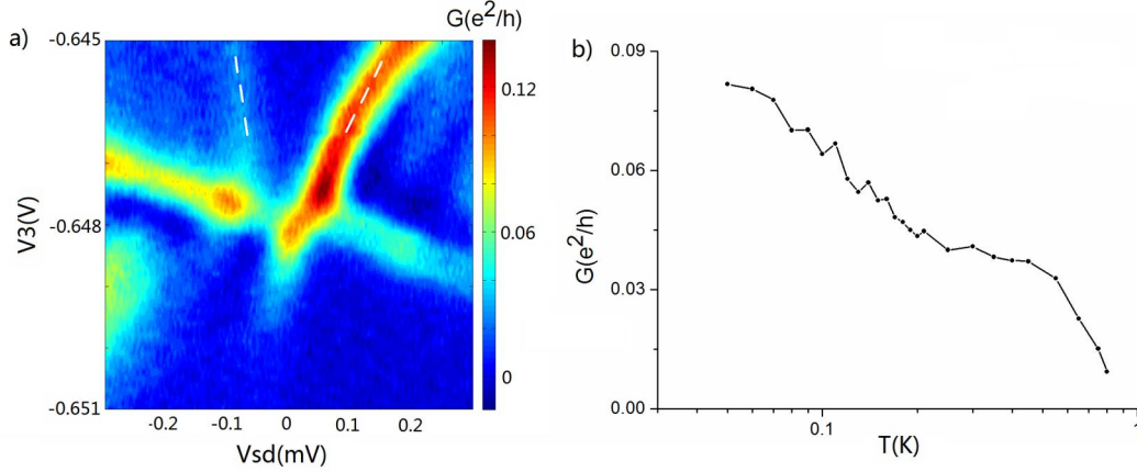
图 5.8 (a) 显示了微分电导 dI/dV 随着上面双量子点中间电极 V3 的变化关系。 V3 的调节范围从 -0.651V 到 -0.645V。在 V3=-0.647V 处，出现了一个单峰到双峰的劈裂现象 (白色虚线标示，此时 V6=-0.774V ， V10=-0.885V ，其余见正文)。(b) 显示了 Kondo 中央峰随着温度的依赖关系 (本底已扣除)，我们推测 Kondo 温度大约在 900mK
