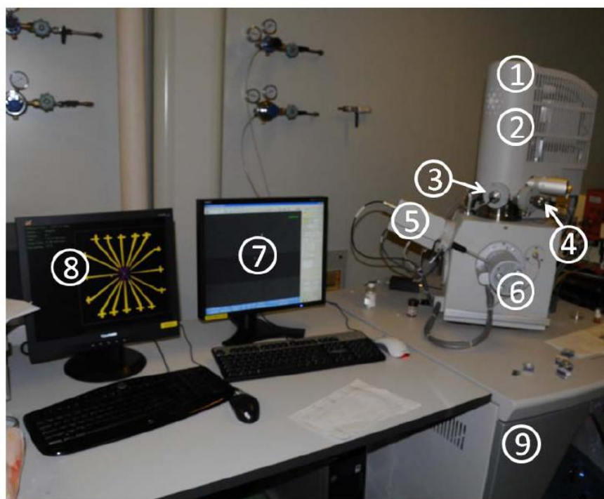
图 2.4 扫描电子显微镜 (SEM) 和电子束直写 (EBL) 装置。各组件为:1 高压电子束发射源 2 各级电学透镜 3 扫描电子显微镜光阑 (光阑的开关构成曝光图样) 4 纳米图形产生系统 (Nanometer Pattern Generation System,NPGS) 控制系统, 用于产生光阑图形 5CCD 探测器 6 样品位置调节装置 (手动在 x,y,z 三个方向调节) 7SEM 控制主机 8NPGS 控制主机 9SEM 机柜
