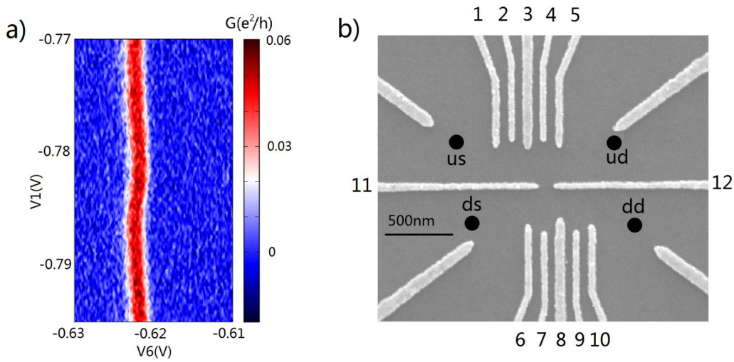
图 5.5 (a) 图展示了扫描下面的双量子点, 从 (N, M)_D 到 (N+1, M)_D 时, 上面双量子点通道的微分电导 dI/dV 。从 V_1 = -0.785V 处的跳跃, 我们可以从中估计出上下两组双量子点的耦合强度在 8GHz。(b) Ti/Au 电极 1-5 和 11,12 定义了一个典型的串联双量子点, 6-10,11,12 定义了另一个。黑色圆点 “us”, “ud” 代表上面双量子点的源漏电极, “ds”, “dd” 代表下面双量子点的。电极 11 和 12 分隔了两个双量子点。
