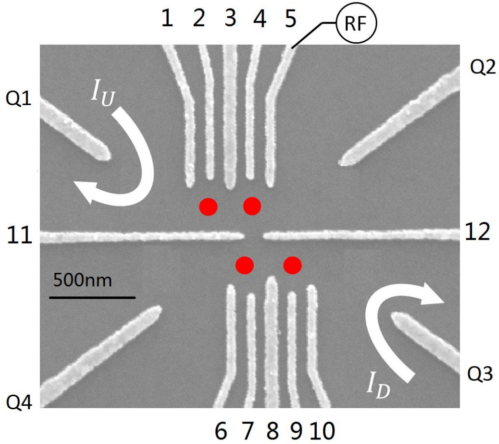
图 4.1 (a)Ti/Au 电极 1-12 定义了一个典型的四量子点结构。在上下两组量子点共用横向电极 11 和 12 的基础上，电极 1-5 定义了一个典型的双量子点；电极 6-10 同样定义了一个典型的双量子点。电极 Q1-Q4 是四个 QPC 电极，用来形成四个 QPC 测量通道。白色箭头表示了测量电流流过的方向。红色的四个圆点表示了四个量子点的假想位置
