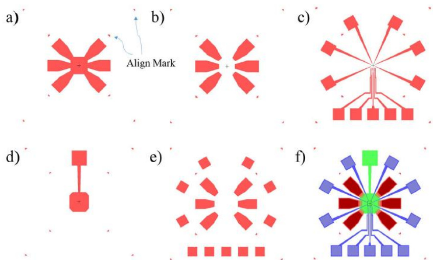
图 2.2 这是一组用 Altium 软件绘制的光刻板 CAD 图样。(a)mesa; 其中虚线箭头处标示了对准位置。(b) 欧姆接触电极；(c) 表面电极；(d)top gate, 在有些样品，比如非掺杂的 GaAs 晶圆上需要使用；(e) 统称为 pad 的大电极；(f) 总体效果。
