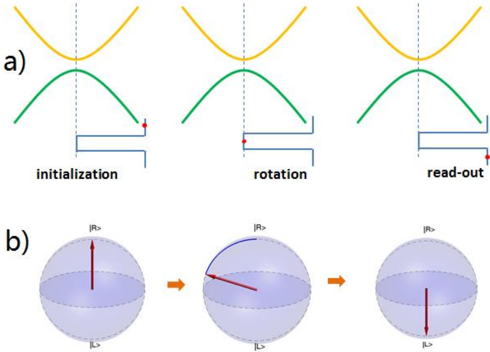
图 1.7 a) 展示了 Rabi 振荡过程的三个不同时间阶段，分别用红色圆点标记。(b) 给出了 bloch 球上，每个演化阶段 qubit 相应的运动行为。
