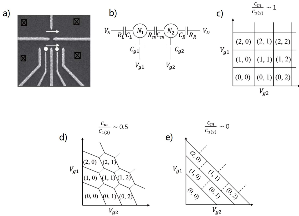
图 1.5 (a) 是一个典型的串联双量子点结构。(b) 是常电容模型下，串联双量子点的等效电路图。量子点与门电极和源漏 (电子库) 之间，两个量子点之间，通过等效电容耦合起来。(c-e) 展现了双量子点之间耦合 C_m 和量子点与电子库之间耦合 C_{1,2} 处在不同区域时，分别呈现的‘弱耦合’，‘一般耦合’，‘强耦合’三种情况。
