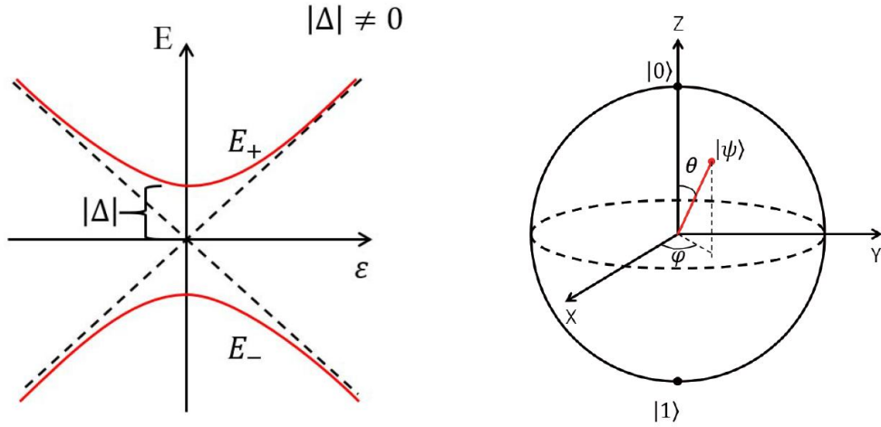
图 1.6 (a) 一个典型的二能级体系的能级图，横轴为失谐量 \epsilon 。 \epsilon = 0 时，上下两个电极之间的差值为 2\Delta 。(b) Bloch 球上的每一点都代表了一个态
