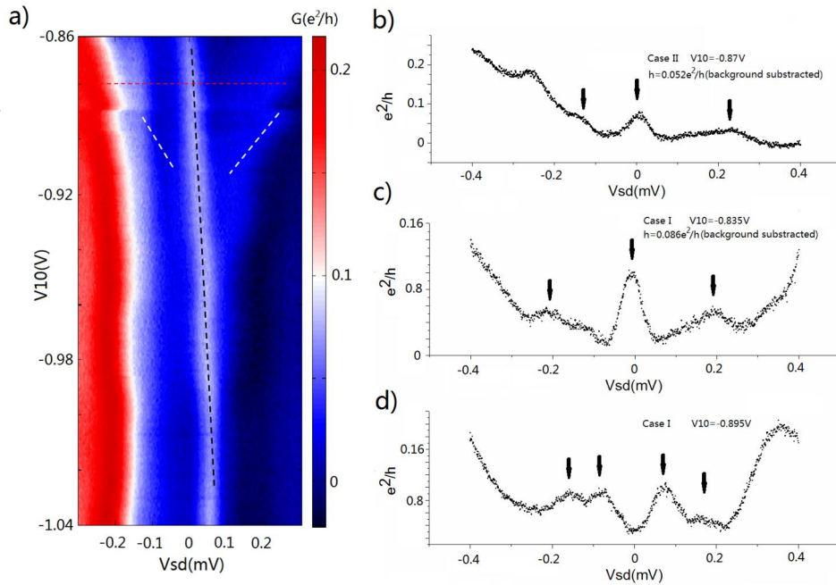
图 5.10 为了证明我们在图 (5.9 a)(情况 1) 中观察的现象是来自于上下两组双量子点之间的耦合，我们将下面双量子点的两个 plunge gate V_7 和 V_9 从 -0.4V 变化到 0V(情况 2)。同时扫描 V_6 和 V_{10} ，读出上面双量子点的微分电导 dI/dV 。(a) 中， V_{10}=-0.875 处的跳跃是一个偶然的随机跳跃，量子点系统中偶尔会出现这种整体的突然移动，可以被忽略。白色虚线标记了中央峰两侧相互靠近的两个“隆起”。它们从 V_{10}=-0.86 V 到 V_{10}=-0.93 V 的区域，依然保持了靠拢的趋势。之后随着 V_{10} 向负方向的增加而消失。(b) 是从 (a) 中抽取的曲线，位置在 ( V_{10}=-0.87 V)，(c) 和 (d) 是从图 (5.9 a) 中抽取的曲线，位置在 ( V_{10}=-0.835 V, -0.895V)。(b) 中，中央峰的高度明显降低了，约在 0.052e^2/h ，而且整个 V_{10} 范围内变化不大。(c) 中的中央峰高度则有 0.086e^2/h 。(d) 图清晰地展示了一个四峰结构 (情况 1)。
