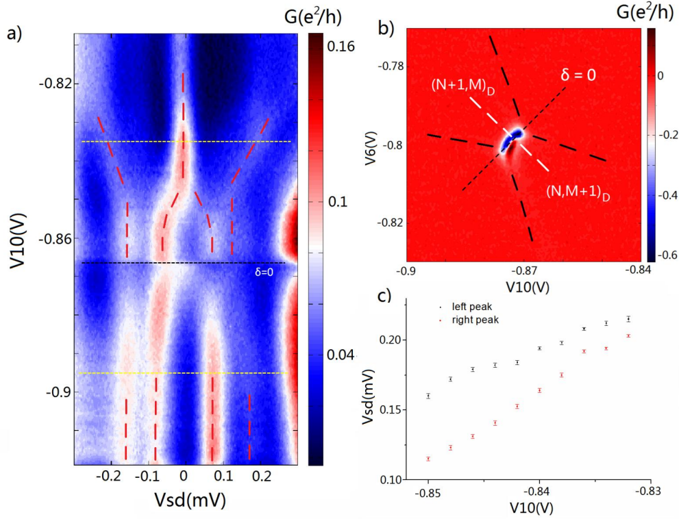
图 5.9 (a) 显示了当沿着 (b) 中白色虚线所示的路径，扫描下面双量子点的相应电压时，上面双量子点源漏通道的微分电导 dI/dV 的变化情况。Kondo 峰用红色虚线标记出来。从 V_{10}=-0.82V 到 V_{10}=-0.85V 阶段，这里出现了中央峰，连同其他两个不断靠拢的侧峰。在 V_{10}=-0.866 的位置，这里出现了一个跳跃 (位置用黑色虚线标记)，对着下面双量子点出现了一个电子态的变化 [从 (N+1, M)_D 到 (N, M+1)_D ]。 (b) 显示了 (N, M)_D 区域附近的细节。黑色虚线标记了库伦峰的位置；较细的虚线标记了失谐量 \delta = 0 的位置；白色虚线标记了扫描路径，从 (V_6=-0.855V, V_{10}=-0.807V) 到 (V_6=-0.752V, V_{10}=-0.919V) 。 (c) 展示了左右两峰到 V=0 位置的绝对距离。可以发现，随着 V_{10} 从 -0.83V 变化到 -0.85V ，其差距越来越大。
