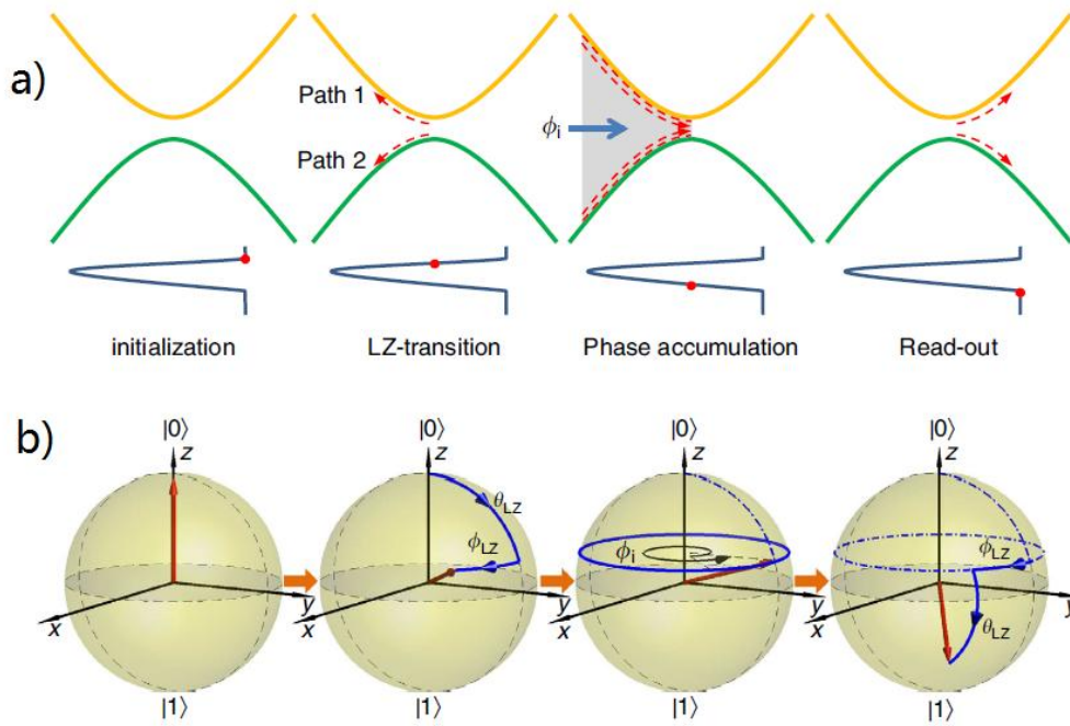
图 1.8 a) 展示了 LZS 干涉过程的四个不同时间阶段，分别用红色圆点标记。(b) 给出了 bloch 球上，每个演化阶段 qubit 相应的运动行为。
