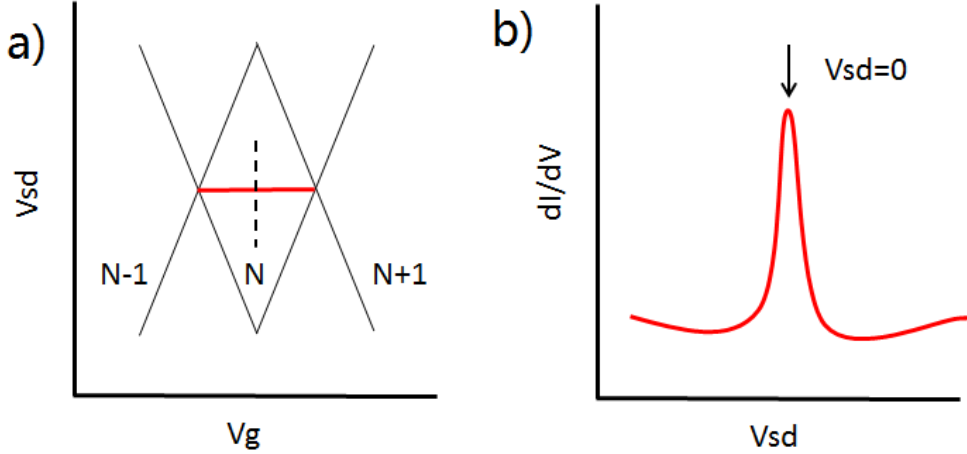
图 5.2 (a) 是一个典型的库伦阻塞。如果出现 Kondo 效应，那么我们能从红线所表示的位置上观察到电导不为 0 的现象。虚线是沿着源漏偏压 V_{sd} 方向扫描，可以绘制出如 (b) 的图。(b) 上的中央电导峰，一般认为是 Kondo 效应的基本特征。
