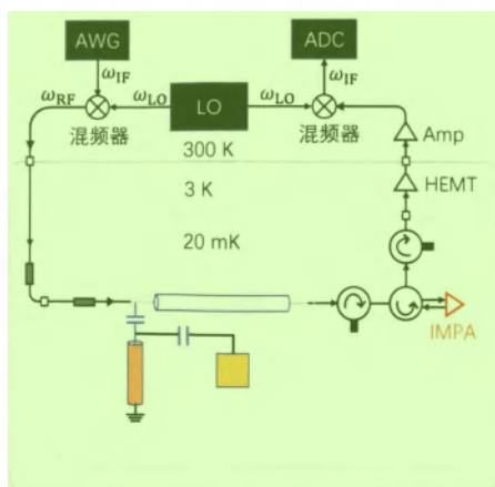
图 5.1 超导量子比特读取线路示意图。
