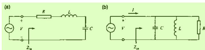
图 3.1 (a) 串联 RLC 电路。(b) 并联 RLC 电路。 7
