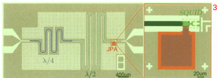
图 4.16 基于片上阻抗变换的 IMPA 的芯片设计版图。
