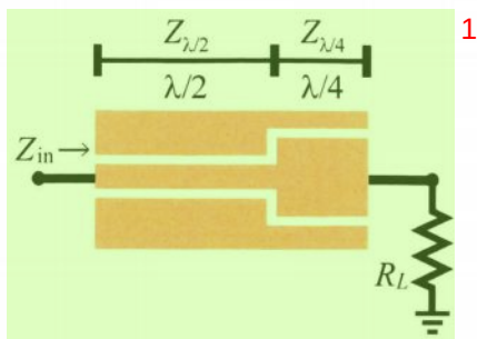
图 4.8 共面波导阻抗变换器示意图。
