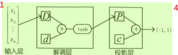
图 5.8 阈值投影法态分类器 (a) 与浅层神经网络态分类器 (b) 的结构以及对应关系。5
