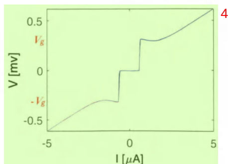
图 4.4 约瑟夫森结直流 I-V 特性曲线。图中 V_g \approx 0.316\ \text{mV} 。
