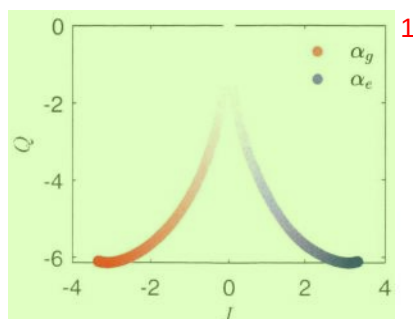
图 2.6 典型的腔光场在 I-Q 平面的演化轨迹图，线条颜色深度的增加代表演化时间的增加。2
