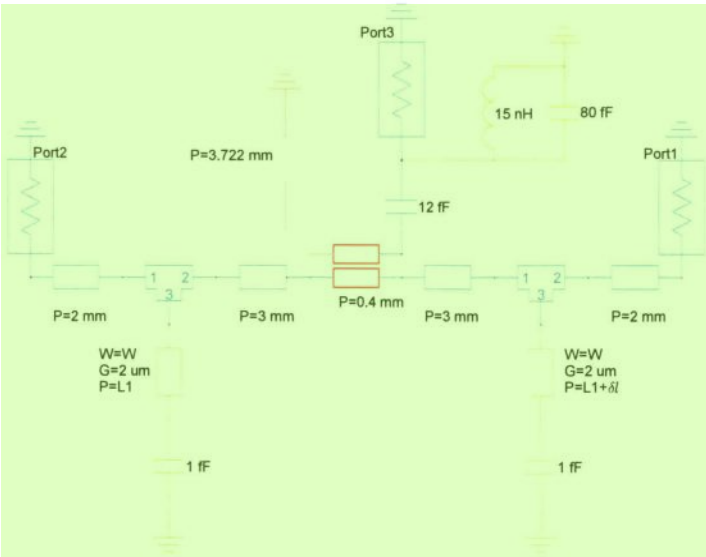
图 3.5 Purcell 滤波器的仿真电路图。黄色部分表示量子比特，橙色表示读取谐振腔，红色部分是谐振腔与读取总线的耦合部分，绿色部分表示滤波器。仿真使用的衬底为理想的本征硅，P 表示各段传输线的长度，G 表示传输线中央导带线距离地平面的距离，对于所有传输线 G=2\text{ }\mu\text{m} ，W 表示滤波器的中央导带线线宽，对于读取总线以及谐振腔，中央导带线线宽为 3.2\text{ }\mu\text{m} ，从而满足 50\text{ }\Omega 的阻抗匹配条件。
