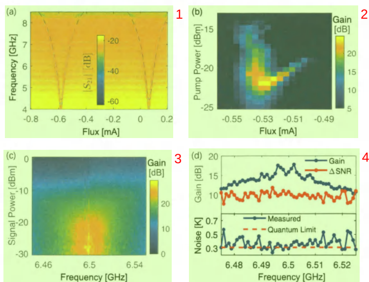
图 4.7 JPA 实验测量结果图。(a) JPA 的直流调制谱图, 谐振频率随着直流偏置磁通周期性变化, 且可调范围大于 4 GHz~8 GHz。图中黑色虚线为拟合曲线。(b) \delta = 10 MHz 时的信号增益与泵浦功率和直流偏置磁通的变化关系。(c) 信号增益随信号输入功率的变化关系, 随着输入功率增大, 增益逐渐减小, 输入线上的总衰减量为 -101 dB。(d) \Delta SNR 法测到的系统噪声温度。
