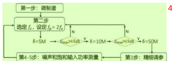
图 4.6 JPA 低温测试表征流程图。5
