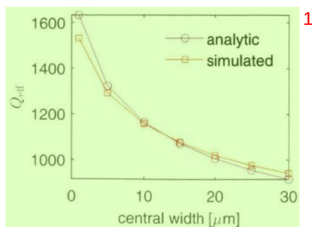
图 3.8 Purcell 滤波器对读取谐振腔的有效外部耦合 Q_{\text{eff}} 的影响。
