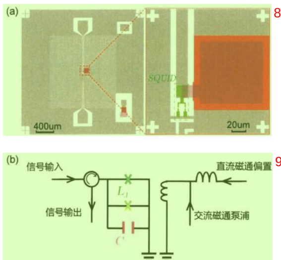
图 4.3 JPA 芯片设计版图 (a) 与它的等效电路图 (b)。版图中灰色代表第一层结构；红色 10 为第二层，代表电容介质层；紫色为第三层，代表电容上级板；绿色为第四层，代表 SQUID 环路（绿色虚线方框）。版图右上角和右下角分别有 SQUID 和电容测试结构，用于常温下的参数表征测试。
