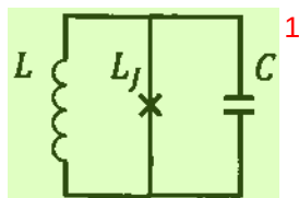
图 1.4 超导量子比特的一般等效电路模型。2
