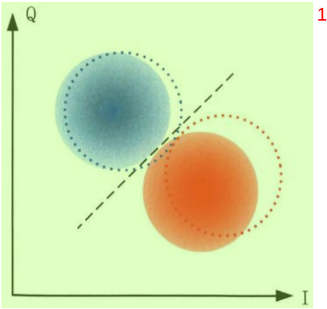
图 5.5 一个两比特体系中 IQ 圆斑偏移的示意图。两个实心圆表示 Q3 处在 |0\rangle 态时 Q4 的两个 IQ 圆斑，蓝色代表 |0\rangle 态，红色则代表 |1\rangle 态。黑色虚线表示此时的最佳二分类直线。两个虚线圆表示 Q3 处在 |1\rangle 态时 Q4 的两个 IQ 圆斑，由于与 Q3 处在 |0\rangle 态时 Q4 的两个 IQ 圆斑有明显的偏移，原来的最佳的分类线此时将不再适用。
