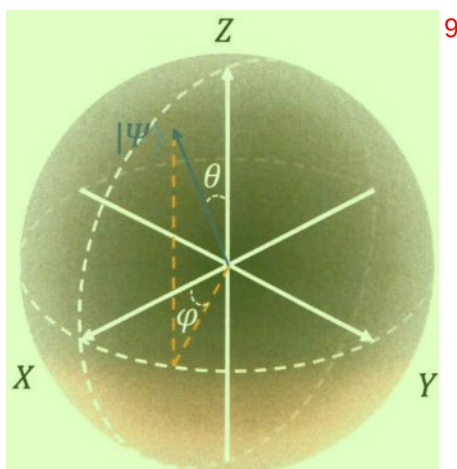
图 1.1 量子态在布洛赫球上的表示。
