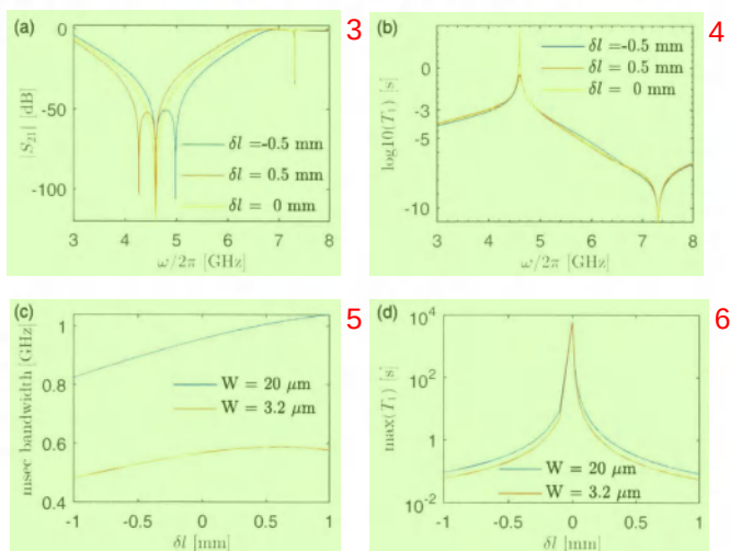
图 3.7 两个 \lambda/4 滤波器的长度差值 \delta l 对结果的影响图。(a) \delta l 取不同值时的 S_{21} 幅值谱。(b) \delta l 取不同值时根据仿真结果计算的量子比特 T_1 , 其中虚线表示 T_1 = 1 \text{ ms} 。(c) W 取不同值时分别扫描 \delta l 得到的毫秒带宽与 \delta l 的变化关系。(d) 滤波器中心保护频率出的 T_1 与 \delta l 的变化关系。
