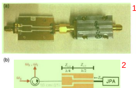
图 4.14 JPA 外接阻抗变换器样品图 (a) 及其等效电路和信号流程图 (b)。阻抗变换器与环形器之间一般用约 10 cm 长的低温同轴线缆相连接。
