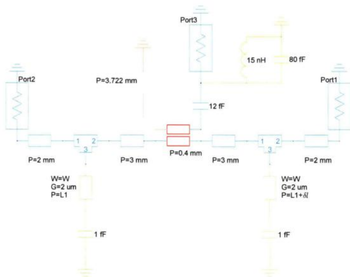
图 3.5 Purcell 滤波器的仿真电路图。黄色部分表示量子比特，橙色表示读取谐振腔，红色部分是谐振腔与读取总线的耦合部分，绿色部分表示滤波器。仿真使用的衬底为理想的本征硅，P 表示各段传输线的长度，G 表示传输线中央导带线距离地平面的距离，对于所有传输线 G=2\text{ }\mu\text{m} ，W 表示滤波器的中央导带线宽，对于读取总线以及谐振腔，中央导带线宽为 3.2\text{ }\mu\text{m} ，从而满足 50\text{ }\Omega 的阻抗匹配条件。
