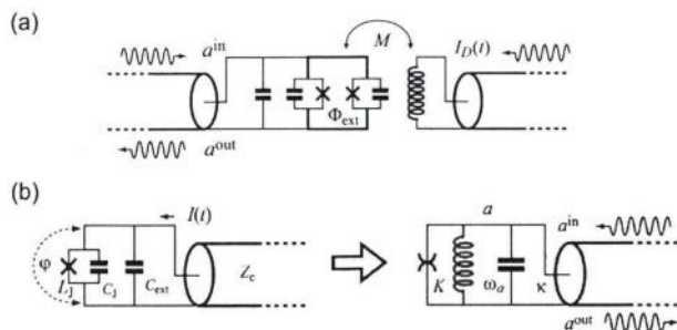
图 4.1 (a) 磁通泵浦模式的等效电路图，外部驱动以外磁通的形式通过互感作用到 SQUID 回路。(b) 直接泵浦模式下的等效电路图， K 表示线路的非谐。图片引自文献 [27] 。
