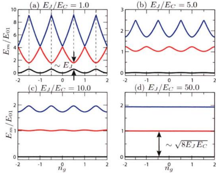
图 1.5 不同参数条件下的电荷量子比特的本征能级图，图片引自文献 [57] 。
