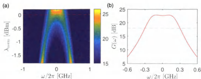
图 4.11 给定的一组合理参数条件, 计算增益曲线以及该曲线随泵浦功率的变化关系。(a) 增益曲线随泵浦功率的变化关系, 其中泵浦功率 \lambda_{\text{norm}} = 20 \log(\lambda_f/\lambda_{\text{opt}}) , 红色虚线表示此处满足阻抗匹配条件。(b) 满足阻抗匹配条件下的增益曲线, 其中 G_0 = 22.7 \text{ dB} , \Gamma_{\text{BW}}/2\pi = 600 \text{ MHz} , 图中蓝色虚线表示最小增益设计目标 G_{\text{min}} = 18 \text{ dB} 。其他相关参数为 Z_{\lambda/2} = 60 \Omega , Z_{\lambda/4} = 33 \Omega , C = 3 \text{ pF} , \omega_f/2\pi = 6.8 \text{ GHz} , \Omega_p/2\pi = 13.6 \text{ GHz} , \lambda_{\text{opt}}/2\pi = 1.132 \text{ GHz} , \Delta_{\text{opt}} = 0 。
