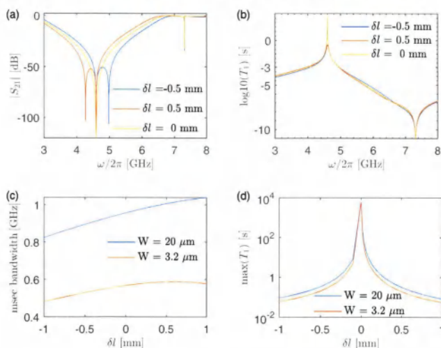
图 3.7 两个 \lambda/4 滤波器的长度差值 \delta l 对结果的影响图。(a) \delta l 取不同值时的 S_{21} 幅值谱。(b) \delta l 取不同值时根据仿真结果计算的量子比特 T_1 , 其中虚线表示 T_1 = 1 \text{ ms} 。(c) W 取不同值时分别扫描 \delta l 得到的毫秒带宽与 \delta l 的变化关系。(d) 滤波器中心保护频率出的 T_1 与 \delta l 的变化关系。
