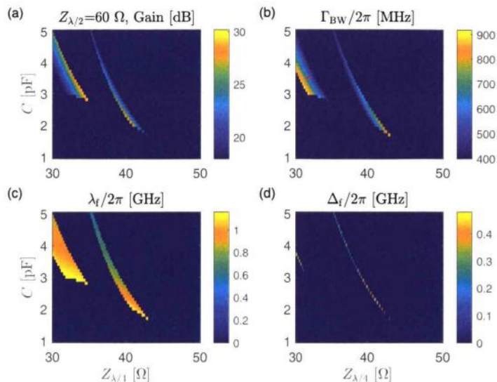
图 4.13 固定 Z_{\lambda/2} = 60\ \Omega , 计算 C 和 Z_{\lambda/4} 对增益和带宽的影响。(a) 满足设计条件前提下计算出来的增益大小。(b) 满足设计条件前提下计算出来的带宽大小, 红色小圆点表示正文中提到的设计参数, 在这个参数条件下, 横向和纵向都有较大的冗余度。(c) 工作点的泵浦强度, 决定磁通泵浦的功率大小。(d) 工作点的泵浦失谐, 决定 JPA 的谐振频率。由于在满足设计条件的前提下, 工作点参数仍然有一定的可调范围, 图 (c) 和 (d) 是按照正文中的最大带宽策略计算的工作点泵浦强度和失谐量。
