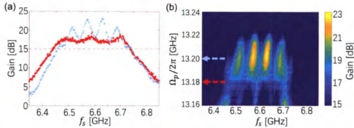
图 4.19 IMPA 测量中微调泵浦频率的效果。环境阻抗中的小波纹振荡会反映到增益曲线中，通过微调泵浦频率，有可能可以测到更加平坦的增益形貌。(a) 图中的两条增益曲线分别对应 (b) 图中对应颜色箭头指示的该泵浦频率处的增益曲线。
