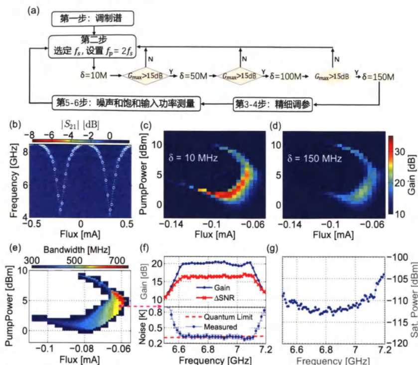
图 4.21 IMPA 的低温测试流程与测量结果。(a) 低温测量流程图, 我们以增益不小于 15 dB, 工作带宽不小于 300 MHz 为筛选目标。(b) 第一步中测到的直流调制谱, 其中白色圆圈虚线是对谐振频率随直流偏置变换关系的拟合结果。(c) (d) 信号增益对直流偏置和泵浦功率的依赖关系。实验中泵浦频率固定在 f_p = 13.7\text{ GHz} , 而网分的输出频率设置为 f_p/2 + \delta , 其中 \delta 根据测量结果可以从 10 MHz (c) 逐步增大到 150 MHz (d), 从而实现对增益形貌的稀疏采样。(e) 经过第三步细调直流偏置和泵浦功率之后测到的工作带宽。图中有颜色区域代表实验中实际的扫描区域, 而该区域正是从第二步测量结果中提取出来的。(f) 在图 (e) 中紫色圆点对应的工作点处测到的增益形貌、 \Delta\text{SNR} 以及计算得到的系统噪声温度。考虑到低温 HEMT 的参考噪声温度平面与 IMPA 之间存在着一定的插损, 而这段插损室温测量值与低温实际值有一定的不确定性, 因此在计算噪声温度时, 引入了 1 dB 的误差范围。(g) 在前述工作点处测量得到的饱和信号输入功率。
