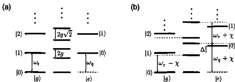
图 2.2 (a) JC 模型共振条件下的能级示意图。(b) JC 模型色散耦合条件下的能级示意图。黑线表示系统无耦合时的本征能级, 蓝线表示系统耦合之后缀饰态本征能级。图片引自文献 [19] 。
