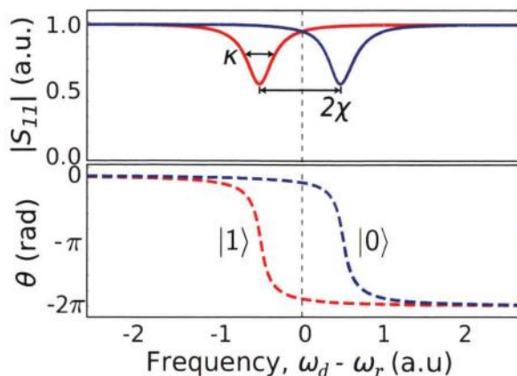
图 2.3 读取谐振腔在不同驱动频率以及不同比特状态下的幅值和相位响应。图片引自文献 [32] 。
