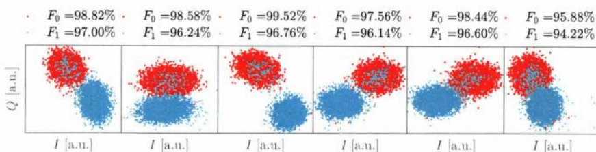
图 4.23 使用 IMPA 之后，六比特芯片的读取效果。
