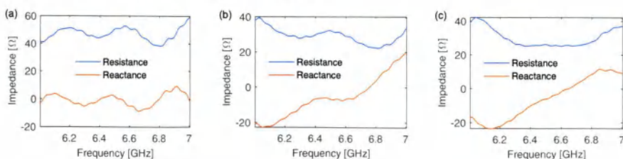
图4.18 实测大部分环形器的端口阻抗(a)以及经过阻抗变换器之后的端口阻抗(b)。(c)个别环形器某个端口阻抗匹配较好,经过阻抗变换器之后的端口阻抗也和预期结果符合得较好。测量过程中环形器的另外两个端口正常连接测量电路,其中一个端口连接信号输入线路,另一个端口连接信号输出线路,也即HEMT所在线路。
