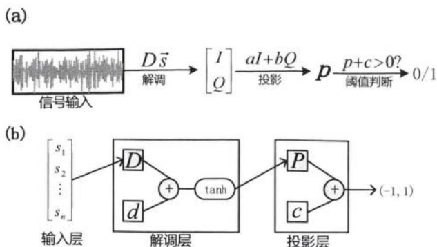
图 5.8 阈值投影法态分类器 (a) 与浅层神经网络态分类器 (b) 的结构以及对应关系。
