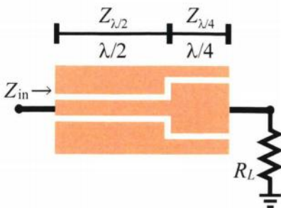
图 4.8 共面波导阻抗变换器示意图。
