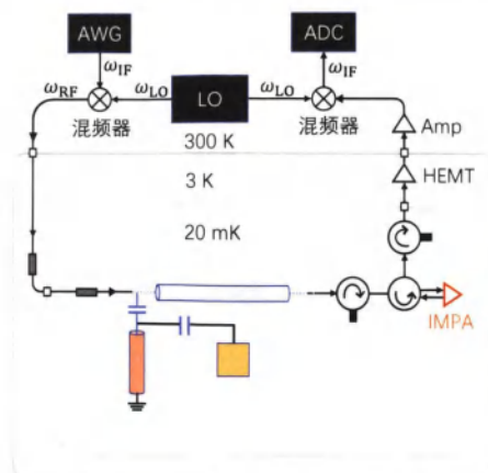
图 5.1 超导量子比特读取线路示意图。
