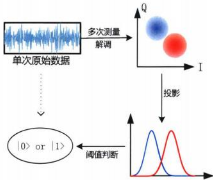
图 5.3 利用投影阈值法构建态分类器过程示意图。
