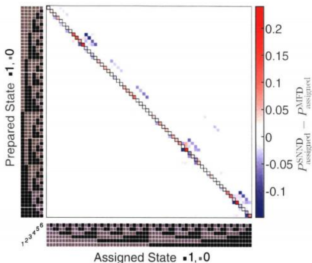
图 5.10 SNND 的混淆矩阵与 MFD 混淆矩阵的差值。比特的状态用一个 6 位的二进制数表示，64 种可能的计算基态在图中的排列顺序为从上到下（从左到右）对应从 000000 到 111111。图中矩阵对角项之和为 247.8%，意味着保真度的大幅度提升。
