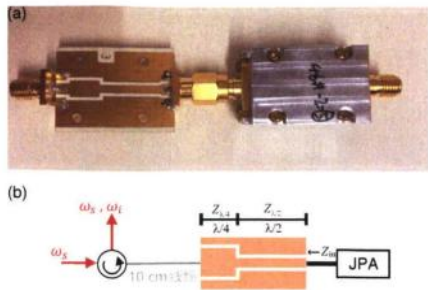
图 4.14 JPA 外接阻抗变换器样品图 (a) 及其等效电路和信号流程图 (b)。阻抗变换器与环形器之间一般用约 10 cm 长的低温同轴线缆相连接。
