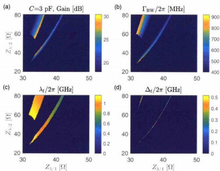
图 4.10 固定 C = 3 \text{ pF} , 计算阻抗变换器的两个特征阻抗值对增益和带宽的影响。(a) 满足设计条件前提下计算出来的增益大小。(b) 满足设计条件前提下计算出来的带宽大小, 红色小圆点表示正文中提到的设计参数。(c) 工作点的泵浦强度, 决定磁通泵浦的功率大小。(d) 工作点的泵浦失谐, 决定 JPA 的谐振频率。由于在满足设计条件的前提下, 工作点参数仍然有一定的可调范围, 图 (c) 和 (d) 是按照正文中的最大带宽策略计算的工作点泵浦强度和失谐量。
