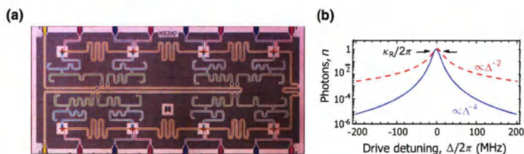
图 5.6 每个读取腔设置独立的 Purcell 滤波器可以有效抑制读取串扰。(a) 样品结构图。(b) 红色虚线表示没有 Purcell 滤波器时谐振腔的激发光子数与驱动频率失谐量的关系，而蓝色线表示有了独立的 Purcell 滤波器之后的情形。图片引自文献 [6] 。
