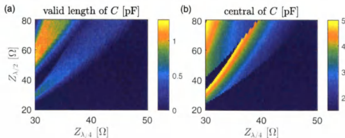
图 4.12 (a) 满足设计条件的参数空间中电容参数的误差容忍度。(b) 满足条件的电容参数的中心值随阻抗变换器两个特征阻抗的变化关系。
