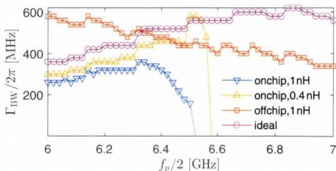
图 4.17 绑线电感对于片外和片上阻抗变换方案的影响。理想条件为环境阻抗 R_L = 50 \Omega ，计算中采用的设计参数为 \omega_i/2\pi = 6.5 \text{ GHz} ， C = 3 \text{ pF} ， Z_{\lambda/2} = 60 \Omega ， Z_{\lambda/4} = 39.2 \Omega 。
