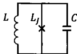
图 1.4 超导量子比特的一般等效电路模型。
