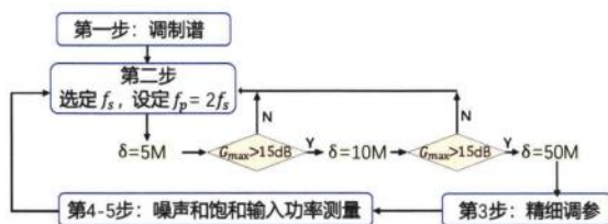
图 4.6 JPA 低温测试表征流程图。
