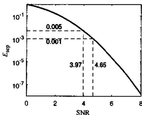
图 2.5 态分离错误率随信噪比的变化关系。图中红色和绿色虚线分别指示 E_{sep} 为 0.005 和 0.001 时对应的 SNR 的大小。
