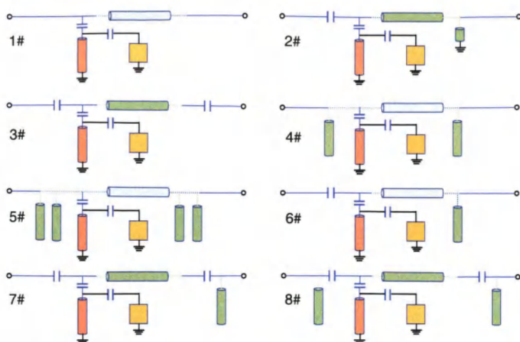
图 3.10 8 种不同设计的 Purcell 滤波器等效电路图，其中 1# 没有 Purcell 滤波器。图中橙色代表读取谐振腔，黄色代表量子比特，绿色代表 Purcell 滤波器。
