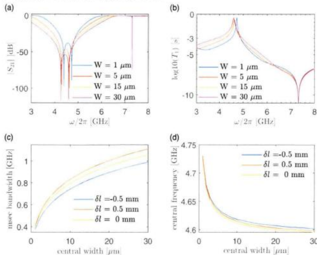
图 3.6 滤波器的中央导带线宽 W 对结果的影响图。(a) W 取不同值时的 S_{21} 幅值谱。(b) W 取不同值时根据仿真结果计算的量子比特 T_1 ，其中虚线表示 T_1 = 1 \text{ ms} 。(c) \delta l 取不同值时分别扫描 W 得到的毫秒带宽与 W 的变化关系，纵轴毫秒带宽表示从图 (b) 中提取的 T_1 \geq 1 \text{ ms} 时的带宽。(d) 滤波器中心保护频率与 W 的变化关系。
