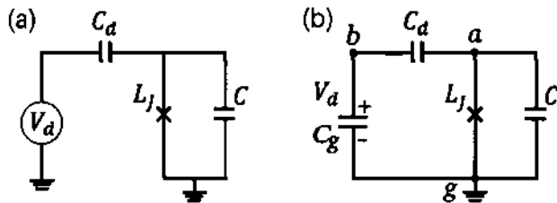
图 1.6 (a) 微波驱动电压 V_d 通过电容 C_d 作用到 transmon 量子比特的电路示意图。(b) 将驱动电压源等效为一个偏置电压为 V_d 的电容, 图中标注的 a, b, g 为电路的几个节点。
