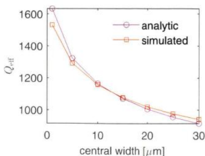
图 3.8 Purcell 滤波器对读取谐振腔的有效外部耦合 Q 值 Q_{\text{eff}} 的影响。
