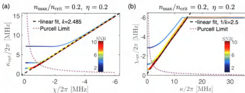
图 2.9 \kappa_{\text{opt}} 随 \chi 的变化关系 (a) 以及 \chi_{\text{opt}} 随 \kappa 的变化关系 (b)。三条彩色圆点状线从上到下依次代表 \tau = 0.2 \mu\text{s} 、 \tau = 0.5 \mu\text{s} 、 \tau = 1 \mu\text{s} 。图中紫色虚线代表 Purcell 极限，黑色虚线是对 \tau = 1 \mu\text{s} 线性部分的拟合。
