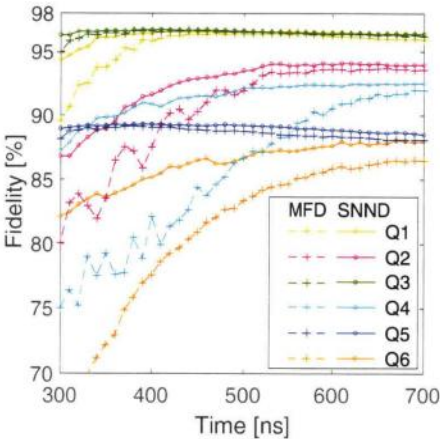
图 5.9 各分类器的保真度与数据解调时间长度的关系。
