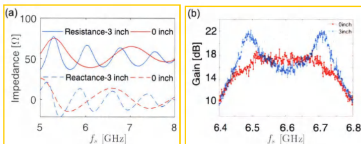
图 4.20 环形器端口到阻抗变换器之间的连接线长度对环境阻抗的影响 (a) 以及对 IMPA 增益的影响 (b)。测量 (a) 图时环形器的另外两个端口接标准 50 \Omega 负载，因此阻抗曲线较为平滑。
