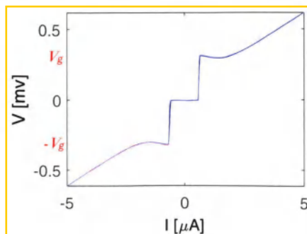
图 4.4 约瑟夫森结直流 I-V 特性曲线。图中 V_g \approx 0.316\ \text{mV} 。
