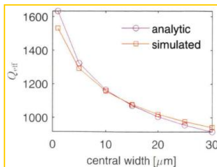
图 3.8 Purcell 滤波器对读取谐振腔的有效外部耦合 Q_{\text{eff}} 的影响。
