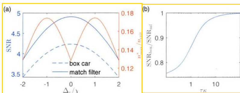
图 2.7 (a) 读取信噪比以及饱和光子数随驱动频率的变化关系。图中蓝线对应左边纵轴，表示信噪比 SNR 与驱动频率的关系，浅红色线对应右边纵轴，表示约化后的饱和光子数 n_{\max}^s/n_{\text{crit}} 与驱动频率的关系，其中 n_{\max}^s = \max(n_{\text{crit}}^s, n_{\text{max}}^s) 。(b) 常系数滤波器与匹配滤波器对信噪比的影响。当积分时间足够长时，二者差距逐渐消失。
