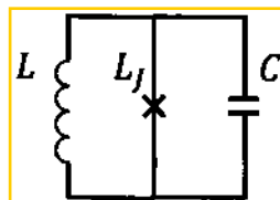
图 1.4 超导量子比特的一般等效电路模型。
