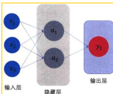
图 5.7 浅层神经网络的基本结构。
