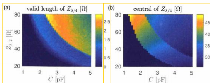
图 4.9 阻抗匹配条件下四分之一波长阻抗变换线的特征阻抗的合法值与另外两个设计参数的关系。(a) Z_{\lambda/4} 的合法区间长度。(b) Z_{\lambda/4} 的合法区间的中心值。
