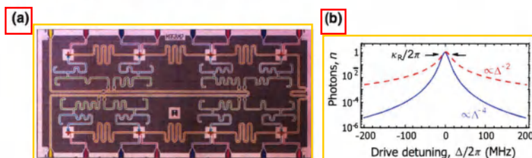
图 5.6 每个读取腔设置独立的 Purcell 滤波器可以有效抑制读取串扰。(a) 样品结构图。(b) 红色虚线表示没有 Purcell 滤波器时谐振腔的激发光子数与驱动频率失谐量的关系，而蓝色实线表示有了独立的 Purcell 滤波器之后的情形。图片引自文献 [6] 。
