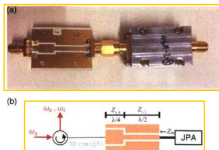
图 4.14 JPA 外接阻抗变换器样品图 (a) 及其等效电路和信号流图 (b)。阻抗变换器与环形器之间一般用约 10 cm 长的低温同轴电缆相连接。
