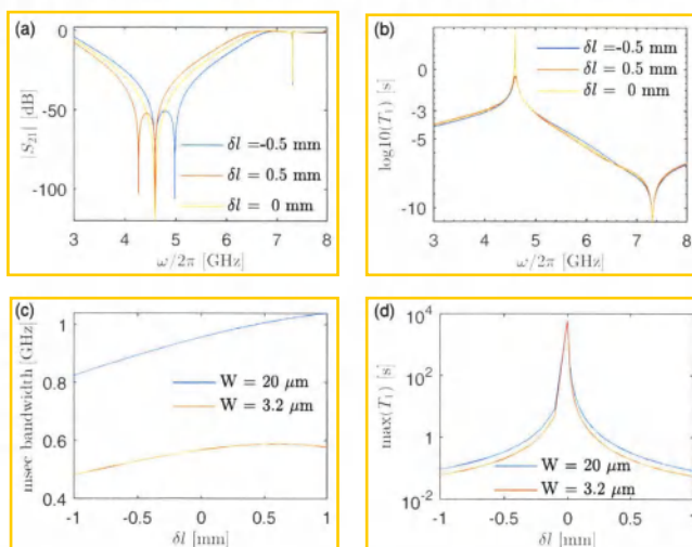
图 3.7 两个 \lambda/4 滤波器的长度差值 \delta l 对结果的影响图。(a) \delta l 取不同值时的 |S_{21}| 幅值谱。(b) \delta l 取不同值时根据仿真结果计算的量子比特 T_1 , 其中虚线表示 T_1 = 1 \text{ ms} 。(c) W 取不同值时分别扫描 \delta l 得到的毫秒带宽与 \delta l 的变化关系。(d) 滤波器中心保护频率出的 T_1 与 \delta l 的变化关系。
