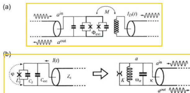
图 4.1 (a) 磁通泵浦模式的等效电路图，外部驱动以外磁通的形式通过互感作用到 SQUID 回路。(b) 直接泵浦模式下的等效电路图， K 表示线路的非谐。图片引自文献 [12] 。
