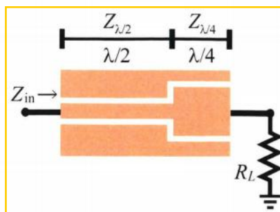
图 4.8 共面波导阻抗变换器示意图。
