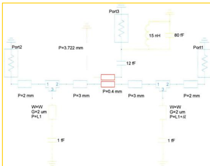
图 3.5 Purcell 滤波器的仿真电路图。黄色部分表示量子比特，橙色表示读取谐振腔，红色部分是谐振腔与读取总线的耦合部分，绿色部分表示滤波器。仿真使用的衬底为理想的本征硅， P 表示各段传输线的长度， G 表示传输线中央导带距离地平面的距离，对于所有传输线 G = 2 \mu\text{m} ， W 表示滤波器的中央导带线宽，对于读取总线以及谐振腔，中央导带线宽为 3.2 \mu\text{m} ，从而满足 50 \Omega 的阻抗匹配条件。
