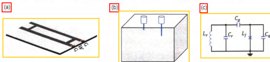
图 2.1 （a）平面共面波导谐振腔结构示意图。灰色为绝缘衬底，浅色为超导金属，中央导带线线宽为 W ，距离两边的地平面的距离为 G 。（b）3D 谐振腔示意图，微波信号通过一个端口耦合到谐振腔内部，通过另一个端口可以探测到谐振腔内部的光场信号。（c）谐振腔与超导量子比特通过电容耦合的等效电路图。
