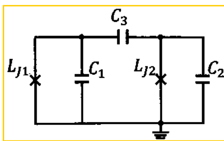
图 1.7 两个 transmon 量子比特通过电容耦合的等效电路图。
