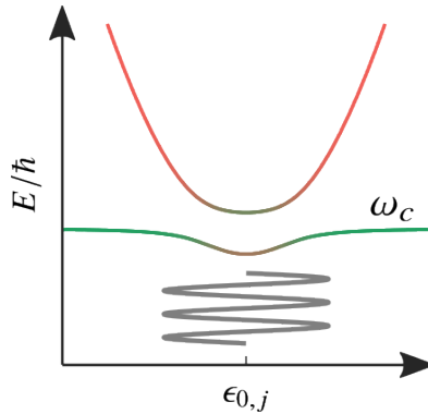
图 5.3 一个双量子点-腔耦合系统的能级示意图。绿色代表腔光子态, 而红色代表双量子点的态, 线的颜色代表了耦合相互作用导致的两个态的杂化程度。灰色的振荡曲线代表微波驱动。裸腔由一个谐振子哈密顿量描述, 其能级是无穷维的, 间隔为 \omega_c , 当然鉴于腔中的较低的光子数占据数目, 一般只需要考虑最低的 N 个能级。这导致耦合后的系统态空间的维度为 2 \times N 维。图中展示的是激发数为 1 的两个态。对于本章涉及的实验参数, 其他能级的能量较高, 可以忽略 [17] 。
