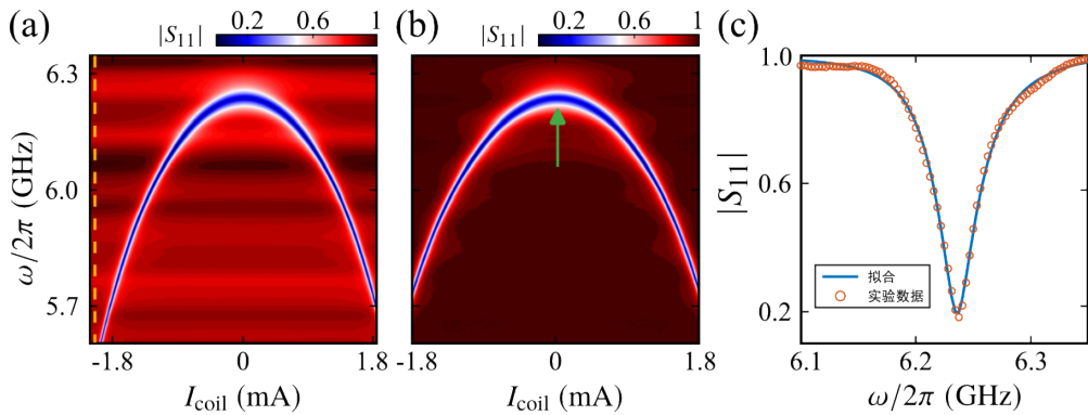
图 3.2 SQUID 阵列反射腔信号。(a) 未去除线路上本底信号的腔反射幅值 |S_{11}| 随线圈中电流 I_{\text{coil}} 和探测频率 \omega/2\pi 变化的相图。(b) 去除本底信号后的腔反射幅值信号。(c) 在 I_{\text{coil}} = 0 \text{ mA} 时（图（b）中的绿色箭头所示位置处）， |S_{11}| 随 \omega/2\pi 的变化。测量时，在量子点电极上施加的负压已经耗尽了量子点处的二维电子气。
