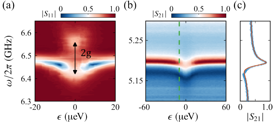
图 2.11 (a-b) 不同样品上测量得到的腔信号随 \epsilon 和探测频率 \omega 变化的相图。此时量子点的转变频率 \omega_q 与腔频 \omega_r 相等。当量子点和腔的耦合强度大于比特和腔的耗散率时，可以看到真空拉比劈裂。(c) 在 \epsilon = -8 \mu\text{eV} 处（图 (b) 绿色虚线）， |S_{21}| 随 \omega_p 的变化。我们可以看到线型并不对称，这是前面讨论的法诺效应导致的 [30] 。
