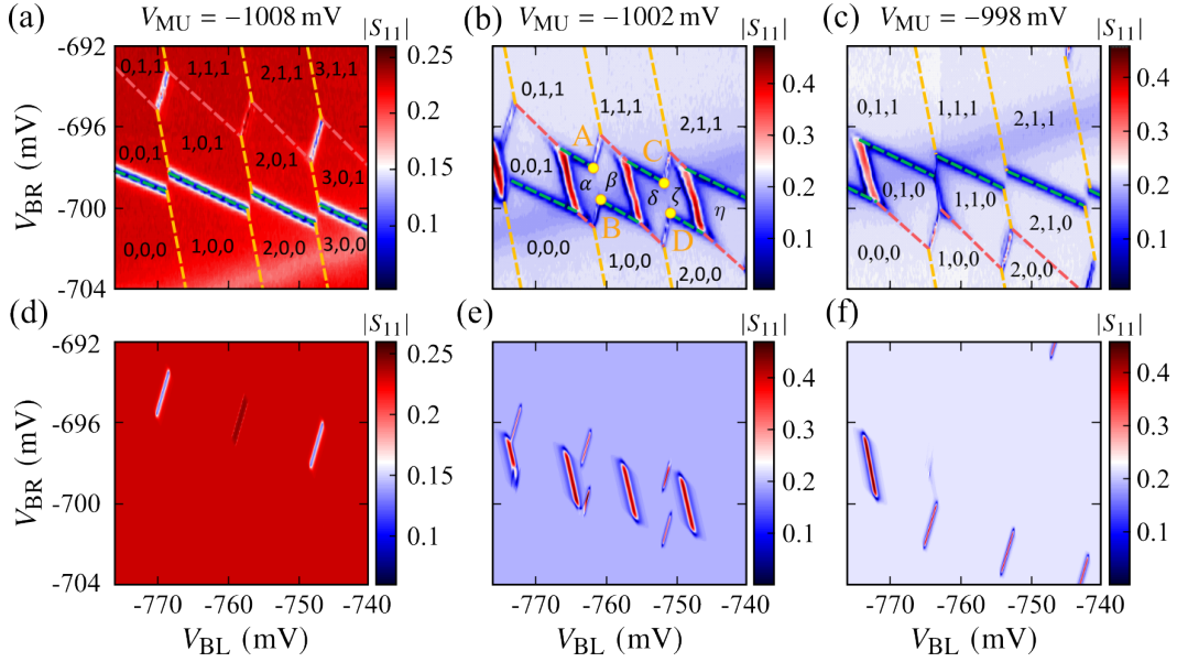
图 3.3 三量子点在不同的 V_{MU} 电压下的电荷稳态图。(a) V_{MU} = -1008 \text{ mV} 。(b) V_{MU} = -1002 \text{ mV} 。其中希腊字母 \alpha, \beta, \delta, \zeta, \eta 分别代表态 (0, 1, 0) , (1, 0, 1) , (1, 1, 0) , (2, 0, 1) 和 (2, 1, 0) 。(c) V_{MU} = -998 \text{ mV} 。为了区别不同的电荷态区域，我们在图中添加了一系列黄色、粉色、绿色的线，这对应于量子点 1、2、3 的充电线。(d-f) 由公式(3.10)计算得到的电荷稳态图。计算时采用的具体参数：(d) (t_{12}, t_{13}, t_{23}) = (9.9, 0, 11.9) \mu\text{eV} ，在中间的隧穿线处 ( V_{BL} = -760 \text{ mV} 附近)， t_{12} = 3.2 \mu\text{eV} ，(e) (t_{12}, t_{13}, t_{23}) = (13.5, 0, 13.1) \mu\text{eV} ，(f) (t_{12}, t_{13}, t_{23}) = (13.3, 0, 13.1) \mu\text{eV} 。此外，我们发现在测量期间，腔频率有所漂移，计算这三幅图时所用的腔频分别为 (d) \omega_r/2\pi = 6.235 \text{ GHz} ，(e) \omega_r/2\pi = 6.234 \text{ GHz} ，(f) \omega_r/2\pi = 6.235 \text{ GHz} 。电子温度 T_e = 80 \text{ mK} ，三量子点的退相干速率为 \gamma = 0.25 \text{ GHz} 。 g/2\pi = 80 \text{ MHz} ， a_1 = -1 ， a_2 = 1 ， a_3 = -0.825 。利用式(3.3)可知，上述参数代表点 1 和 2 之间的耦合强度为 g^{12}/2\pi = 80 \text{ MHz} ，而点 2 和 3 之间的耦合强度为 g^{23}/2\pi = 73 \text{ MHz} 。值得注意的是，在模拟结果图中，我们没有看到量子点的充电线。正如3.3节所讨论的，这是因为我们的模型只能描述腔对总电子数目相同的态之间的跃迁的响应。考虑腔对电子在量子点和源漏之间的信号，需要其他的模型 [26-27] 。
