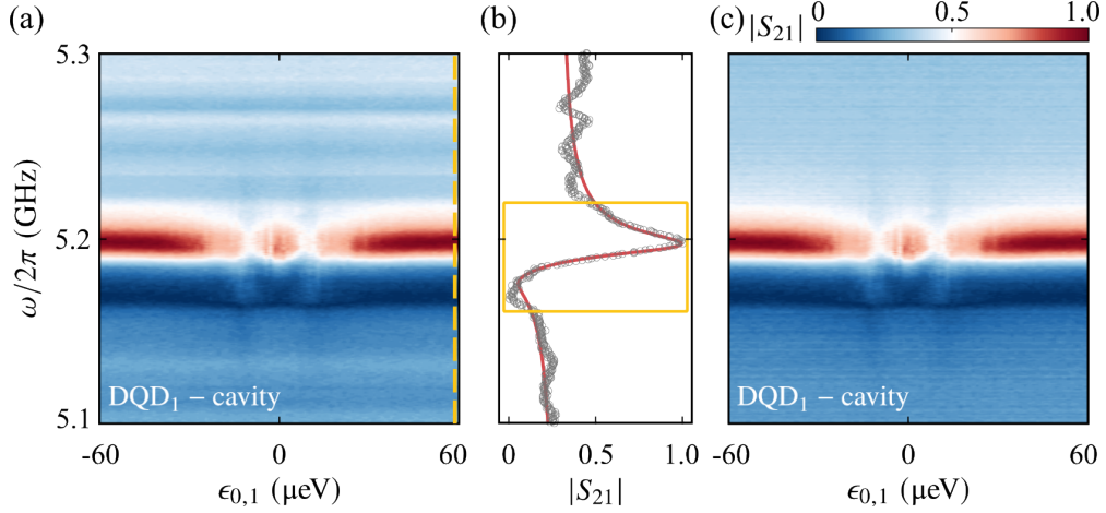
图 8 (a) 测量到的原始数据 |S_{21}| 随探测频率 \omega 和失谐偏移量 \epsilon_{0,1} 的变化。我们可以看到图中有很多水平方向的横线。(b) 图 (a) 中的黄色虚线处提取的 |S_{21}| 随 \omega 的变化。灰色的空心圆为数据点。红色的实线为利用裸腔的透射信号公式得到的。这里可以看到腔的共振峰关于中心频率并不对称，这是2.4.2讨论的法诺效应导致的。为了避免对数据过处理，我们只没有去除黄色方框范围内 ( \omega_p/2\pi = 5.16 \text{ GHz} \sim 5.22 \text{ GHz} ) 的本底。去除本底后的数据展示在图 (c) 中。
