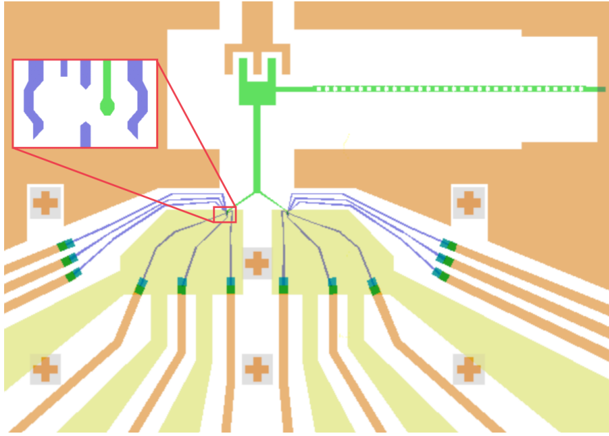
图 2.5 SQUID 阵列反射腔和量子点耦合样品设计图。图中绿色部分为 SQUID 阵列，构成了腔的中心导体，橘色部分为腔的地平面。紫色的小电极代表两个双量子点，插图部分为放大的双量子点的电极结构，两个量子点的结构相同，成镜像对称。腔中心导体部分伸出一根金属导体连接到两个双量子点的 plunger 电极（绿色）上，实现腔和量子点的耦合。
