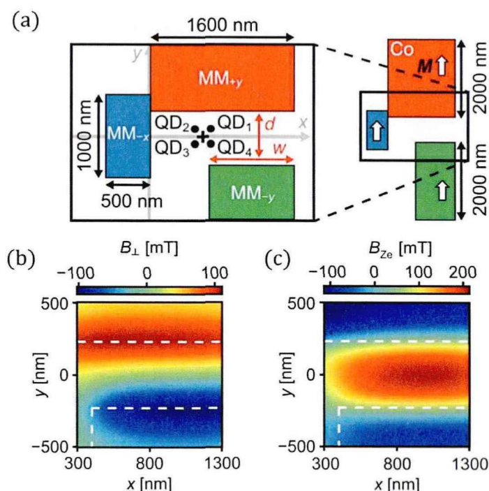
图 3.9 (a) 2 \times 2 量子点阵列的微磁体结构设计。x-y 坐标系定义了微磁体与量子点的相对位置。微磁体结构+y 部分和微磁体结构-y 部分的右边缘在 x=1600 \text{ nm} 处对齐。白色箭头指示的方向为微磁体的磁化方向。设置微磁体的饱和磁化强度为 1.8 \text{ T} 。(b) 有效磁场梯度分布图。白色虚线表示微磁体的边缘。(c) 用于寻址操作的磁场差值分布图。图片引用自[105]。
