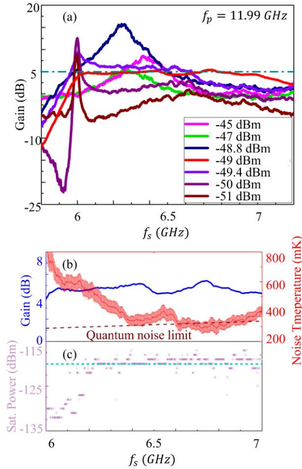
图 3.5.9 (a) 当 f_p = 11.99 \text{ GHz} 时改变 pump 功率，所得到的 J-IMPA 增益曲线变化关系，特别是当 P_p = -49 \text{ dBm} 时（红色曲线），我们得到了非常平坦的增益曲线，在 1.2 GHz 的 3 dB 带宽内有非常稳定的 5 dB 增益，5 dB 阈值用虚线标出； (b) P_p = -49 \text{ dBm} 时对应的带 error-bar 的噪声温度曲线（红色曲线）与量子噪声极限曲线（褐色曲线）对比图，增益也画在同一张图中，见蓝色曲线； (c) P_p = -49 \text{ dBm} 时对应的信号饱和功率曲线，浅蓝色虚线标出的是 -120 dBm 的阈值。
