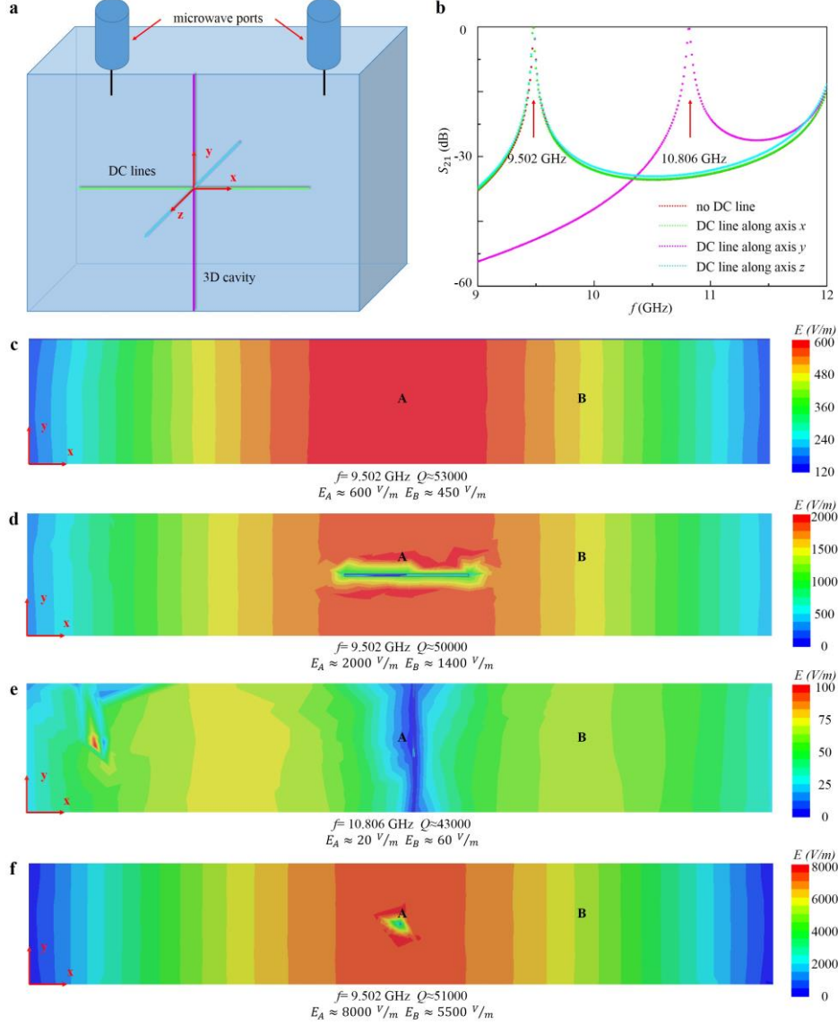
图 3.8.3 引入直流调控的 3D 微波谐振腔 HFSS 仿真结果。(a) 仿真结构示意图，其中， x ， y ， z 为所研究的三个直流电极引入的方向。微波通道的方向为 y 方向。(b) HFSS 仿真得到的 S_{21} 随电极引入方向的不同结果。我们发现，DC 电极引入方向为 y 方向时，会严重破坏 TE 101 模式，而其他的引入方式对 TE 101 模式几乎没有影响。(c) – (f) 分别为不引入直流电极、引入一根 x 方向电极、引入一根 y 方向电极、引入一根 z 方向电极所导致的 xy 平面电场分布剖面仿真图。从结果来看，沿着 y 方向引入电极已经完全破坏了 TE 101 的模式。而沿着 x ， z 方向引入电极，仅会使得电极周围局部区域电场强度减弱，但不会导致 TE 101 模式的变化。
