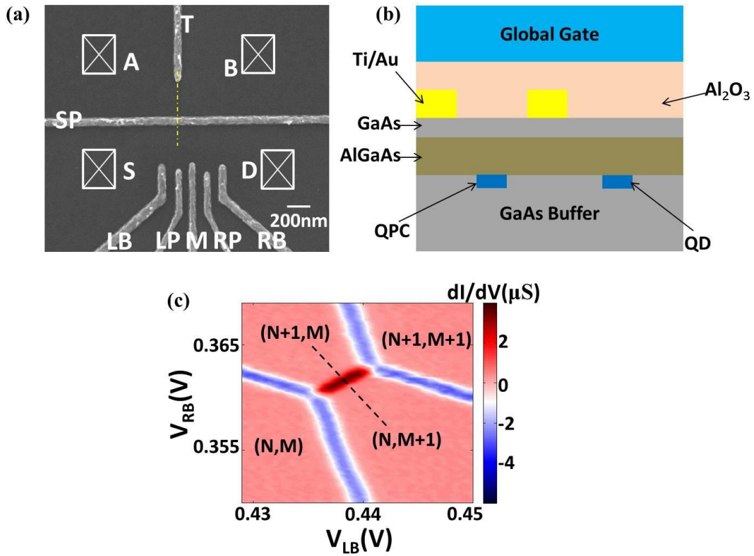
图 6.1 (a) 这次实验所使用双量子点器件的 SEM 图片。下面的五个电极限制出双量子点, T 电极用来调节 QPC 通道的电导, SP 电极用来隔离量子点与 QPC 通道。白色方框 A,B,S,D 表示欧姆电极, 与 2DEG 直接相连。(b) 非掺杂双量子点器件横截面图, 这次实验顶部电极电压 V_T=2.9\text{V} 。(c) QPC 微分电导 dI/dV 随门电极电压 V_{\text{LB}} 和 V_{\text{RB}} 的变化相图。沿着黑色虚线方向, 电子态从 (N+1, M) 到 (N, M+1) 发生转变。
