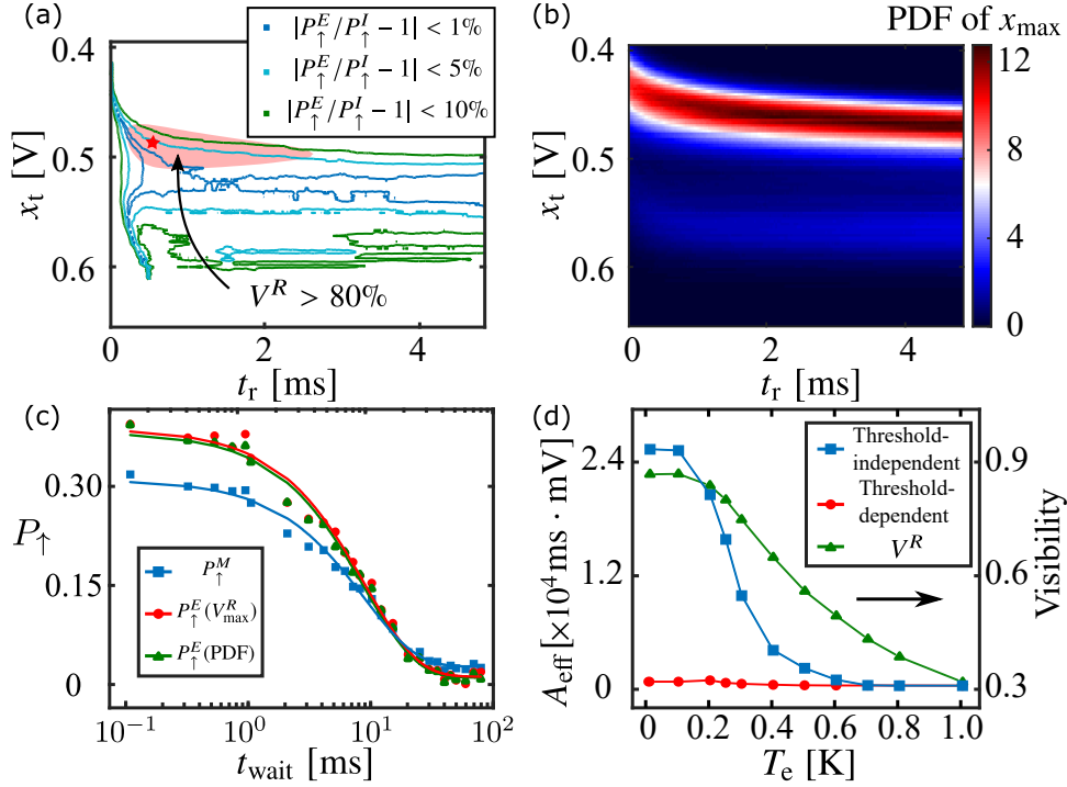
图 3.5 (a) 期望概率 P_{\uparrow}^E 与读取阶段初始概率 P_{\uparrow}^I 的偏差关于时间窗口和电压阈值的轮廓图。图中蓝色、青色和绿色实线分别为 |P_{\uparrow}^E/P_{\uparrow}^I - 1| < 1\% 、 5\% 和 10\% 区域的轮廓线。作为对比，我们用红色星形符号标识出了 V_{\max}^R 的位置，并用粉色阴影区域标识出了 V^R > 80\% 的区域；(b) 不同时间窗口下，读取信号最大值的分布相图。图中可以明显看出信号最大值分布中的双峰位置随着时间窗口增大而向增大的方向平移。图中双峰之间的低谷区域轮廓和 (a) 图中的青色轮廓线相近；(c) 采用阈值无关单发读出方法处理实验数据，我们比较了在 V_{\max}^R 处（红色圆点）和同样时间窗口下读取信号最大值分布的双峰之间最小值位置处（绿色三角形）的 P_{\uparrow}^E ，并用指数衰减函数拟合，发现两者差异较小；与用传统方法处理得到的测量概率 P_{\uparrow}^M （蓝色方形）相比，采用阈值无关单发读出方法处理得到的 P_{\uparrow}^E 更加接近目标值 P_{\uparrow}^I 、且暗记数较小；(d) 蓝色方形和红色圆形分别表示不同电子温度下阈值无关单发读出方法和传统方法的有效参数空间大小 A_{\text{eff}} ，绿色三角形为该温度下的最大读取可见度。
