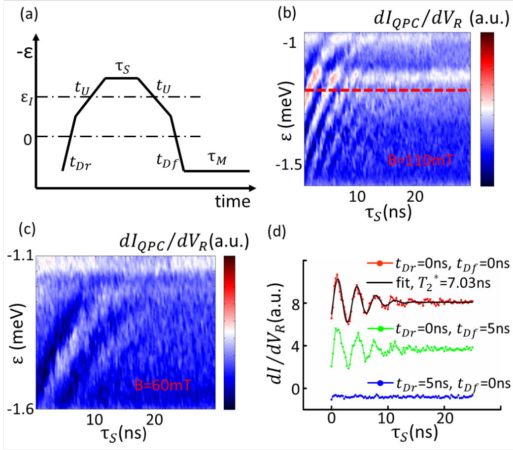
图 3.4 (a)用于测量 LZS 振荡的失谐脉冲。(b)LZS 振荡随着 \epsilon 和 \tau_s 的变化。磁场 B = 110 \text{ mT} 。(c)和(b)一样，但是磁场 B = 60 \text{ mT} 。(d)在与 D_s - D_s 反交叉相关脉冲参数设为不同值时所测得的 LZS 振荡随 \tau_s 的变化。脉冲尖端失谐 \epsilon 设在(b)中红色虚线所指示的位置上。对所有情况 t_U 都设为 5 \text{ ns} 。用高斯衰减余弦函数拟合最上边的红色曲线给出 T_2^* = 7 \text{ ns} 。
