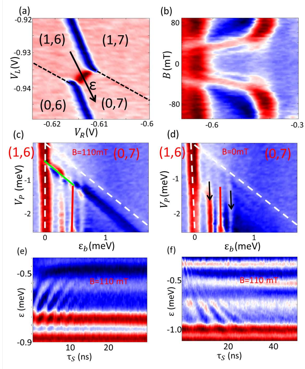
图 3.10 (a) (1,6)-(0,7)电荷跃迁区域附近的相图。黑色箭头定义了失谐轴。施加在电极 L 和 R 上的两个同步脉冲经过校准后沿着此轴改变失谐量。(b) 在沿负失谐轴施加脉冲的情况下，所测得的 QPC 互导 dI_{QPC}/dV_R 随着脉冲尖端的失谐 \varepsilon_t 和磁场 B 的变化。(c) 在沿负失谐轴施加脉冲的情况下，所测得的 QPC 互导 dI_{QPC}/dV_R 随着基准失谐 \varepsilon_b 和脉冲幅度 V_p 的变化。磁场 B=110\text{ mT} 。(d)和(c)一样，只不过磁场 B=0\text{ mT} 。在(b)-(d)中，脉冲宽度 \tau_s = 200\text{ ns} ，测量时间 \tau_m = 5\text{ }\mu\text{s} 。(e) LZS 振荡随着 \varepsilon 和 \tau_s 的变化。磁场 B=110\text{ mT} 。(f) 交换振荡随着交换阶段的失谐 \varepsilon 和持续时间 \tau_s 的变化。磁场 B=110\text{ mT} 。
