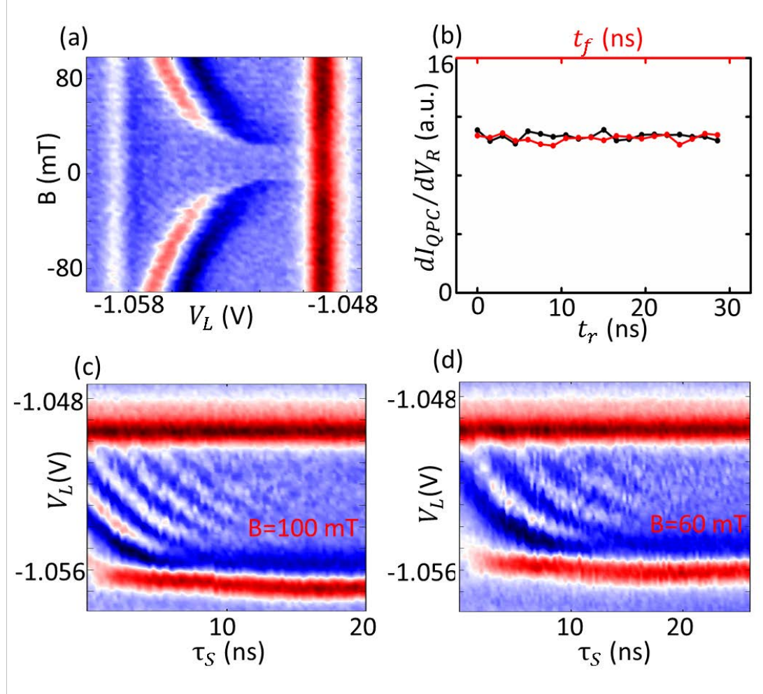
图 4.5 (1,3)-(0,4) 区域的补充数据。(a) 自旋漏斗。实验所用的方脉冲的持续时间为 200ns, 周期为 10 \mu s。(b) 自旋漏斗的信号随脉冲上升沿 t_r 或下降沿 t_f 的变化。当其中一个改变时, 另一个设为零。(c) 磁场 B=100mT 时的 LZS 振荡。(d) 磁场 B=60mT 时的 LZS 振荡。LZS 振荡实验采用的是梯形波, 上升沿为 6ns, 测量时间为 5 \mu s。
