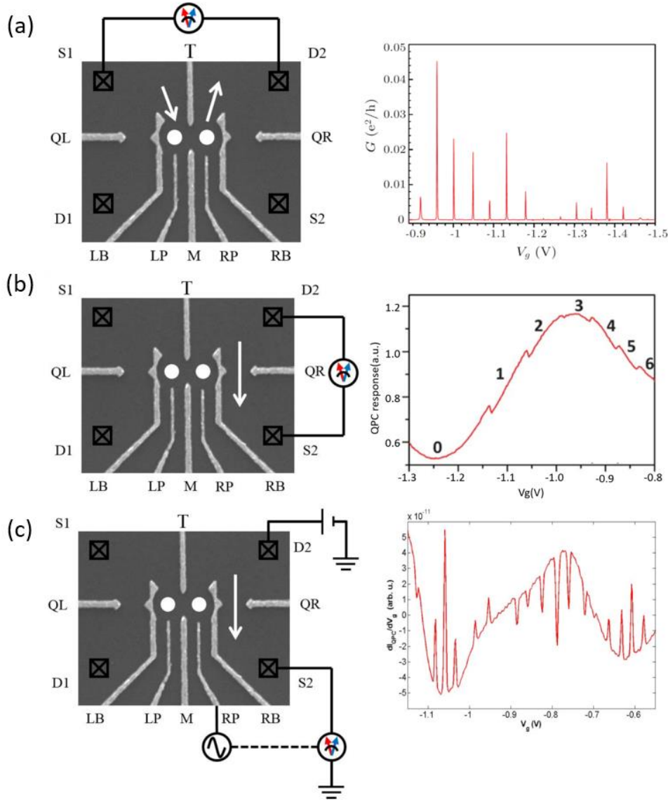
图 2.5: (a) 量子点通道运输测量电路、样品连接示意图和测得信号示意图, (b) 量子点接触运输测量电路、样品连接示意图和测得信号示意图, (c) 量子点接触调制测量电路、样品连接示意图和测得信号示意图。
