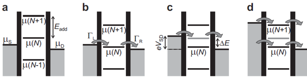
图 1.5：单量子点的四种输运情形。
