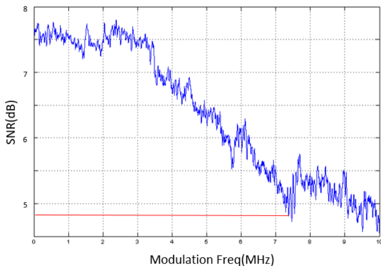
图 3.14: 扫描施加在电极 T 上调制信号的调制频率, 测量其中一个边带的信噪比, 所得到的的关系图。
