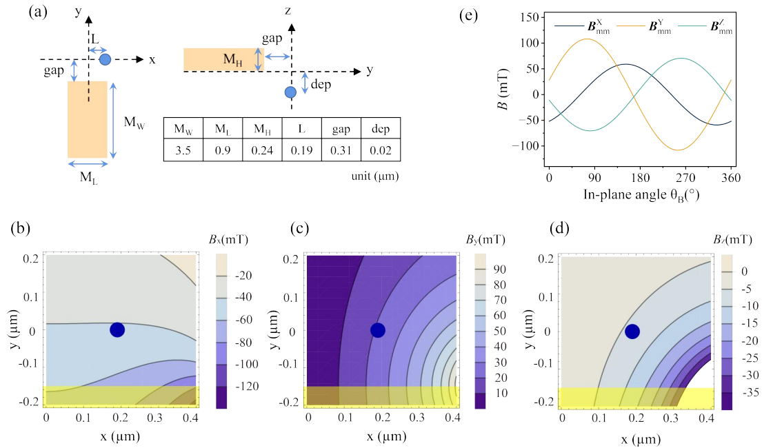
图 4.9 微磁体的模拟。(a) 微磁体的顶视图和侧视图，其中估计的电子位置用蓝色圆圈表示。笛卡尔轴与图4.3中使用的轴一致，表中提供了模拟的尺寸参数。(b-d) 当沿 y 轴施加外部磁场时，在微磁体均匀饱和和磁化的情况下，量子点附近沿 x 、 y 和 z 方向的磁场分量的二维图如图所示。黄色区域代表微磁体的部分。蓝色圆圈表示量子点的位置，圆圈尺寸放大了 10 倍以便看得更清楚。(e) 当外部磁场 B_{ext} 以不同的角度 \theta_B 施加时，微磁体沿三个不同方向的磁场分量的变化。
