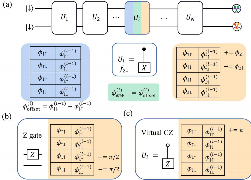
图 5.14 非共振哈密顿相位误差补偿程序。(a) 对线路中的每一个门，首先计算在相关状态下累积的相位的相位误差补偿表（如蓝色区域所示），然后减去脉冲相位的微波偏移量（如绿色区域所示）。最后，将由脉冲引起的相位误差加到相位误差补偿表中，用于获得以下脉冲的偏移量（如黄区域所示）。(b) 线路的虚 Z 门在表格统计中所产生的相位累积。(c) 线路的虚 CZ 门在表格统计中所产生的相位累积。
