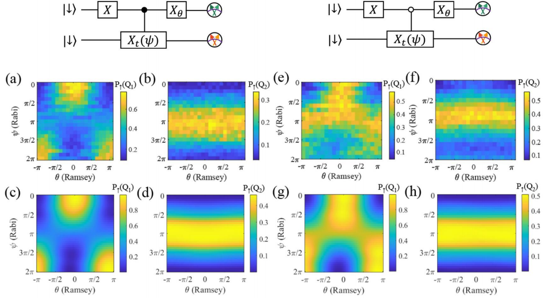
图 5.22 在 CNOT 门中未对控制比特 \lambda 子空间进行相位矫正的测试与模拟。(a,b) 使用上方的量子线路图进行测试, Q_2 作为受控比特进行 CROT 的旋转 X_t(\psi) , 受控旋转 f_{2\downarrow} 的角度为 \psi ; 同时在这个序列中对控制比特 Q_1 上用拉姆齐序列进行相位测试。。(a) 为 Q_1 的测试结果, (b) 为 Q_2 的测试结果。(c,d) 根据矩阵的演化, 分别给出了对应 (a,b) 图的计算结果。(e,f) 使用上方的量子线路图进行测试, 将受控旋转改为 f_{2\uparrow} , 进行相同的实验。(g,h) 根据矩阵的演化, 分别给出了对应 (e,f) 图的计算结果。
