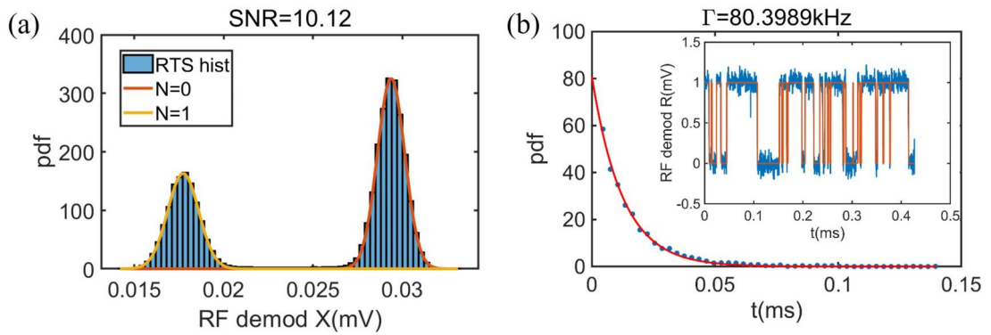
图 6.16 Ge/SiGe 量子点结构中的射频探测结果。(a) 解调反射信号的 X 分量分布，积分时间为 t_{int}=100 ns，信噪比为 10.12，橙色和黄色条包络别表示在检测到的量子点中电子数为 0 和 1 时，SET 反射的 V_Q 电压分布。(b) 插图中时间轨迹所获得时间的概率密度，通过射频检测获得的平均 RTS 调谐率高达 80.4 kHz。
