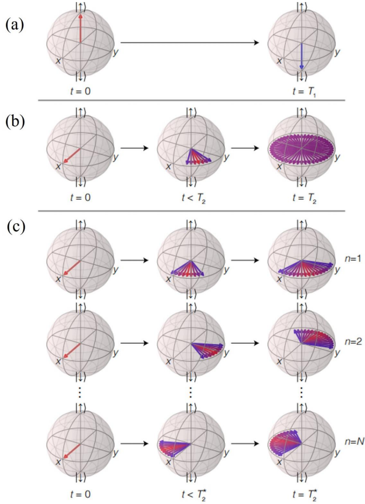
图 2.4 弛豫与退相干。(a) 量子比特激发态弛豫到基态，具有特征时间尺度 T_1 。(b) 自旋去相，初始自旋沿 x 轴，在时间 T_2 后，自旋完全失去了相位相干性，有任意的相位角 \phi 。(c) 自由演化时间 T_2^* 对应于自旋系综。这是 N 次单发测量下退相位的平均结果，由系综所经历的涨落引起。
