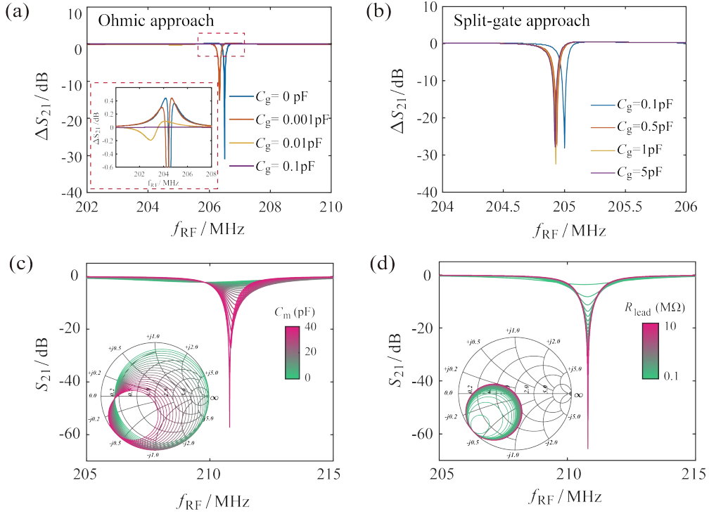
图 6.6 对两种结构的射频模拟。(a) 在欧姆方法中，测量的信号幅度是射频频率 f_{\text{RF}} 的函数，不同颜色的线条代表不同的 C_g 值。当 C_g 为 0 pF 时，反射信号在某一频率处出现 dip，称为谐振频率 f_{\text{res}} ，表明此点实现了阻抗匹配。随着 C_g 的增加，dip 迅速消失，表明在此方法中较高的 C_g 值导致信号泄漏。(b) 在劈裂栅极方法中， C_g 是耦合通道而非泄漏通道。阻抗匹配对 C_g 的值非常宽容，可以在 0.1 pF 到 5 pF 之间实现阻抗匹配。根据同一样品的直流测量结果，我们选择了 625 k \Omega 和 500 k \Omega 的两种不同阻抗。(c) 在劈裂栅极结构的模拟中，研究了 C_m 的调整以实现阻抗匹配。通过线性调整 C_m ，系统耦合可以从过耦合状态（绿色）过渡到阻抗匹配（粉色）。插图：通过改变 C_m ，可以调整相应的史密斯圆通过原点。(d) 在我们的模拟中，我们为 R_{\text{lead}} 生成了 121 个对数间隔的数据点，以探索阻抗匹配的条件。只有当 R_{\text{lead}} 足够大 ( R_{\text{lead}} > 10 \cdot R_{\text{QD}} , R_{\text{QD}} = 625 \text{ k}\Omega ) 时，才能有效抑制来自引线栅极方向的射频泄漏。有关详细的参数范围和相应的二维图形，请参阅补充材料的模拟部分。图片来源于文献 [200] 。
