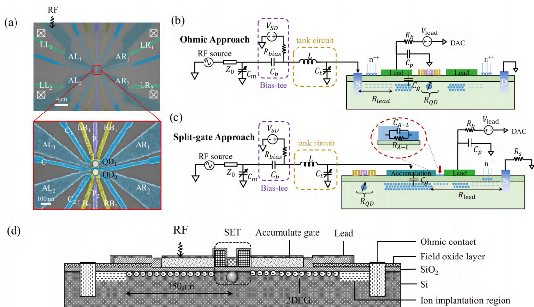
图 6.5 Si-MOS 中的劈裂栅极结构。(a) Si-MOS 器件的伪彩色 SEM 图像。为了便于相互检测，我们设计了一个对称结构。下标 1 和 2 表示上下两侧具有完全相同的结构。两个量子点 QD_1 和 QD_2 分别位于栅极 P_1 和 P_2 下方（紫色），并在栅极 LB_1 、 LB_2 、 RB_1 和 RB_2 下方形成势垒（黄色）。限制栅极 C_1 、 C_2 和 C 用于控制量子点的横向尺寸。先前的大引线栅极被分为两层：引线栅极（ LL 和 LR ）和劈裂累积栅极（ AL 和 AR ）。在测试中，我们利用上方的量子点作为 SET 来检测来自下方量子点的信号，射频电路连接到 AL1 栅极。(b) 欧姆方法。在欧姆设计中，偏置三通（紫色虚线）和储能电路（黄色虚线）在 PCB 上实现。 R_{lead} 表示累积在引线栅极下方的二维电子气的电阻，它阻止了射频信号的泄露。 C_g 表示引线栅极与二维电子气之间的电容，它导致射频信号的泄露。 C_p 是来自键合线和累积栅极到 PCB 接地平面的寄生电容。 R_b 是 PCB 上的电阻，用于防止射频信号泄漏到直流线路中。匹配电容 C_m 可以将射频电路与高阻抗的 SET 匹配。 n^{++} 是离子注入区域。(c) 劈裂栅极方法。射频信号施加到累积栅极。引线栅极和累积栅极被分成两部分，减少它们的重叠以最小化电阻 R_{A-L} 和电容 C_{A-L} 。重叠区域的长度为 0.1\text{ }\mu\text{m} ，宽度为 0.3\text{ }\mu\text{m} 。为方便起见， R_{A-L} 包含在引线栅极至欧姆接触电阻 R_{lead} 中。(d) 劈裂栅结构的横截面图。离子注入区位于距 SET 中心 150\text{ }\mu\text{m} 处。 \text{Al}_2\text{O}_3 层厚度为 30\text{ nm} ，芯片中心 100\text{ }\mu\text{m}\times 100\text{ }\mu\text{m} 区域中的氧化铝已被蚀刻掉。图片来源于网络文献 [200] 。
