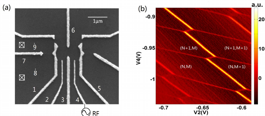
图 3.1 (a)Ti/Au 电极 1-6 定义了一个典型的双量子点结构。电极 7 称为 QPC 电极，用来调节 QPC 通道。电极 2 和 4 称为 plunge gate。电极 1 和 5 称为 barrier gate。电极 3 称为 middle gate。QPC 电通通过源极 8 流向漏极 9(数字上方加一点表示连接到欧姆接触)。
