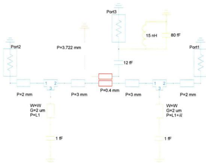
图 3.5 Purcell 滤波器的仿真电路图。黄色部分表示量子比特，橙色表示读取谐振腔，红色部分是谐振腔与读取总线的耦合部分，绿色部分表示滤波器。仿真使用的衬底为理想的本征硅，P 表示各段传输线的长度，G 表示传输线中央导带线距离地平面的距离，对于所有传输线 G = 2 \mu\text{m} ，W 表示滤波器的中央导带线宽，对于读取总线以及谐振腔，中央导带线宽为 3.2 \mu\text{m} ，从而满足 50 \Omega 的阻抗匹配条件。
