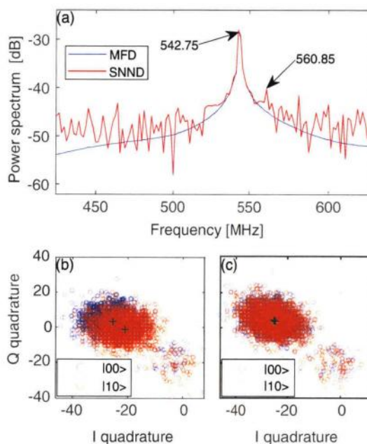
图 5.12 (a) 解调系数的功率谱，蓝线代表 MFD，在这条线上只有一个关于目标比特中频频率的信号峰。红色代表 SNND，可以看到，除了目标比特自身的频率信号峰之外，还有一个信号峰的频率刚好等于 Q3 的中频频率。(b) 使用 MFD 的解调系数获得的 IQ 圆斑以及 (c) 使用 SNND 的解调系数获得的 IQ 圆斑，其中的态表示 |Q3, Q4\rangle ，黑色的交叉交叉记号代表每个圆斑的中心点，可以发现采用 MFD 方案时，随着 Q3 状态的变化，圆斑发生了偏移，而在 SNND 中则没有这种现象。
