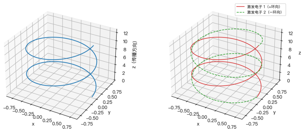
模型 A：单激发电子圆柱螺旋 (轴向直线速度 = 光速)
