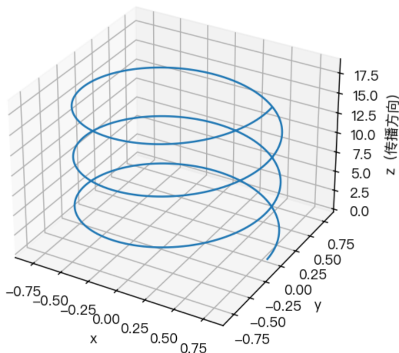
图 6. 数条数：光子螺旋的每圈 = 一个频率周期 = 角动量 h ； E = h \cdot f = 每圈角动量 \times 每秒圈数。
