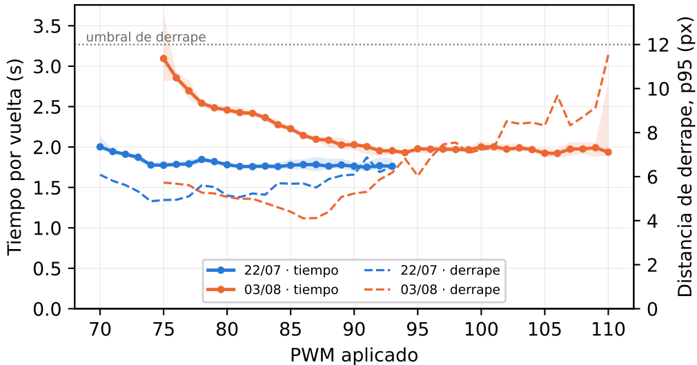
Coche azul: tiempo por vuelta y derrape frente al PWM
