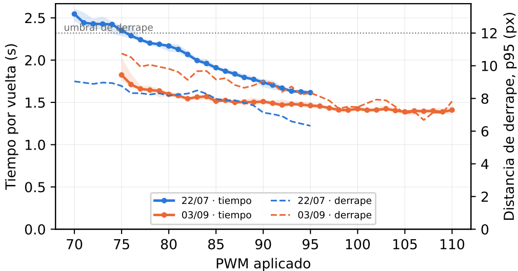
Coche rojo: tiempo por vuelta y derrape frente al PWM
