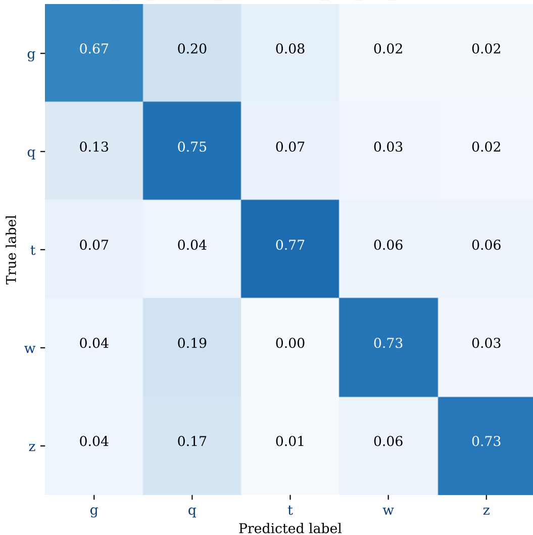
y_dut_QKeras_acc=0.7298_VU_DA_bitfile.npy
