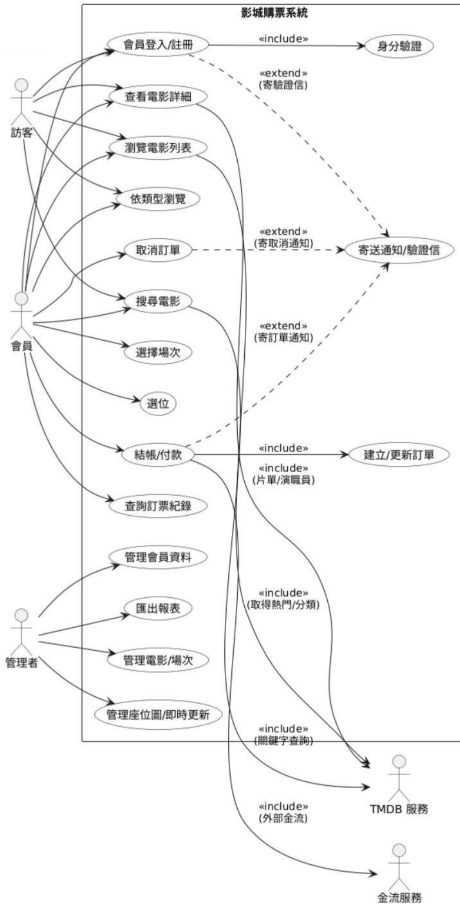
影城購票系統 - 用例圖
