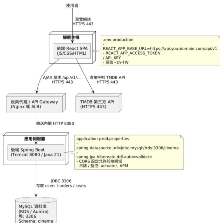
圖3-1 系統架構圖
