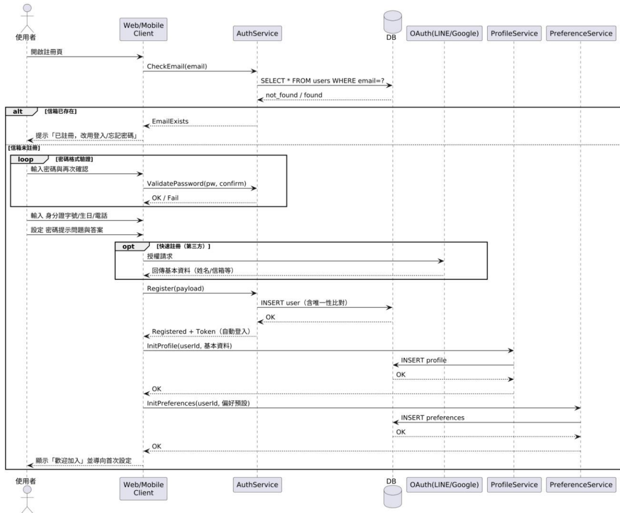
註冊流程—循序圖
