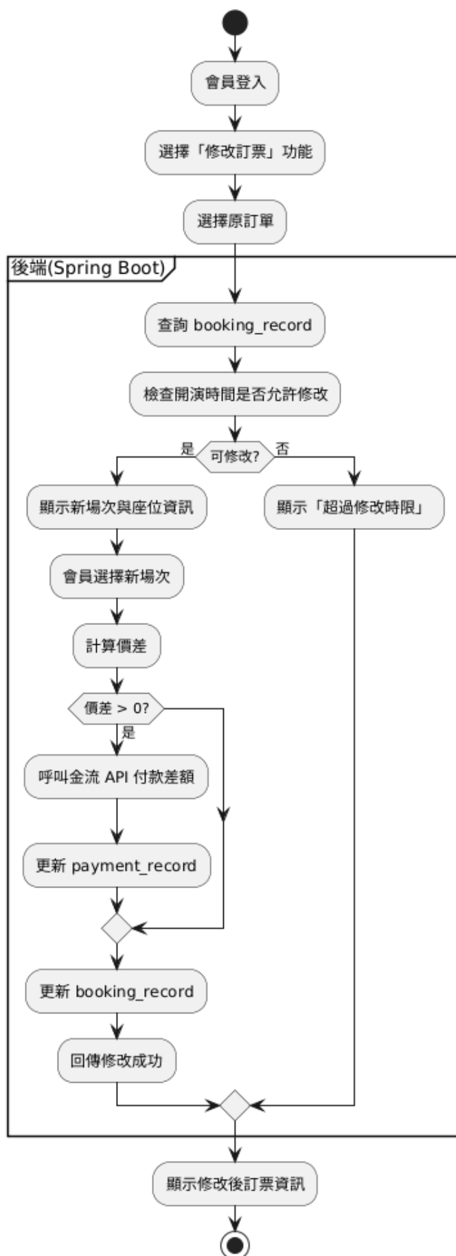
修改訂票子系統活動圖
