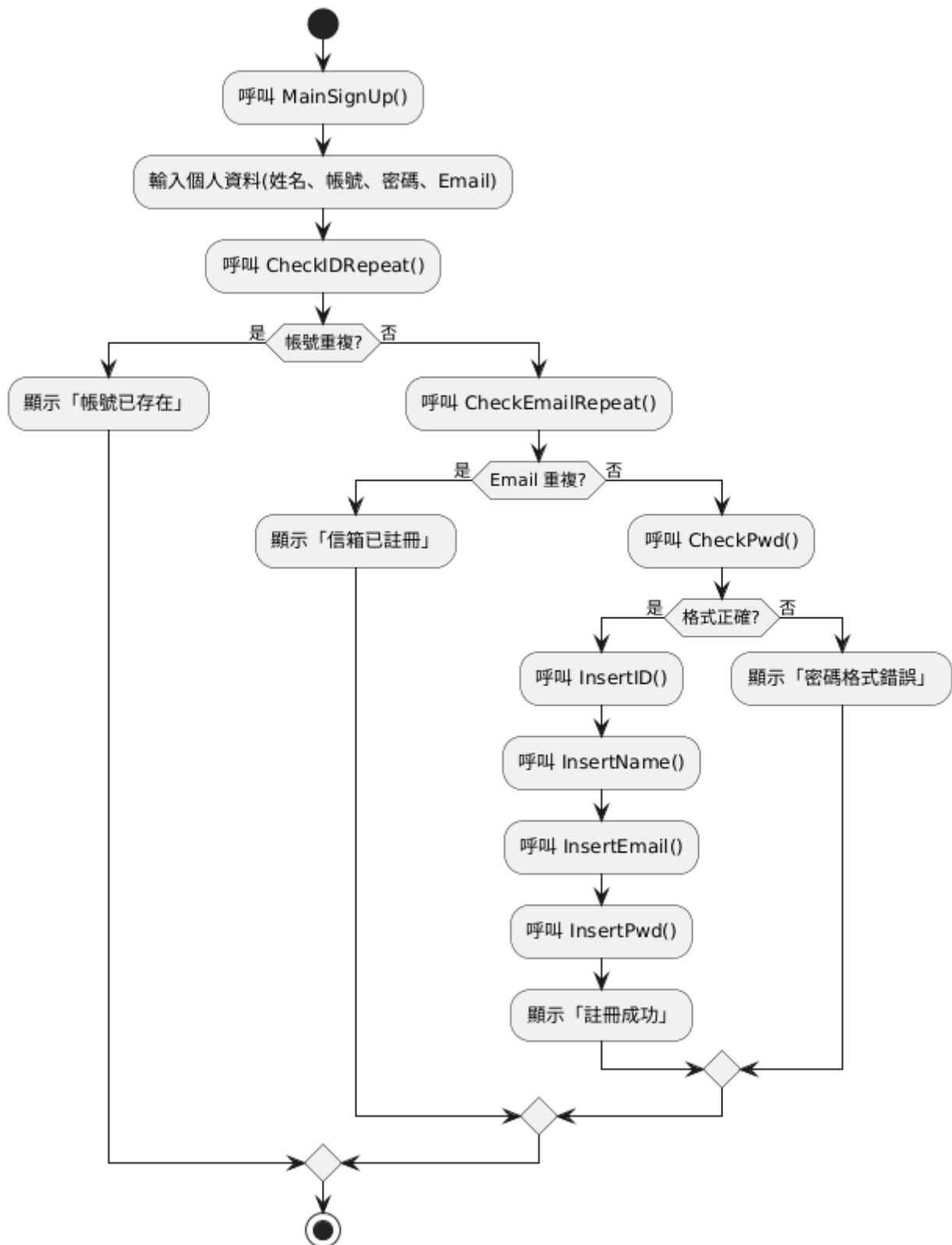
S1 MainSignUp() 流程圖
