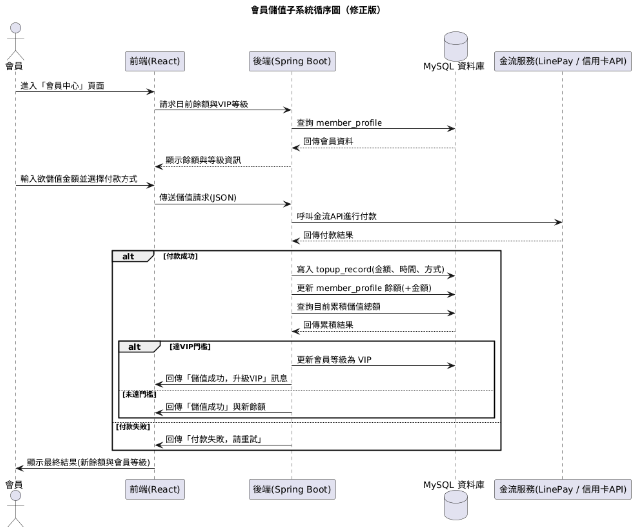
圖 2.2.2-6 會員儲值子系統循序圖
