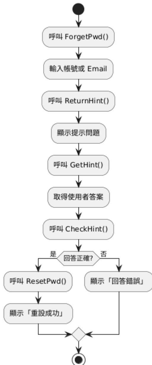
L6 ForgetPwd() 流程圖
