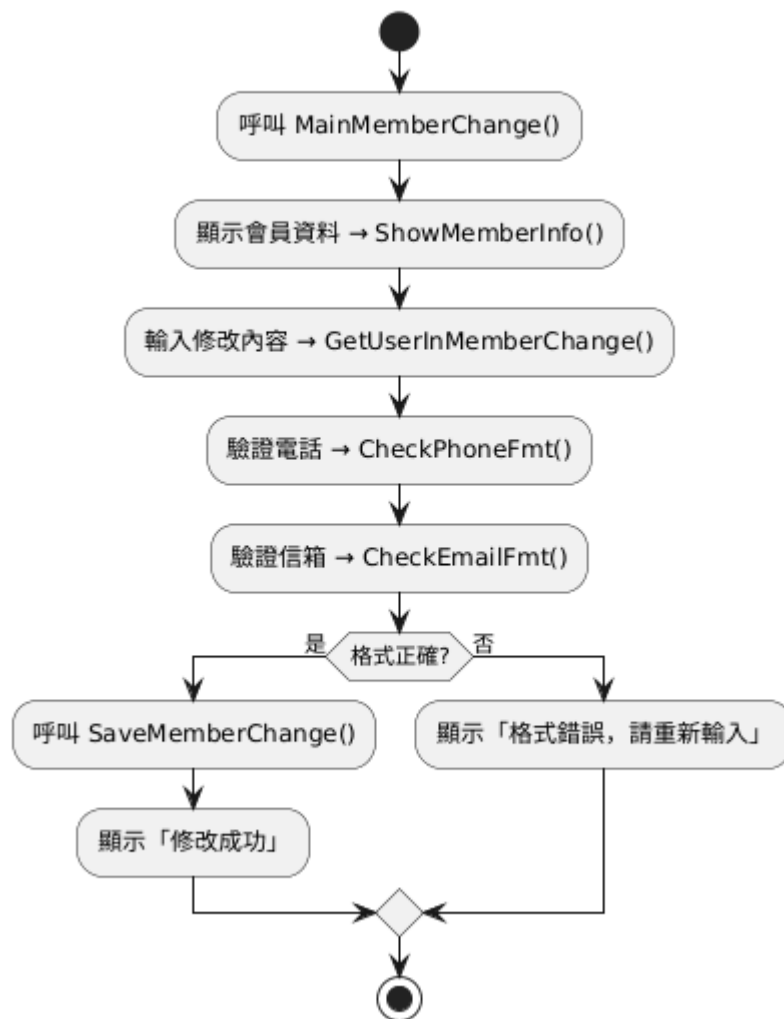
M1 MainMemberChange() 流程圖
