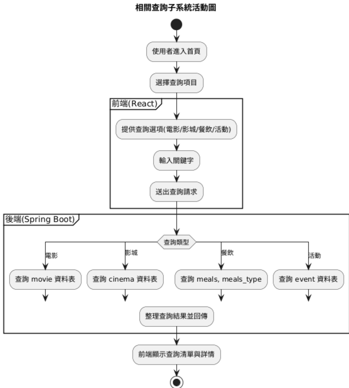
圖 2.2.1-8 相關查詢子系統活動圖
