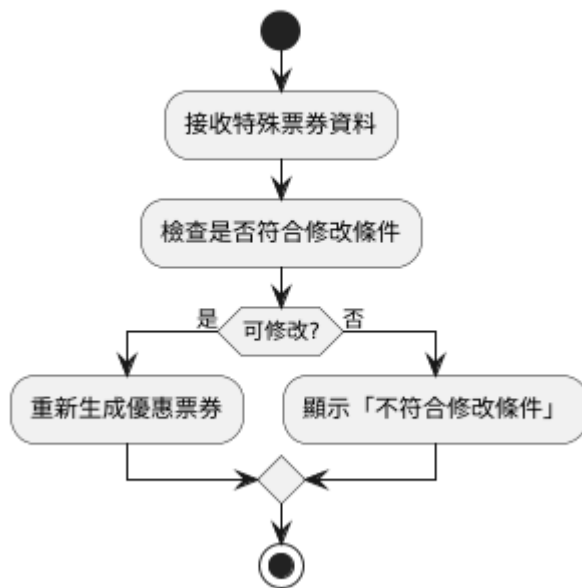
C7 ChangeForSpecial() 流程圖
