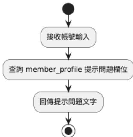
L7 ReturnHint() 流程圖
