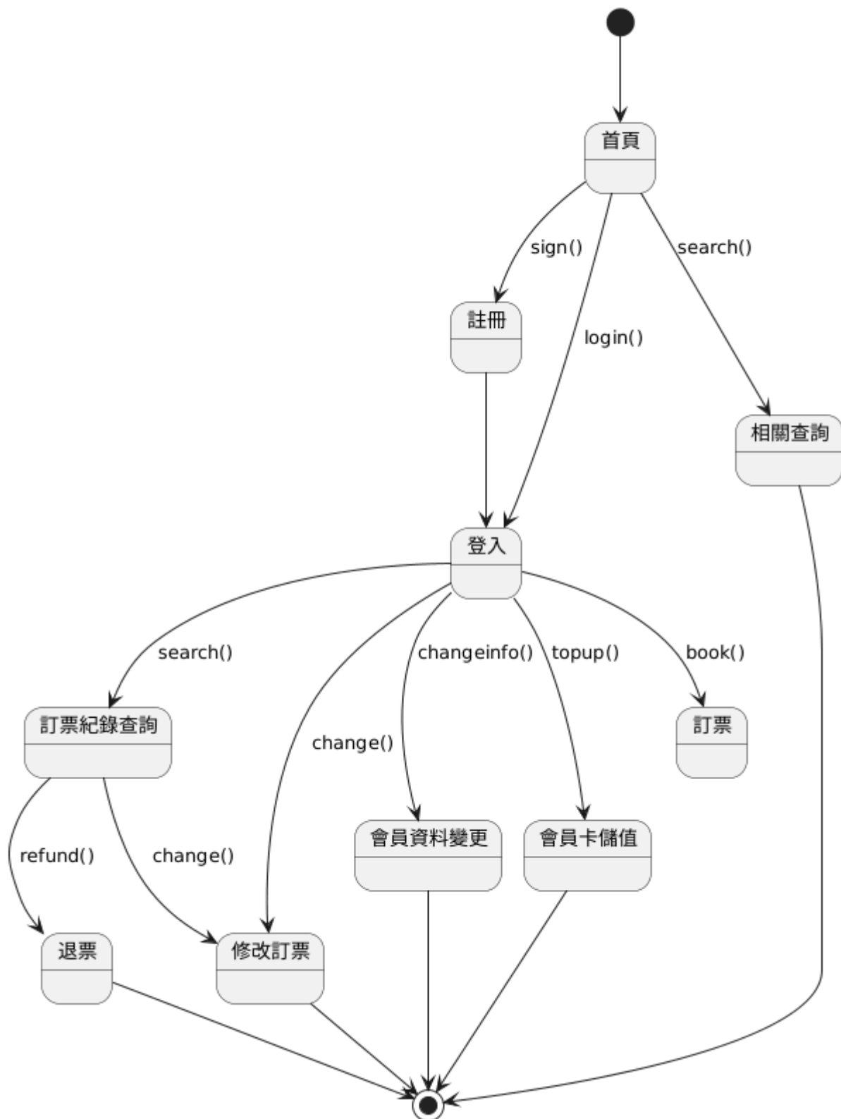
威泰影城售票系統 - 狀態圖
