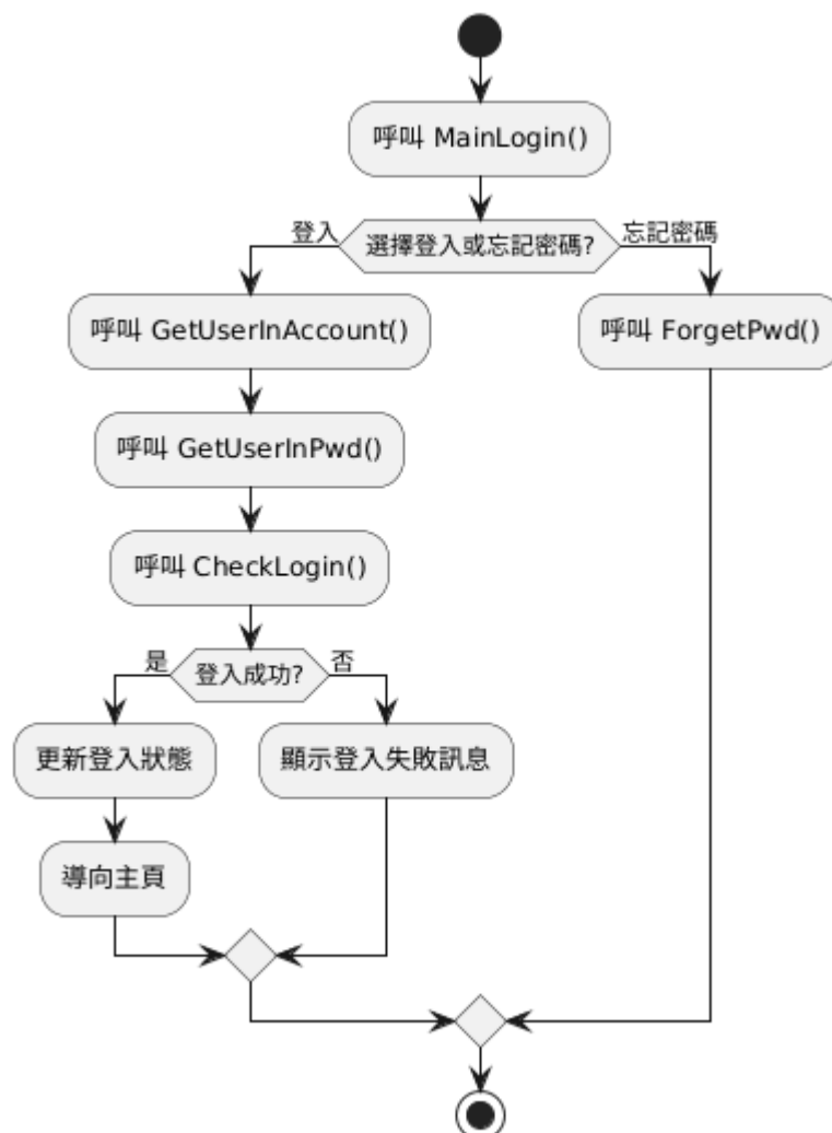
L1 MainLogin() 流程圖
