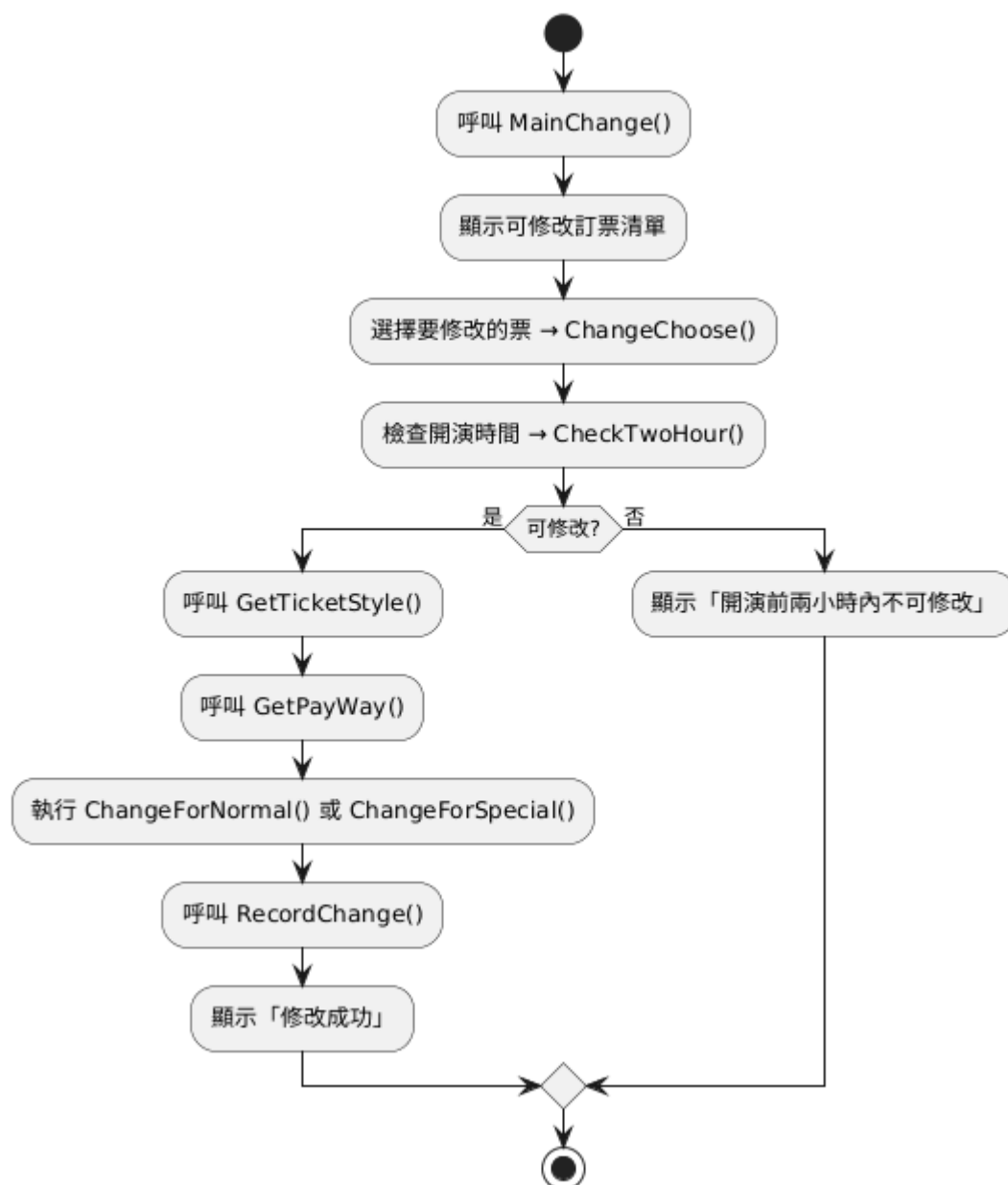
C1 MainChange() 流程圖
