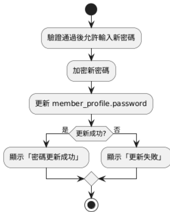
L10 ResetPwd() 流程圖
