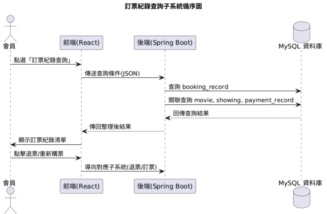
圖 2.2.2-4 訂票紀錄查詢子系統循序圖
