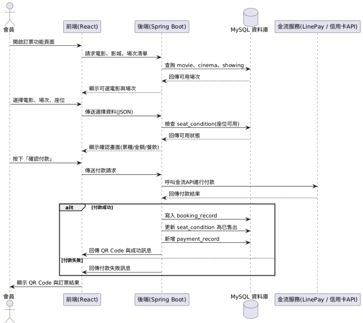
訂票子系統循序圖 (修正版)
