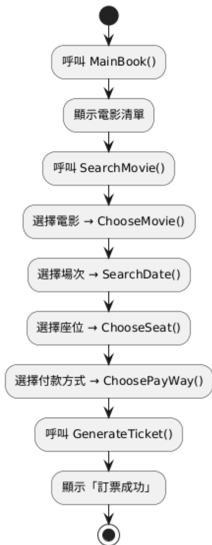
B1 MainBook() 流程圖
