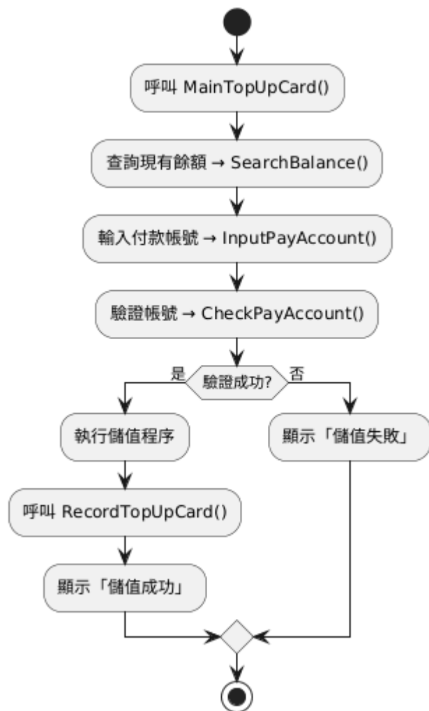
T1 MainTopUpCard() 流程圖
