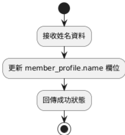
S6 InsertName() 流程圖
