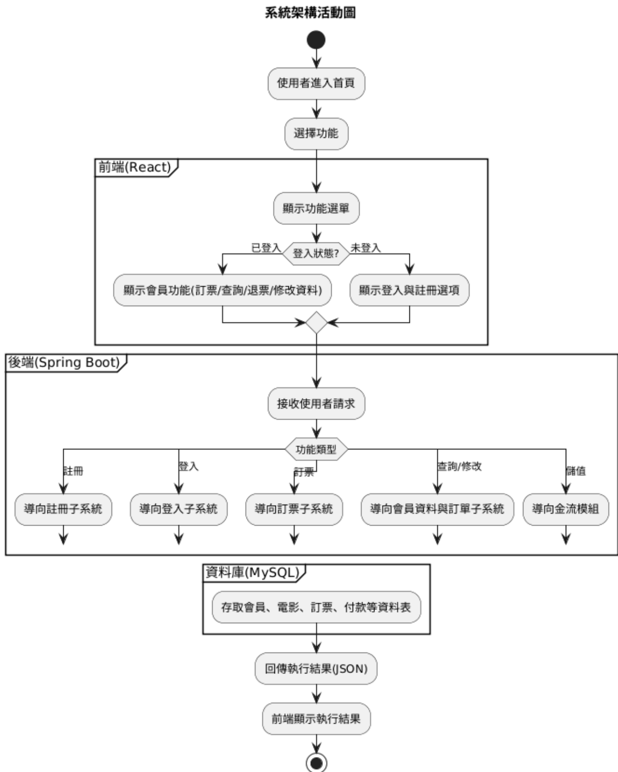
圖 2.2.1-1 系統架構活動圖
