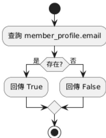
S8 CheckEmailRepeat() 流程圖
