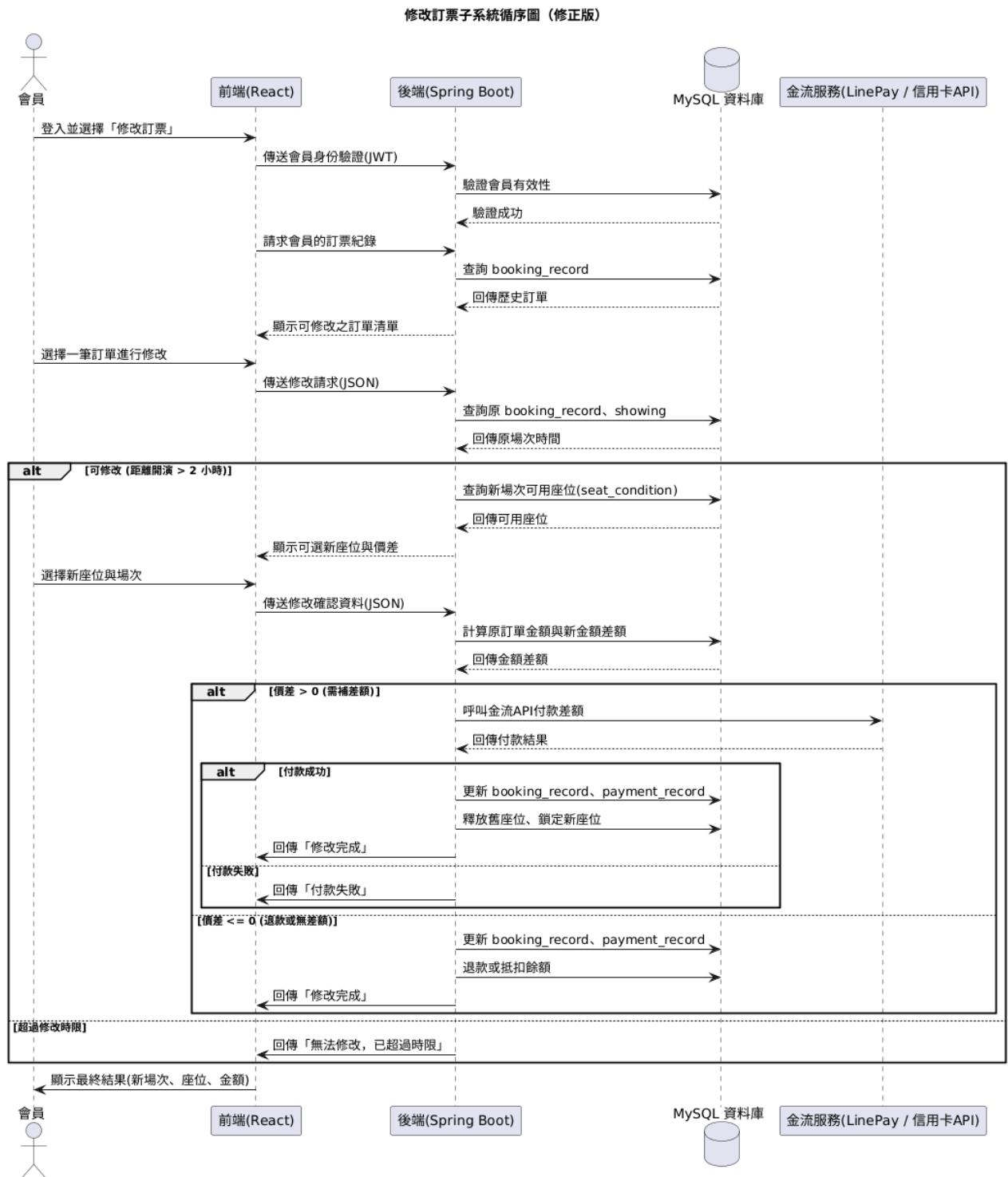
圖 2.2.2-8 修改訂票子系統循序圖
