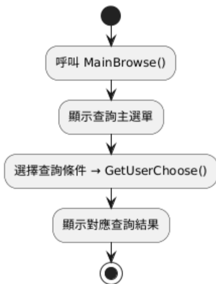
Br1 MainBrowse() 流程圖
