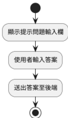
L8 GetHint() 流程圖
