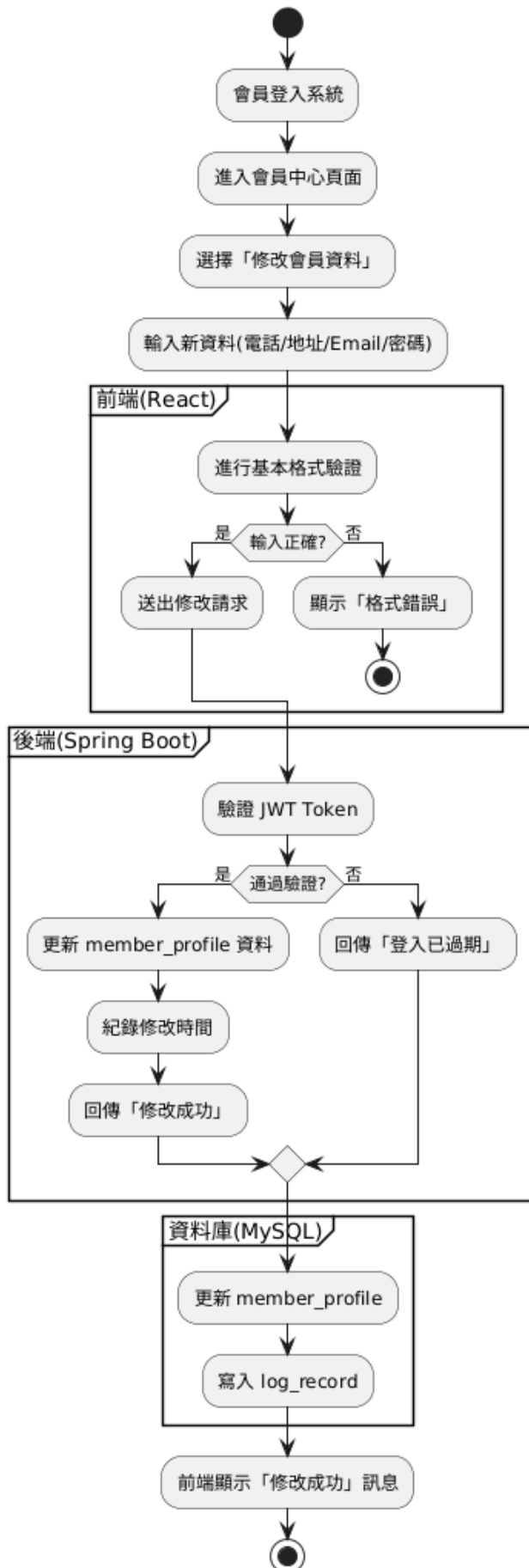
會員變更資料子系統活動圖
