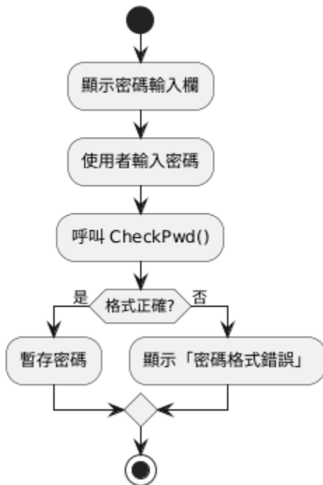
S10 GetPwd() 流程圖
