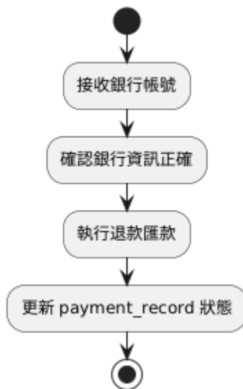
R6 RefundToBank() 流程圖
