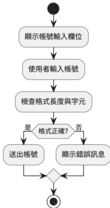
S2 GetID() 流程圖
