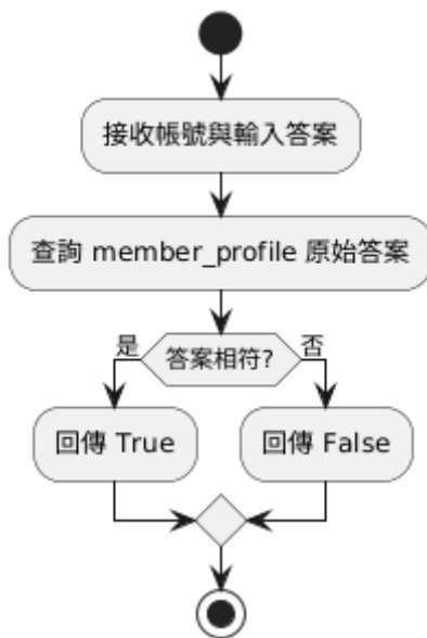
L9 CheckHint() 流程圖
