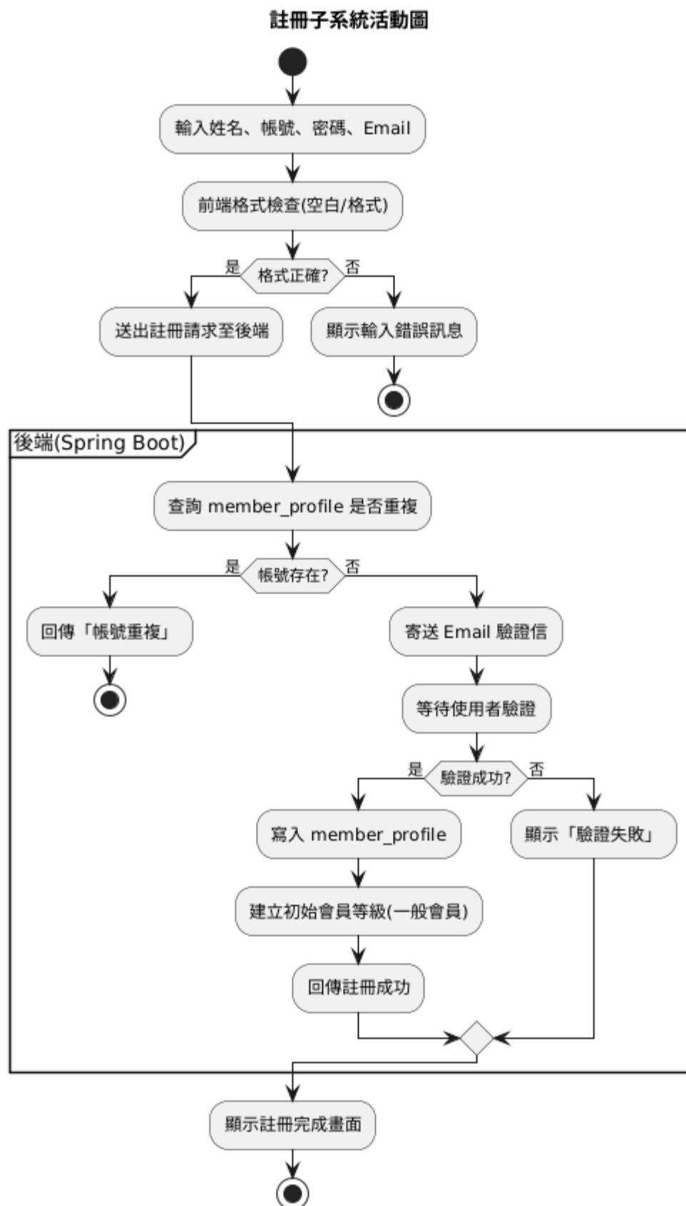
圖 2.2.1-2 註冊子系統活動圖
