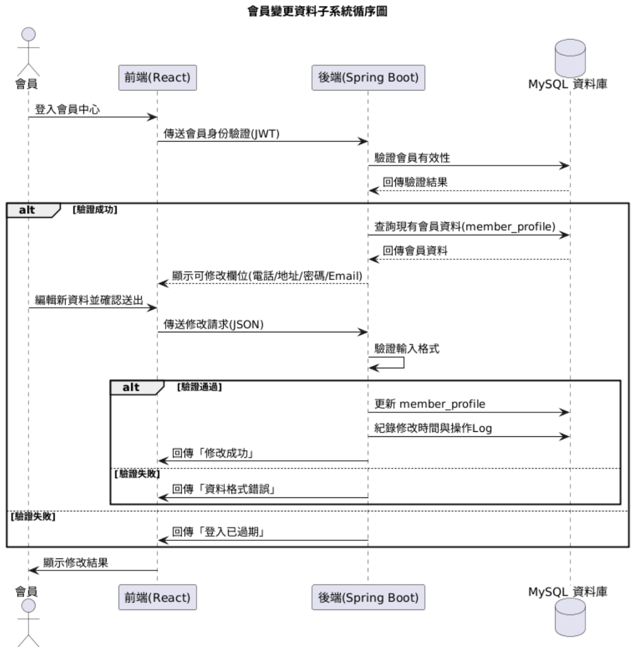
圖 2.2.2-3 會員資料變更子系統循序圖
