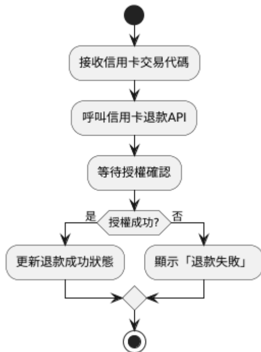
R7 RefundToCard() 流程圖
