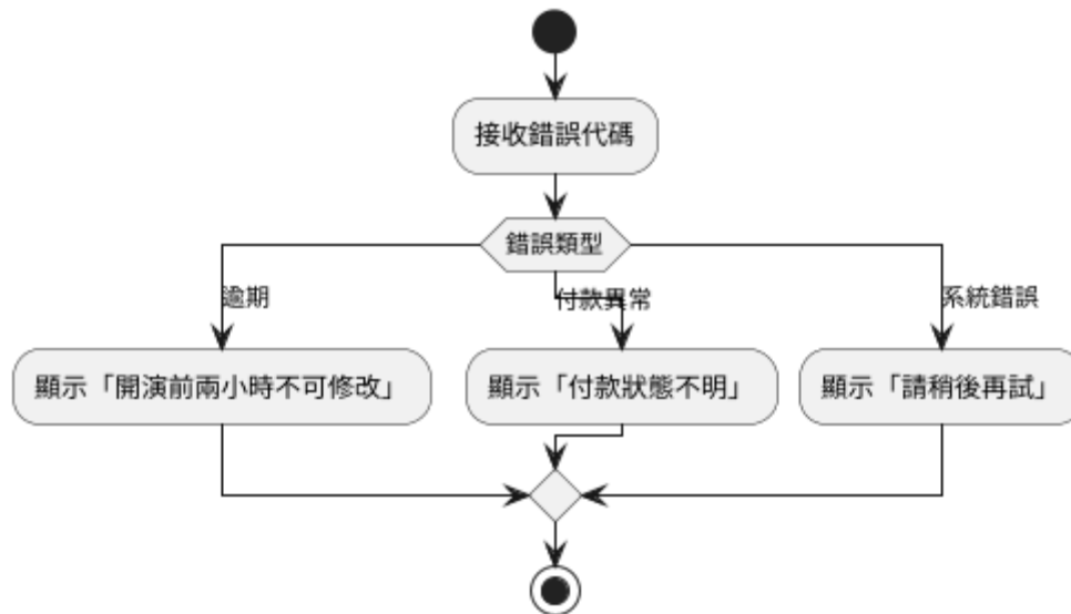
C11 DisplayChangeError() 流程圖
