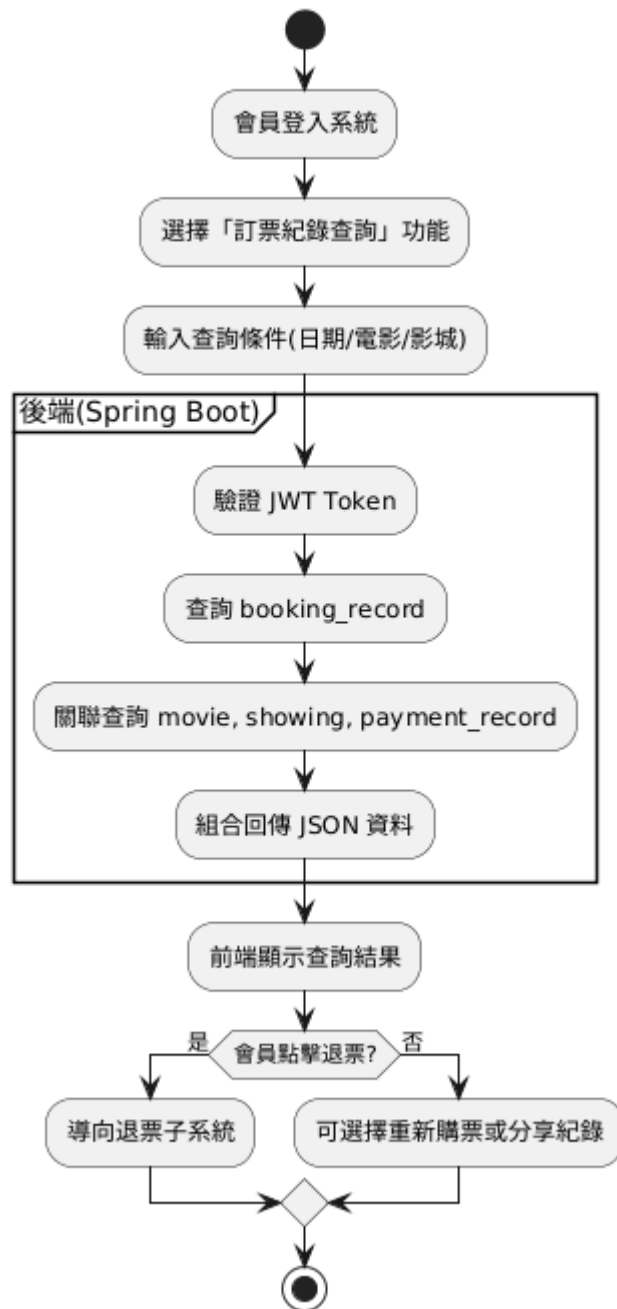
訂票紀錄查詢子系統活動圖
