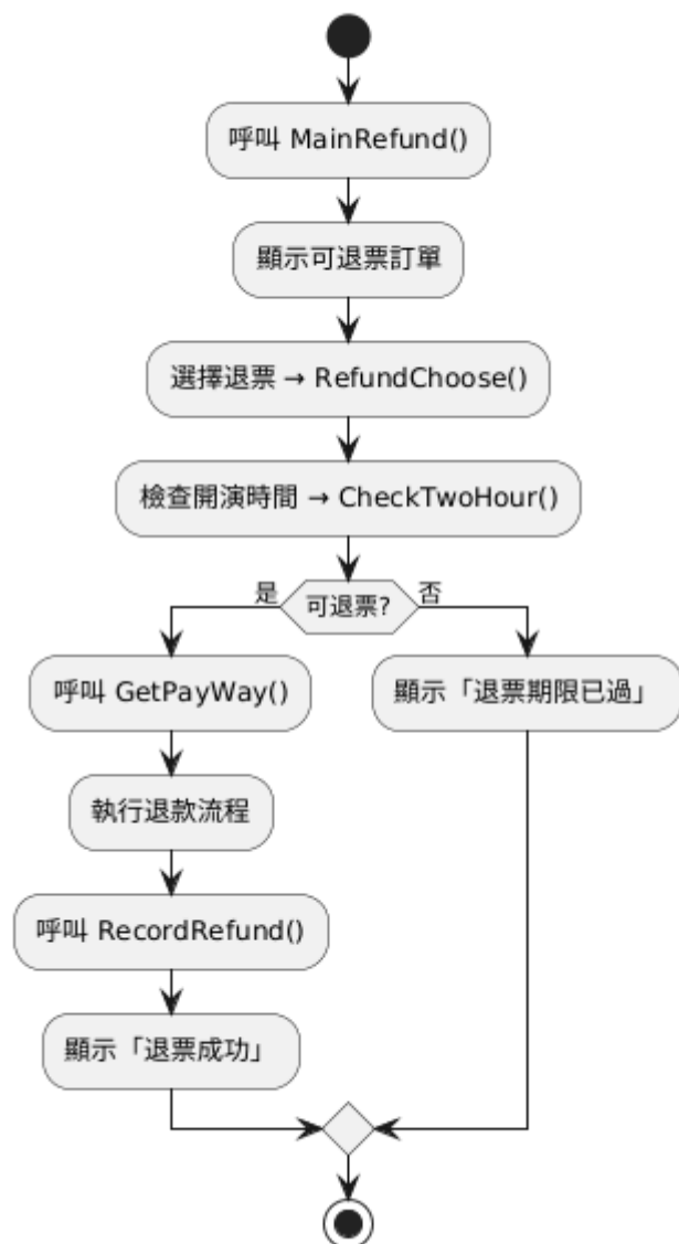
R1 MainRefund() 流程圖
