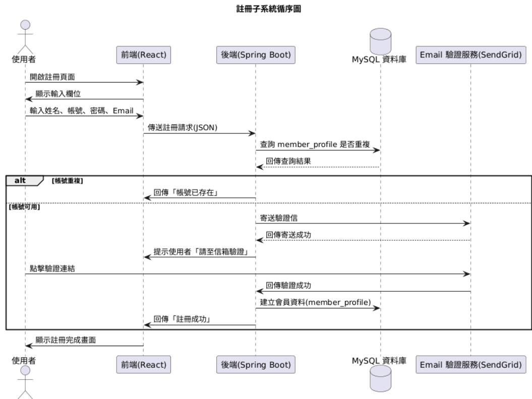
圖 2.2.2-1 註冊子系統循序圖
