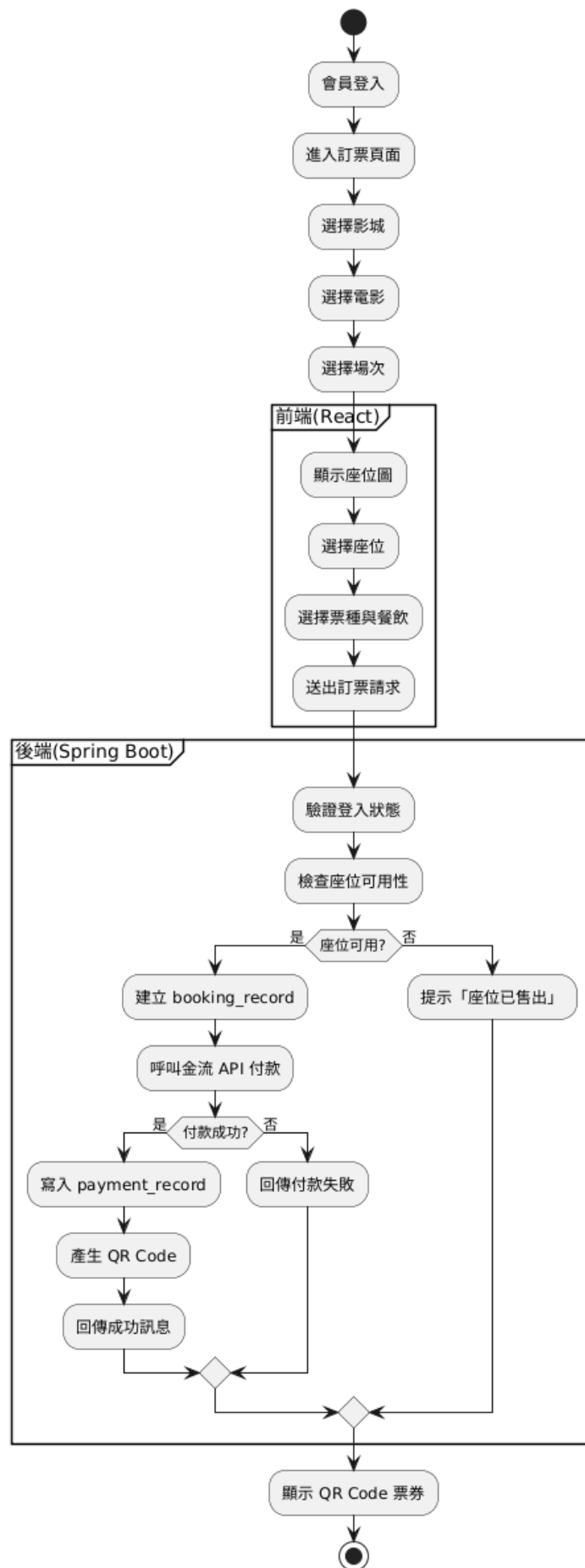
訂票子系統活動圖
