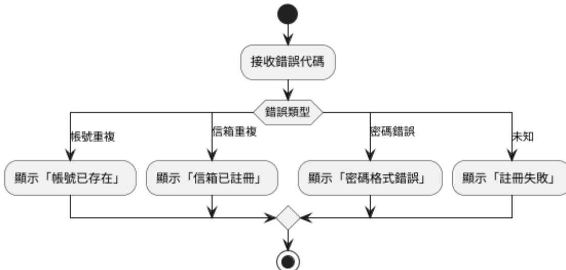
S13 ShowRegError() 流程圖
