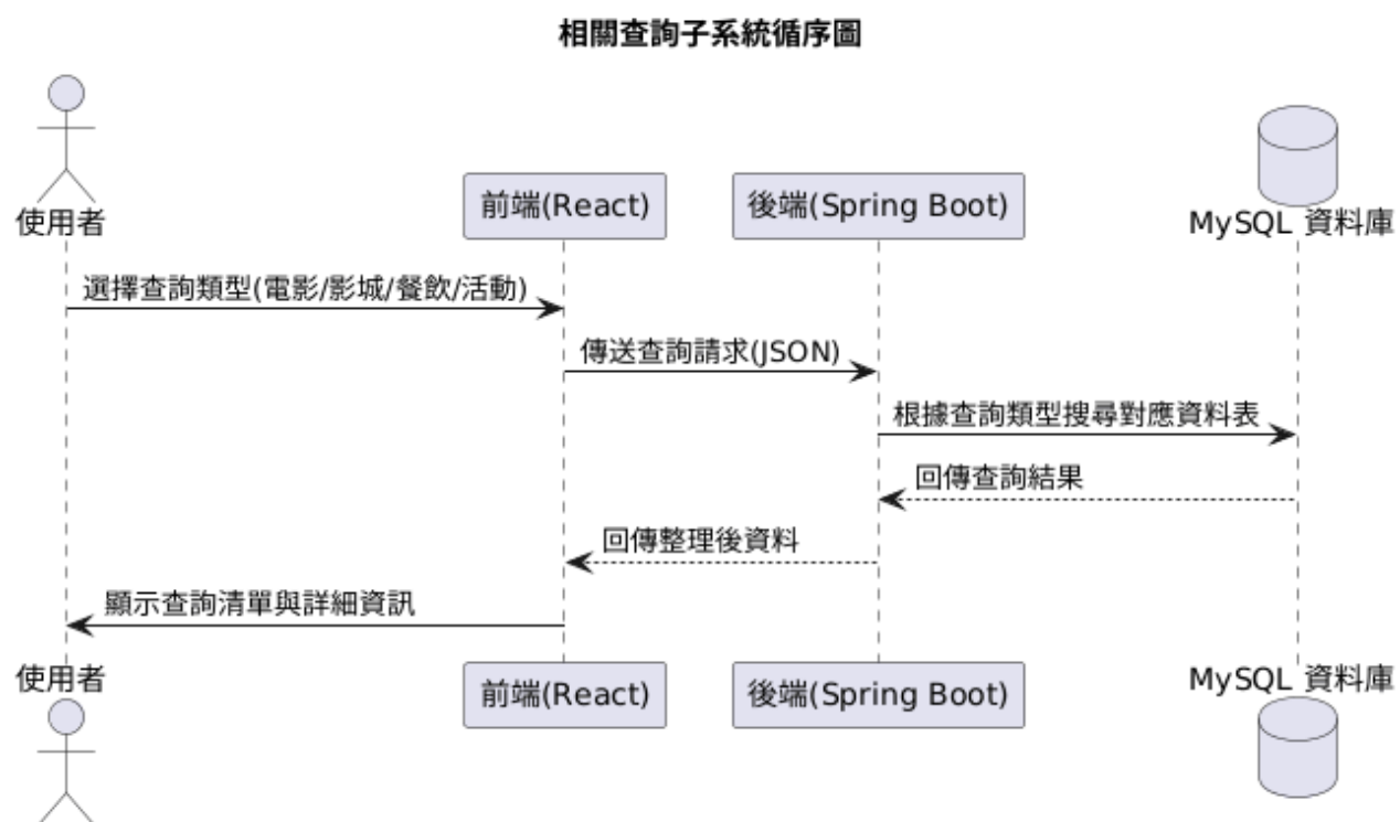
圖 2.2.2-7 相關查詢子系統循序圖
