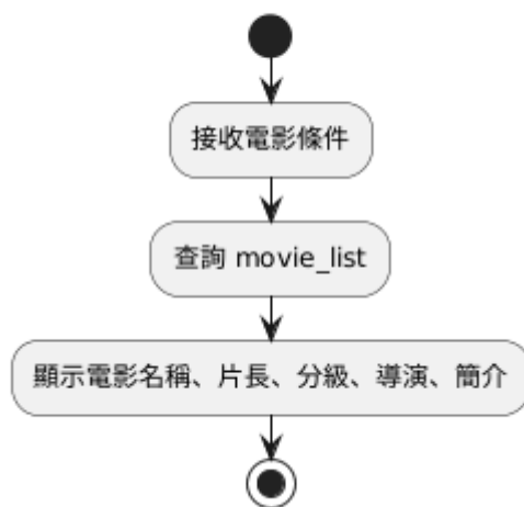
Br10 DisplayMovie() 流程圖
