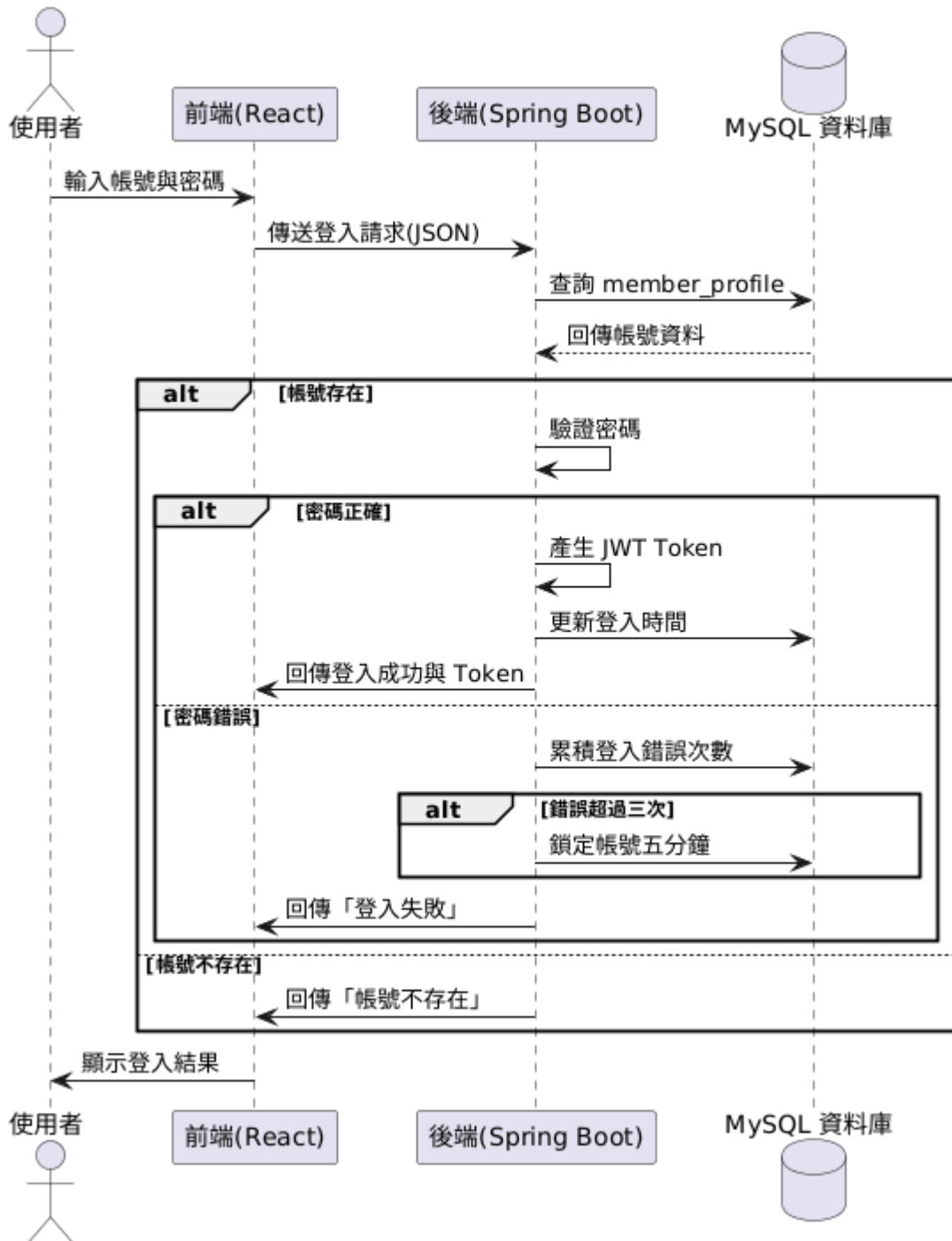
登入子系統循序圖
