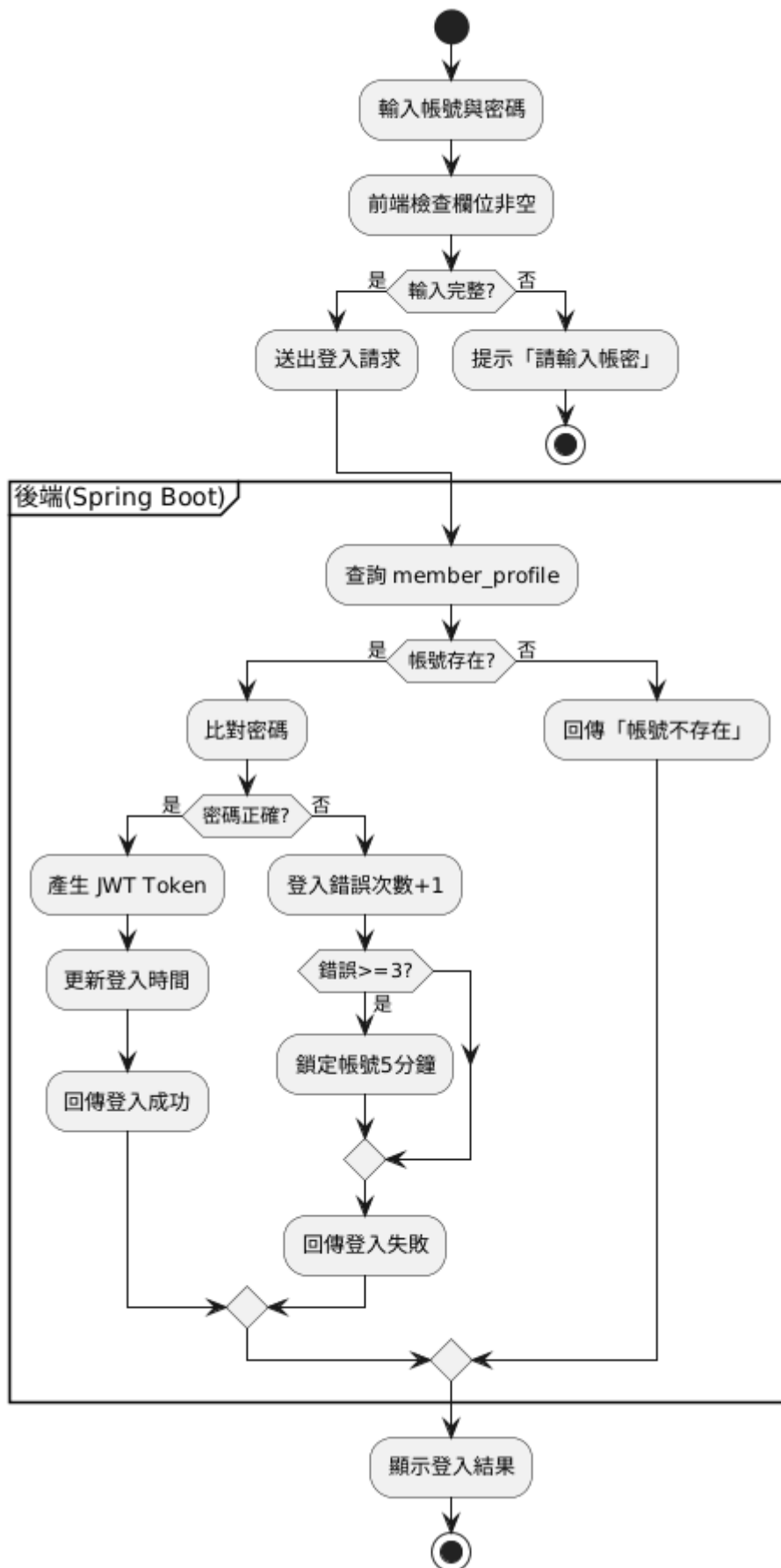
登入子系統活動圖
