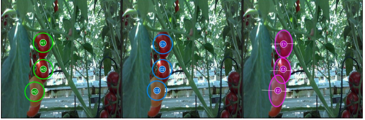
Figura 6: Inversione delle priorità di picking su un grappolo verticale. (a) Scelta umana di riferimento ( H_1, H_2, H_3 ). (b) Baseline BBox ( C_1, C_2, C_3 ), che sceglie per errore il frutto centrale ( C_2 ) prima di quello in basso ( C_3 ). (c) Planner ellittico ( E_1, E_2, E_3 ), che si adatta alla forma allungata del pomodoro inferiore assegnandogli il Rank 2 ( E_2 ), rispecchiando esattamente la scelta dell'operatore umano.
