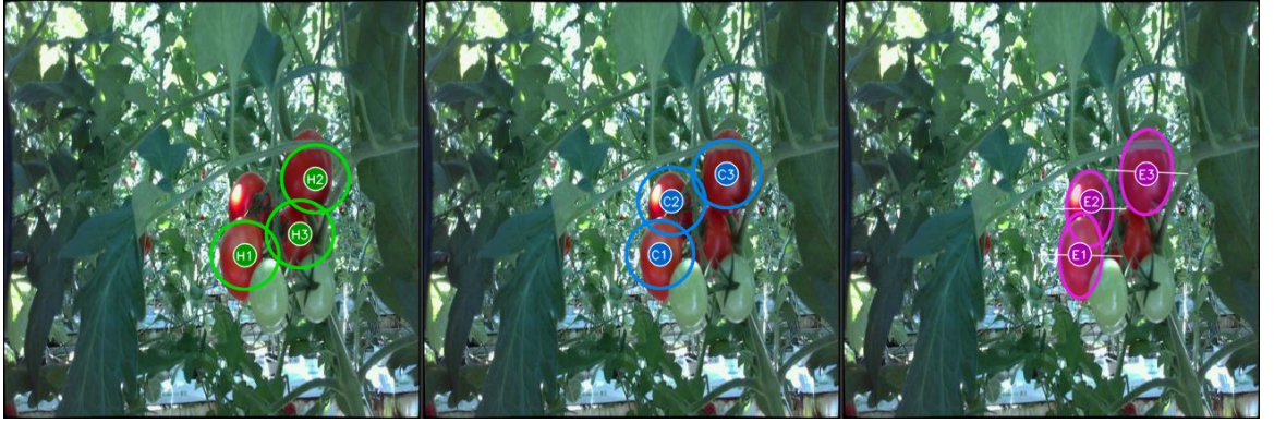
Figura 4: Dinamica di sblocco su un grappolo denso con occlusioni multiple. (a) Ground Truth umano ( H_1, H_2, H_3 ); (b) Baseline a bounding box ( C_1, C_2, C_3 ); (c) Planner ellittico ( E_1, E_2, E_3 ), in cui la rimozione di E_1 sblocca E_2 assegnandogli il bonus \beta_{\text{unlock}} = 1.20 e consentendogli di scavalcare il frutto laterale E_3 .
