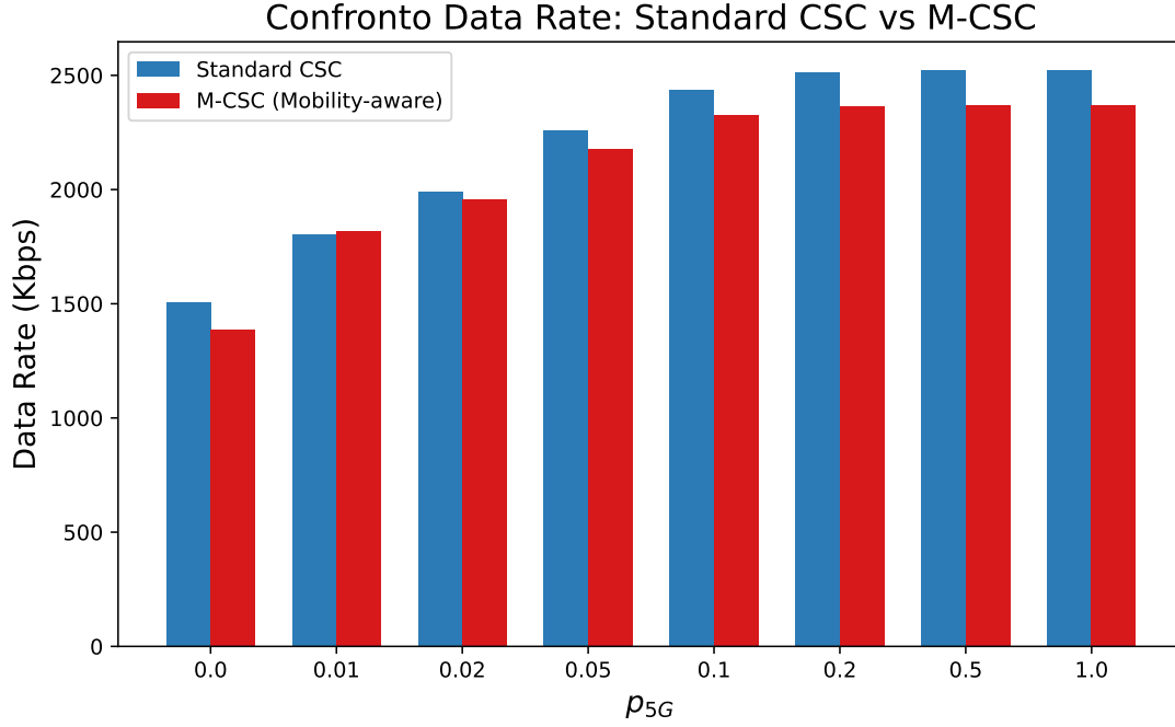
Figura 5.7: Confronto del data rate medio ottenuto dal metodo CSC standard e dal metodo M-CSC al variare della probabilità di disponibilità della rete 5G. La frequenza di aggiornamento presa in considerazione è f = 0.2 Hz.
