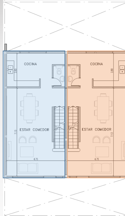
Planta 1° piso
