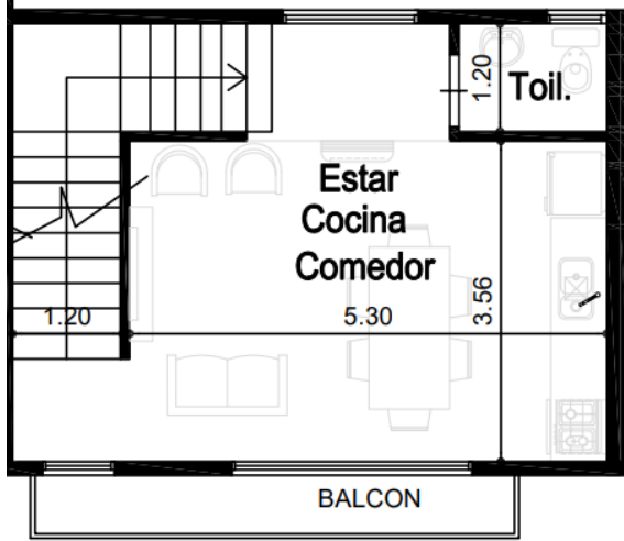
1° PISO
