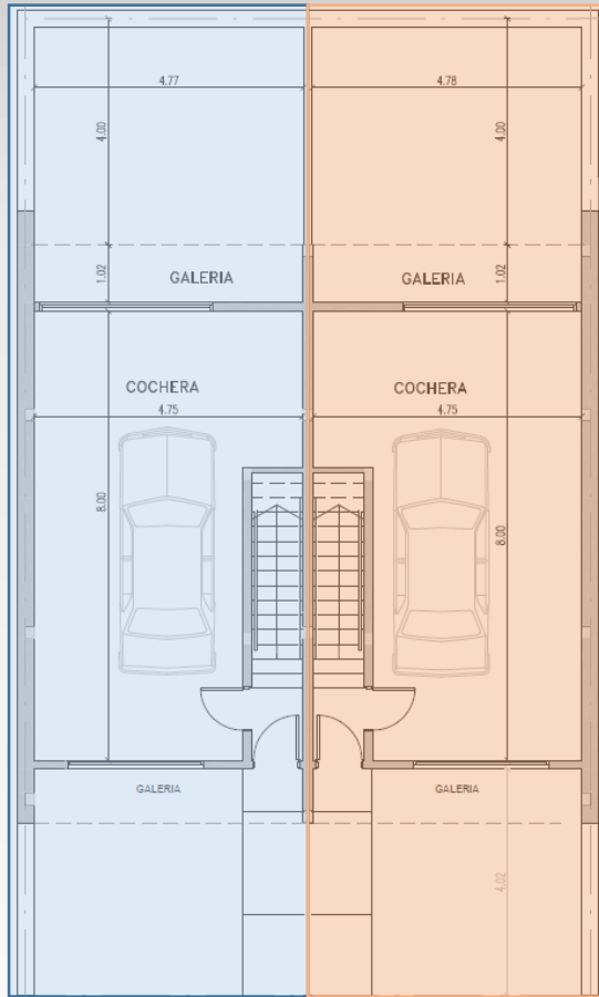
Planta Baja
