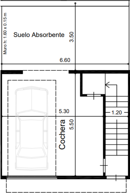
PLANTA BAJA
