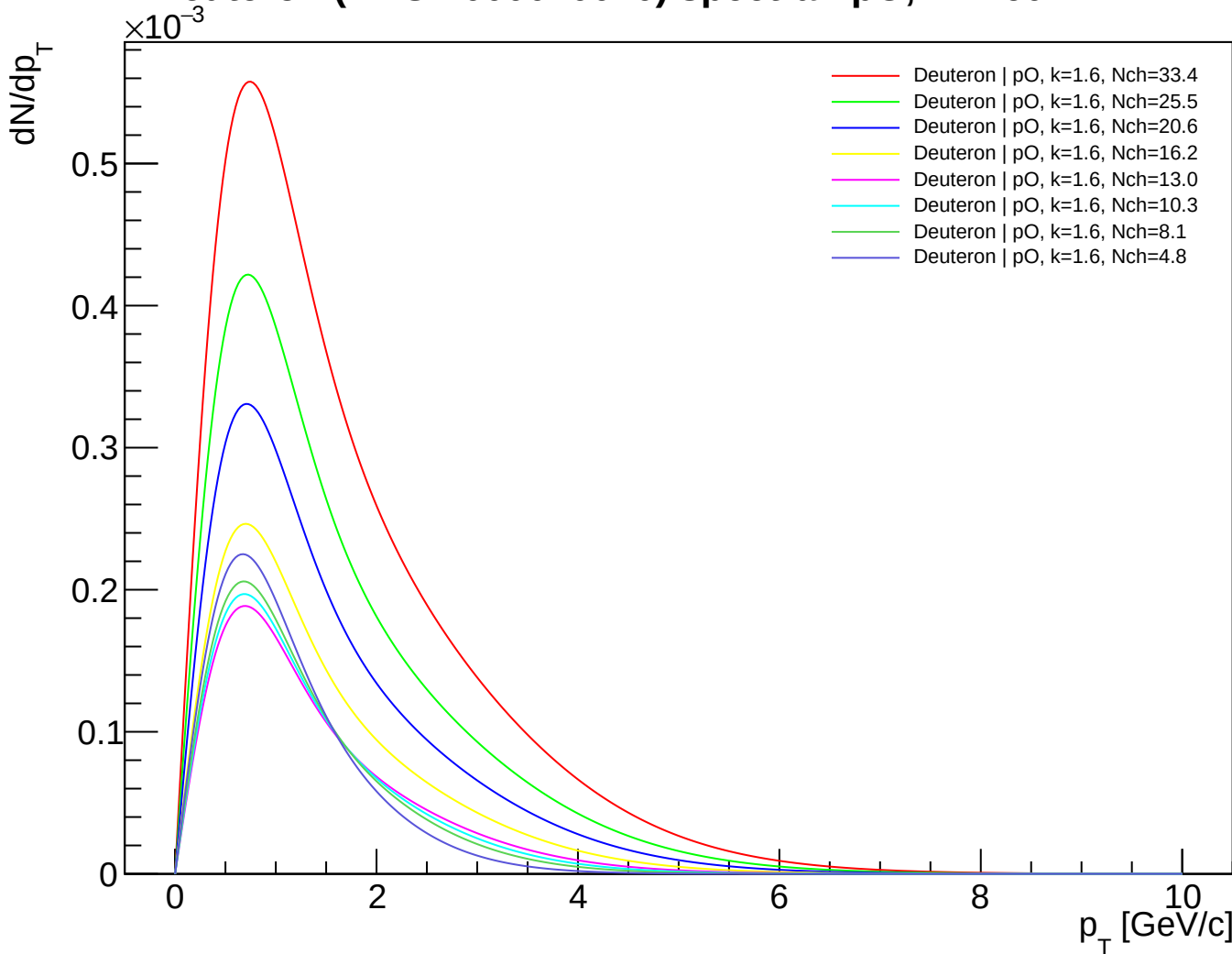
Deuteron (PDG 1000010020) spectra - pO, k=1.60
