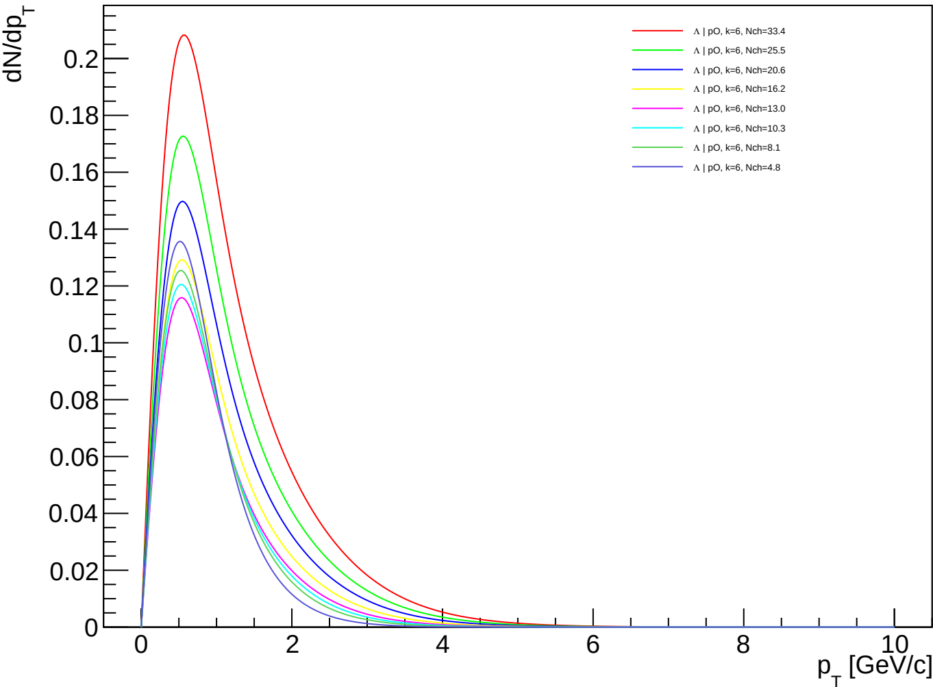
\Lambda (PDG 3122) spectra - pO, k=6.00
