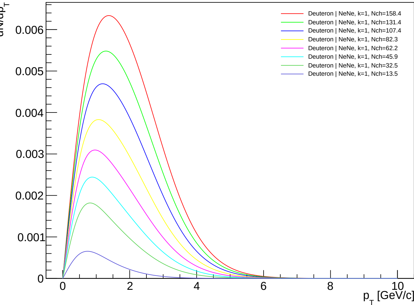
Deuteron (PDG 1000010020) spectra - NeNe, k=1.00
