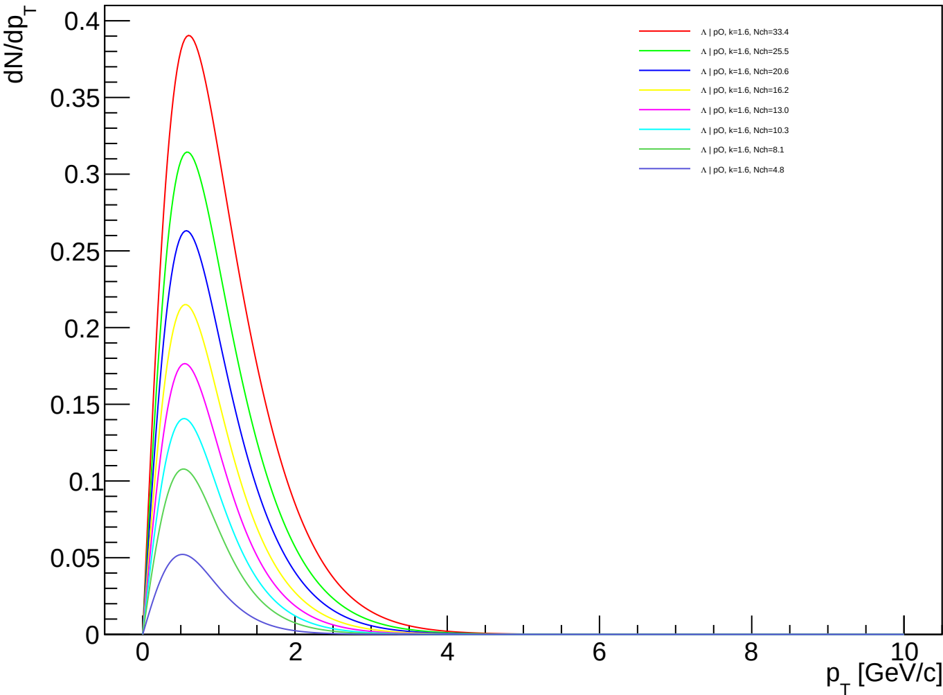
\Lambda (PDG 3122) spectra - pO, k=1.60
