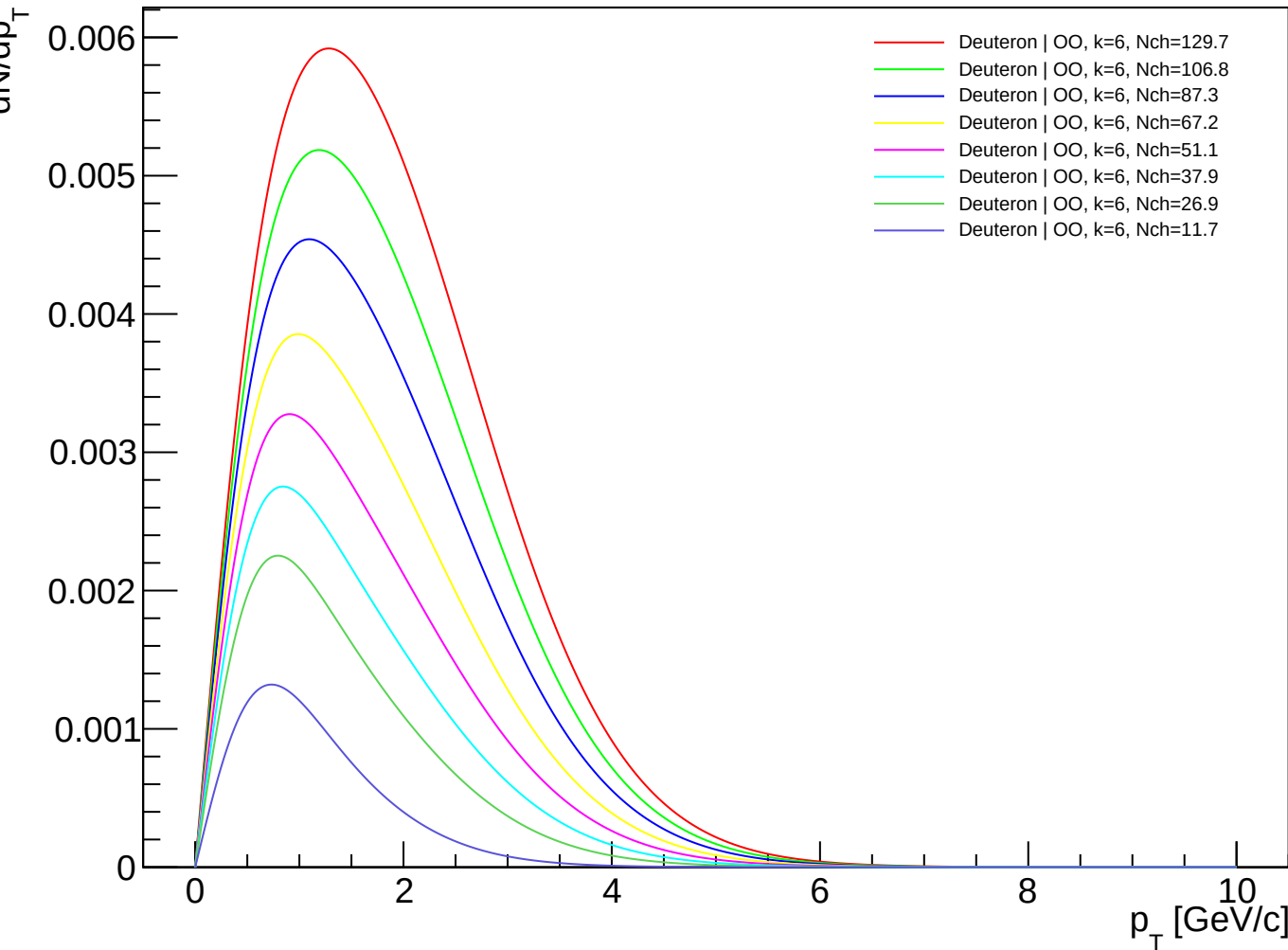
Deuteron (PDG 1000010020) spectra - OO, k=6.00
