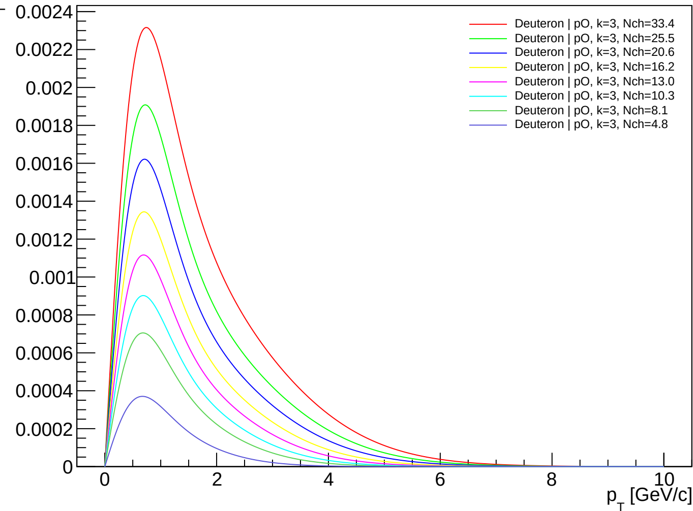
Deuteron (PDG 1000010020) spectra - pO, k=3.00
