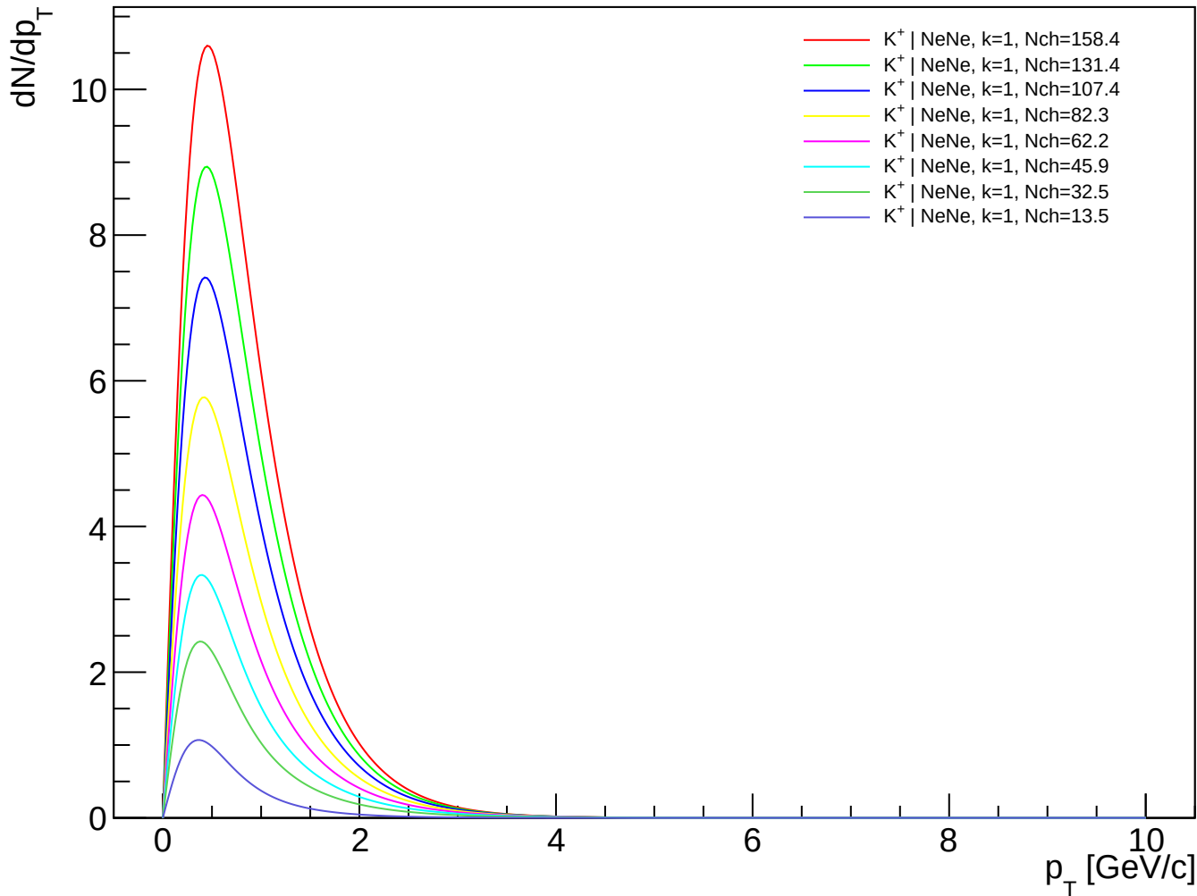
K + (PDG 321) spectra - NeNe, k=1.00
