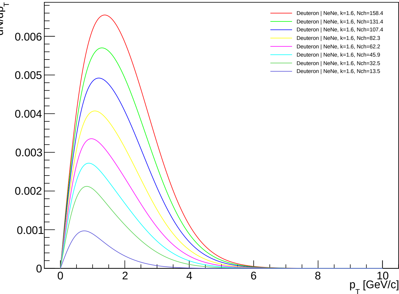
Deuteron (PDG 1000010020) spectra - NeNe, k=1.60
