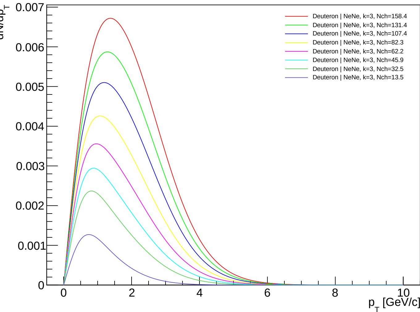
Deuteron (PDG 1000010020) spectra - NeNe, k=3.00
