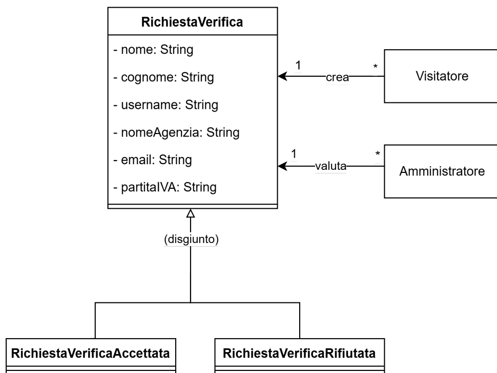
Figura 7: Richiesta Verifica e relazione con attori
