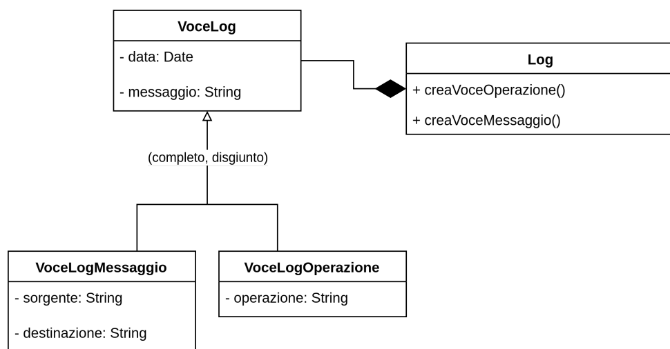
Figura 8: Struttura delle classi di Log
