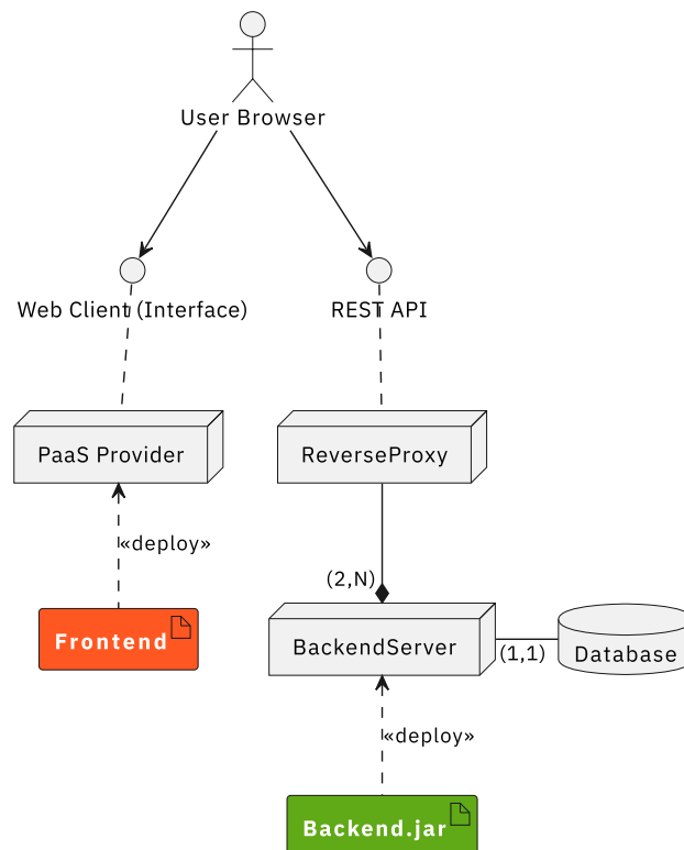
Figura 63: Schema dei target di deploy nell'ipotesi di utilizzo di PaaS 2
