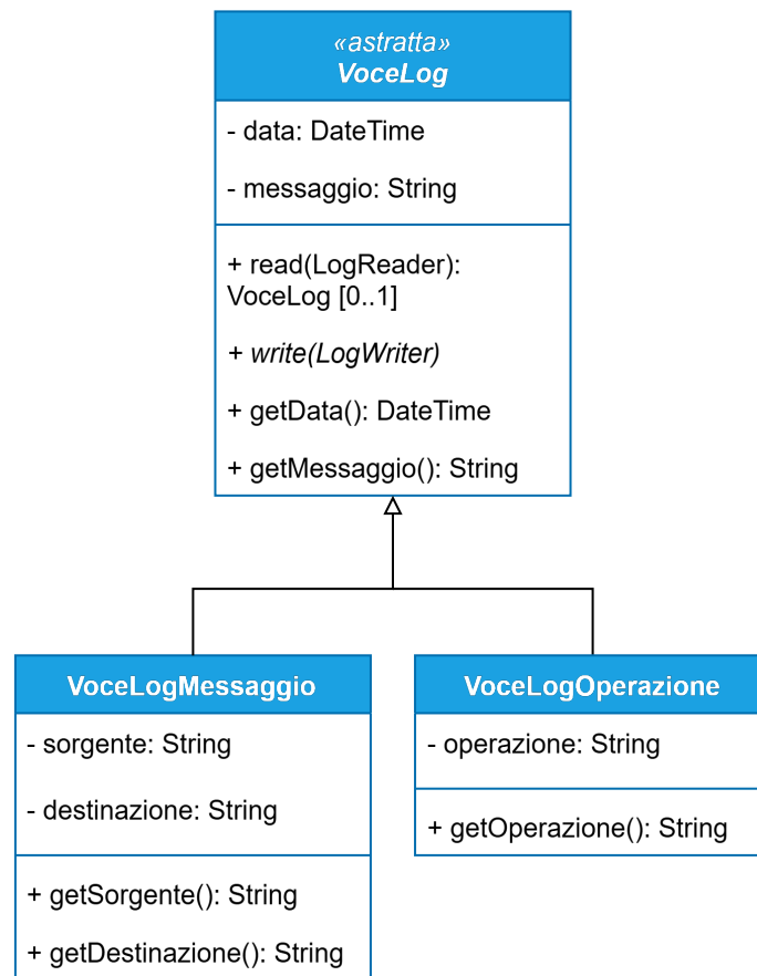
Figura 39: Struttura del dominio relativo al log
