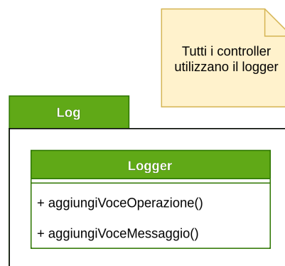
Figura 14: Diagramma delle classi relativo al Log
