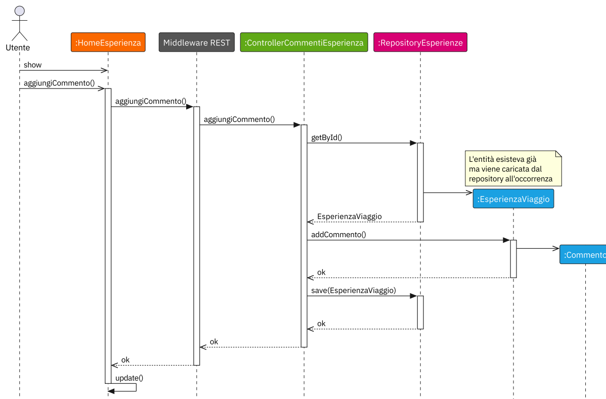
Figura 55: Interazione con un'Esperienza da parte di un Utente
