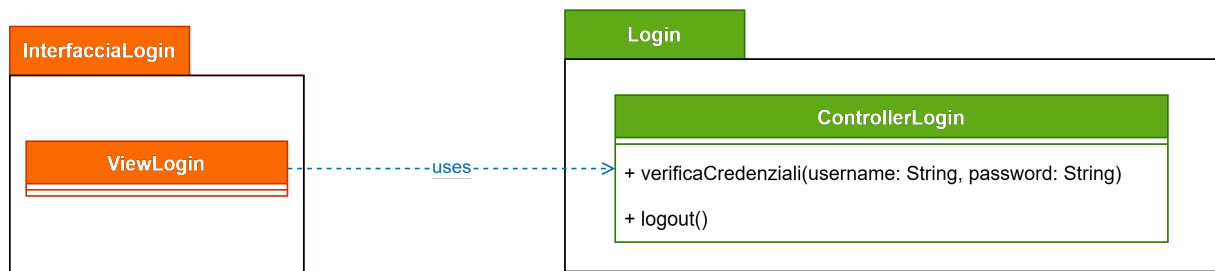
Figura 11: Diagramma delle classi relativo al login
