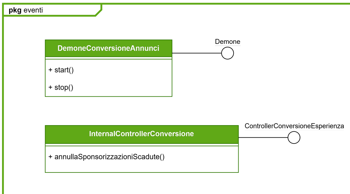
Figura 36: Struttura dei controller relativi alla scadenza della sponsorizzazione di un'esperienza di viaggio
