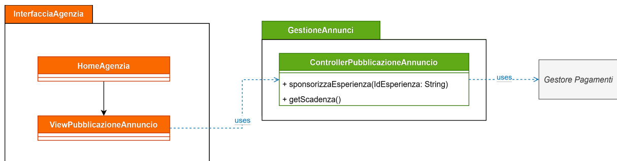
Figura 13: Diagramma delle classi relativo all'Agenzia di Viaggio
