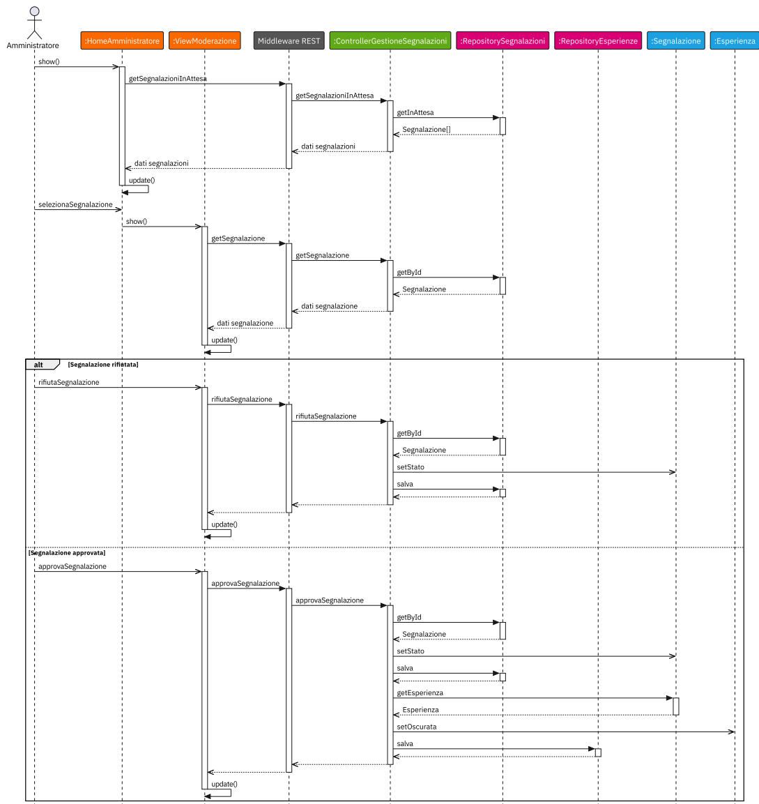
Figura 54: Approvazione o rifiuto di una segnalazione ed oscuramento dell'Esperienza di Viaggio
