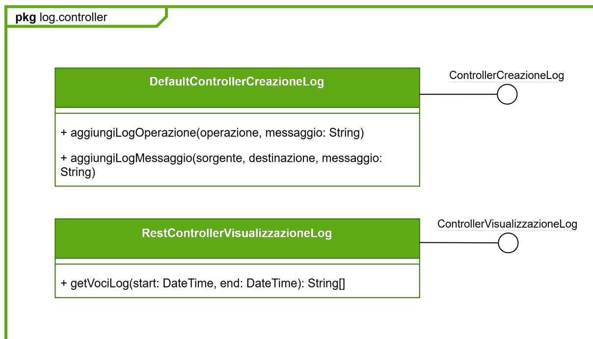
Figura 37: Struttura dei controller relativi alla lettura e scrittura del log
