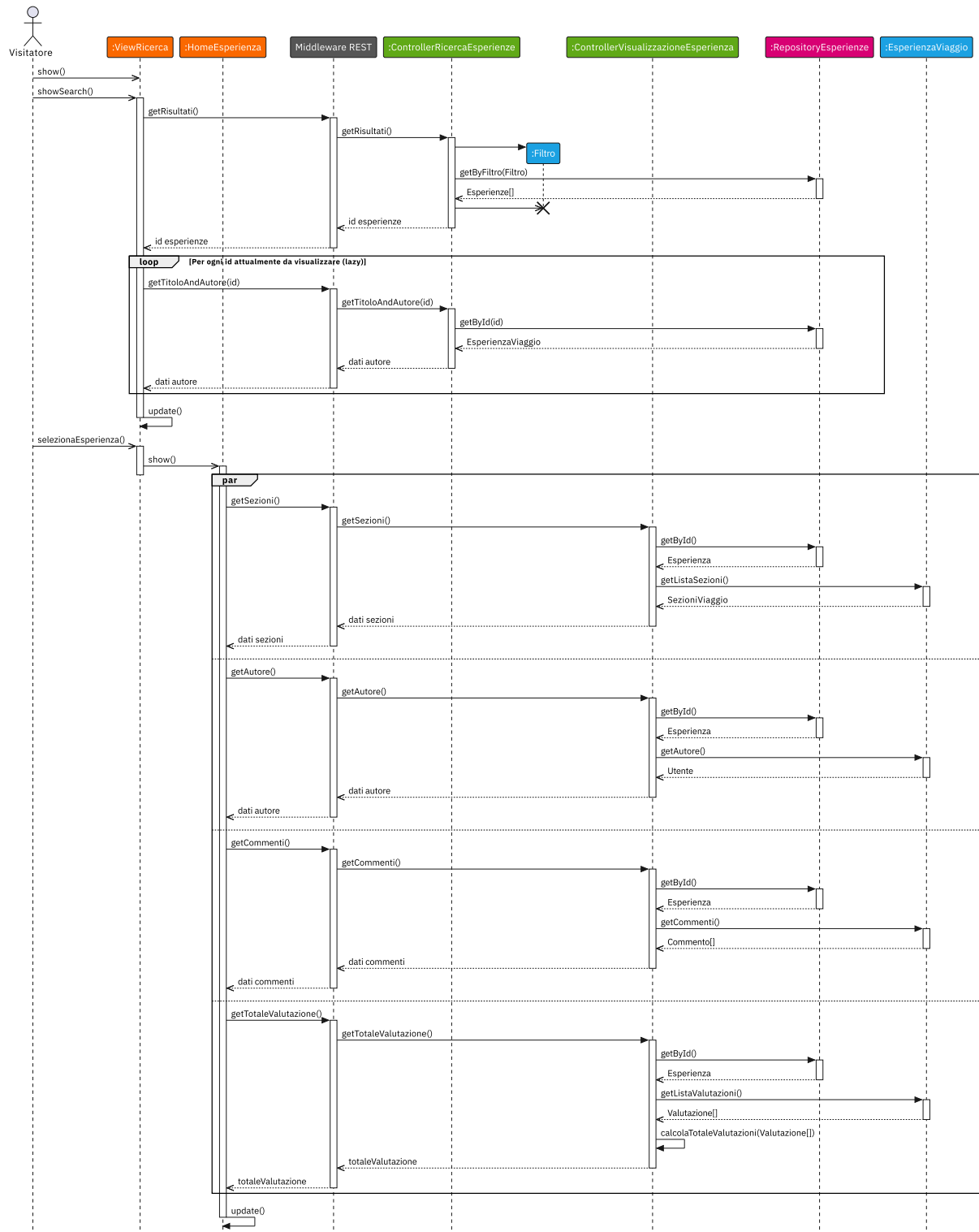
Figura 56: Ricerca delle Esperienze e visualizzazione di un'Esperienza
