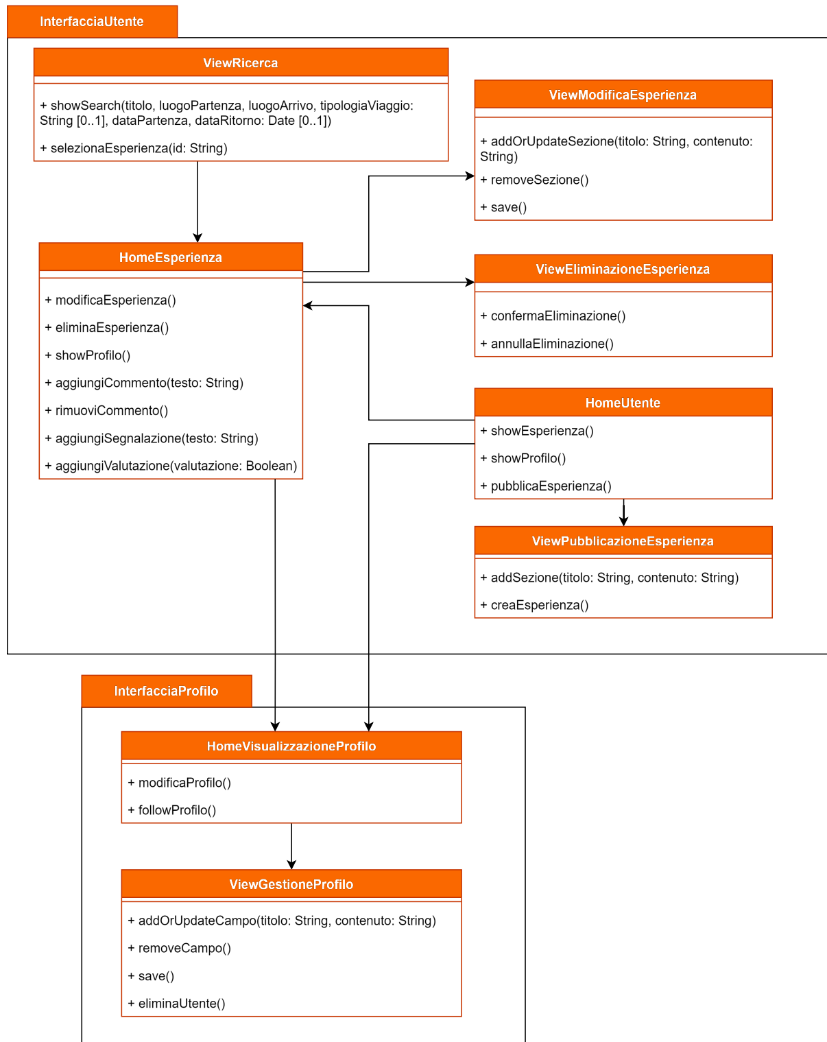
Figura 40: View visibili agli utenti
