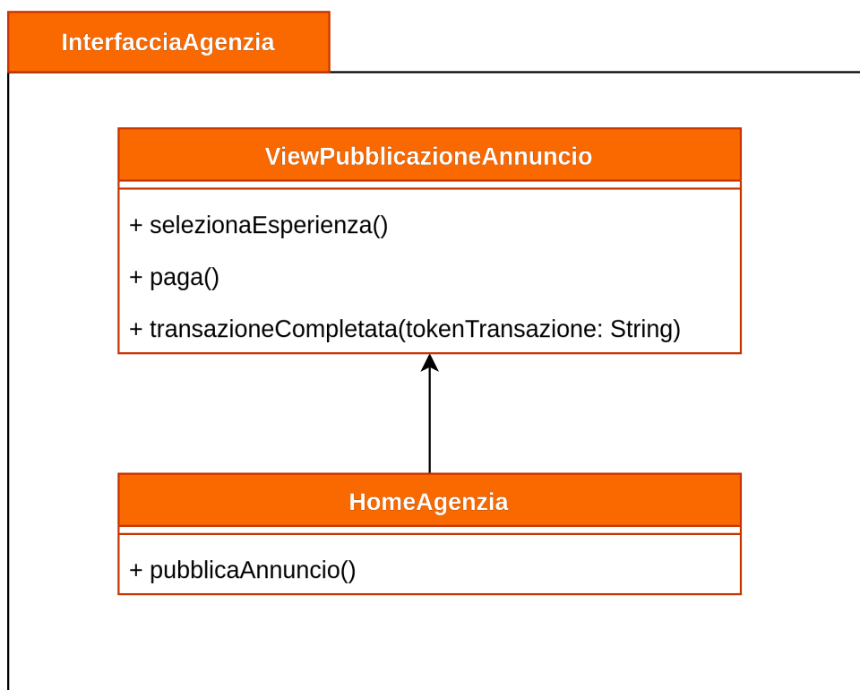
Figura 42: View visibili alle agenzie di viaggio
