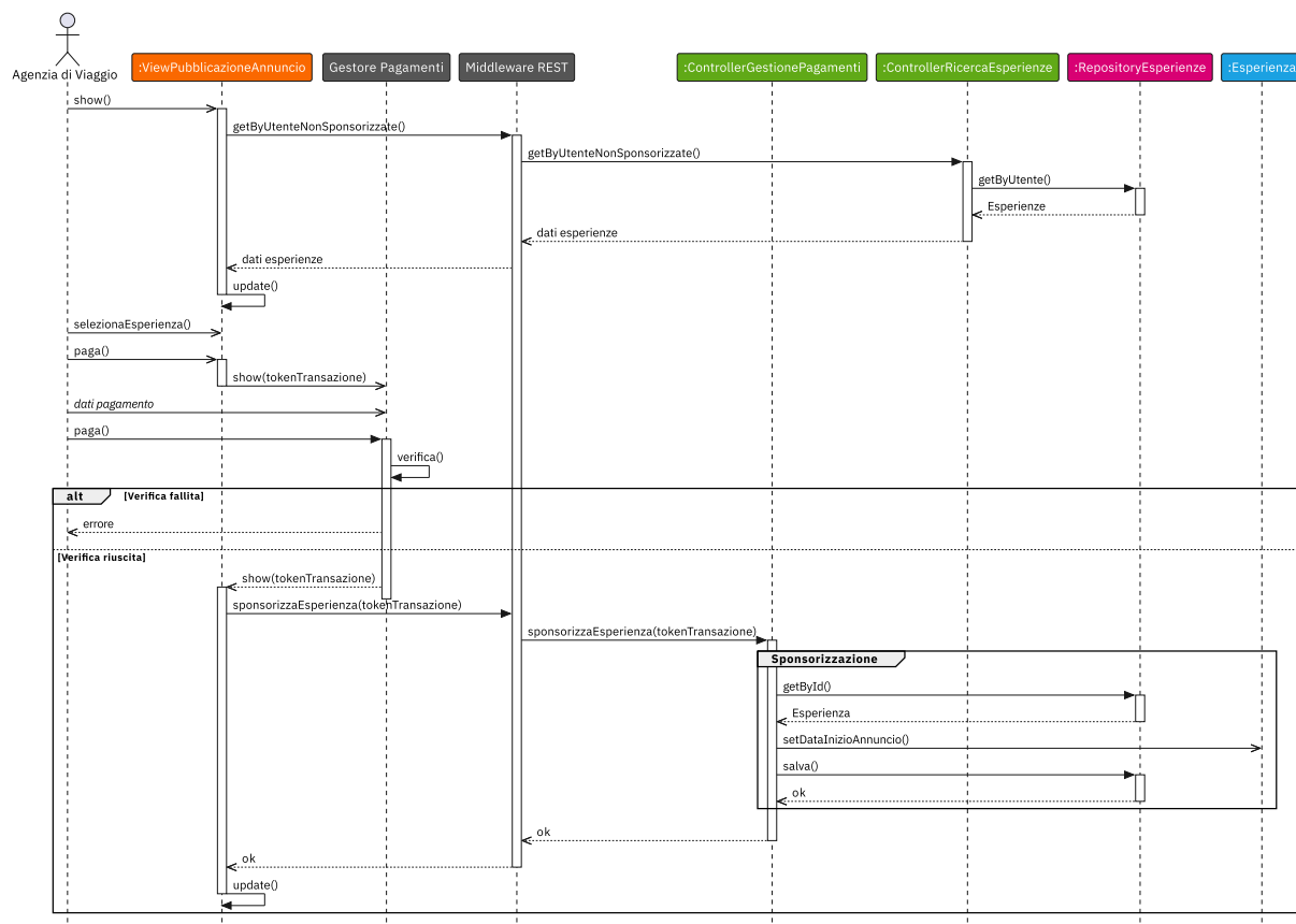
Figura 50: Creazione di un annuncio (Sponsorizzazione)
