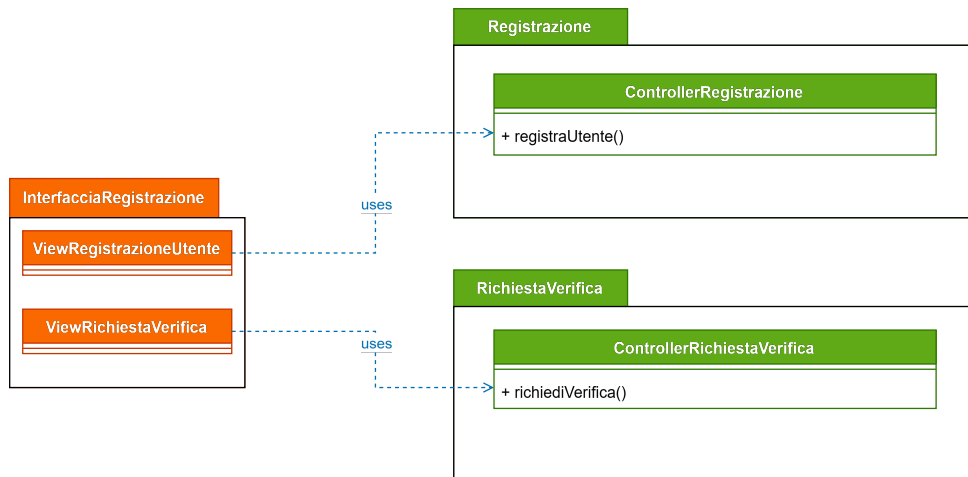
Figura 10: Diagramma delle classi relativo alla Registrazione
