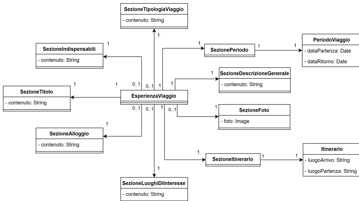
Figura 2: Relazione tra Esperienza di Viaggio e Sezioni associate
