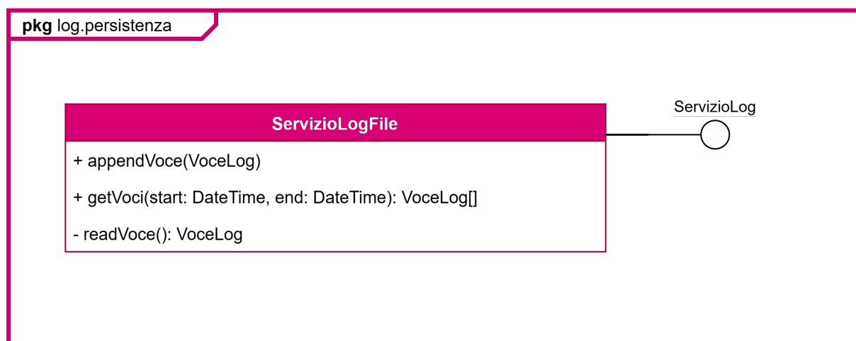
Figura 38: Struttura della persistenza relativa al log
