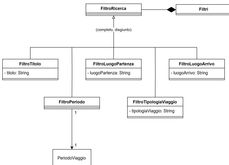
Figura 6: Generalizzazione Filtri ricerca
