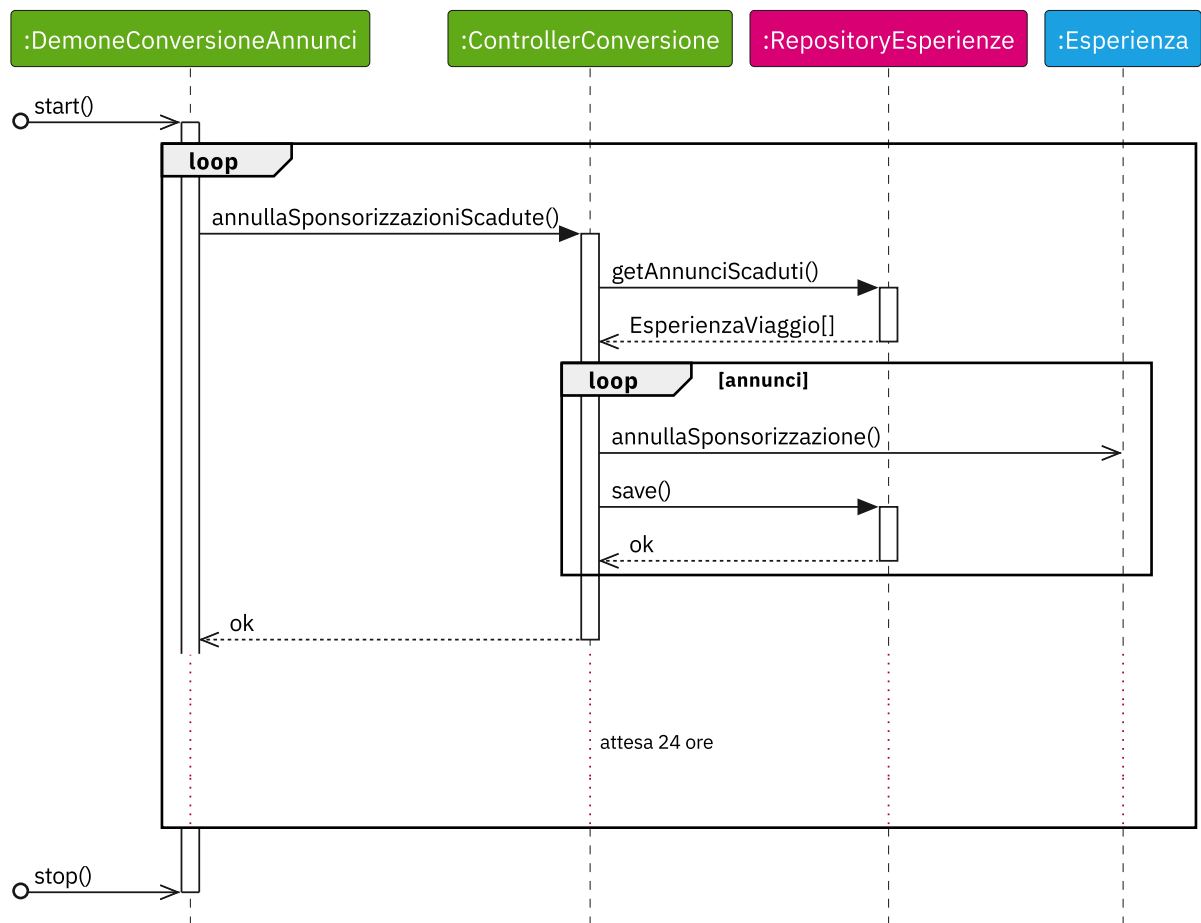
Figura 57: Processo di conversione degli annunci in esperienze di viaggio alla scadenza del periodo di sponsorizzazione
