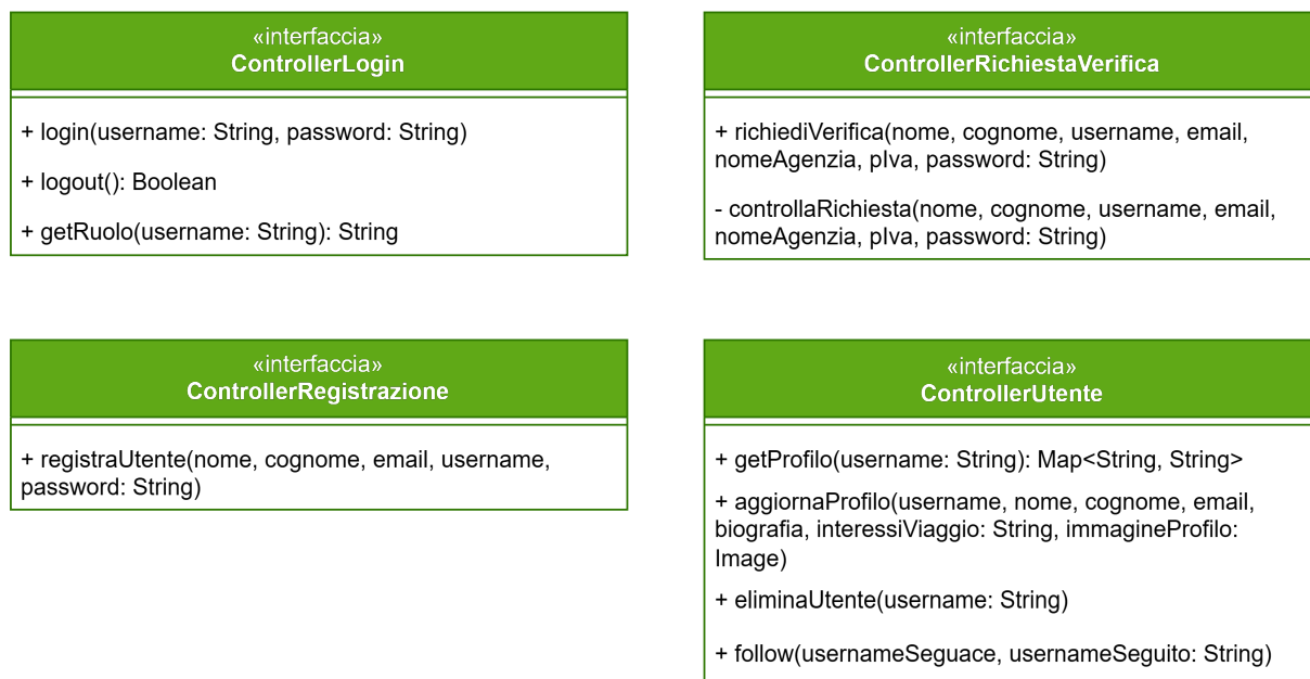
Figura 21: Interfacce dei controller relativi agli utenti
