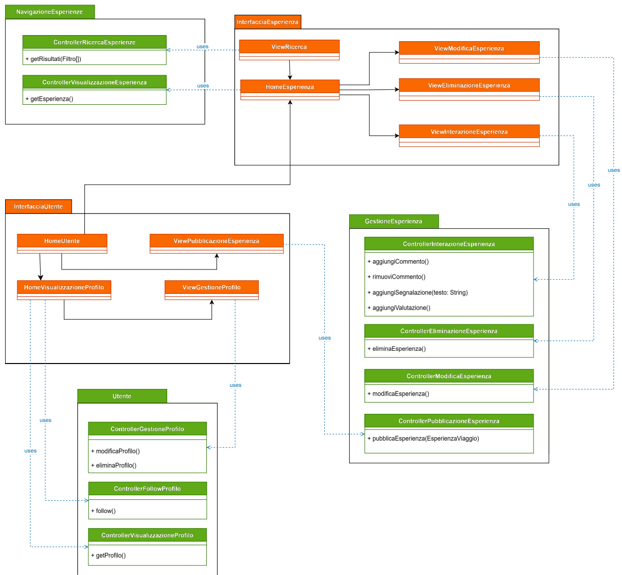
Figura 9: Diagramma delle classi relativo all'Utente e all'Esperienza di Viaggio
