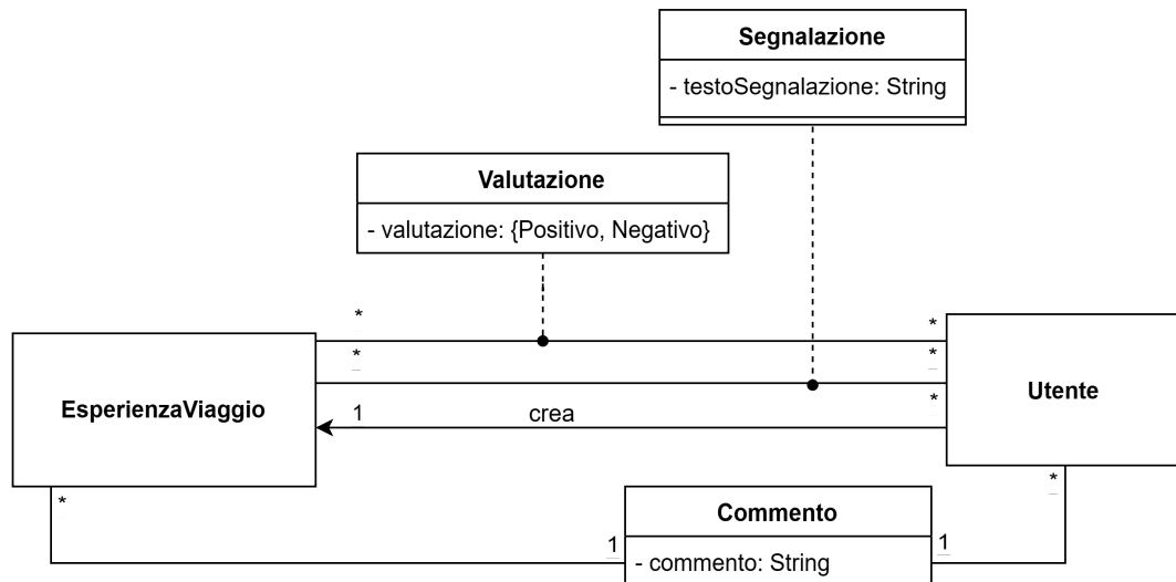
Figura 4: Relazione tra l'Utente e l'Esperienza di Viaggio
