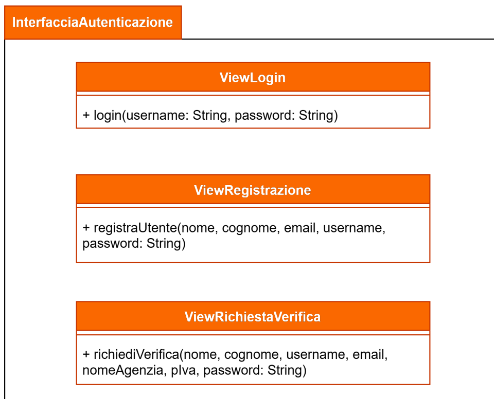
Figura 41: View relative all'autenticazione
