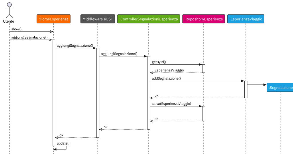
Figura 53: Creazione di una segnalazione da parte di un Utente
