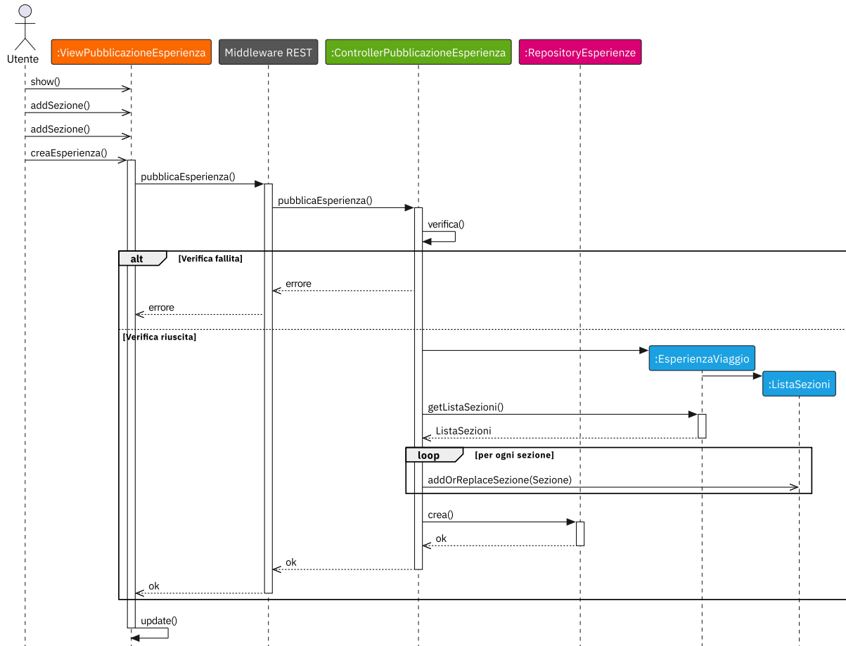
Figura 49: Creazione di un Esperienza di Viaggio da parte di un Utente
