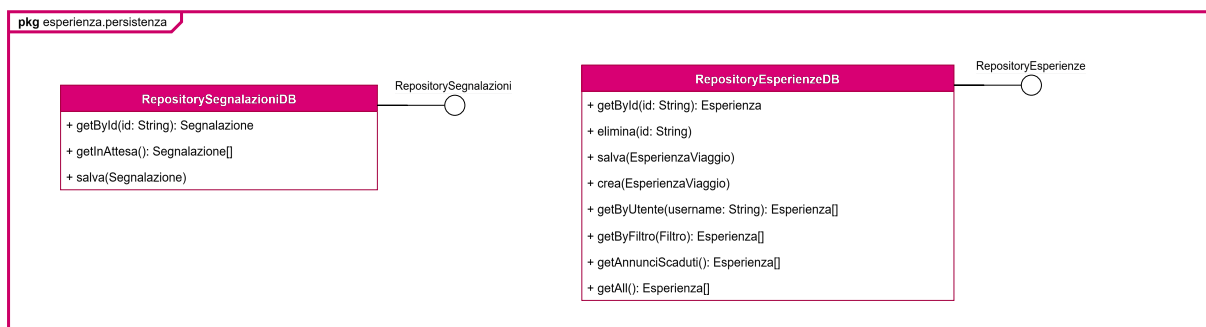
Figura 33: Struttura della persistenza relativa alla gestione delle esperienze
