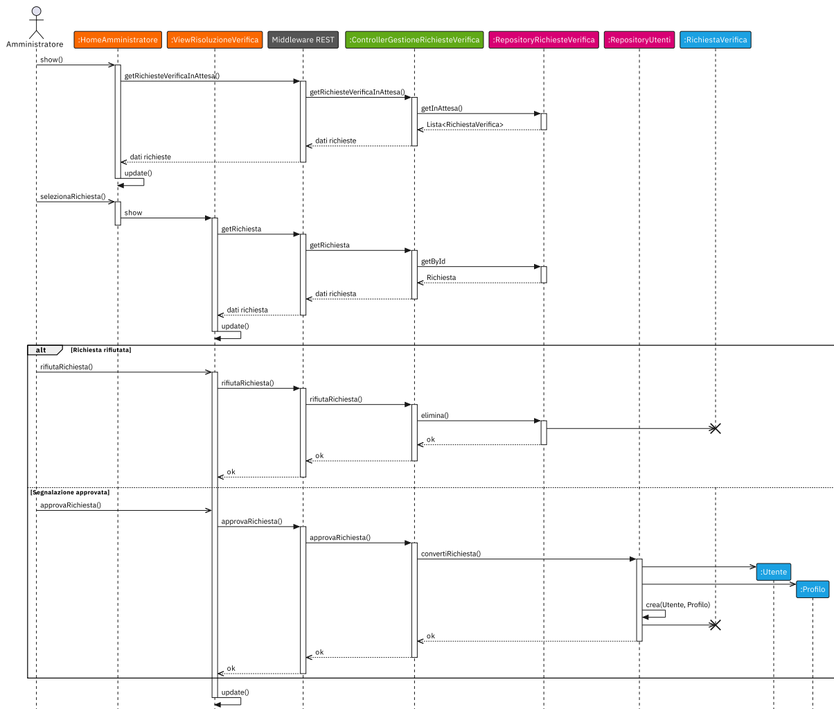
Figura 52: Approvazione o rifiuto da parte dell'amministratore di una richiesta di verifica già creata
