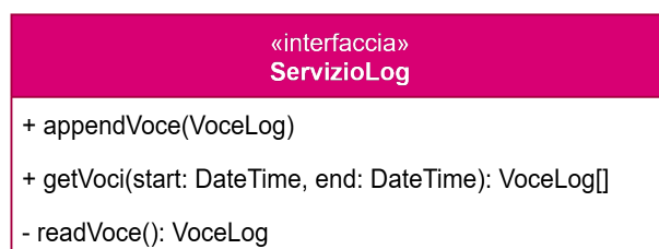
Figura 28: Interfaccia del repository relativo alla scrittura e lettura del Log
