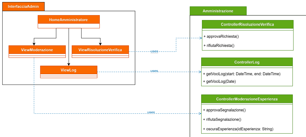
Figura 12: Diagramma delle classi relativo all'Amministratore
