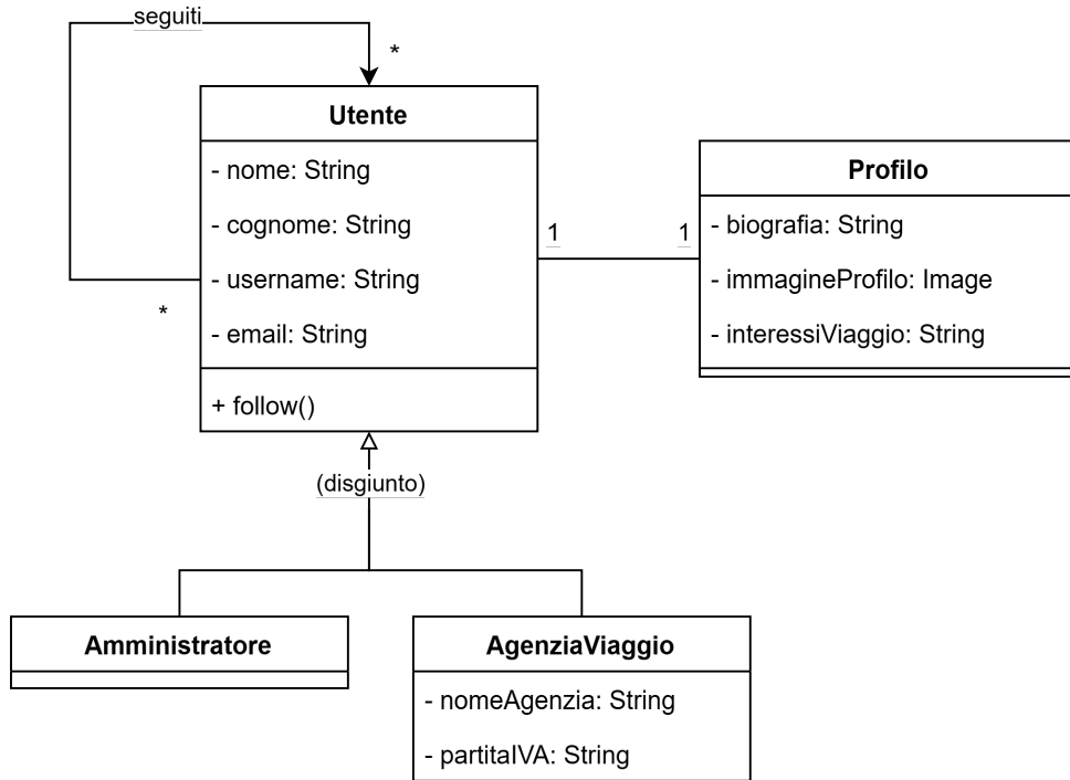
Figura 1: Relazione tra le utenze dell'applicazione
