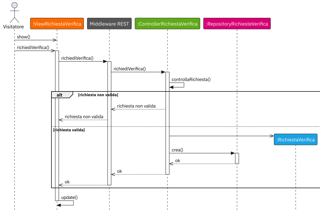
Figura 51: Creazione di una RichiestaVerifica da parte di un Visitatore
