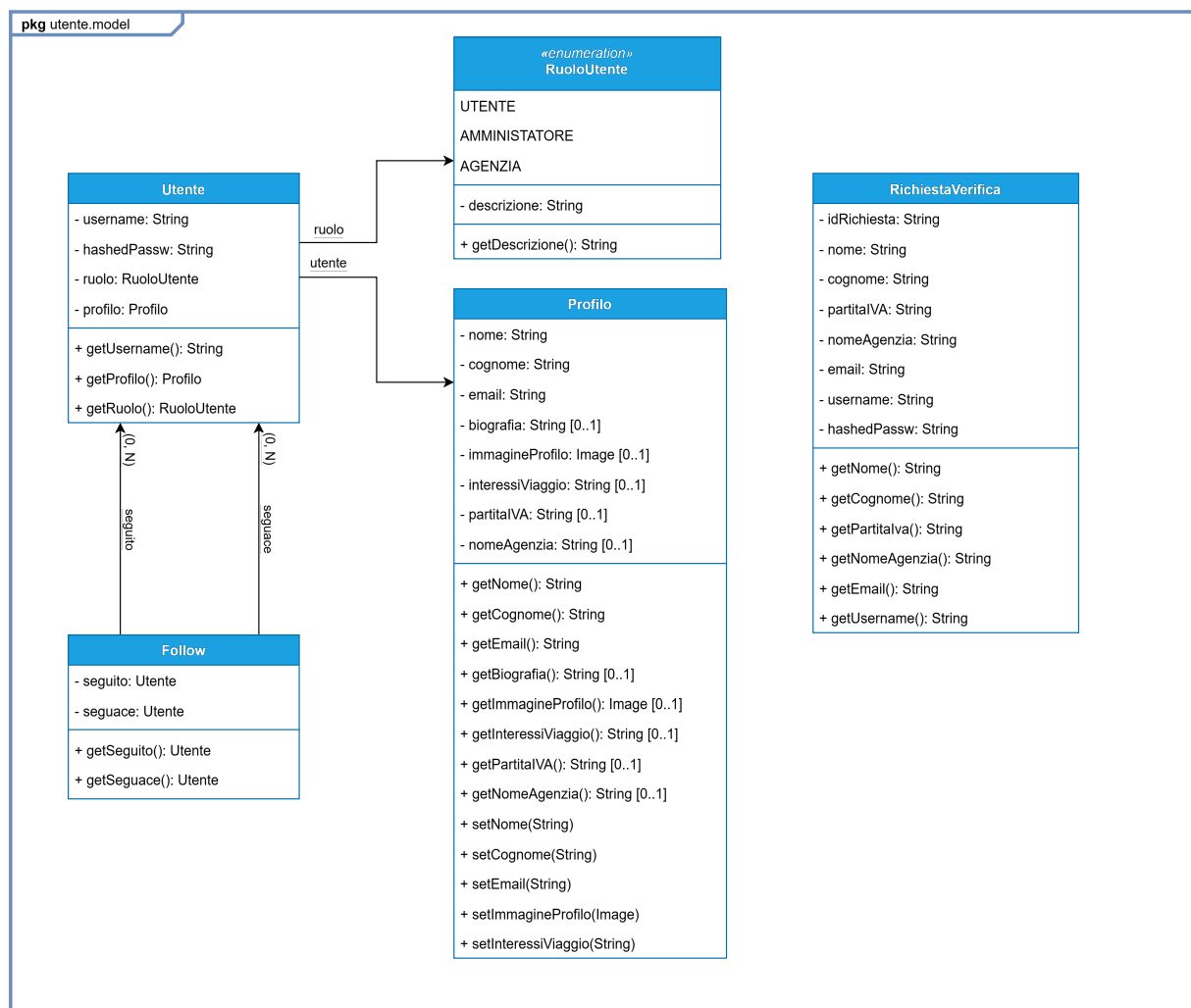
Figura 31: Struttura del dominio relativo agli utenti
