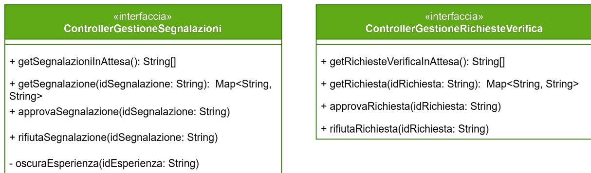
Figura 25: Interfacce dei controller relativi all'Amministratore
