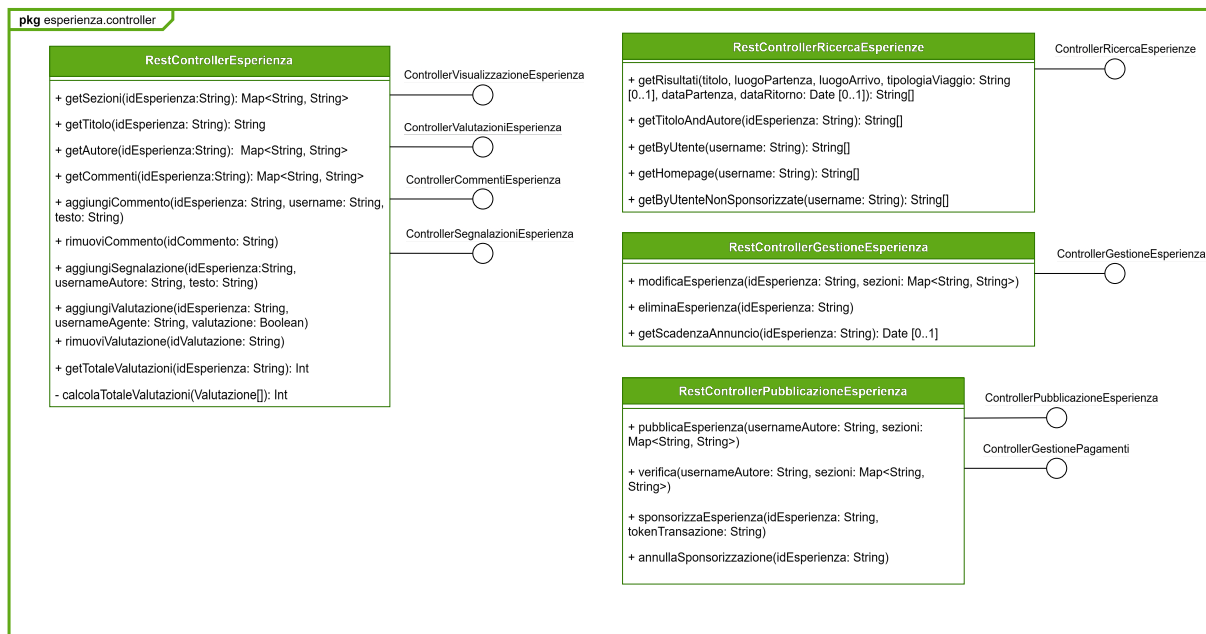
Figura 32: Struttura dei controller relativi alla gestione delle esperienze
