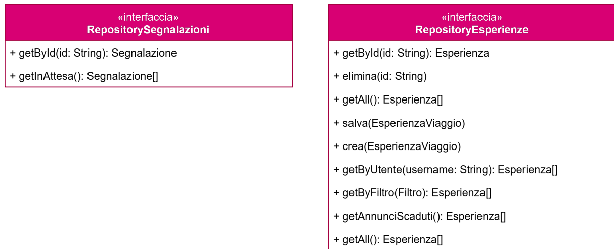
Figura 24: Interfacce dei repository relativi alle Esperienze
