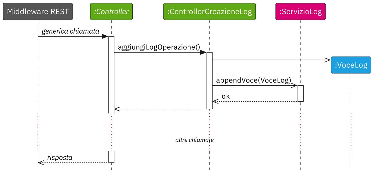
Figura 58: Interazione tra un generico Controller e il sottosistema di log
