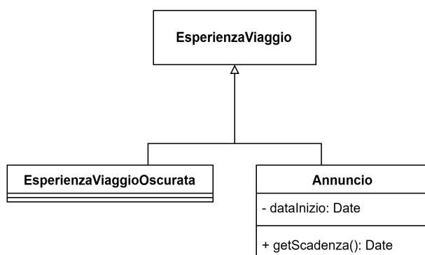
Figura 3: Generalizzazione Esperienza di Viaggio
