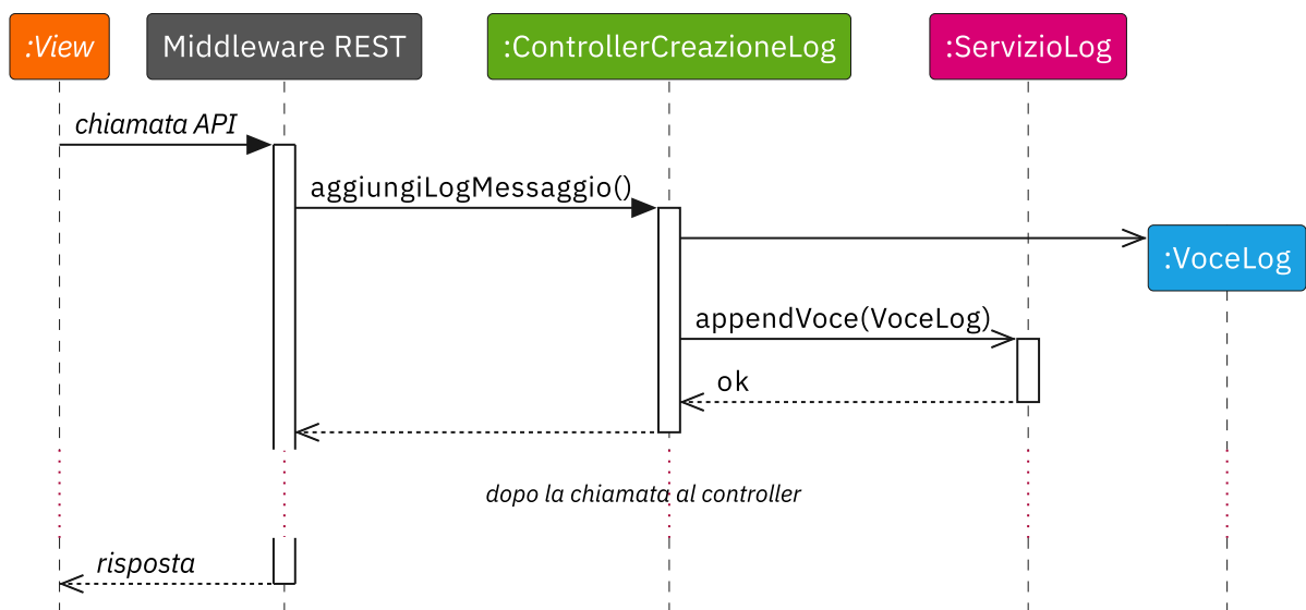
Figura 59: Interazione tra il Middleware REST e il sottosistema di log
