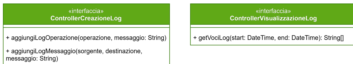
Figura 27: Interfacce dei controller relativi alla scrittura e lettura del Log
