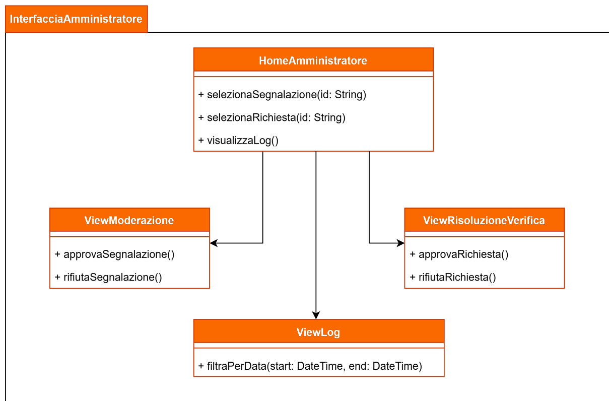
Figura 43: View visibili all'Amministratore
