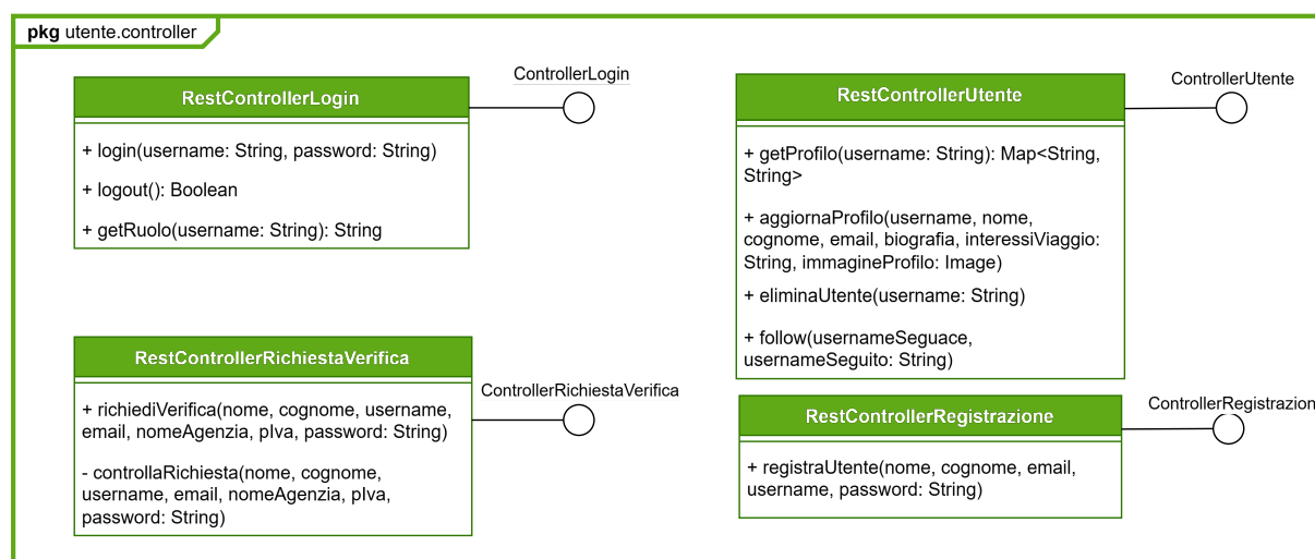
Figura 29: Struttura dei controller relativi alla gestione degli utenti
