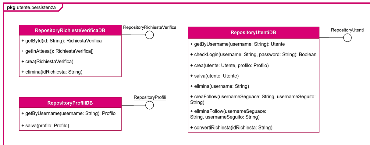
Figura 30: Struttura della persistenza relativa alla gestione degli utenti
