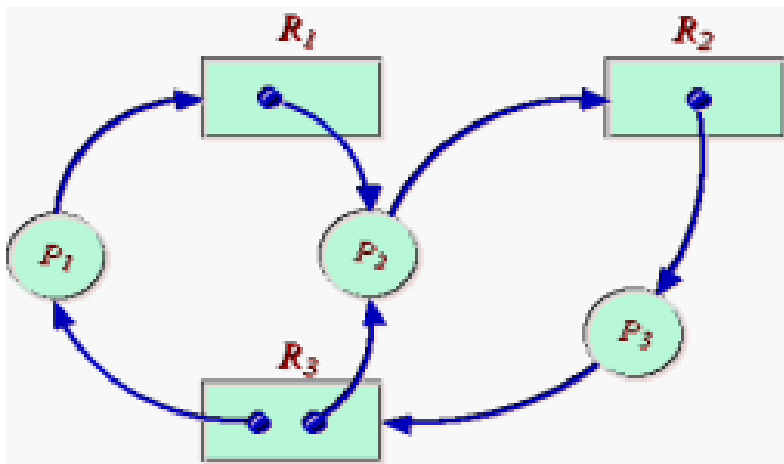
有环有死锁
