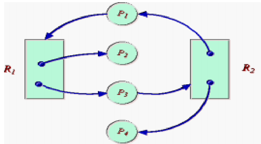
有环无死锁
