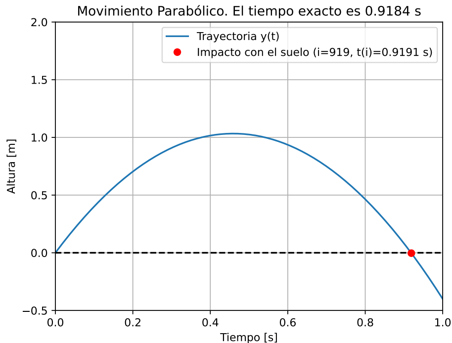
Figura 1: Gráfica de la altura y en función del tiempo t para y_0 = 0 m, v_0 = 4,5 m/s.
