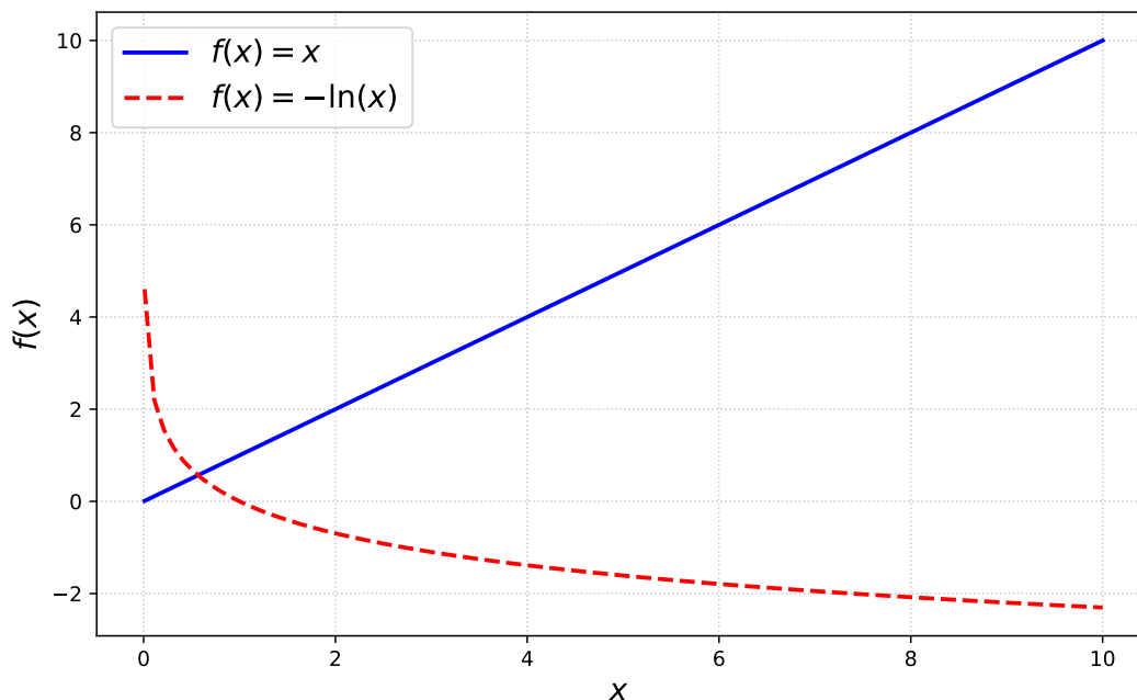
Figura 3: Gráfica de x y -\ln(x) vs x .
