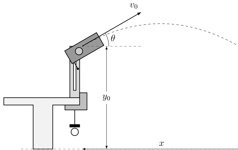
Figura 1: Montaje de laboratorio para lanzamiento de proyectiles con altura inicial y_0 .
