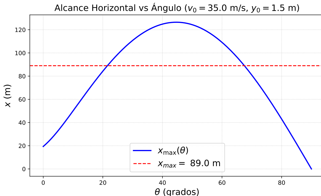
Figura 2: Alcance máximo en función del ángulo de lanzamiento.
