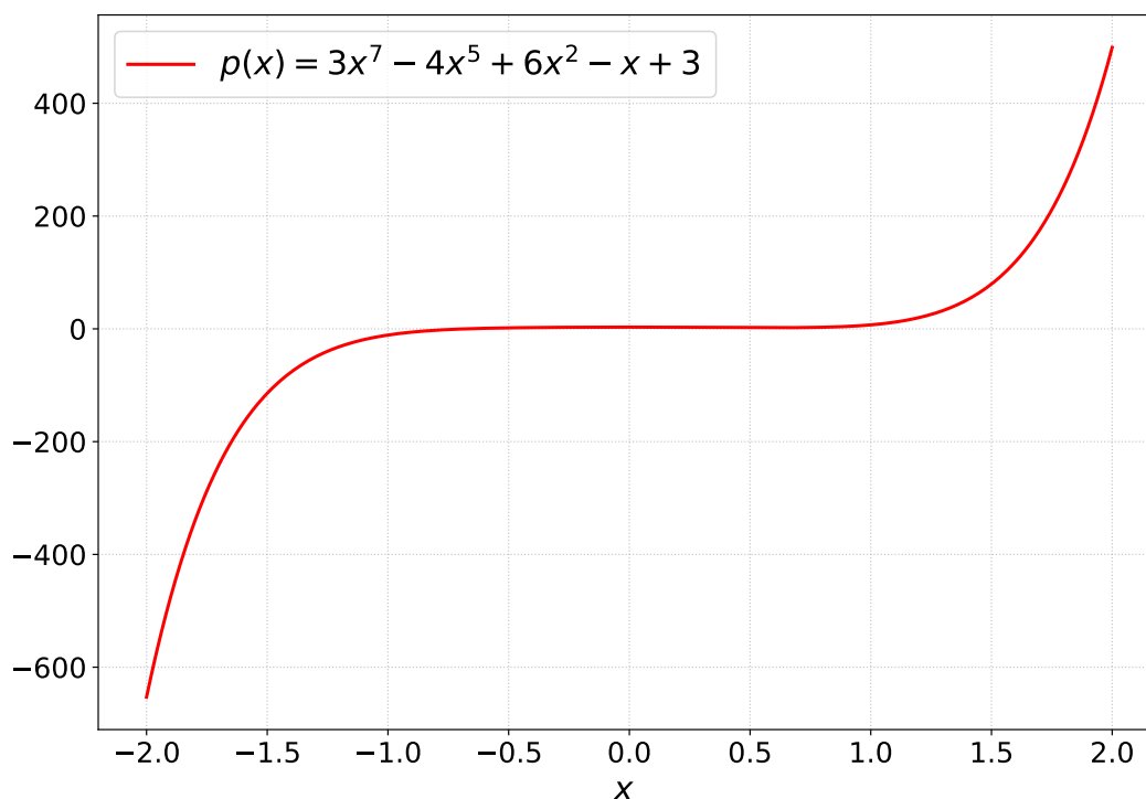
Figura 4: Gráfica de p(x) = 3x^7 - 4x^5 + 6x^2 - x + 3 vs x .
