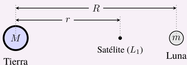
Figura 5: Esquema del sistema Tierra-Luna y la posición del punto L_1 .
